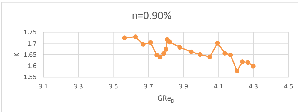
Figura 50 Grafica del factor de fricción en función ( K ) del número de Reynolds Generalizado ( GRe_D ) para la Tabla 2 n=0.90\%
