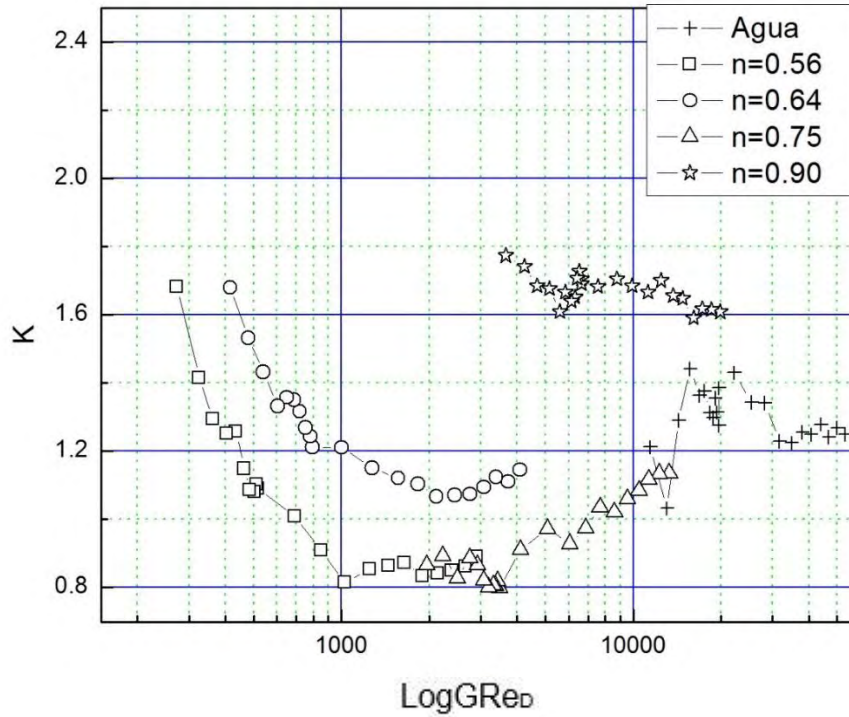
Figura 28 Se observa el Factor de fricción ( f ) en función del número de Reynolds ( GRe_D ) de varias concentración de CMC (1%, 2%, 3% y 4%) en peso, y fluido newtoniano (agua). Para una válvula de esfera de una pulgada.
