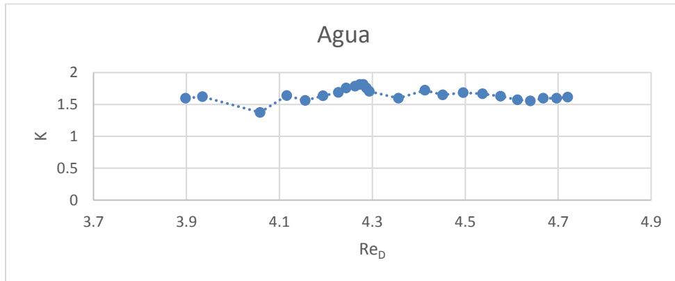
Figura 30 Grafica del factor de fricción en función (k) del número de Reynolds (Re D ) para la Tabla 1 Agua
