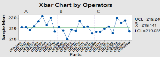
Imagen B.2 Análisis gráfico ANOVA del estudio R & R para el voltaje entre la Línea 1 y Línea 2 con una capacidad de carga eléctrica al 75%.
