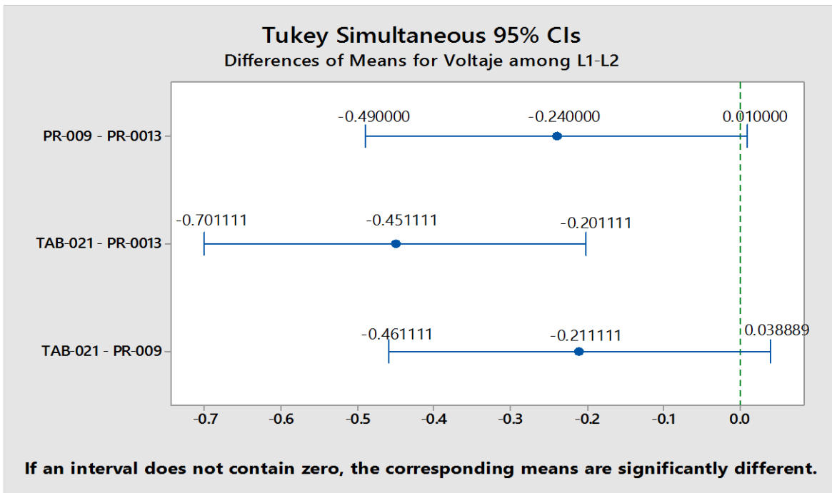
Gráfico 3.25 Comparativo de intervalos de confianza donde se tiene un 95% de certeza que los promedios del voltaje entre L1 y L2 son significativamente diferentes ya que, para el intervalo de TAB-021 – PR-0013 no contienen al cero.
