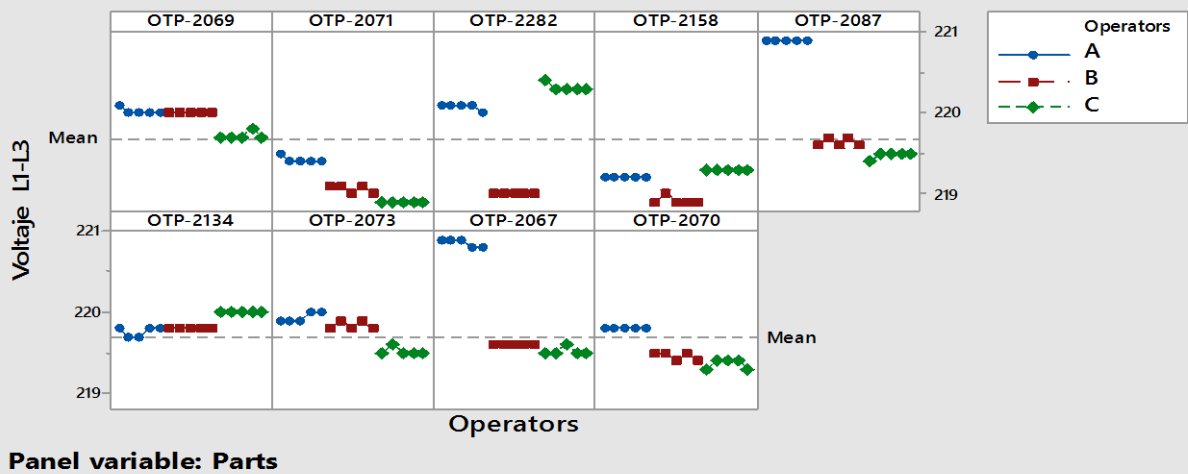
Imagen B.6 Gráfica de corridas para partes y operadores relacionadas al voltaje entre las Líneas 1 y 3 con una capacidad de carga en el banco resistivo del 75%.
