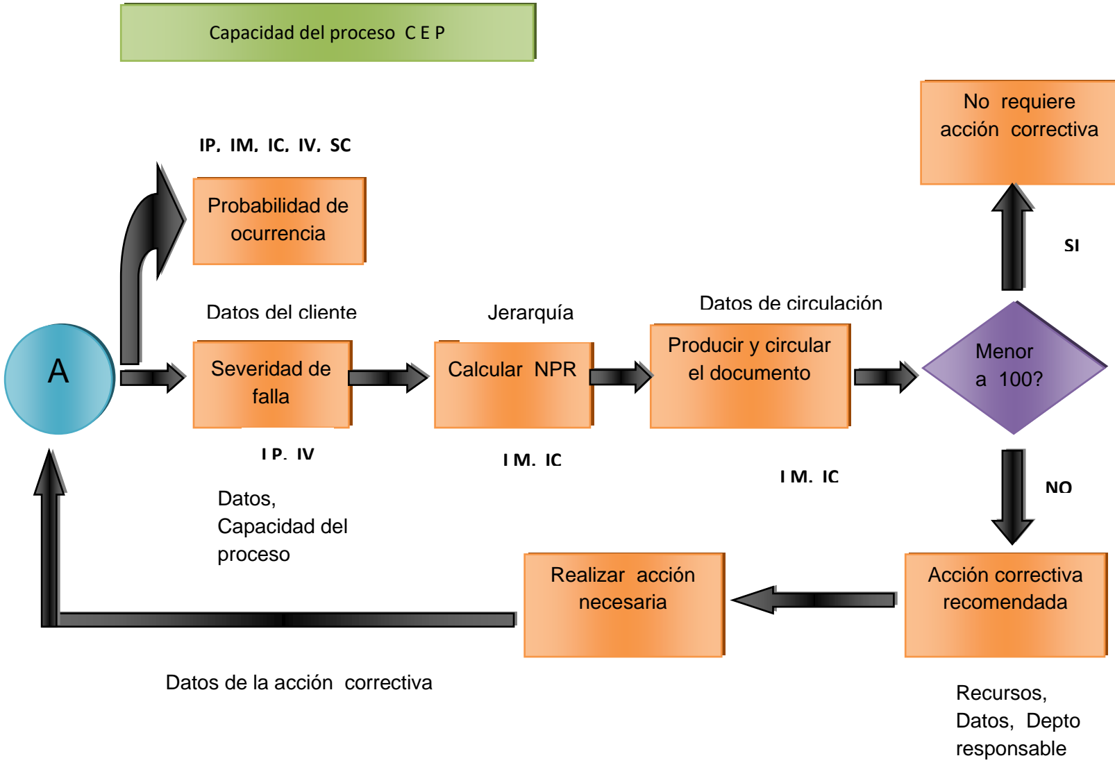
Imagen 3.7 Diagrama de flujo para la elaboración de un AMEFP 9
