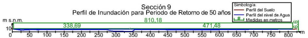
Ilustración 89.- Perfil de inundación para periodo de retorno de 50 años en la sección 9.
