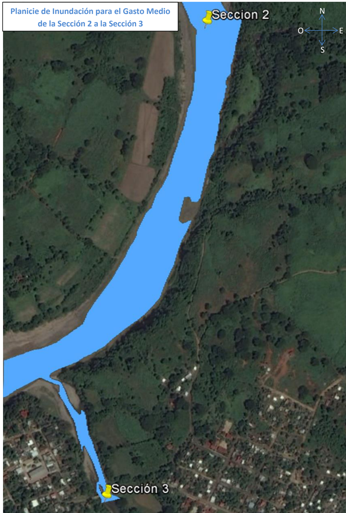
Ilustración 92.- Planicie de inundación para gasto medio, sección 2 a sección 3.
