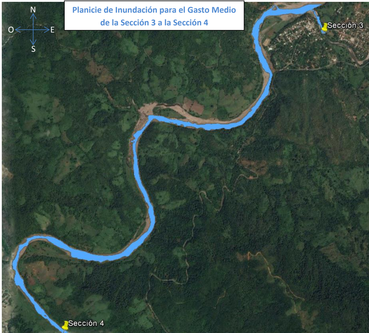
Ilustración 93.- Planicie de inundación para gasto medio, sección 3 a sección 4.
