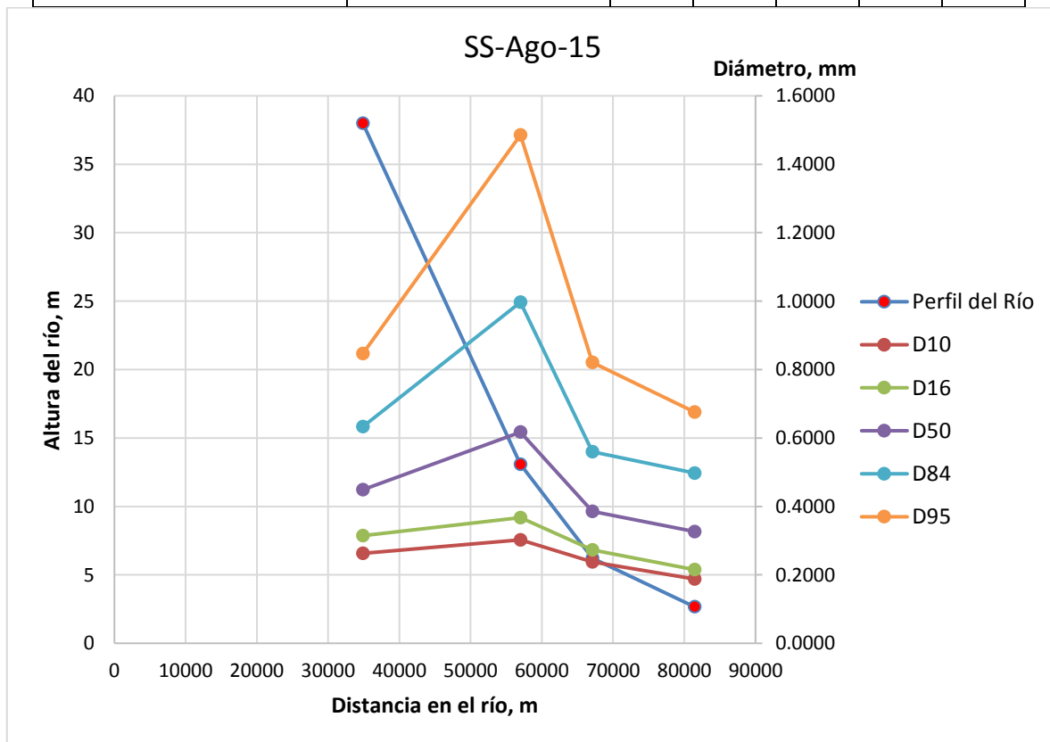
Ilustración 17.- Sedimento en suspensión de agosto 2015.
