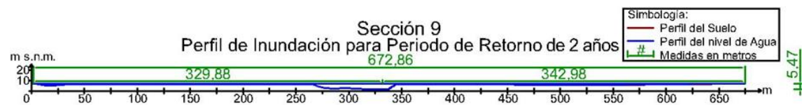
Ilustración 85.- Perfil de inundación para periodo de retorno de 2 años en la sección 9.
