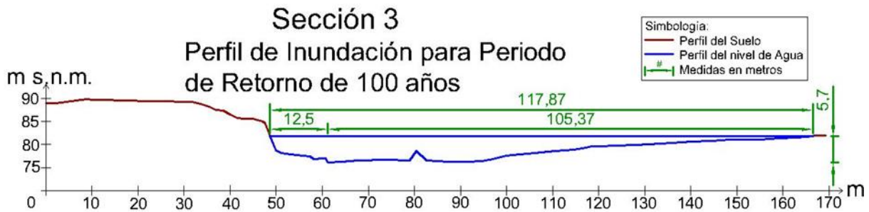
Ilustración 48.- Perfil de inundación para periodo de retorno de 100 años en la sección 3.
