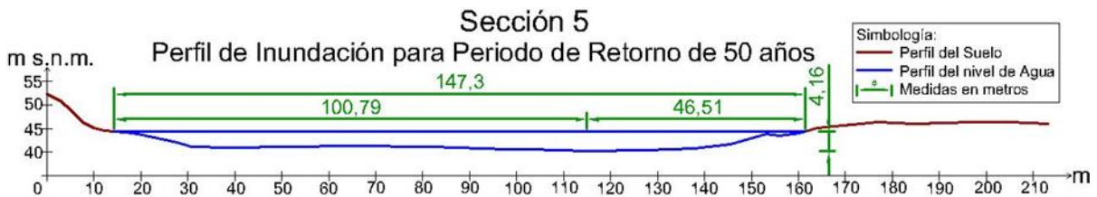
Ilustración 61.- Perfil de inundación para periodo de retorno de 50 años en la sección 5.
