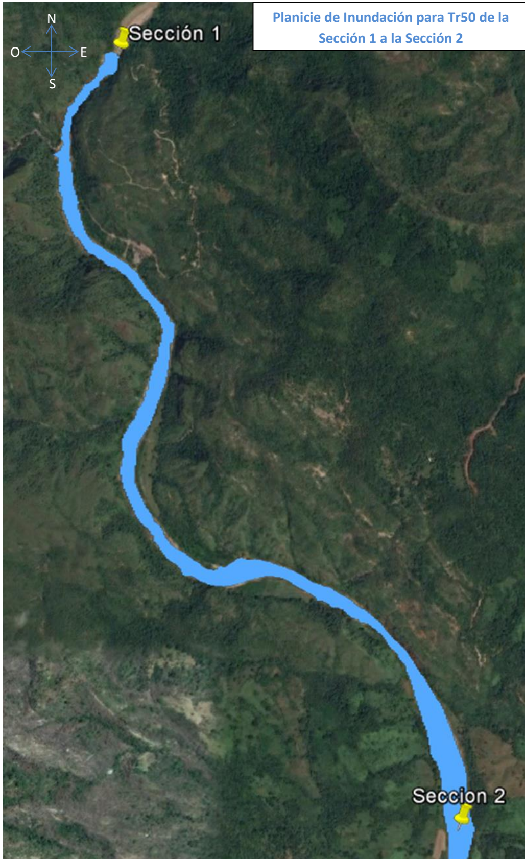
Ilustración 131.- Planicie de inundación para Tr50, sección 1 a sección 2.
