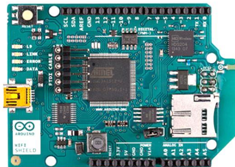
Ilustración 65 Shield Wifi de Arduino
