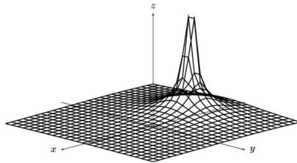
Ilustración 45 Campo potencial parabólico de un obstáculo
