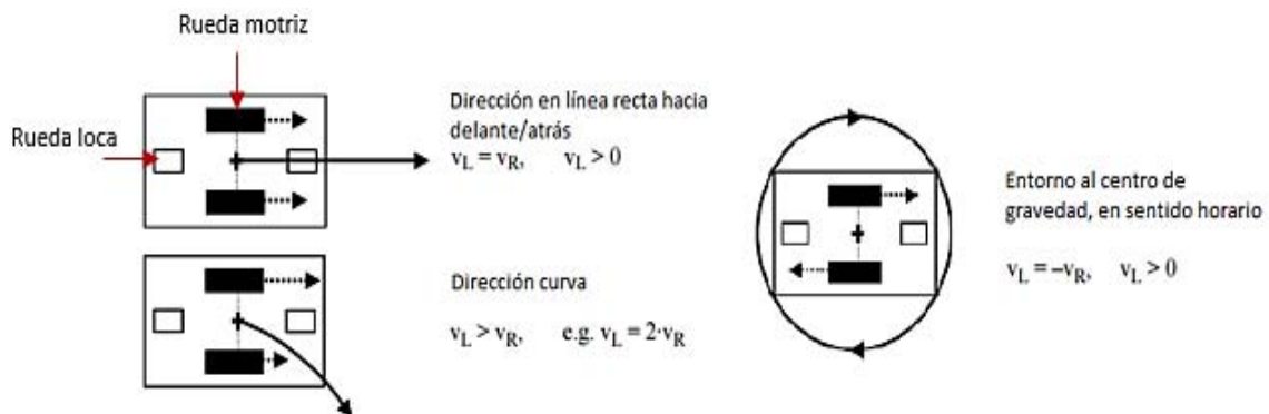
Ilustración 14 Configuración diferencial [16]
