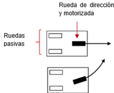
Ilustración 13 Triciclo clásico [16]
