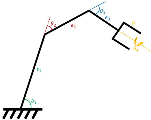
Ilustración 25 Definición del manipulador serial con base en sus variables
