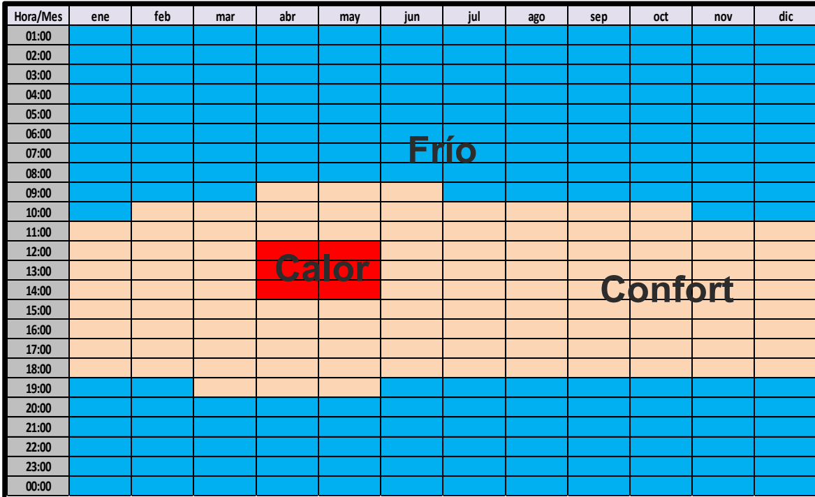
Figura 4.5 Diagrama de isorrequerimientos para Texcoco, México Fuente: Elaboración propia mediante datos de las cartas bioclimáticas mensuales de Olgyay
