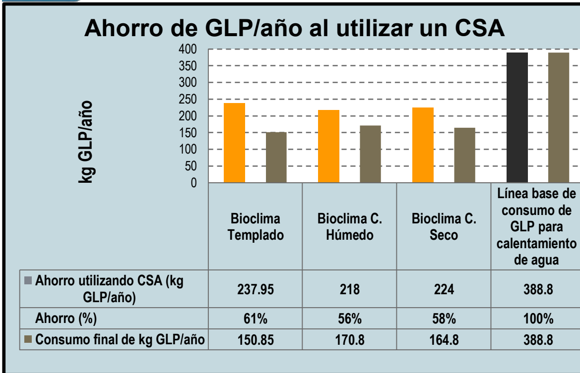
Gráfica 5.6 Ahorro de kg GLP/año en los casos de estudio, utilizando calentador solar plano comparado con el consumo de gas por calentamiento de agua definido por la línea base Fuente: Elaboración propia considerando: *Líneas base para la vivienda sustentable en México, Informe Técnico, Banco Mundial (Morillón, 2009)
