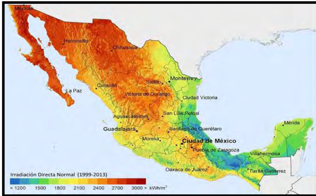
Figura 2.3 Irradiación directa normal incidente en la República Mexicana, período 1999 – 2013 13
