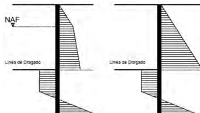
Figura 3.5 Distribución de presiones de una tablestaca empotrada en material arcilloso
