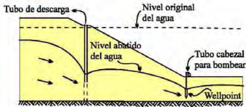
Figura 2.6 Desagüe de una excavación profunda por medio de pozos profundos y pozos punta
