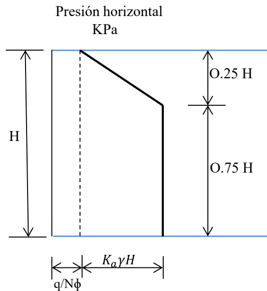
Figura 4.3 Criterio de Peck (1969)
