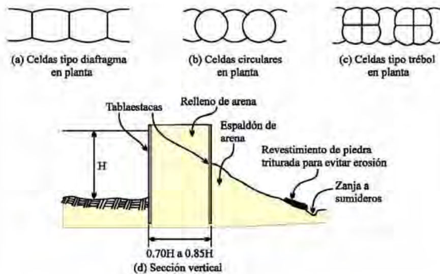
Figura 3.9 Ataguía celular de tablaestacas
