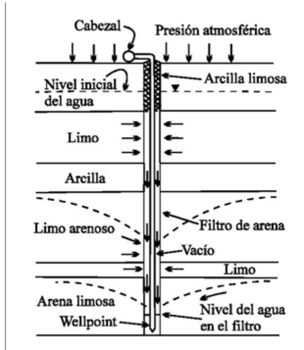
Figura 2.7 Sistema de drenaje por vacío
