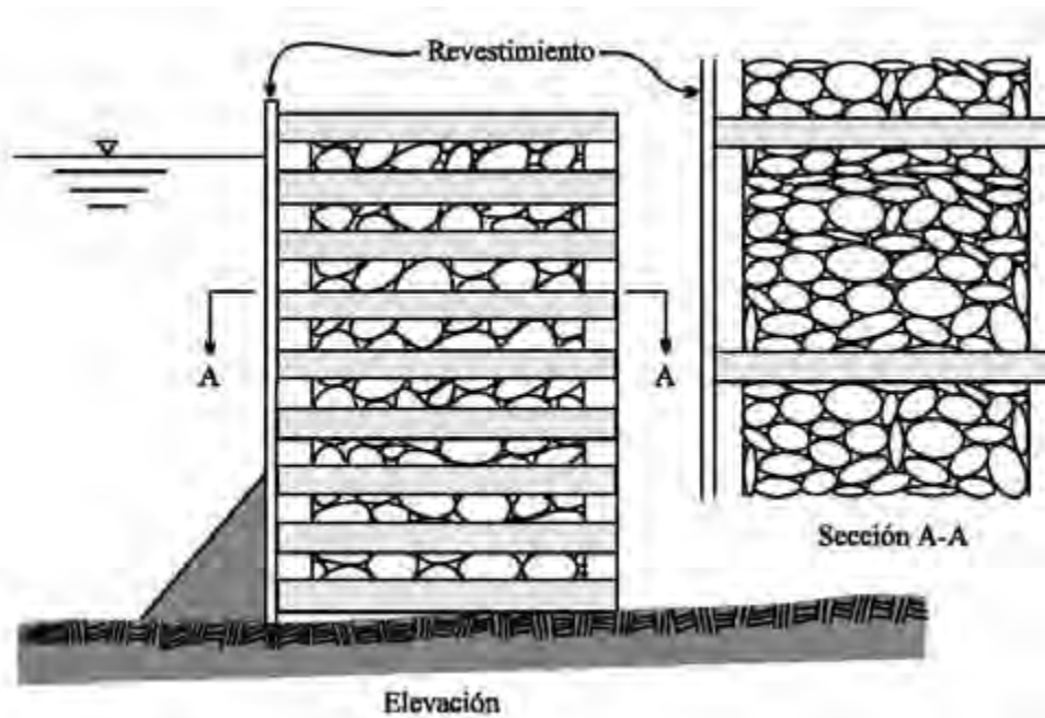
Figura 3.7 Entramado de madera con lastre de piedra
