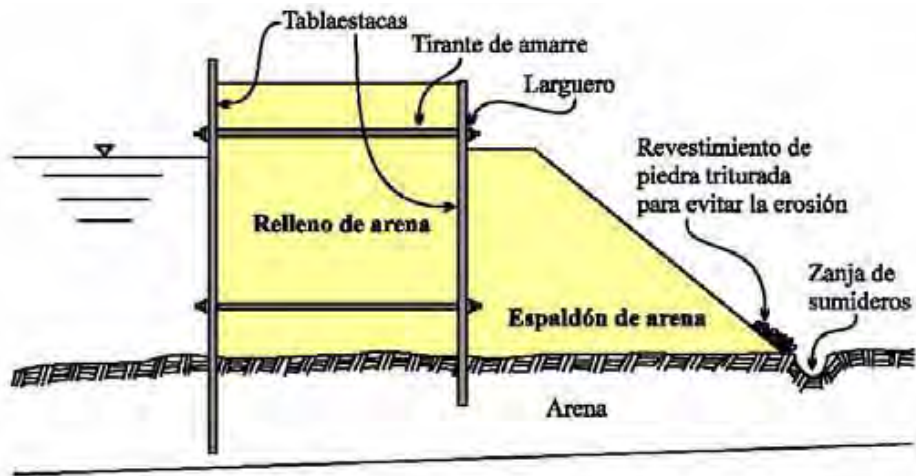
Figura 3.8 Ataguía de doble pared
