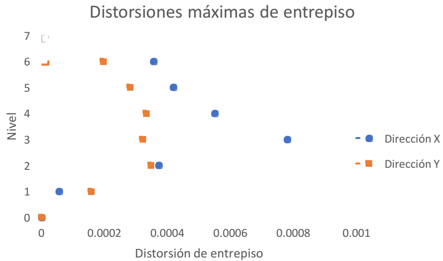
Figura 24: Distorsiones de entrepiso para las dos direcciones en estudio.
