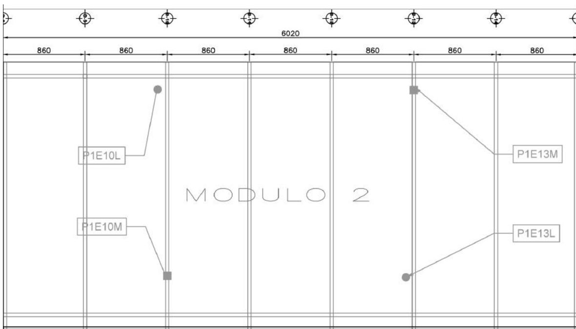
Figura 13: Ejemplo ilustrativo de la ubicación de 4 especímenes extraídos del módulo 2, primer nivel.
