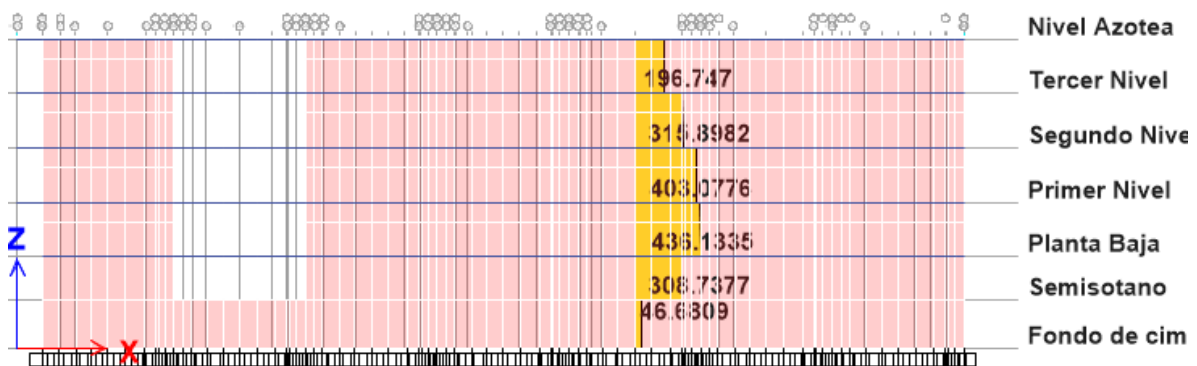
Figura 30: Fuerzas cortantes (tonf) en el muro exterior para la condición de base empotrada.
