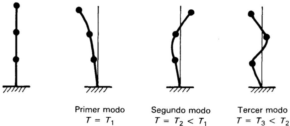
Figura 6: Modos de vibración de un sistema de tres grados de libertad, fuente: Meli, 2002.
