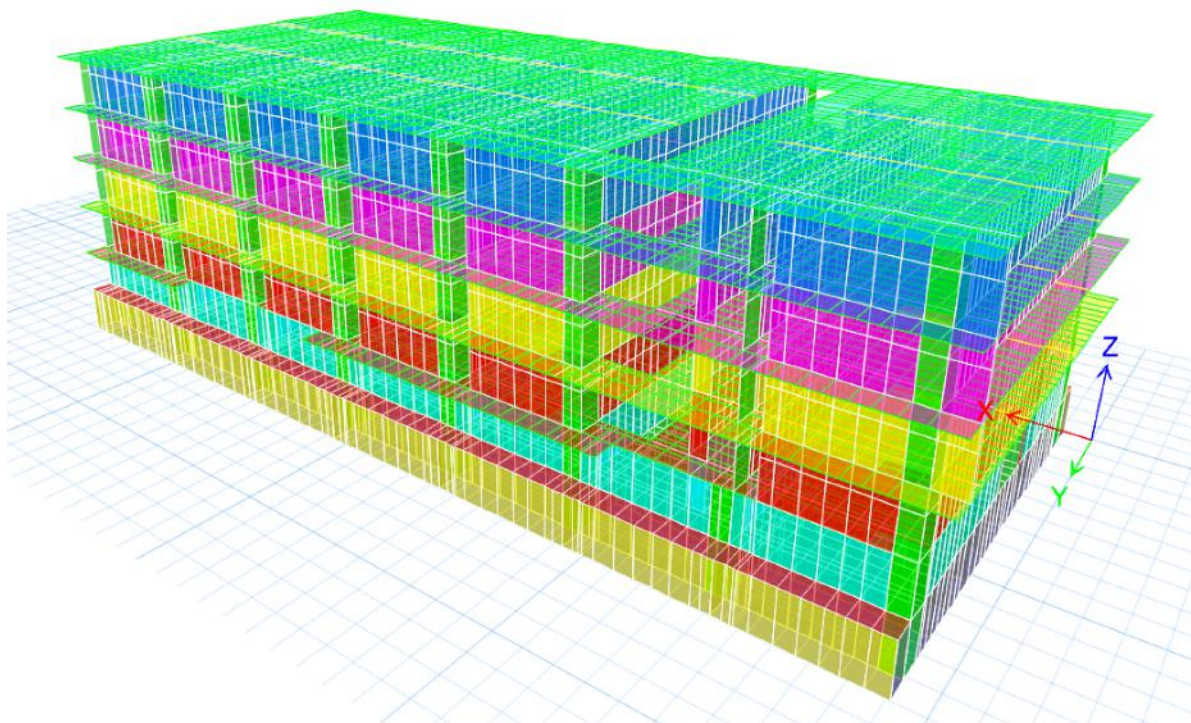
Figura 18: Vista del modelo en donde cada tono representa una sección de concreto diferente.
