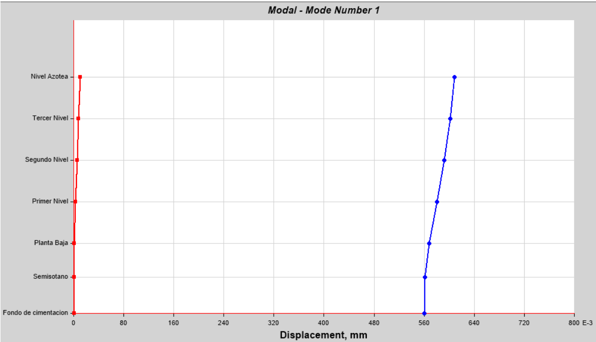
Figura 37: Forma modal para el primer modo de vibrar en la dirección X.
