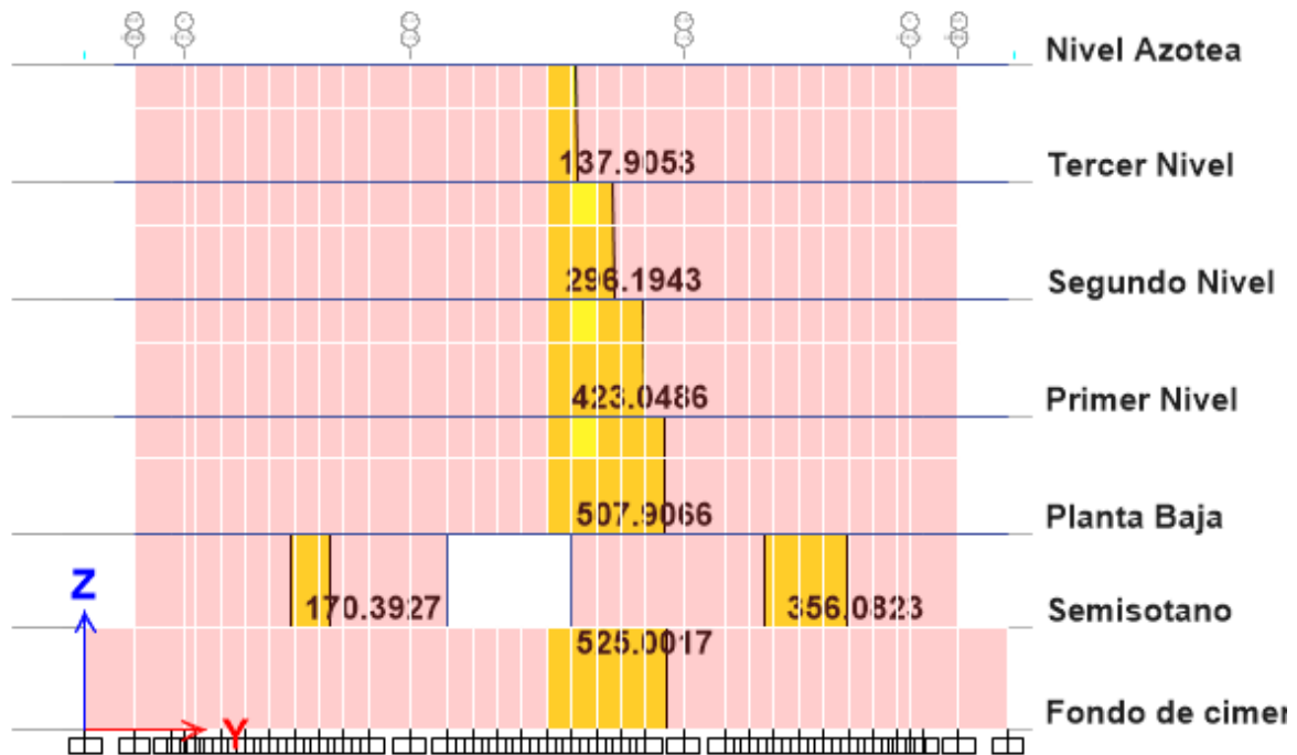
Figura 29: Fuerzas cortantes (tonf) en el muro interior para la condición de base empotrada.
