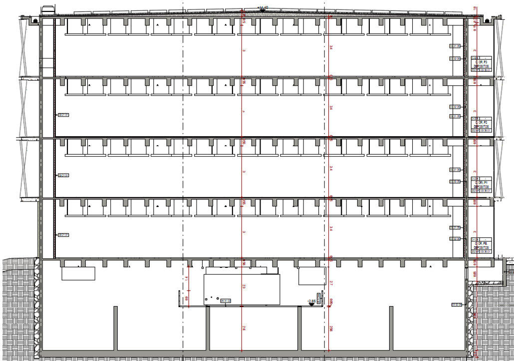
Figura 1: Elevación tipo del edificio en estudio en su dirección transversal.
