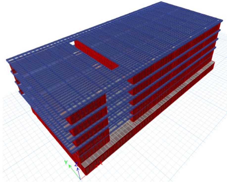
Figura 17: Vista tridimensional extruida del modelo matemático.
