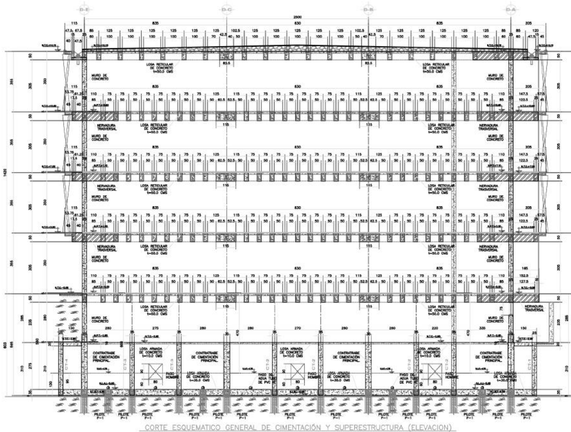
Figura 12: Vista en elevación de la estructura.
