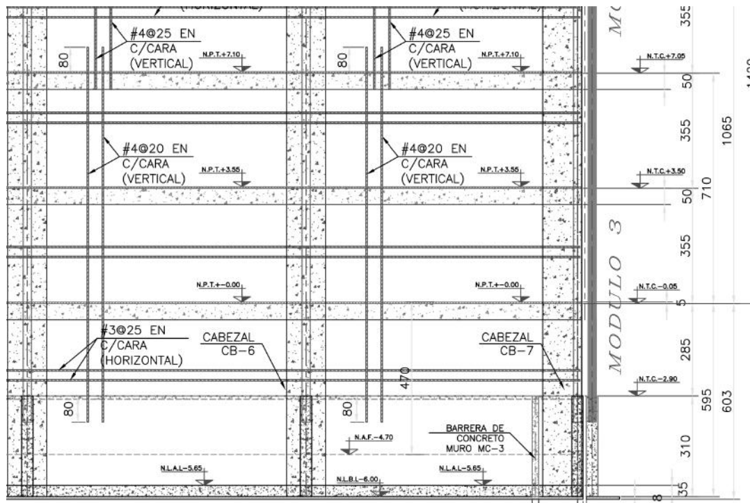
Figura 31: Acero de refuerzo horizontal y vertical en el muro interior.
