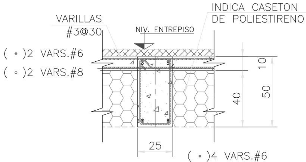
Figura 35: Geometría y armado de nervadura secundaria.
