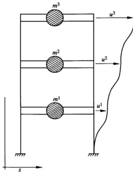
Figura 5: Sistema de tres grados de libertad dinámicos, fuente: Bazan & Meli.
