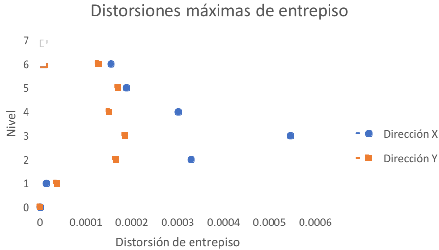
Figura 40: Distorsiones de entrepiso para las dos direcciones en estudio.
