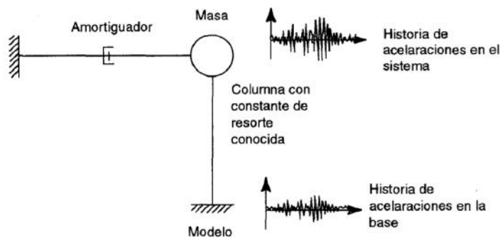
Figura 4: Sistema de un grado de libertad, fuente: Meli, 2002
