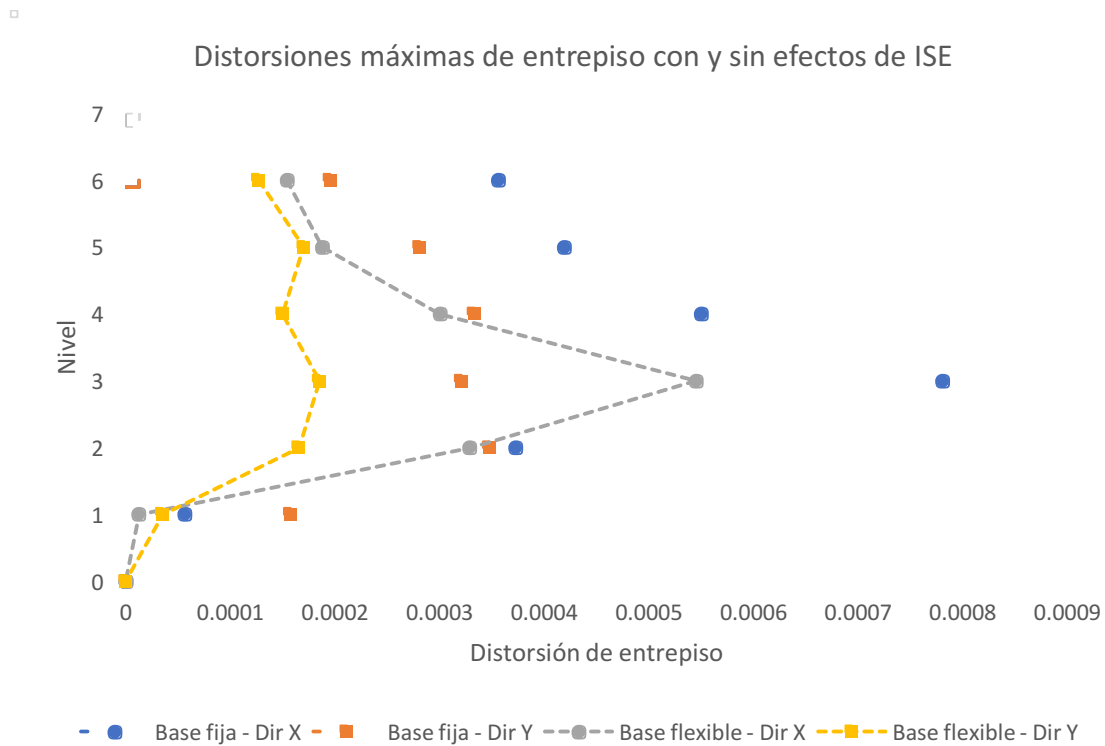
Figura 46: Comparación gráfica de las distorsiones encontradas en todos los niveles.
