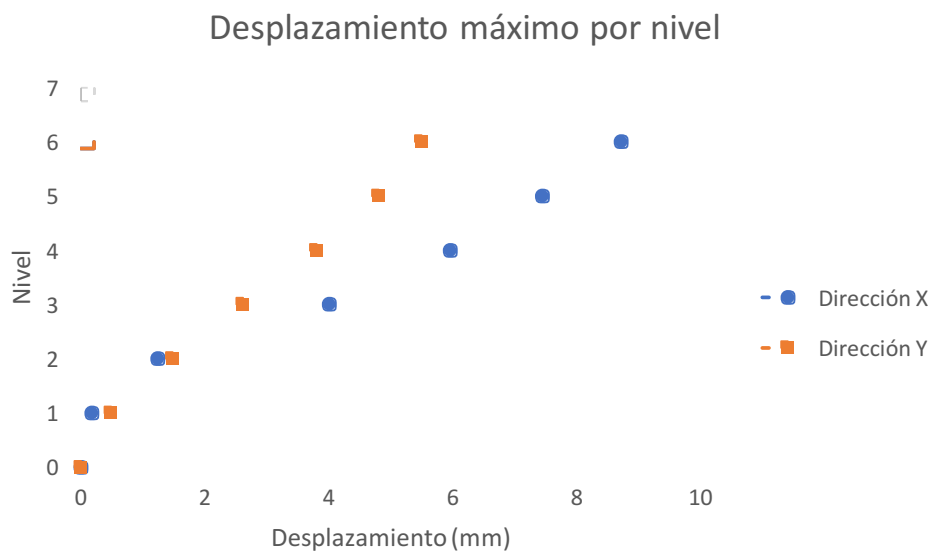
Figura 25: Desplazamientos máximos en ambas direcciones de análisis.
