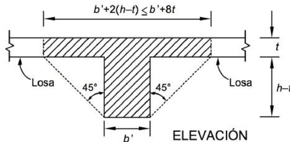
Figura 33: Dimensiones para diseño por torsión.
