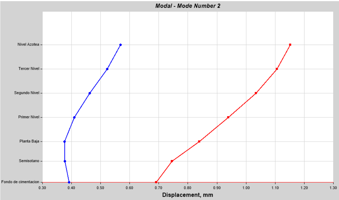
Figura 38: Forma modal para el primer modo de vibrar en torsión.
