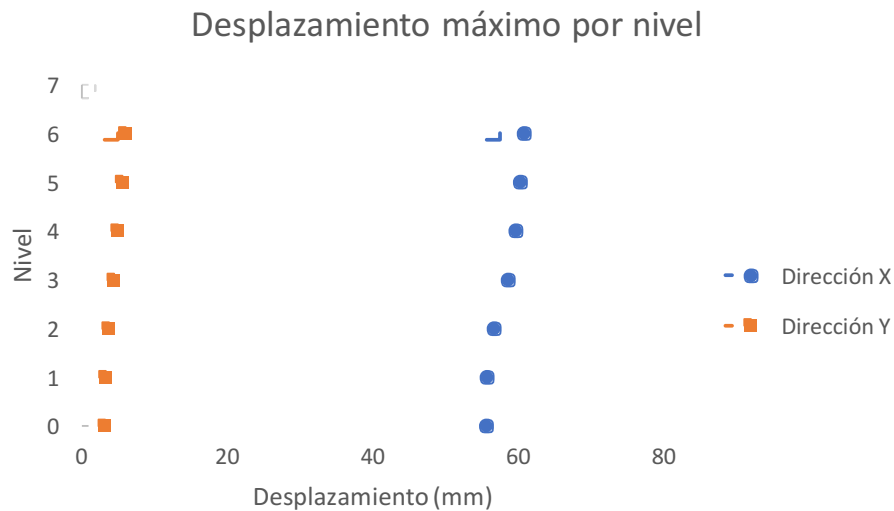
Figura 41: Desplazamientos máximos en ambas direcciones de análisis.
