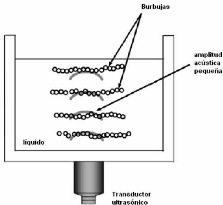
Figura 8. Dispositivo experimental para la producción de SLMB de tipo de onda estacionaria[14].
