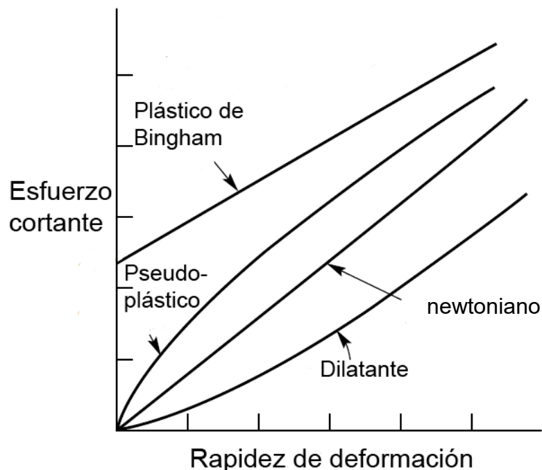
Figura 2. Esfuerzo cortante en función de la rapidez de deformación de materiales viscosos [4].
