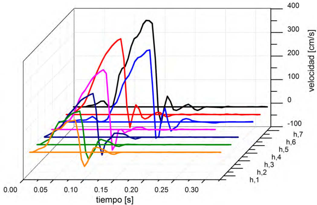
Figura 22. Curvas en cascada de la velocidad de la columna de líquido para cada una de las 'h'.
