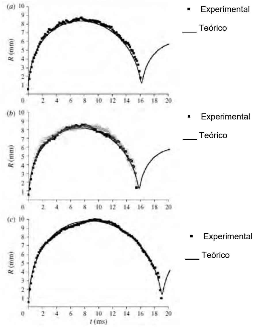
Figura 41. Cálculo del proceso de crecimiento y colapso de una burbuja esférica de acuerdo a Dular y Coutier [29].
