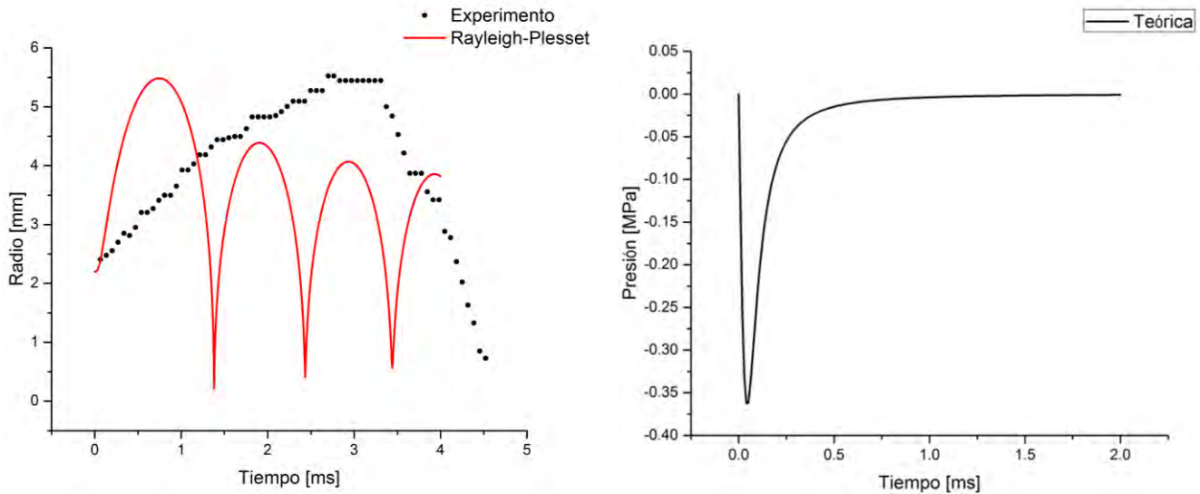
Figura40. a) Gráficas de los radios de la burbuja experimental (realizada con una h'= 18\text{cm.} ) y con la ERP- b) pulso de tensión en el líquido.
