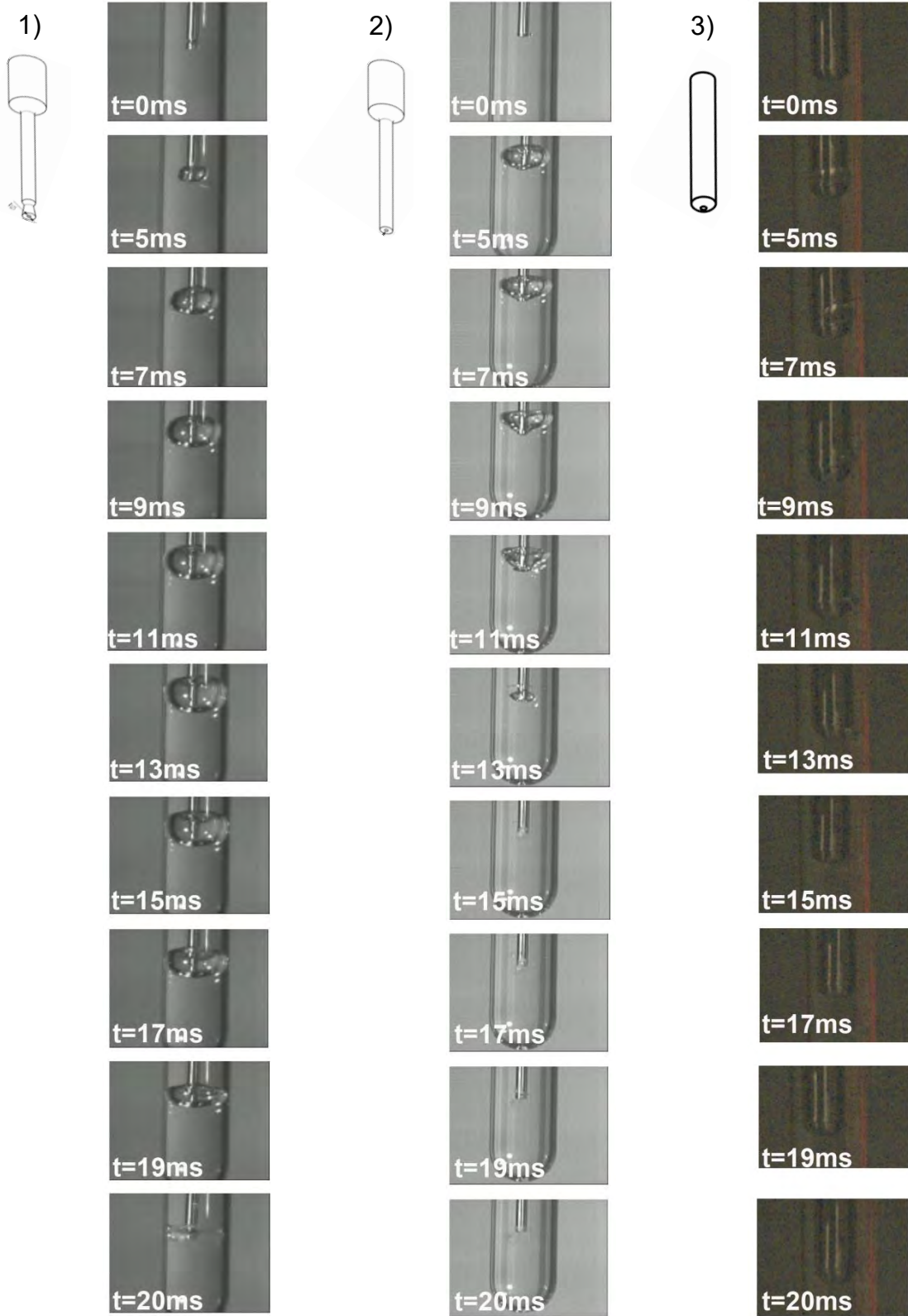
Figura 32. Se muestra una serie de fotografías con la evolución de la burbuja en el tiempo, cada una con distinto diseño de punta que contiene a la muesca donde se inserta el núcleo de burbuja. 1) Punta de tobera, 2) punta recta, 3) punta redondeada con la misma sección transversal que la barra, donde no hay generación de burbuja y solo se alcanza a ver una estela del fluido que pasa a través de sus paredes, además que la calidad de las fotografías es menor a las anteriores ya que la cámara de alta velocidad fue también de menor velocidad. Todas las pruebas se realizaron con una carrera 'h' de 14cm.
