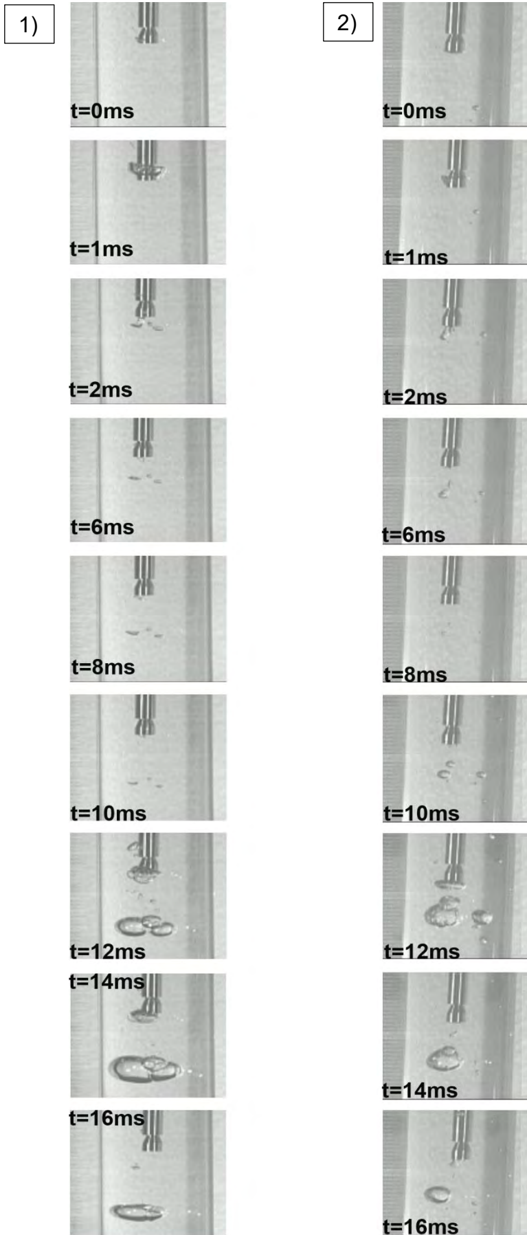
Figura 35. Secuencias fotográficas realizadas con 1) fluido newtoniano y 2) fluido no newtoniano (adelgazante), a una carrera 'h' de 15cm. En ambos experimentos se logra desprender la burbuja de las puntas, creciendo en el tiempo para luego disminuir su radio, en ambas se logran crear diferentes burbujas, que se adhieren unas con otras en su superficie y al final lograr cohesionarse hasta convertirse en una sola.
