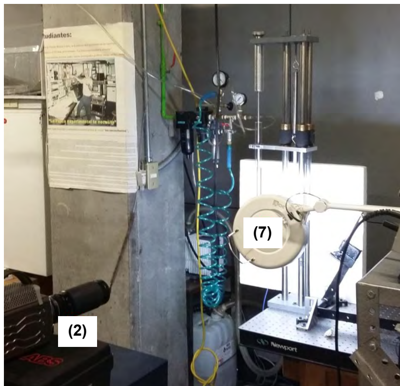
Figura 18. Arreglo experimental para generar cavitación transitoria , este arreglo consta de (2) cámara de alta velocidad Phantom V 9.1, (3) osciloscopio Tektronix TDS540 A 500 MHz de 4 canales y (4) acondicionador de señal PCT (5) sensor de fuerza modelo PCB 200B04 4.448kN (6) cámara digital Casio Exilim Exf1 60 fps (7) lámparas de xenon, (8) dispositivo mecánico, (9) gatillo mecánico.
