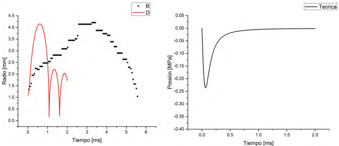
Figura 42. a) Gráficas de los radios de la burbuja experimental (realizada con una h' = 11\text{cm.} ) y con la ERP; b) pulso de tensión en el líquido.
