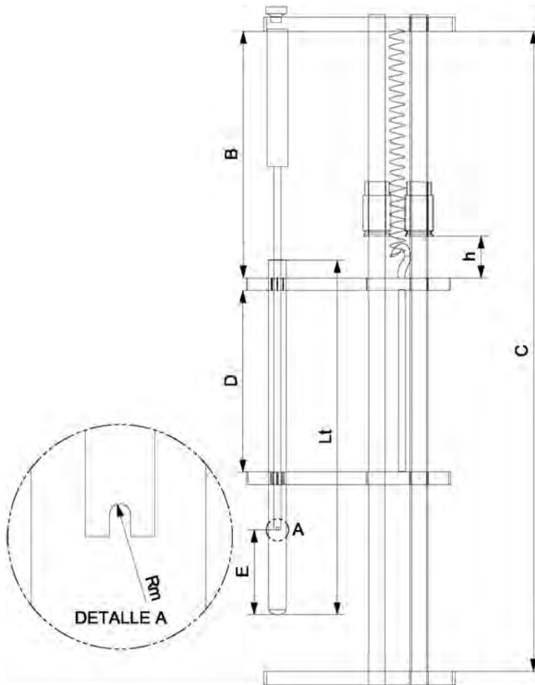
Figura 16. Plano del dispositivo mecánico para crear cavitación transitoria. Los parámetros a considerar para el experimento de cavitación son: h , que corresponda a la carrera del tubo hacia arriba hasta el punto donde se detiene subitamente con los topes de neopreno; L_t , es la longitud del tubo que contiene el líquido; R_m , es el radio de la muesca del vástago que se introduce en el tubo con líquido; B , es la distancia de la placa de sujeción superior a la placa-corredera superior; C , es la distancia entre la placa de sujeción inferior y la placa de sujeción superior; D , es la distancia entre la placa-corredera superior y la placa-corredera inferior; E , es la distancia de la punta que contiene la muesca donde se inserta el núcleo de burbuja a la punta del tubo que contiene el líquido. El detalle A , muestra la muesca donde inicialmente se atrapa una cantidad de gas que sirve de núcleo para hacer propicia la cavitación.
