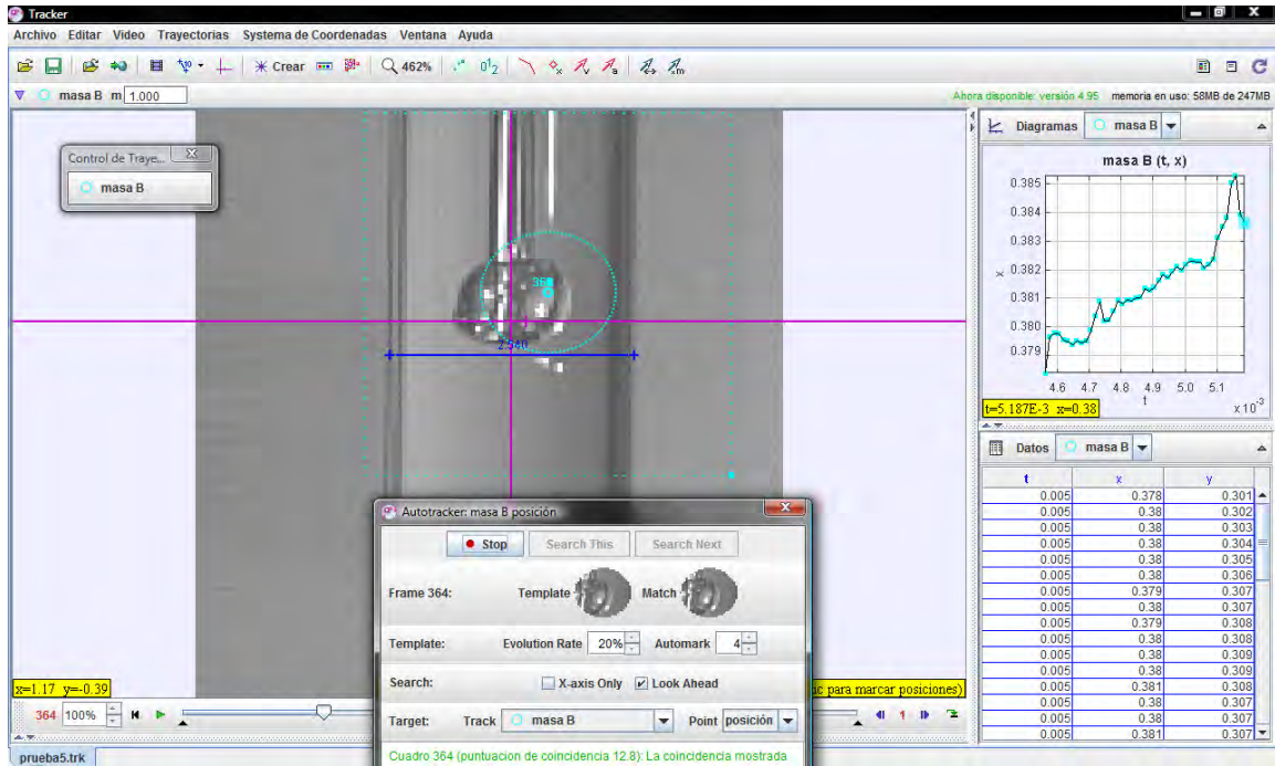
Figura C.2. El programa de Tracker, requiere un control de trayectoria (masa B en color verde agua), mismo que seguirá una partícula u objeto, definiendo su desplazamiento, velocidad, aceleración, etc. En este caso, cómo evoluciona el tamaño de la burbuja.
