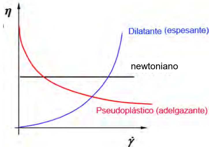
Figura 3. Comportamiento de fluidos Newtonianos y no Newtonianos, la viscosidad vs velocidad de corte [5].
