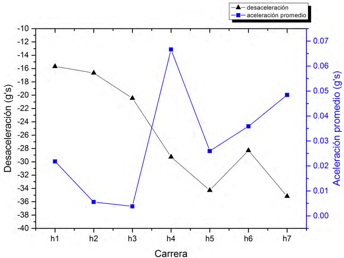
Figura 27. Gráfica de desaceleración y aceleración promedio máxima contra carrera.
