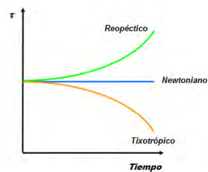
Figura 4. Efecto del tiempo sobre el esfuerzo aplicado en algunos fluidos [7].
