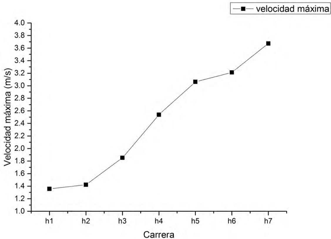
Figura 26. Gráfica velocidad contra carrera.
