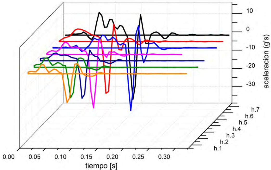
Figura 23. Curvas en cascada de la aceleración de la columna de líquido para cada una de las 'h'.
