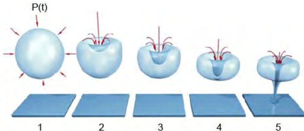
Figura 5. (1) La presión P(t) del líquido actúa sobre la burbuja, (2) iniciando el colapso de la misma, (3) y (4) la formación del chorro de agua y finalmente (5) impactando sobre una superficie, provocando posteriormente erosión en equipos de trabajo como bombas o en álabes de una turbina [10].
