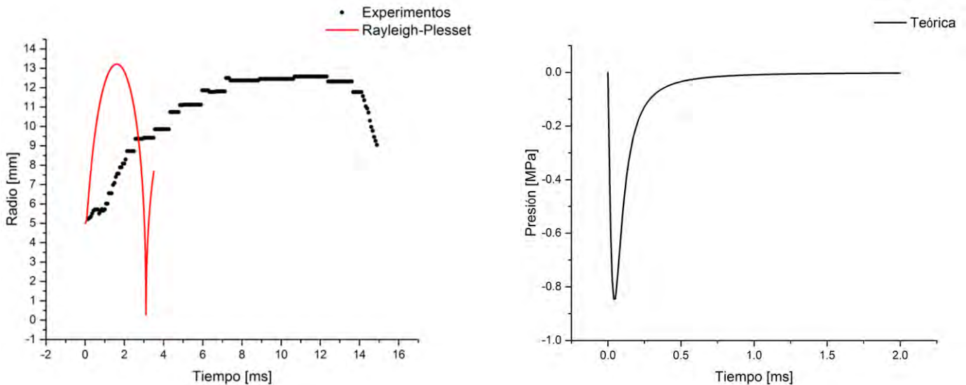
Figura 39. a) Gráficas de los radios de la burbuja experimental (realizada con una h'=14\text{cm.} ) y con ERP; b) pulso de tensión en el líquido.
