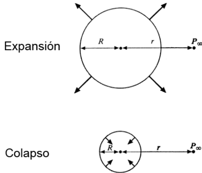
Figura 14. Expansión y colapso de burbujas [30].
