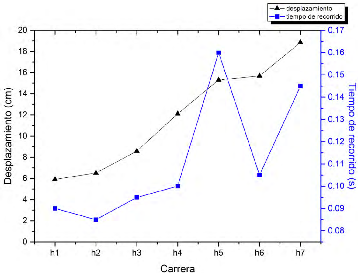
Figura 25. Desplazamiento y tiempo de recorrido contra carrera.
