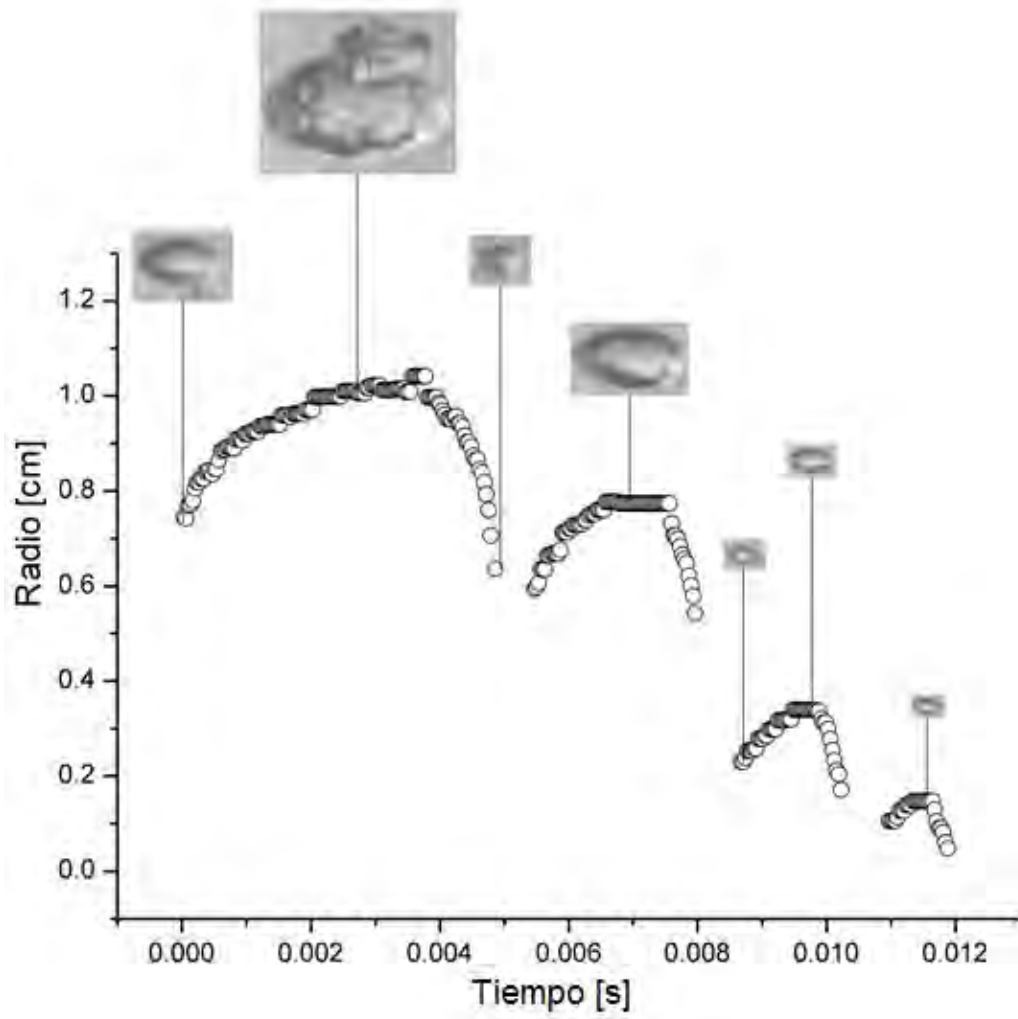
Figura 31. Gráfica de una burbuja que experimentó diversos rebotes, hasta desaparecer.
