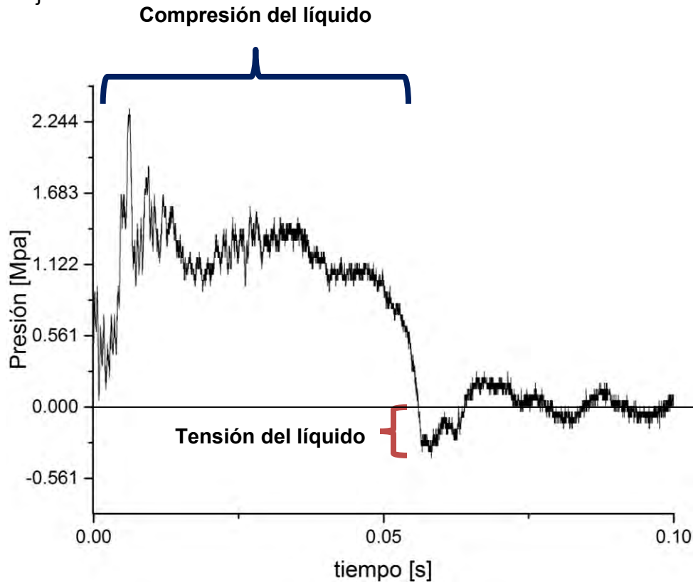
Figura 28. La tensión del líquido es registrada por el sensor, midiendo una disminución en la presión.
