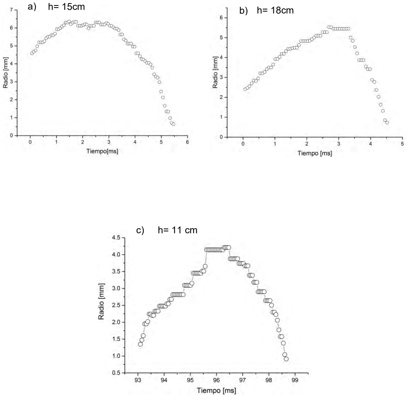
Figura 30. Gráficas que muestran la evolución del radio de una burbuja con respecto al tiempo.
