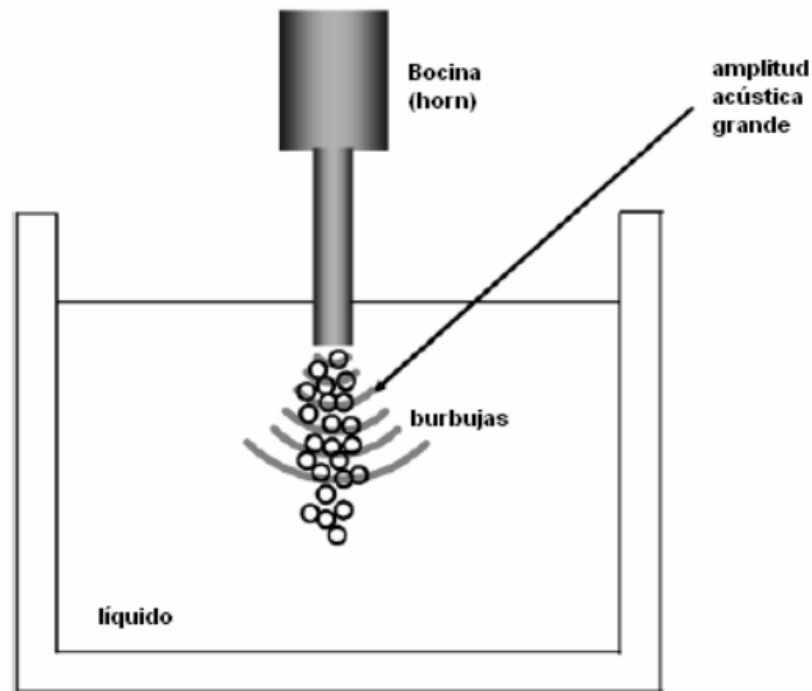
Figura 9. Dispositivo experimental para producir SLMB de tipo bocina [14].
