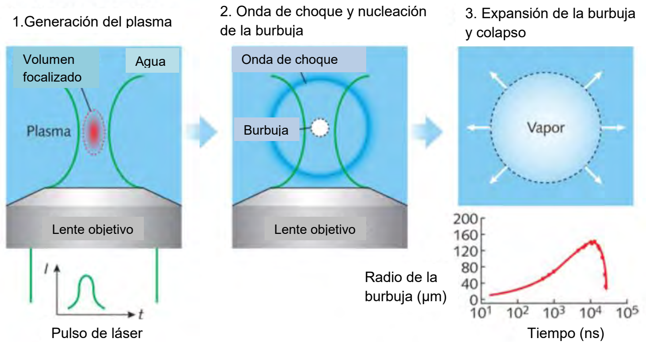
Figura 11: Cavitación transitoria por medio de un punto focalizado utilizando un láser [17].
