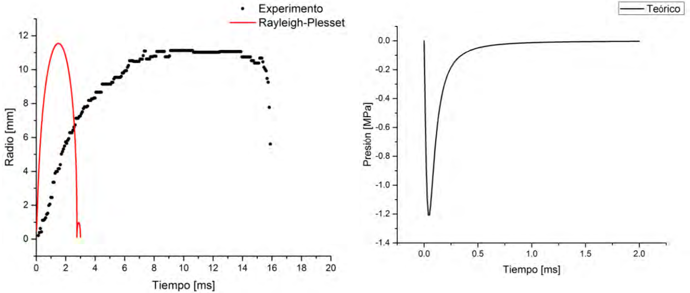
Figura 38. a) Gráficas de los radios de la burbuja experimental (realizada con una h'=14\text{cm.} ) y con la ERP- b) pulso de tensión en el líquido.
