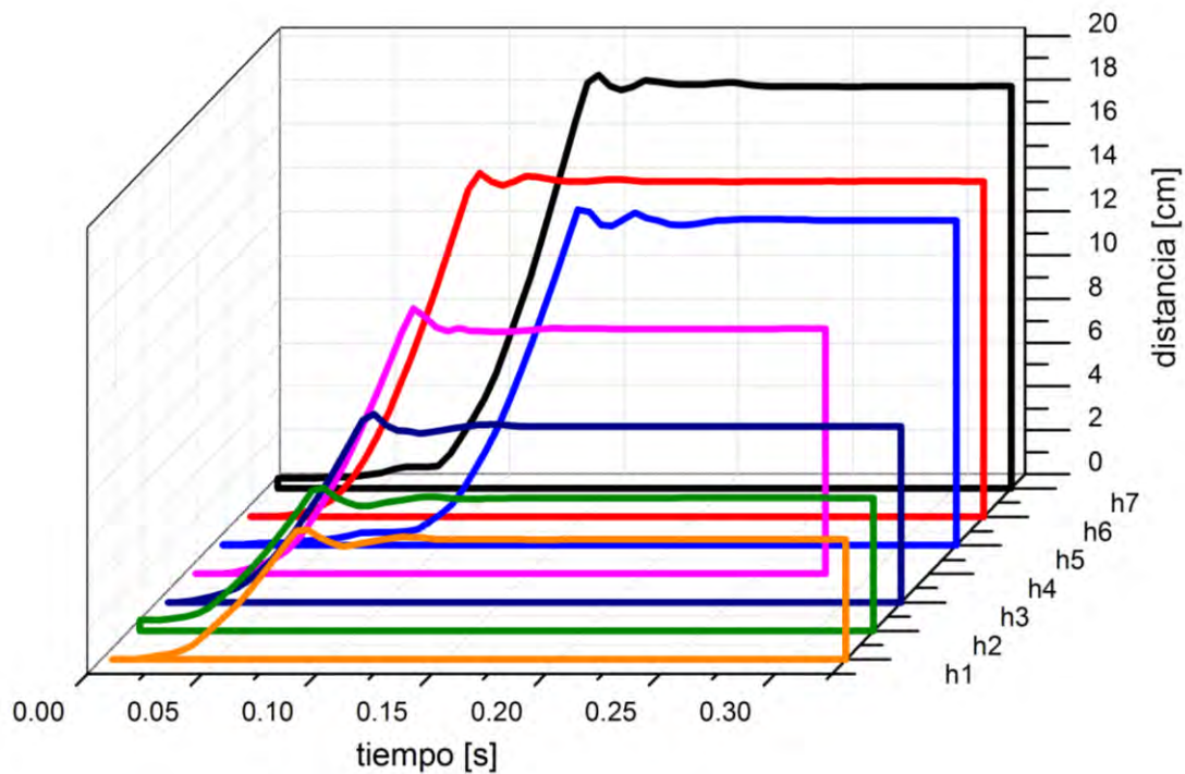
Figura 21. Curvas en cascada del desplazamiento de la columna de líquido para cada una de las 'h'; los tiempos de recorrido, son los alcanzados en el punto máximo de las curvas.
