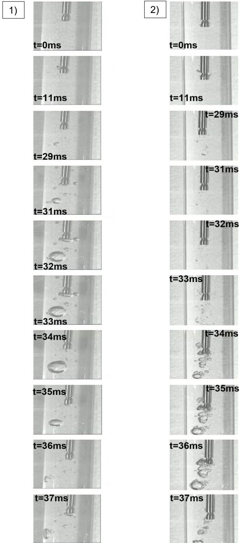
Figura 36. Experimentos realizados en 1) fluido newtoniano y 2) fluido no newtoniano (adelgazante) a una carrera 'h' de 18 cm. En el fluido newtoniano se logra observar que la burbuja se desprende y crece en el tiempo con una serie de burbujas de menor tamaño radial a su alrededor para luego decrecer en tamaño. En el fluido adelgazante ocurre un fenómeno donde muchas burbujas crecen en el tiempo distanciadas a una corta distancia unas de otras para luego disminuir en su tamaño radial.
