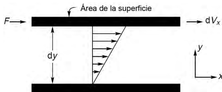
Figura1. Representación esquemática del flujo cortante unidireccional [1].
