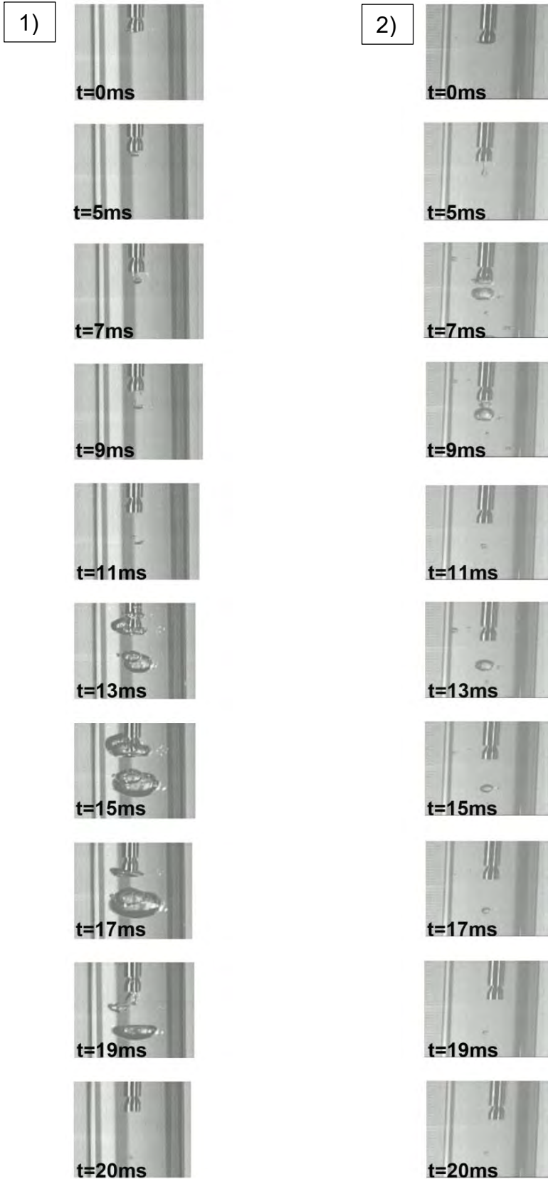
Figura 34. Se comparan dos series de fotografías, 1) fluido newtoniano y 2) fluido no newtoniano (adelgazante), los experimentos se realizaron con una carrera 'h' de 8.0 cm; en el fluido newtoniano 1) se desprende la burbuja de la punta y creciendo en el tiempo muy alejada de una forma circular y colapsando posteriormente, a la par que en la punta se logra formar otra cavidad que al final se desprende sin crecer; en 2) se logra desprender una burbuja sin crecer con un radio considerable y teniendo algunos rebotes hasta solo quedar una pequeña burbuja de radio mínimo.
