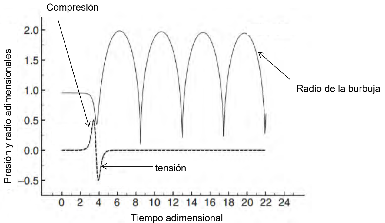
Figura 37. Representación gráfica del crecimiento, colapso y frecuencia de rebotes de una burbuja y la primera fase de un pulso de presión y su contra parte de tensión, calculados con la ecuación (5.7) [32].
