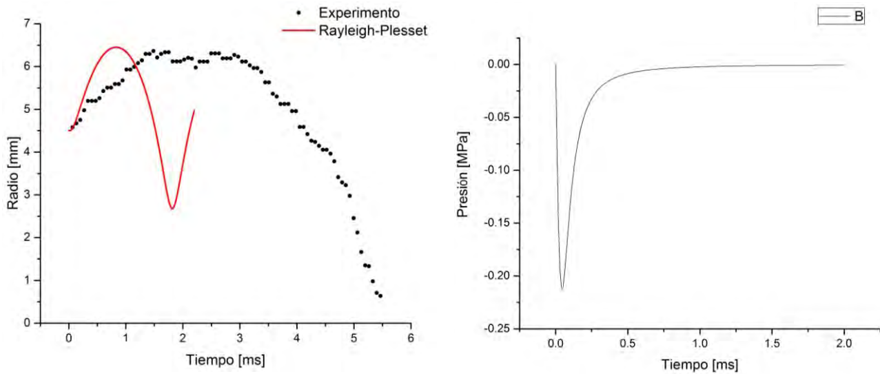
Figura 41. a) Gráficas de los radios de la burbuja experimental (realizada con una h' = 15\text{cm.} ) y con la ERP-b) pulso de tensión en el líquido ec.5.7.
