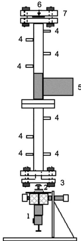
Figura 10. Arreglo experimental del método bala-pistón. (1) pistola Magnum modelo 700, (2) “cabezal tipo hongo”, (3) pistón de acero, (4) transductores de presión montados al tubo, (5) soporte de brazo, (6) junta de sellado, (7) brida de sellado [16].
