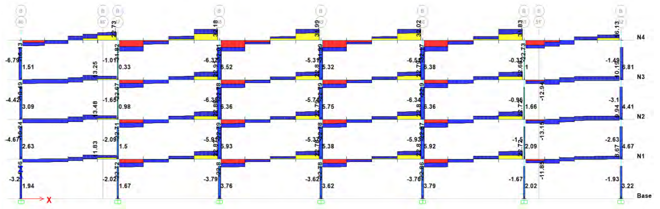
Figura 31 Diagrama de elementos mecánicos para fuerza cortante, eje B.
