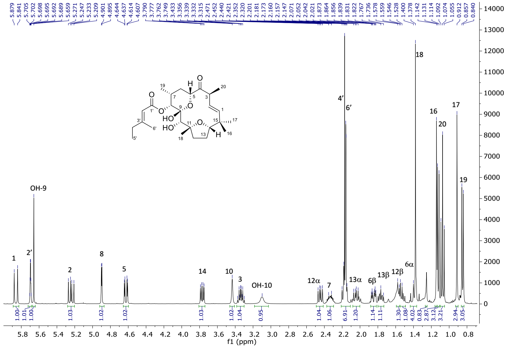
Espectro 43. RMN 1 H (CDCl 3 , 400 MHz) de tonantzitolona ( 38 )
