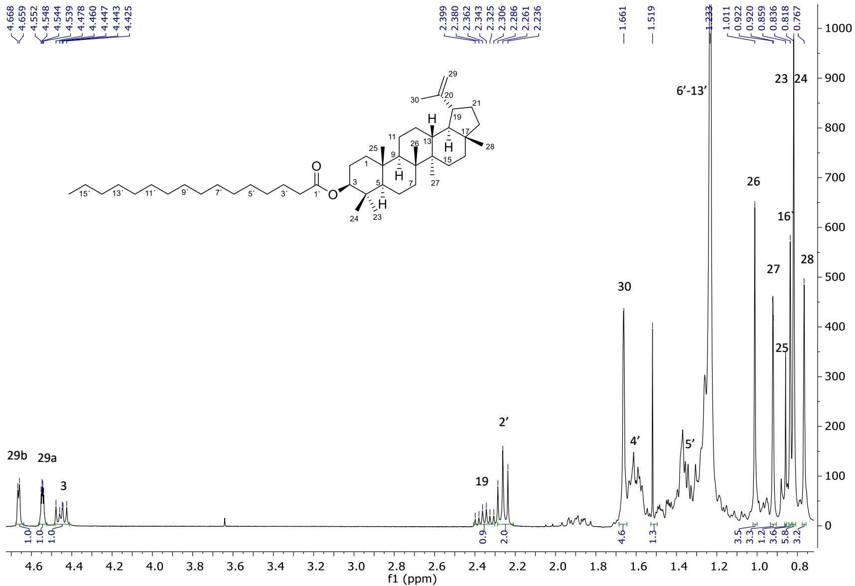
Espectro 3. RMN 1 H (CDCl 3 , 400 MHz) de palmitato de lupeól (89)
