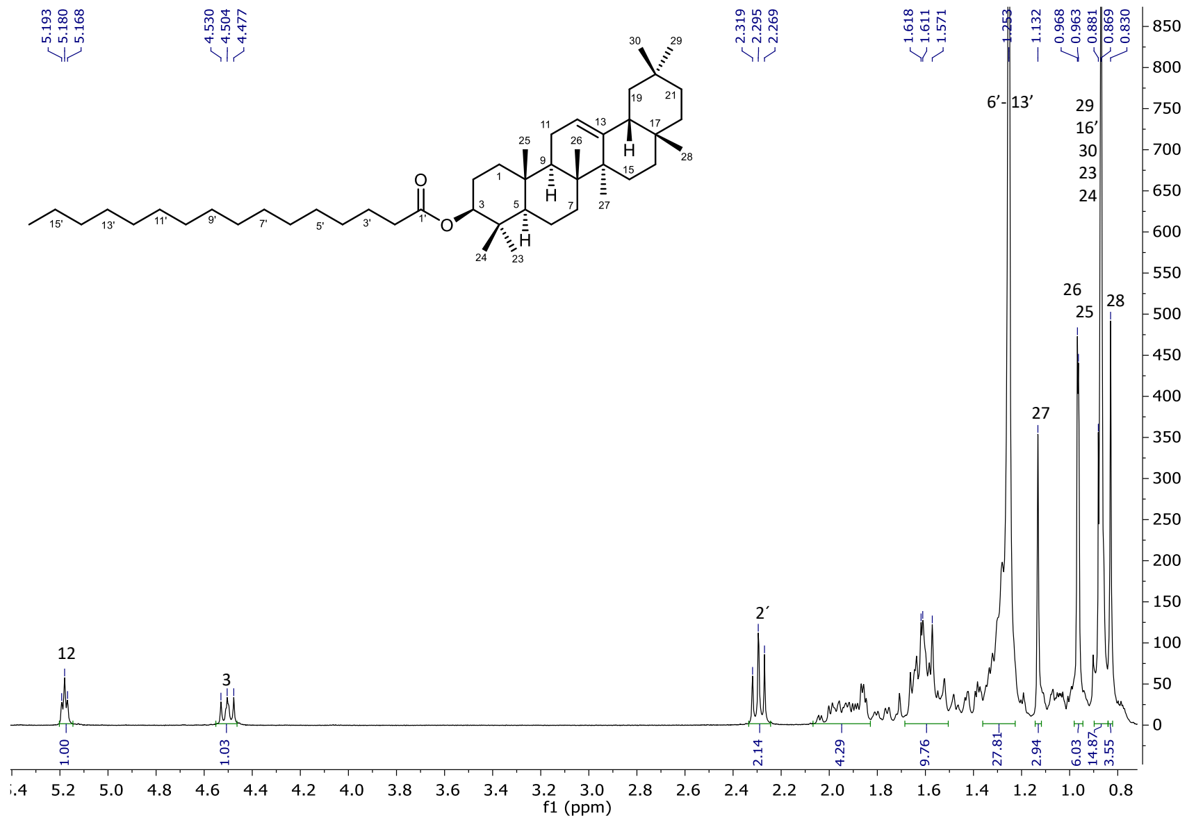
Espectro 1. RMN ^1\text{H} ( \text{CDCl}_3 , 400 MHz) de palmitato de \beta -amirilo ( 88 )
