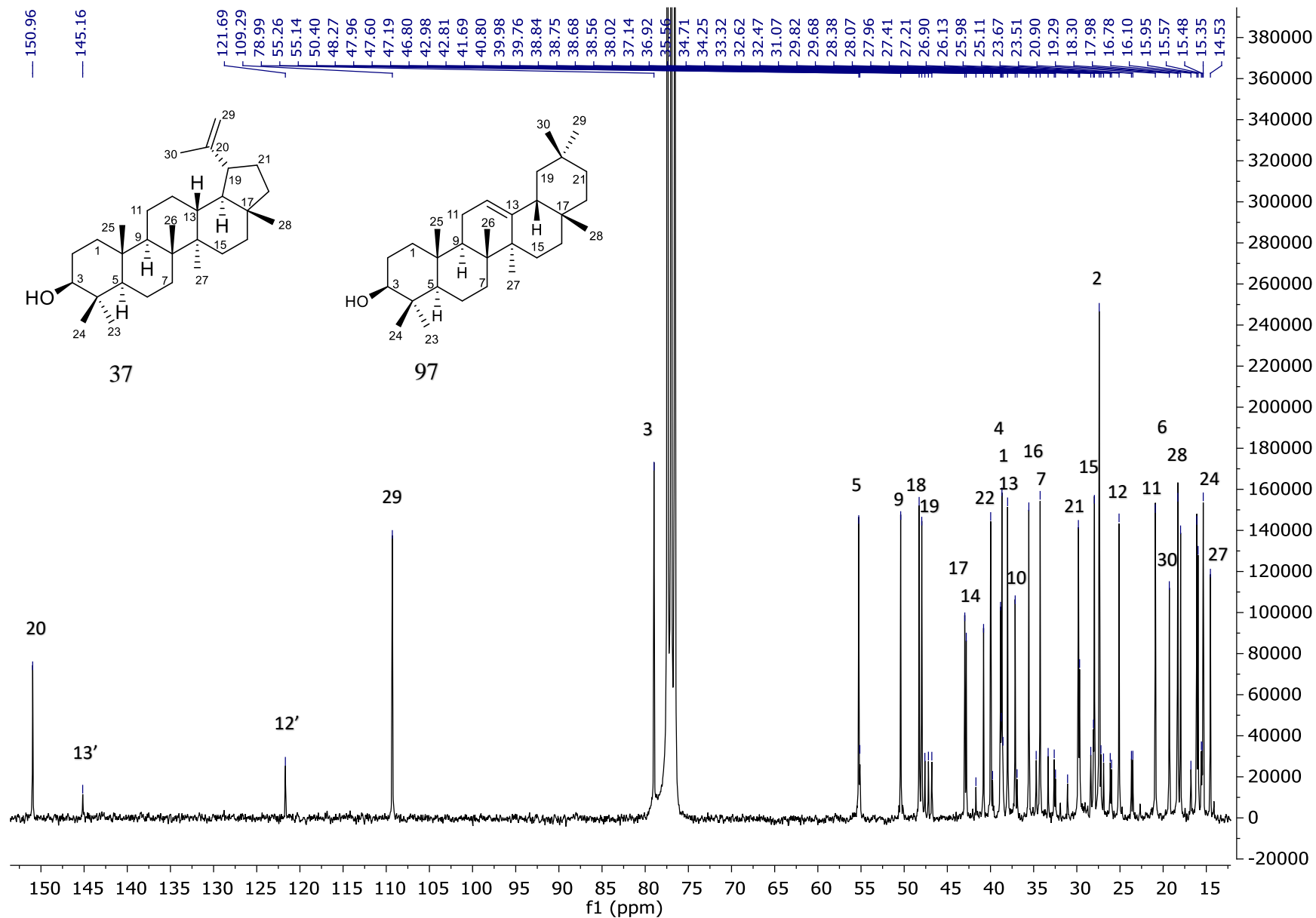
Espectro 28. RMN ^{13}\text{C} (CDCl 3 , 75 MHz) mezcla de 19\beta\text{H} -lupeol ( 37 ) y \beta -amirina ( 97 ) (9:1)
