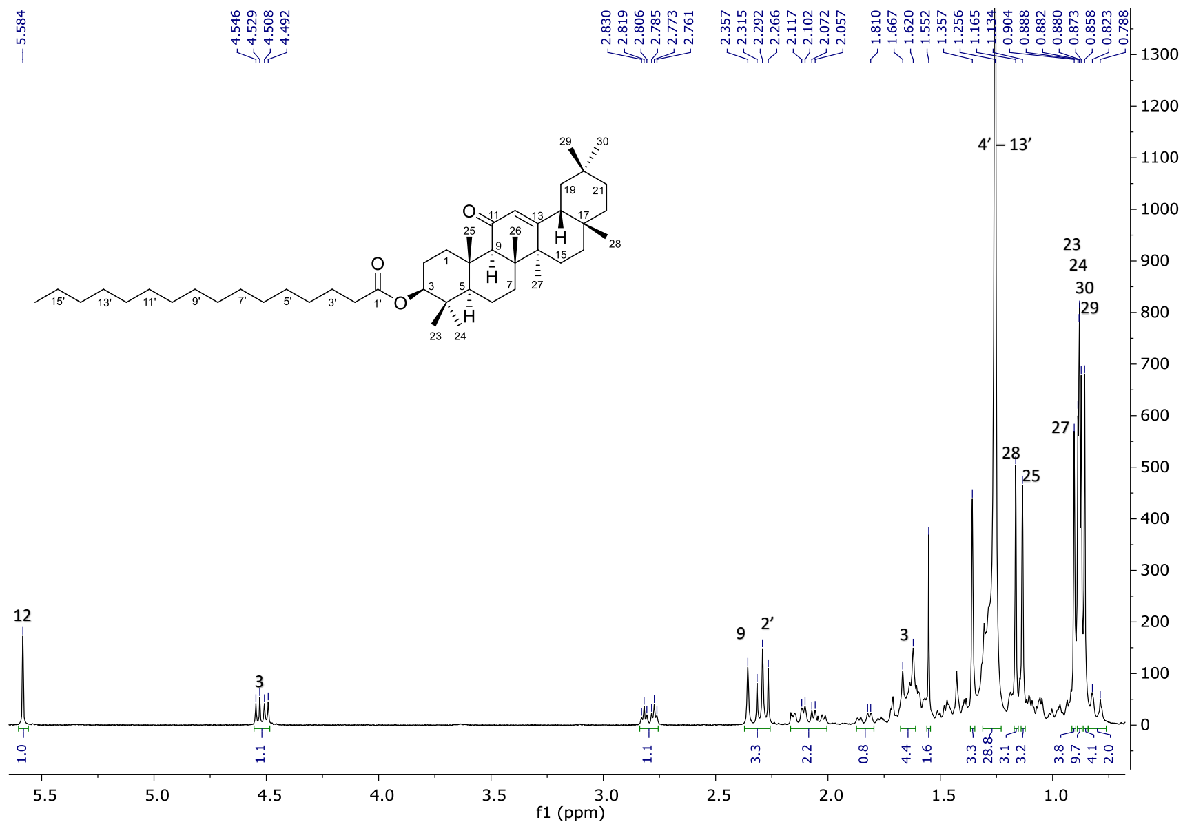
Espectro 7. RMN 1 H (CDCl 3 , 300 MHz) de palmitato de 11-oxo-β-amirilo (91)
