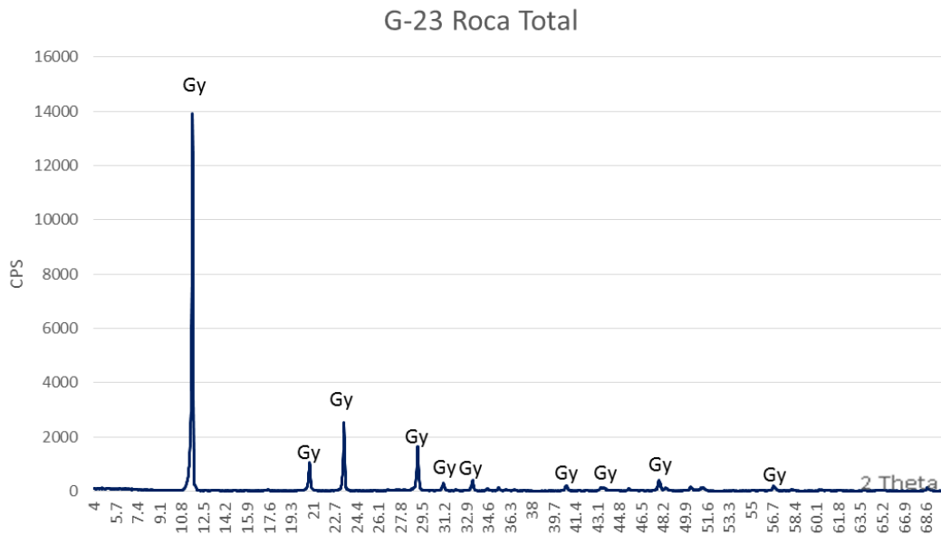
Figura 4.7. Difractograma de la muestra G-23. Se observa claramente la presencia de yeso (Gy).
