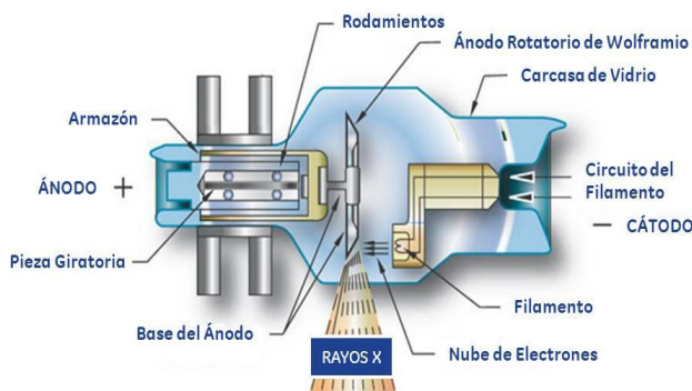
Figura 2.7. Tubo de Rayos X. (Sabaté, 2012).
