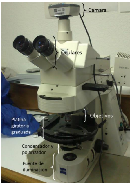
Figura 2.3. Esquema del microscopio petrográfico. Laboratorio de petrografía y minerografía, Instituto de Geofísica, UNAM.
