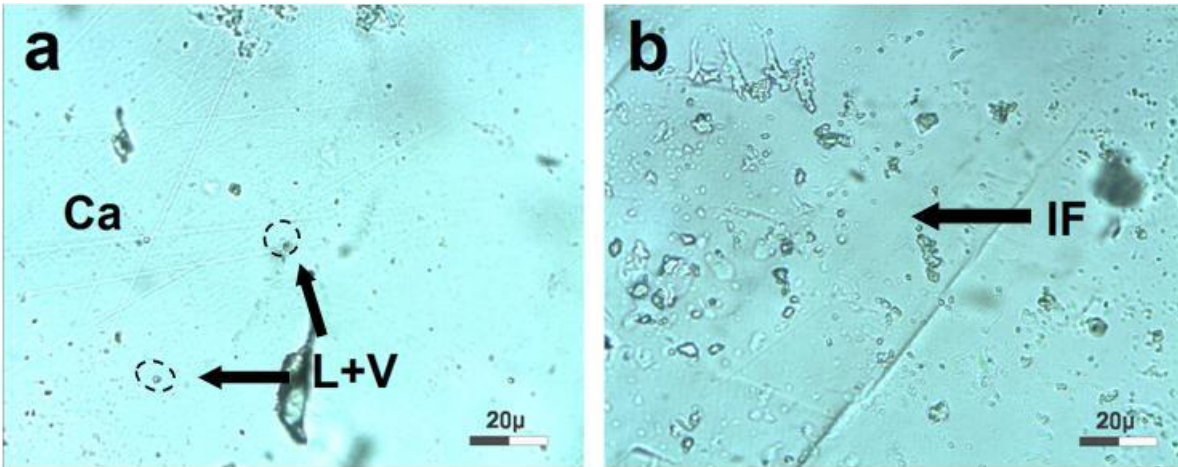
Figura 17. a) Cristal de calcita donde se muestran IF con una relación L+V. b) Distribución de inclusiones de tipo L de formas irregulares. Muestra: Alteración por manifestación geotérmica. M-9A, 50X.
