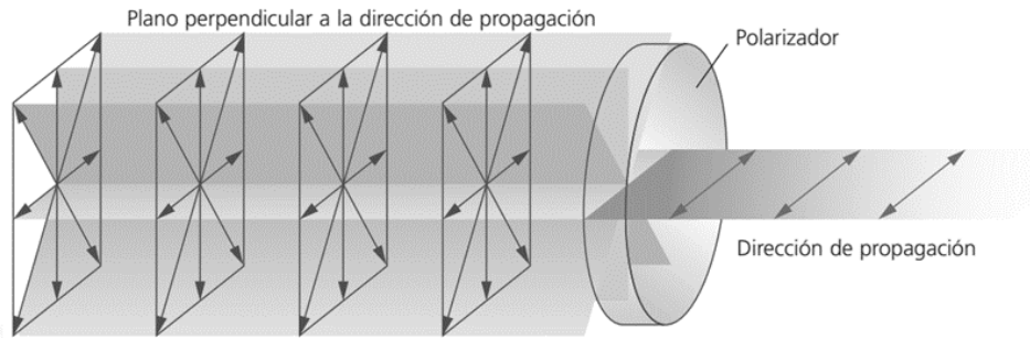
Figura 2.4. Comportamiento de la luz a través de un polarizador. Como se puede observar la luz en un principio se propaga en varias direcciones, al entrar en contacto con el polarizador la dirección de propagación va en una sola dirección [6].
