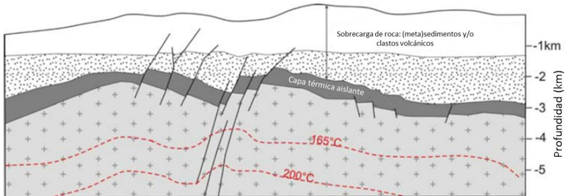
Figura 1.14 Los controles geológicos sobre la temperatura en un tipo de play de basamento de roca cristalina consiste en la producción de calor roca cubierta por capas aislantes térmicamente como la pizarra y otros sedimentos de sobrecarga. (Best Practices Guide For Geothermal Exploration, IGA, 2014).
