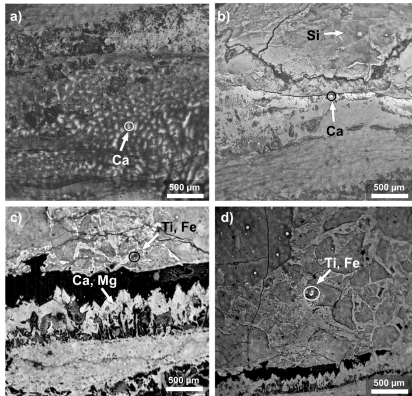
Figura 4.20. Identificación de concentraciones de elementos en puntos específicos de la lámina de la muestra M-13a. a) El contenido de Ca en esta sección hace referencia a la presencia de calcita, mientras que en la imagen b) y c) el contenido de Ca es evidencia de la existencia del mineral romboédrico de dolomita. Los cristales de ilmenita c) y d) presentan concentraciones en Ti y Fe en fragmentos de 100 v 200 μm.
