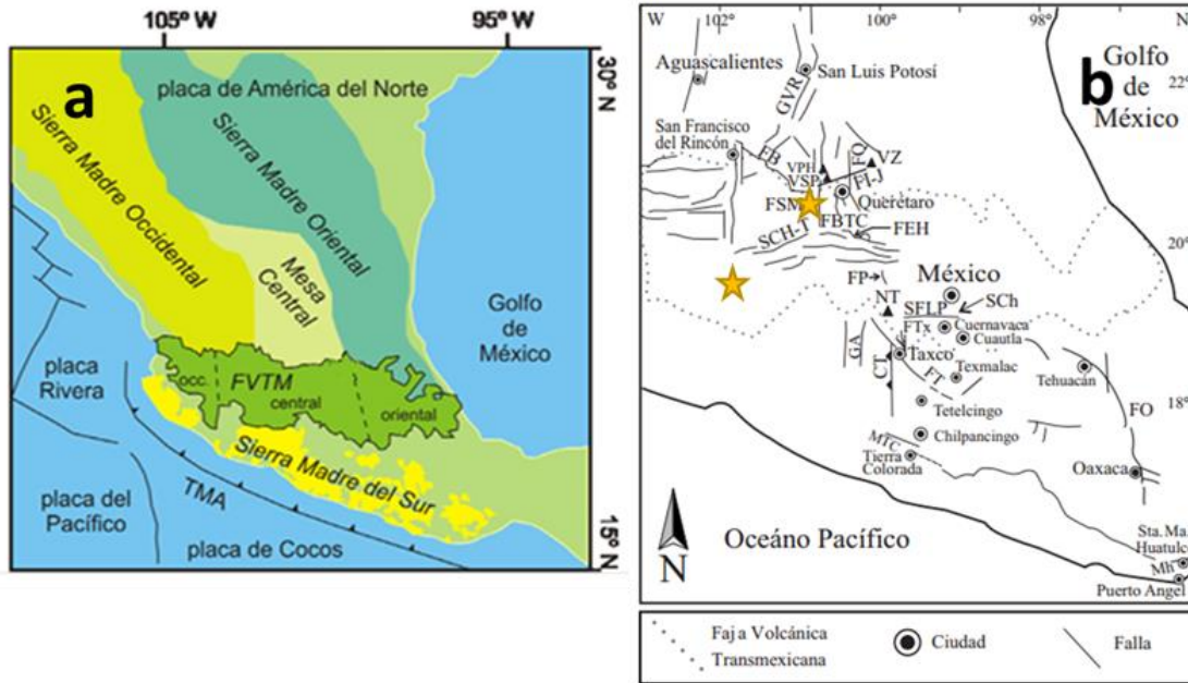
Figura 3.2. a) Ubicación geográfica de la Faja Volcánica Trans-Mexicana, de las principales provincias geológicas de México, de las placas tectónicas actuales y la Trincheras Mesoamericana (TMA) (Mori, et al. , 2007). También se muestra la división de la FVTM en tres sectores (occidental, central y oriental) (Pasquarè et al. , 1988). b) Ubicación de las fallas mayores, volcanes y ciudades. FSMA: falla San Miguel de Allende.
