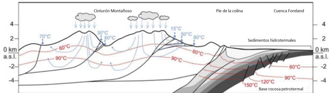
Figura 1.13 Estructura típica de conducción térmica (isotermas rojas), rutas de flujo del agua subterránea, y temperaturas de descarga (flechas azules) en zonas orogénicas. (Best Practices Guide For Geothermal Exploration, IGA, 2014).
