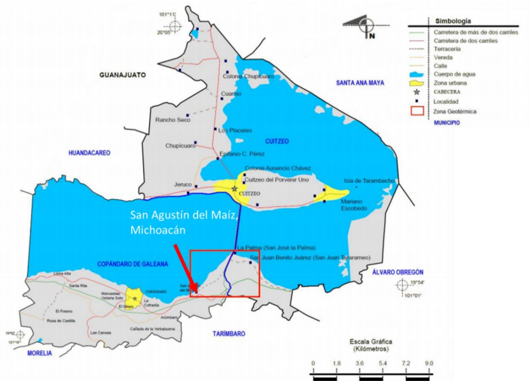
Figura 3.8. Localización de la zona de estudio San Agustín del Maíz, Michoacán. También se ubica la zona geotérmica San Juan Tarameo (INEGI, 2005).
