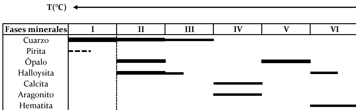
Figura 5.2. Secuencia paragenética de las muestras de roca de San Agustín del Maíz, Michoacán. Las etapas que se presentan son: I) Paragénesis hipogénica, cuarzo + plagioclasa + hornblenda ± pirita; II) Argílica avanzada, cuarzo + ópalo ± halloysita; III) Argílica, cuarzo ± halloysita; IV) Veta, calcita ± aragonito; V) Sinter, ópalo; VI) Supergénica, halloysita ± hematita.
