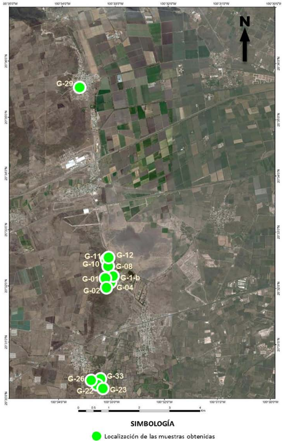
Figura 3.7. Mapa de distribución de las muestras estudiadas en San Bartolomé de los Baños, Guanajuato.
