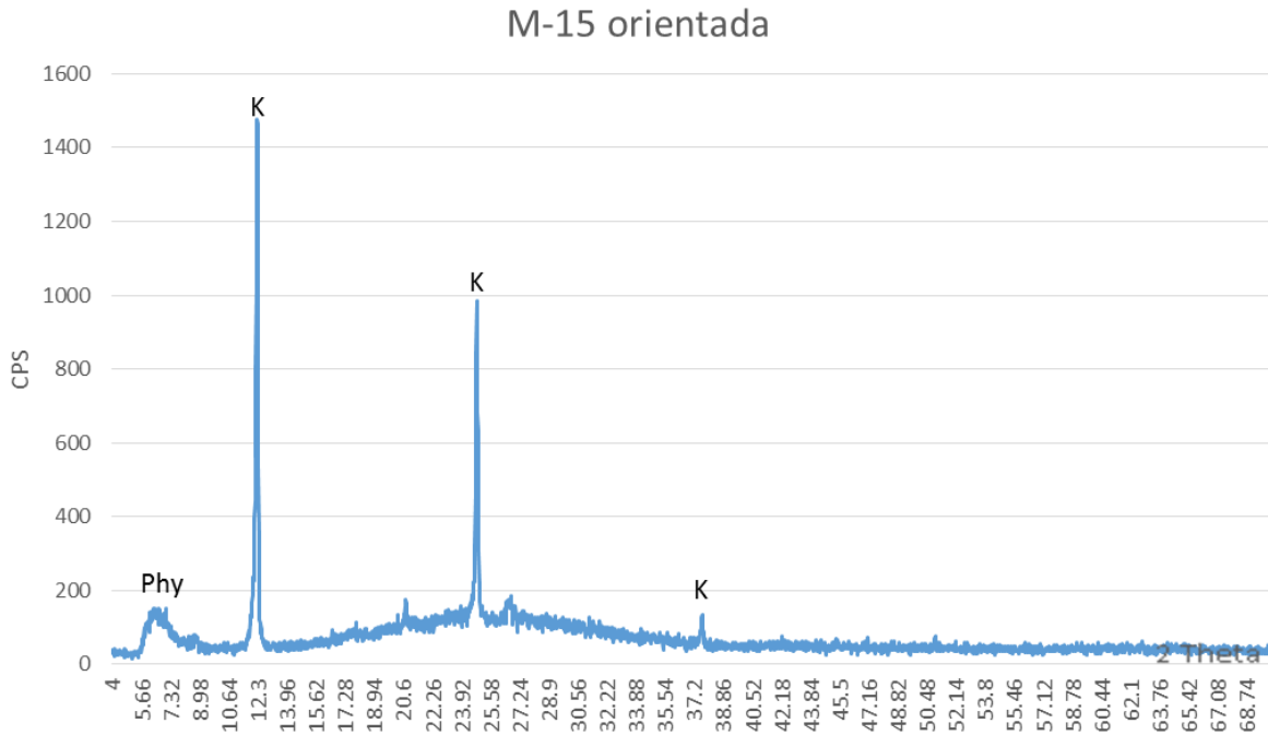
Figura 4.16. Identificación del mineral caolinita (K) en la muestra M-15.
