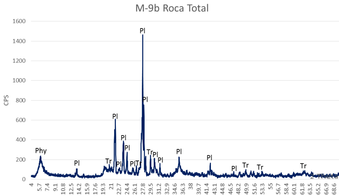
Figura 4.14. Plagioclasa (PI), tridimita (Tr) y filosilicatos (Phy) identificados en el difractograma por análisis de roca total de la muestra M-9b.
