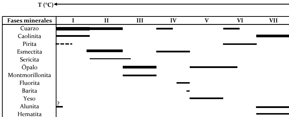
Figura 5.1. Secuencia paragenética de las muestras de roca de San Bartolomé de los Baños, Guanajuato (SBB). Las etapas que se presentan son: I) Argílica avanzada, II) Argílica, III) Argílica- sericitización, IV) Veta, V) Mineralización, VI) Sinter, VII) Supergénica. Las temperaturas en la secuencia oscilan entre los 100°C.
