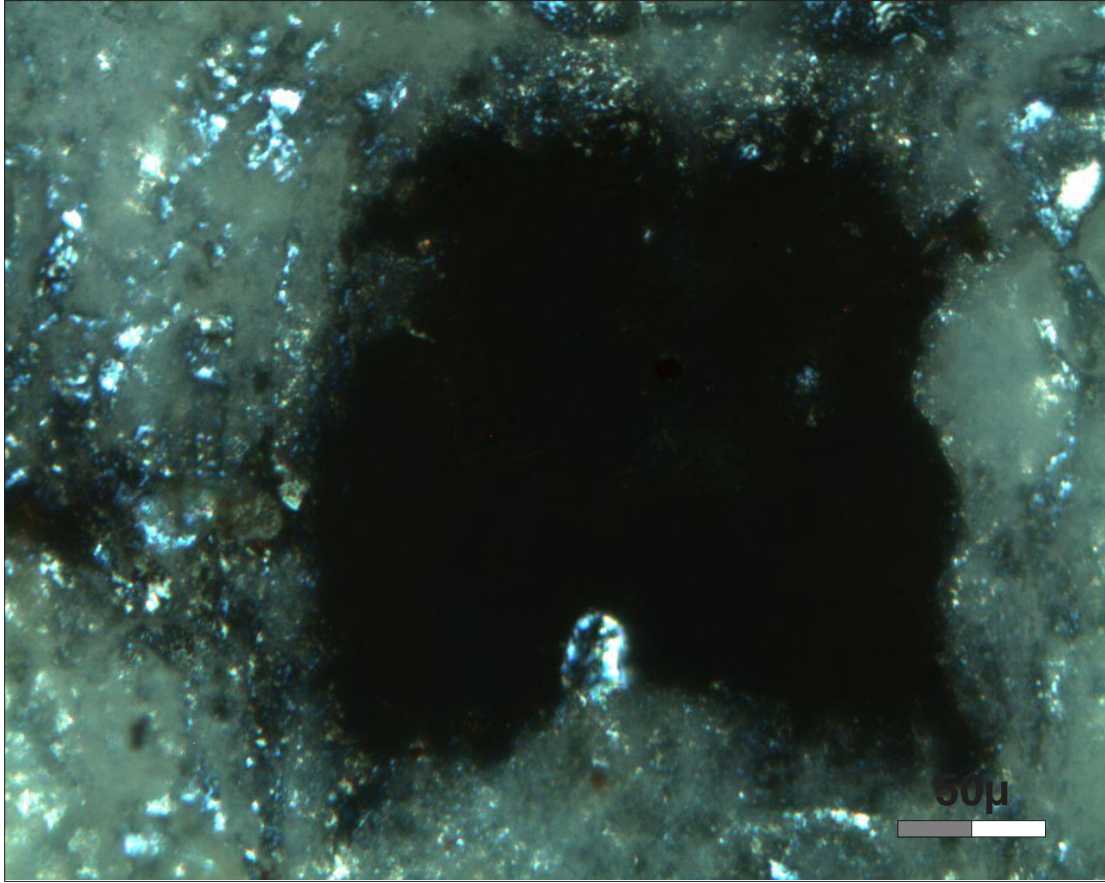
Cavidad formada por un cristal de pirita. Muestra: G-01, 20x.
