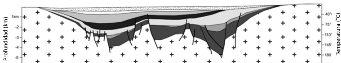
Figura 1.12 Configuración típica de una cuenca sedimentaria intracratónica con varias depresiones o subcuencas (Best Practices Guide For Geothermal Exploration, IGA, 2014).
