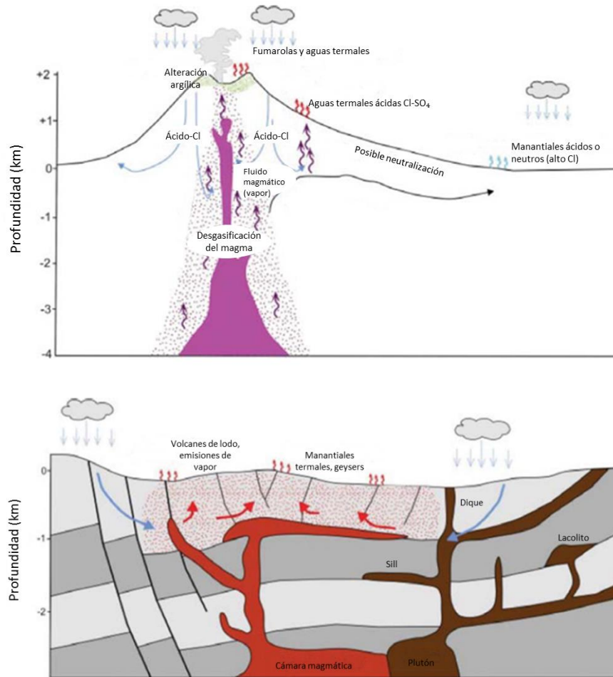
Figura 1.9 Ejemplos de un play activo o de intrusión magmática reciente (Best Practices Guide For Geothermal Exploration, IGA, 2014).
