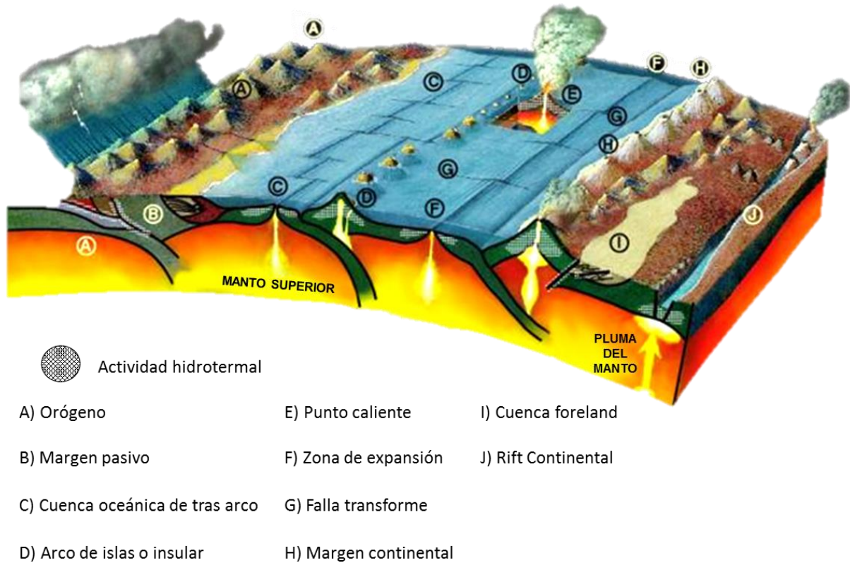
Figura 1.5. Dibujo representativo de la actividad tectónica que existe en la litósfera señalando los límites e interacción entre placas [5].
