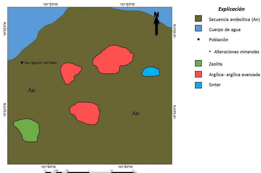
Figura 3.11. Mapa de distribución de las alteraciones en la zona de San Agustín Del Maíz, Michoacán.
