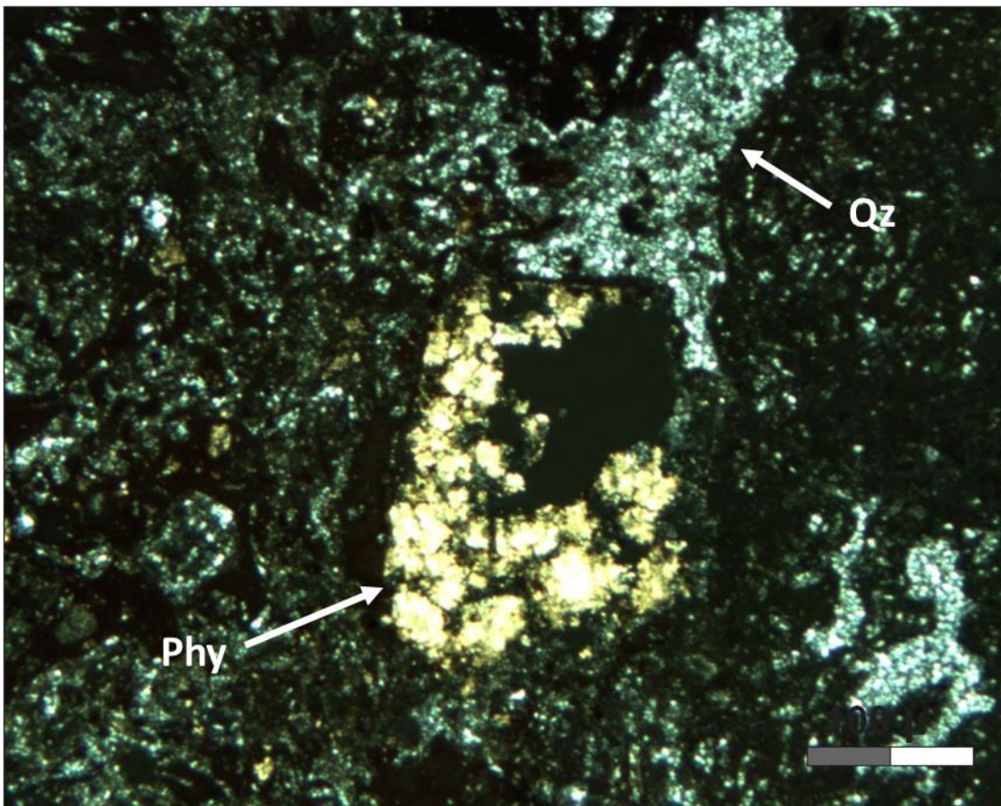
Feldespatos alterados reemplazados por arcilla y alunita. G-29, 2.5x.
