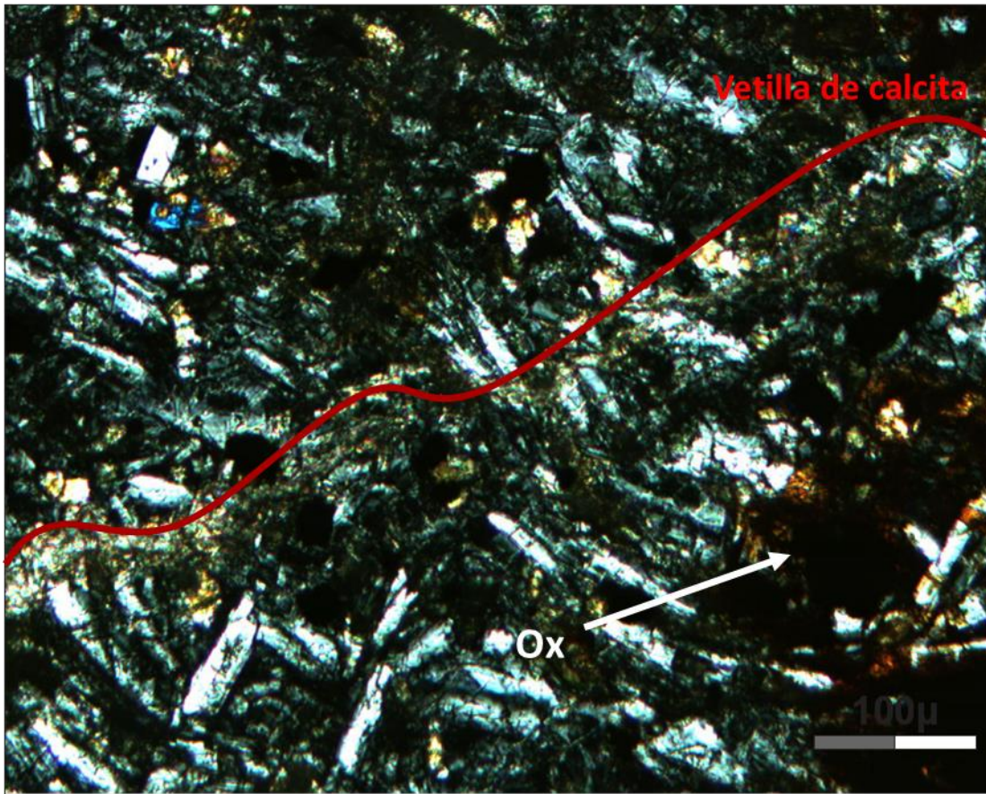
Vetilla de calcita que cruza de izquierda a derecha y en la parte inferior derecha hay presencia de oxidación. Muestra: M-8, 10x.
