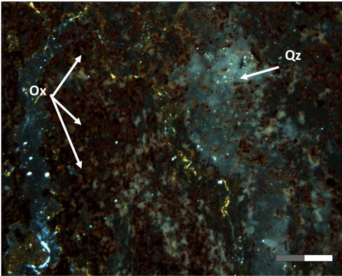
Oxidación la cual se presentó por la precipitación de óxidos posterior a la roca. Muestra: G-01, 2.5x.
