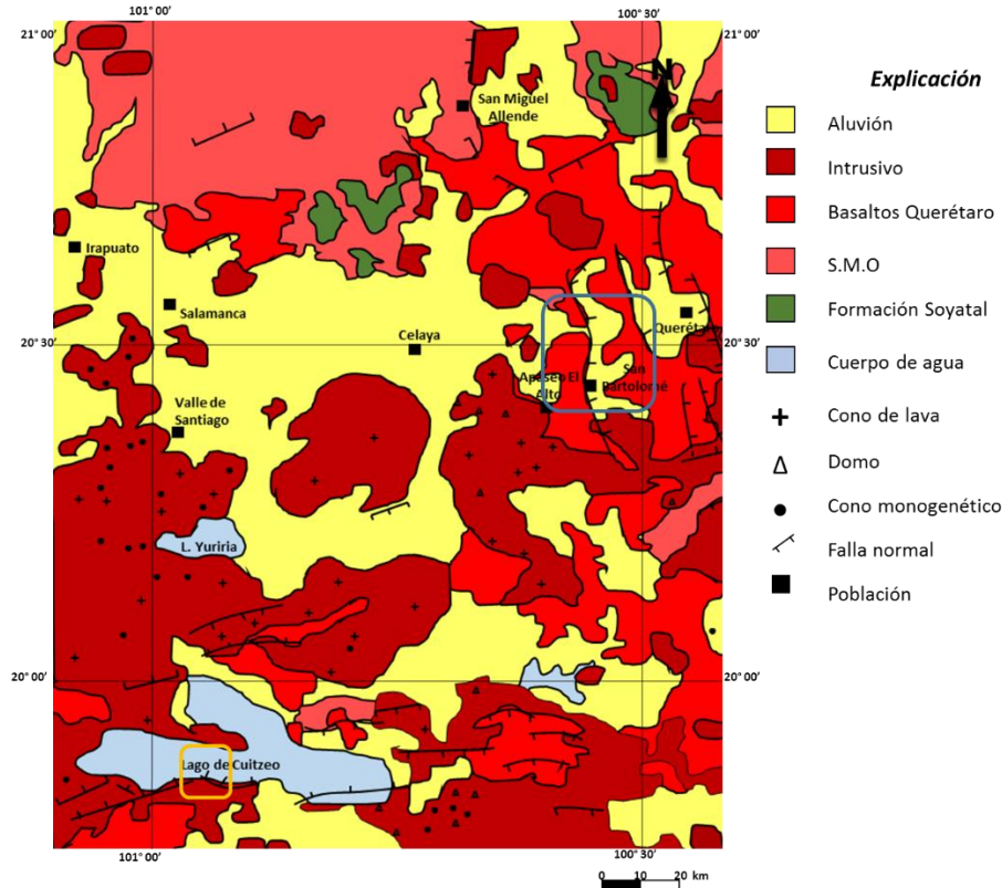
Figura 3.4 . Mapa geológico de la región centro occidental de la FVTM adaptada de López, 1996. Se marca en un recuadro azul la ubicación de la zona de estudio relacionado San Bartolomé de los Baños y la falla San Bartolomé que pertenece al sistema de fallas Taxco-San Miguel de Allende y en otro recuadro amarillo la región de estudio de Cuitzeo.
