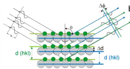
Figura 2.9. a) Ecuación de Bragg. b) Descripción del modelo de Bragg cuando se trata de secuencias de planos del mismo espaciado, pero formados a su vez por átomos de distinto tipo, separados por \Delta d . Esta separación geométrica origina diferencias de fase dentro de un mismo haz difractado que provoca interferencias y que dan lugar a variaciones de intensidad (según la dirección), lo que permite obtener información de la estructura de los átomos que forman el cristal (Consejo Superior de Investigaciones Científicas, 2015).
