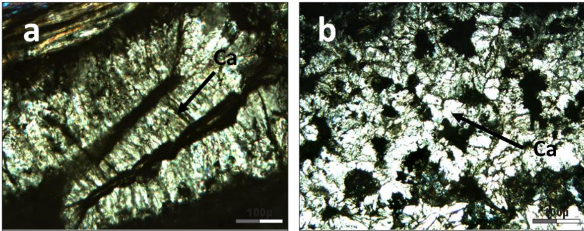
a) y b) Calcita normal con magnesio. Muestra: M- 13a, 10x.
