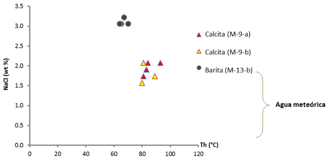
Figura 4.18. Diagrama de dispersión de temperatura de homogeneización Th(°C) vs salinidad NaCl (wt%) en la zona de San Agustín del Maíz. De acuerdo a diagrama se presenta un proceso de dilución durante la precipitación de carbonatos en la alteración, siendo un pulso hidrotermal diferente para el caso de la barita. Esta disolución se corrobora con las observaciones texturales de los precipitados hidrotermales, donde la barita no se encuentra en el mismo evento paragenético con la calcita.
