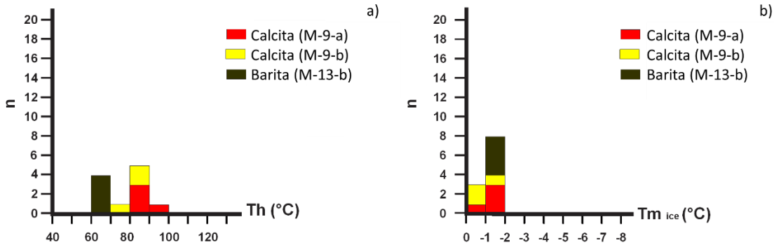
Figura 4.19. a) Histograma de temperatura de homogenización Th (°C) y b) temperatura de fusión del hielo Tm ice (°C), vs frecuencia absoluta "n".
