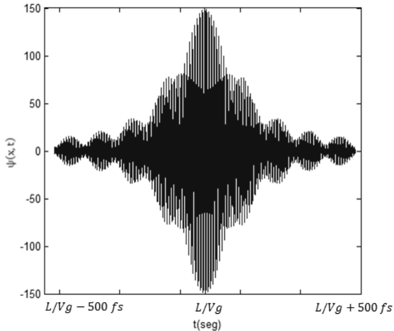
Figura 1.10.- Pulso que se propaga en vidrio BK7. La amplitud de las frecuencias es la misma.
