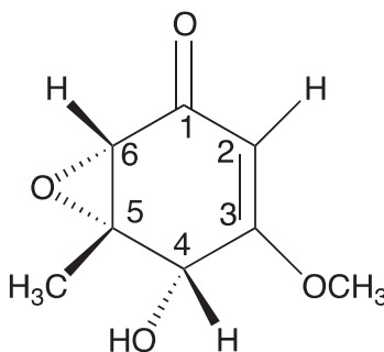
Figura 28. (4S,5S,6S)-5,6-epoxi-4-hidroxi-3-metoxi-5-metil-2-ciclohexen-1-ona ( 70 )
