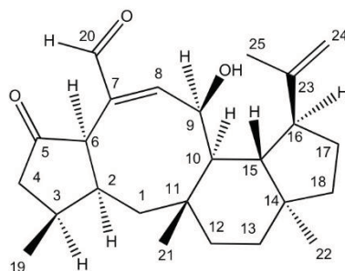
Figura 40. variecolina A
