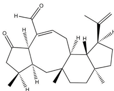
Figura 41. variecolina
