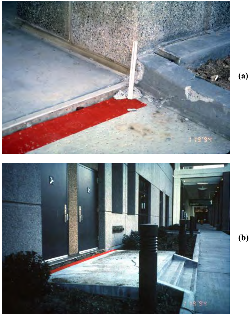
Fig 2.11 a) Acercamiento al asentamiento provocado por licuación del suelo, b) panorama abierto del mismo caso de estudio (Lew y Tran, 2012)
