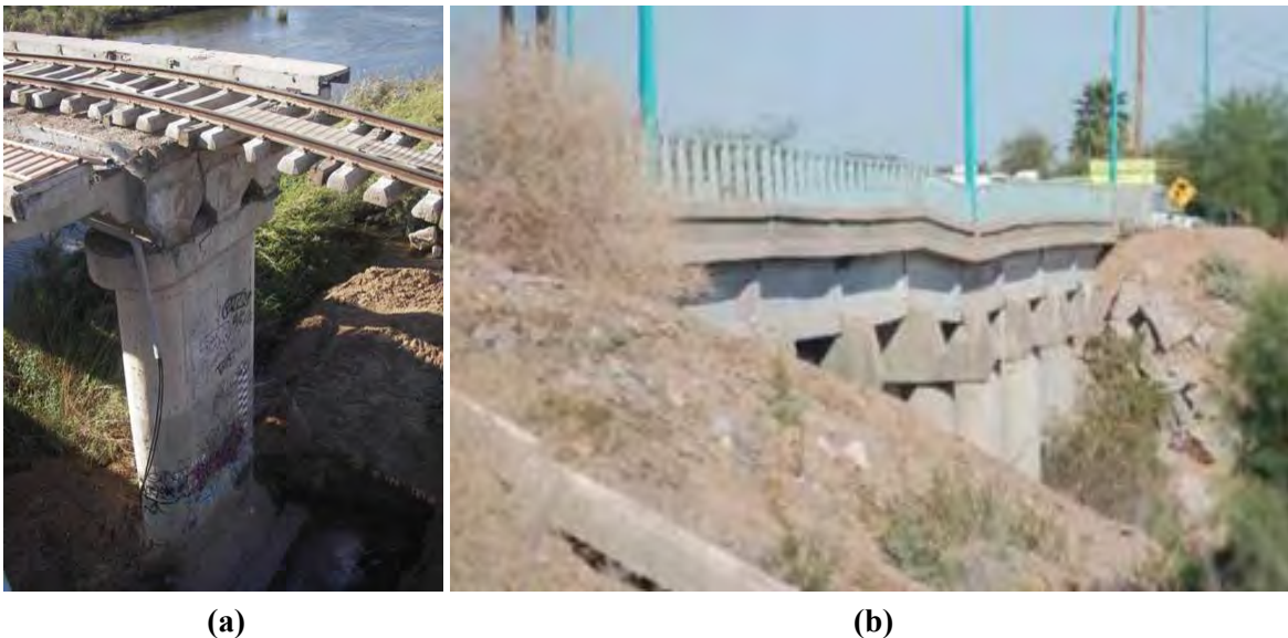
Fig 2.37 a) Tramo colapsado debido al desplazamiento lateral en el puente ferroviario San Felipito, b) puente San Felipito (carretero) con asentamientos diferenciales en las pilas que lo soportan (GEER Association, 2010b)
