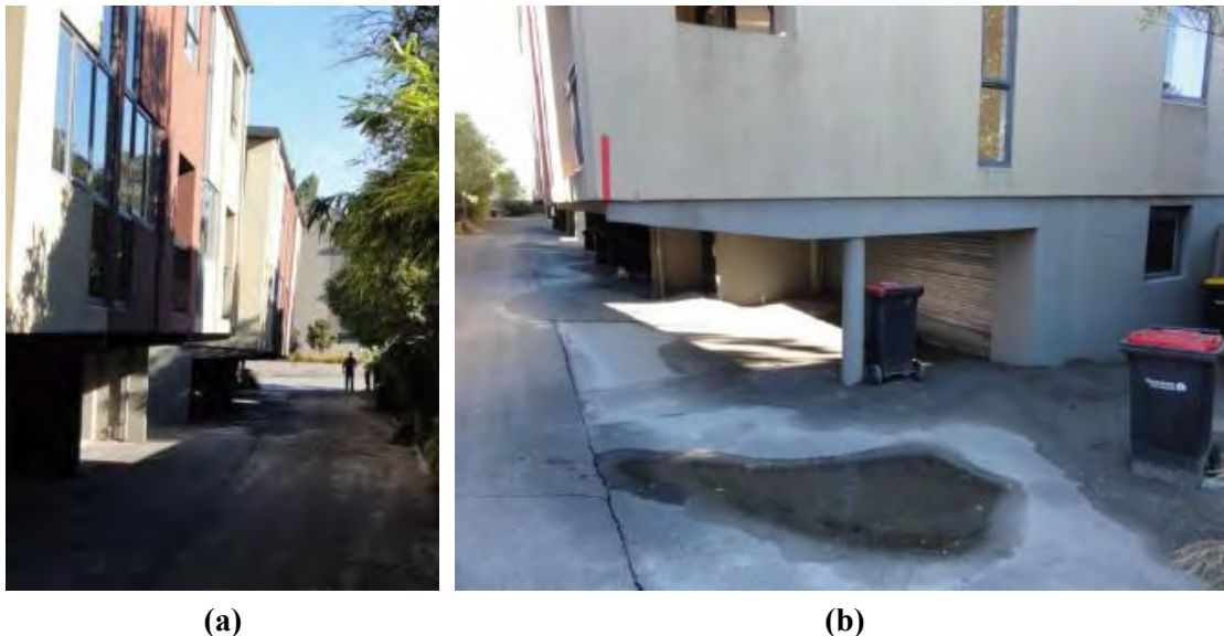
Fig 2.48 a) Asentamiento e inclinación en edificio de tres niveles, b) material eyectado producto de la licuación del suelo inducida por el sismo (GEER Association, 2011a)
