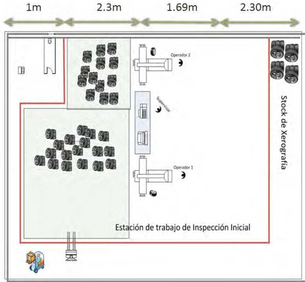
Figura 4.5. Área de las propuestas de distribución 1,2 y 3 en inspección inicial.
