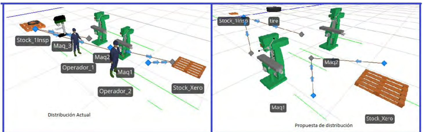
Figura 12 Propuestas de distribución en la estación de inspección inicial.
