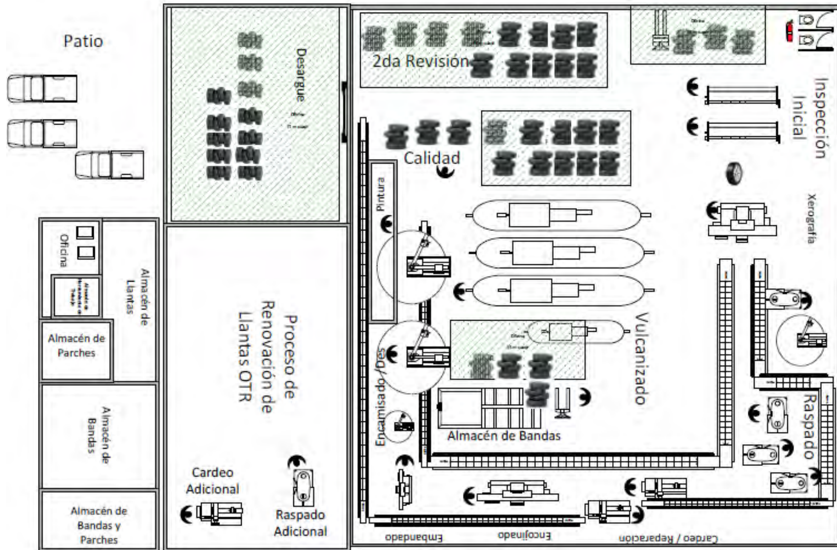
Figura 3.2. Distribución actual de la planta Fuente: Elaboración propia con apoyo del programa Visio.
