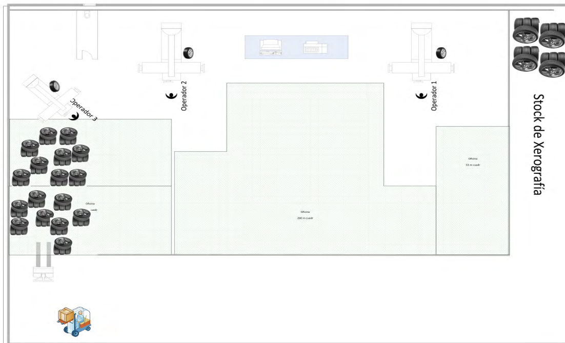
Figura 13. Distribución actual de inspección inicial
