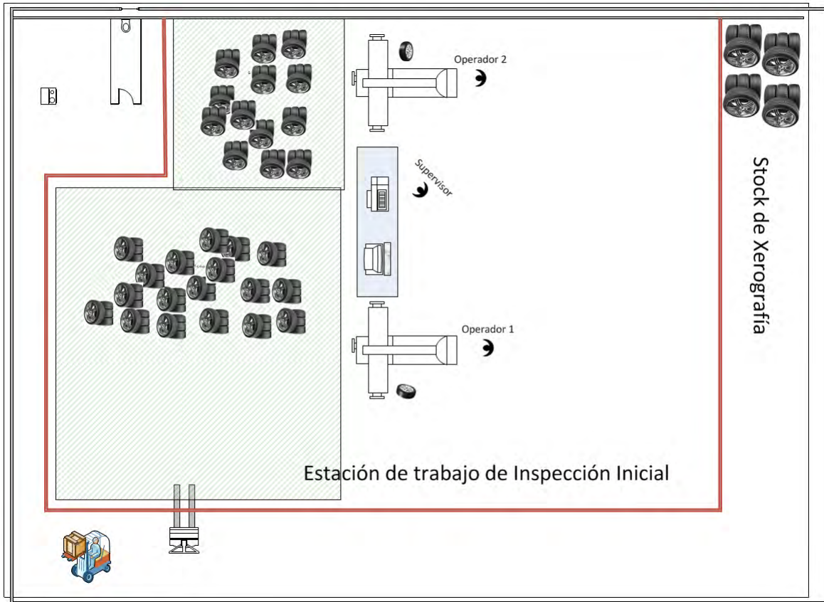
Figura 4.4. Propuestas de una nueva distribución en Inspección inicial.
