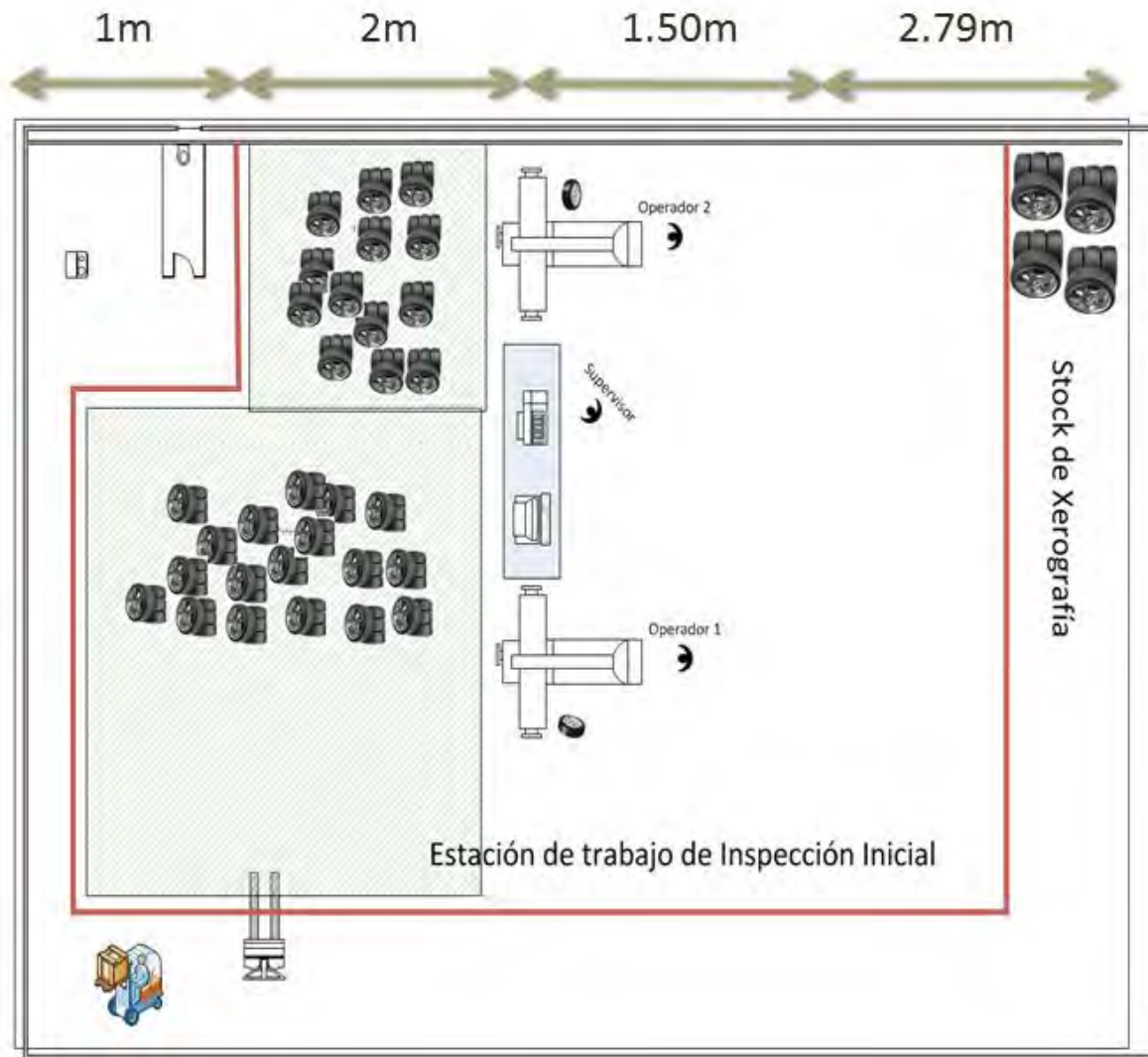
Figura 4.6. Área de las propuestas de distribución 4,5 y 6 en inspección inicial.
