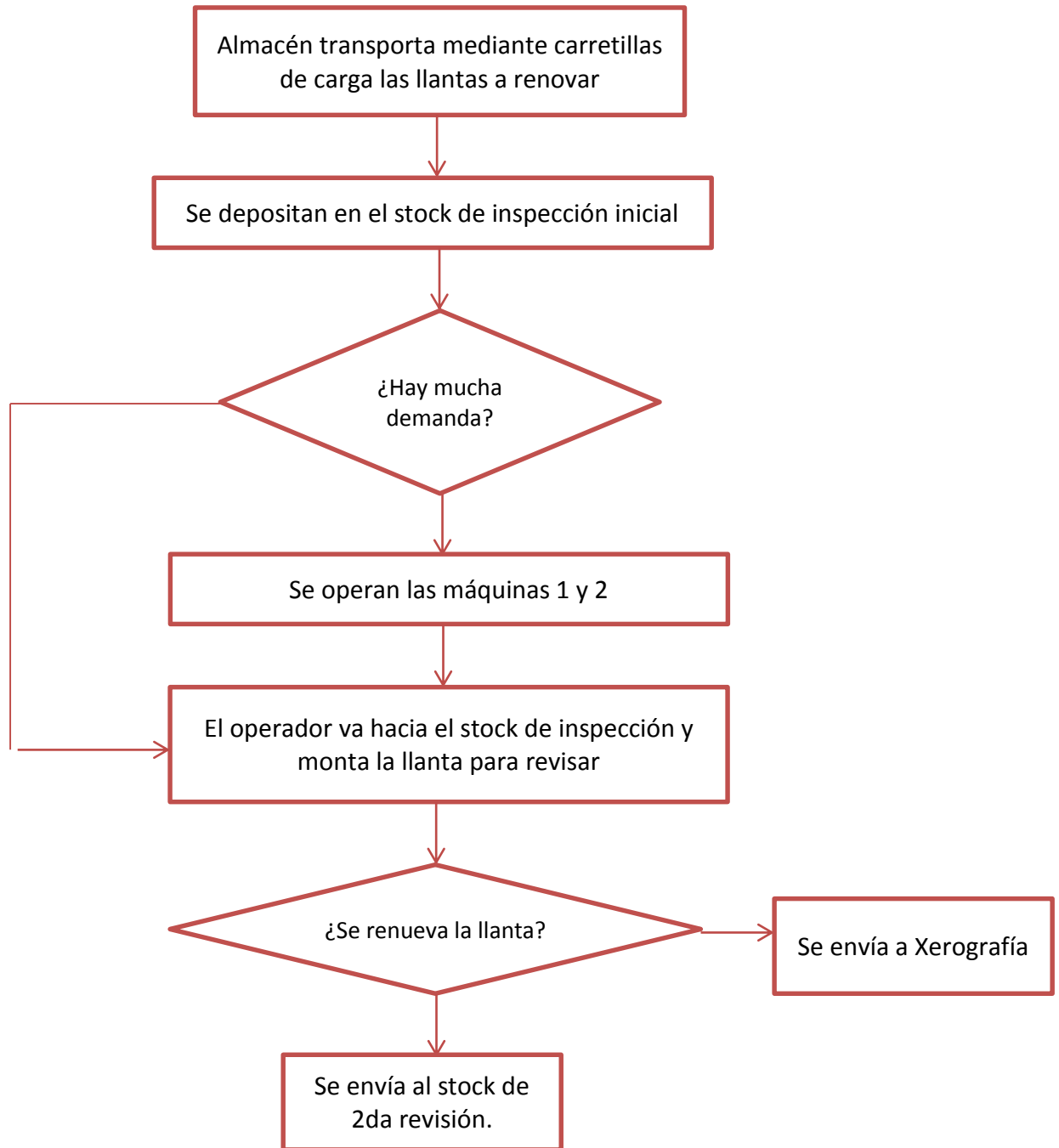
Figura 4.2. Flujo del proceso de inspección inicial
