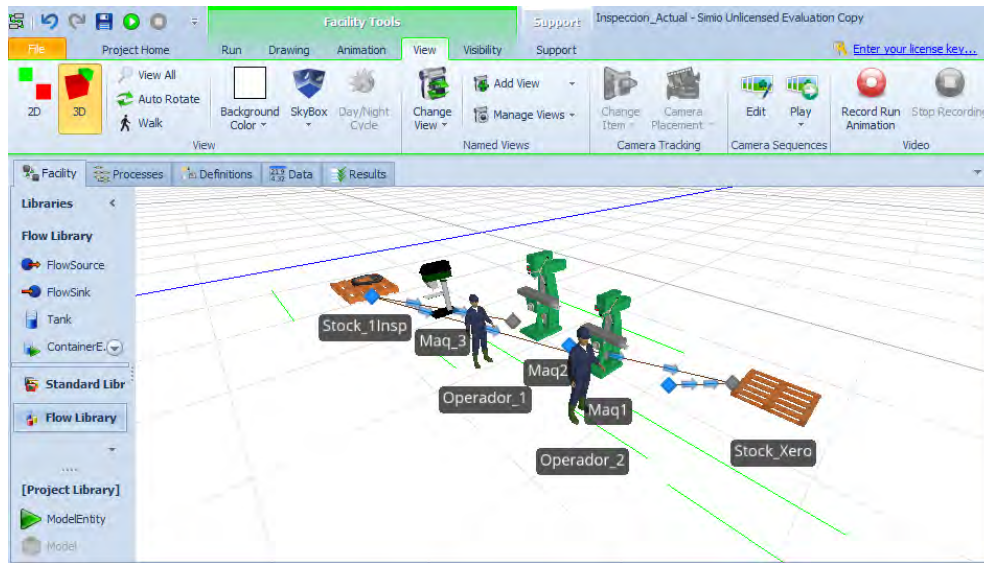
Figura 3.5. Distribución actual de Inspección inicial, representada en SIMIO.
