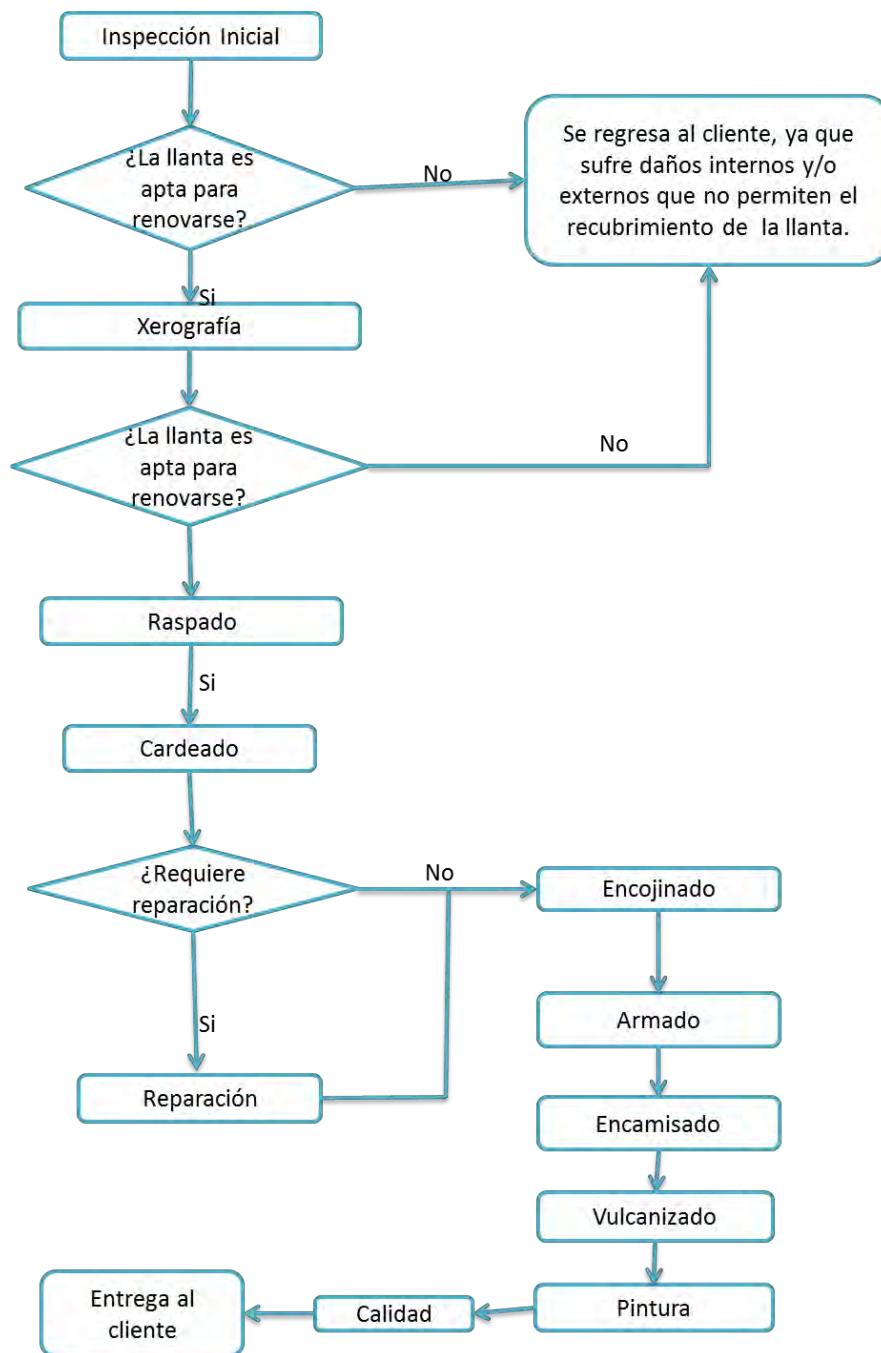
Figura 3.1. Proceso de renovación de Renovadora de México, S.A de C.V.
