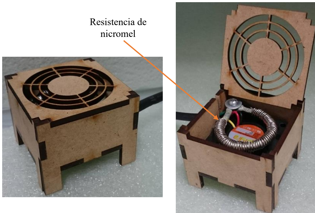
Fig. 3.13. Dispositivo calefactor.
