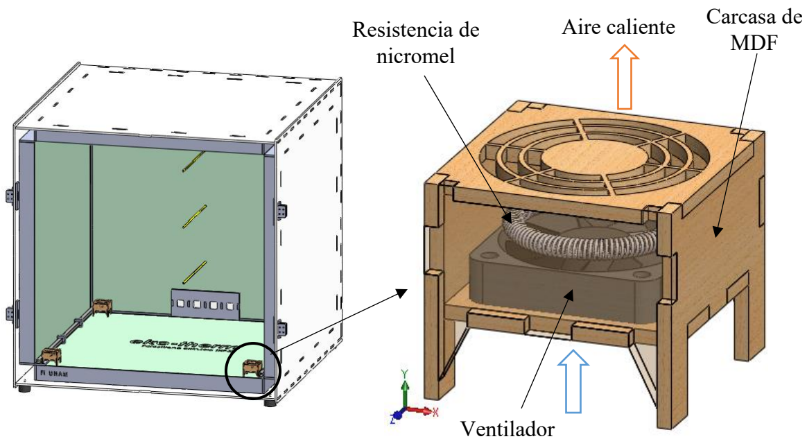
Fig. 3.9. Dispositivo calefactor.
