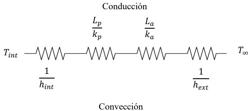
Figura 2.3. Circuito térmico equivalente.
