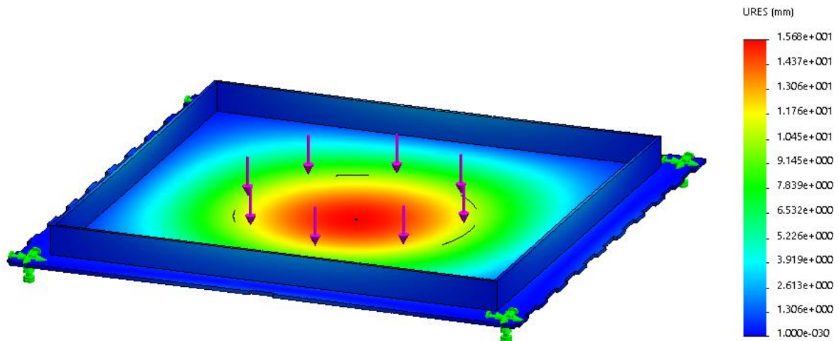
Fig. 3.8. Análisis de la base de la cámara.
