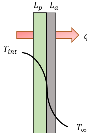
Fig. 2.2. Pared de la cámara de temperatura.
