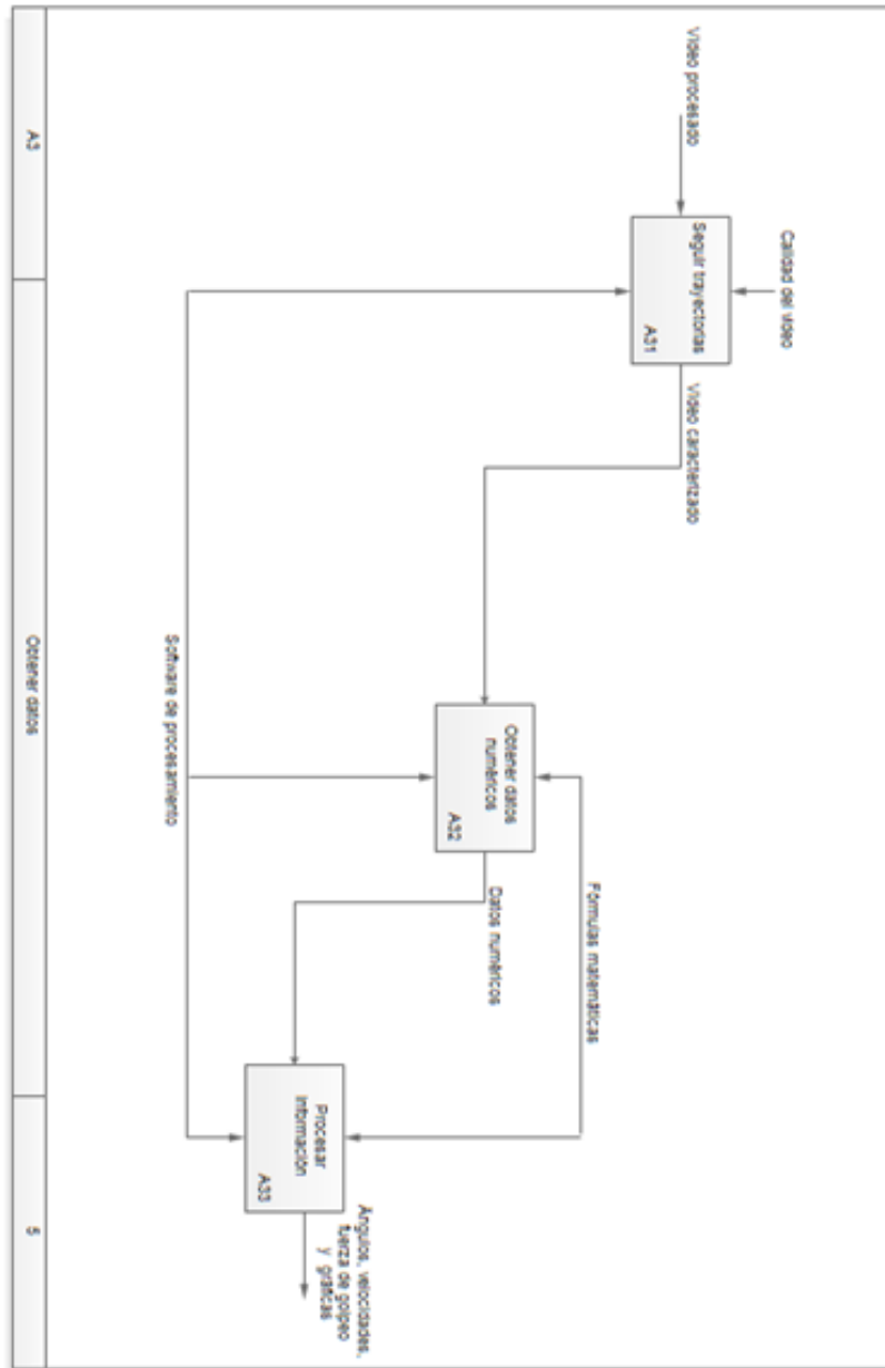
Figura 3.6. Diagrama nieta 3
