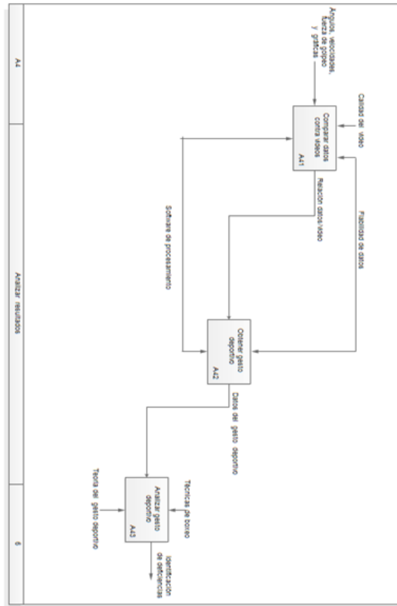
Figura 3.7. Diagrama nieta 4
