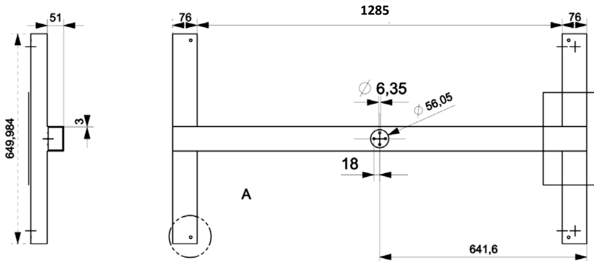
Figura 1.G. Vista inferior y de perfil de la base inferior
