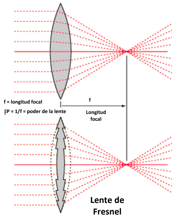
Figura F. Diferencia geométrica entre una lente biconvexa y una lente de Fresnel, el punto focal se encuentra a la misma distancia en este caso.
