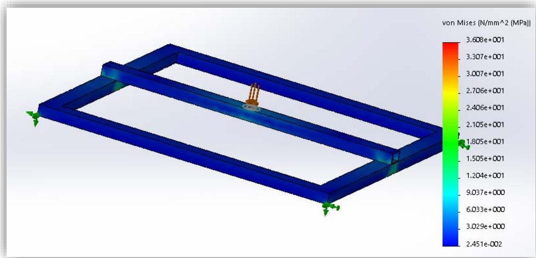
Figura 3.W. Vista diagonal de la base después del análisis mostrando tensiones de Von Mises
