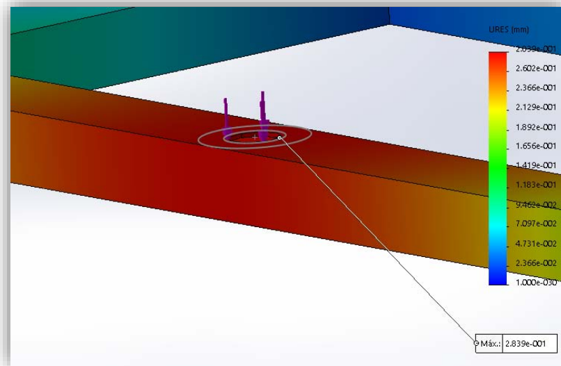
Figura 3.Z. Mayor desplazamiento por parte del perfil de acero central
