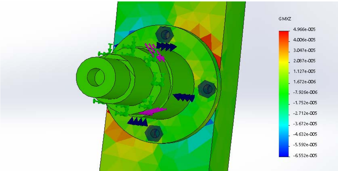
Figura 3.AF. Tensión cortante en dirección Z en el plano YZ
