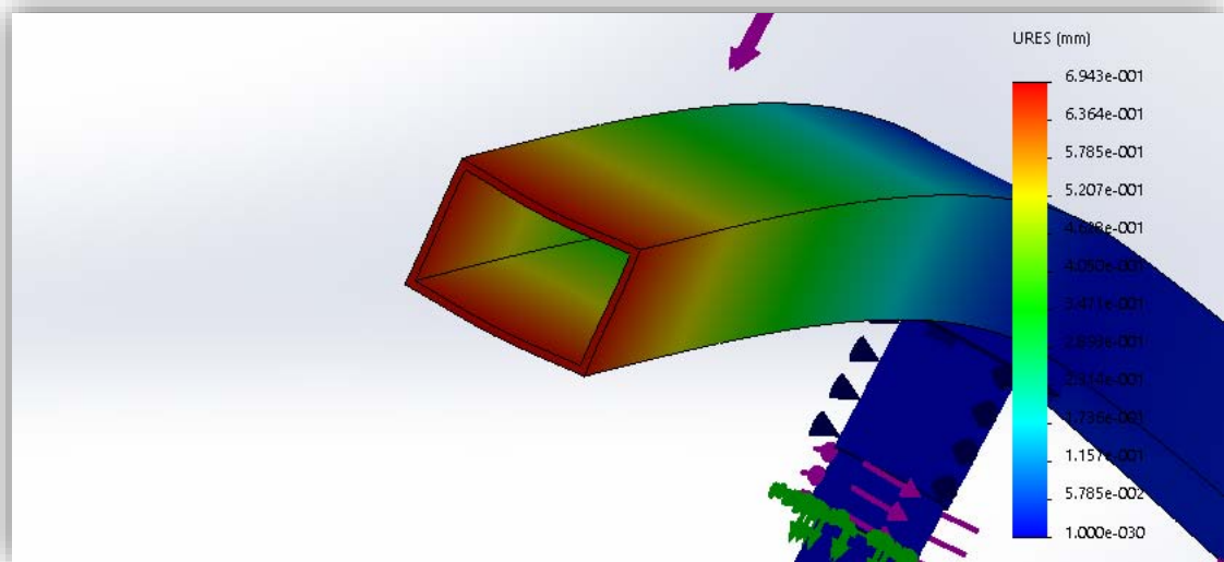
Figura 3.AJ. Máximo desplazamiento del PTR
