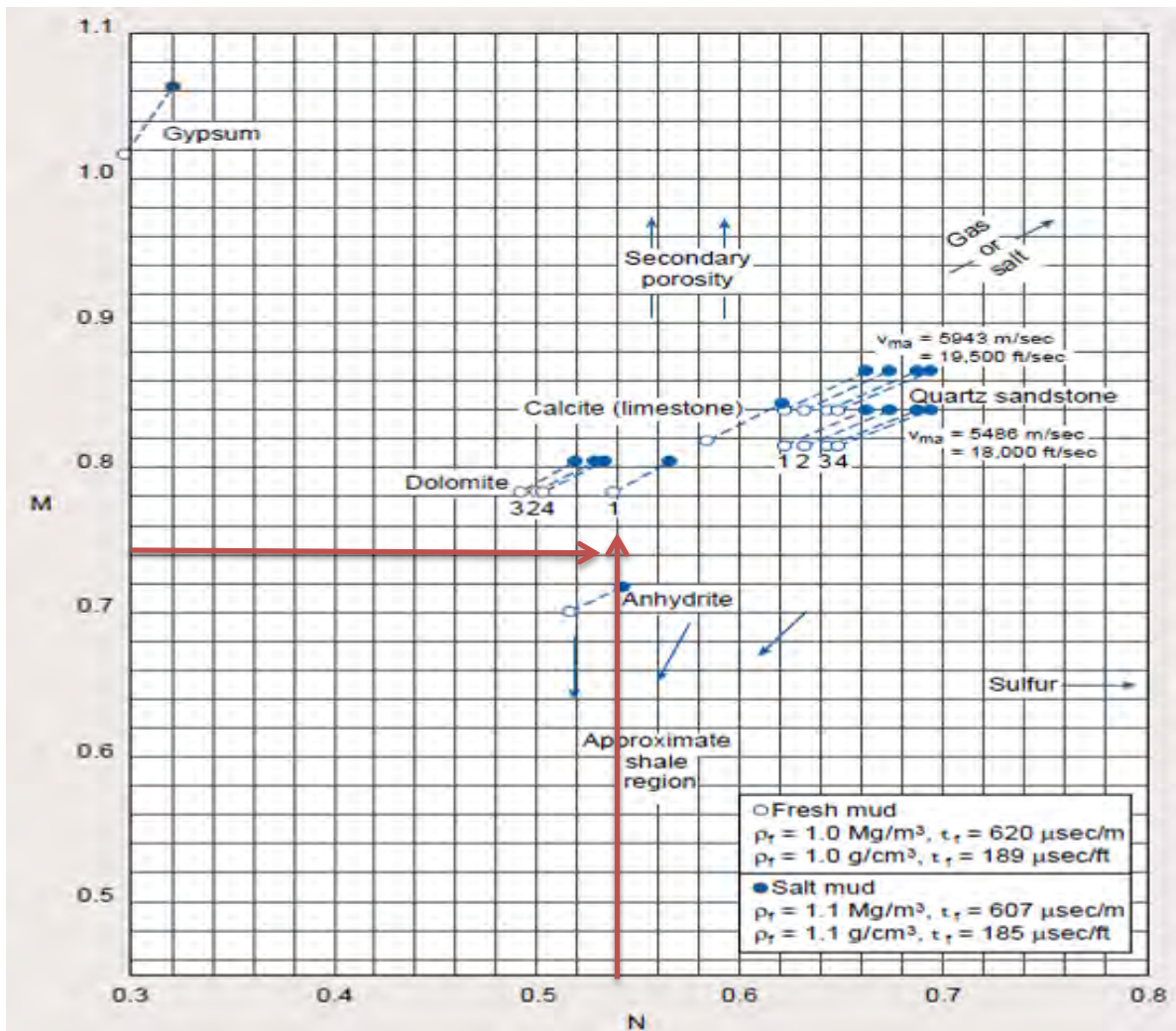
Gráfico de identificación de minerales M-N (Schlumberger, 2000)
