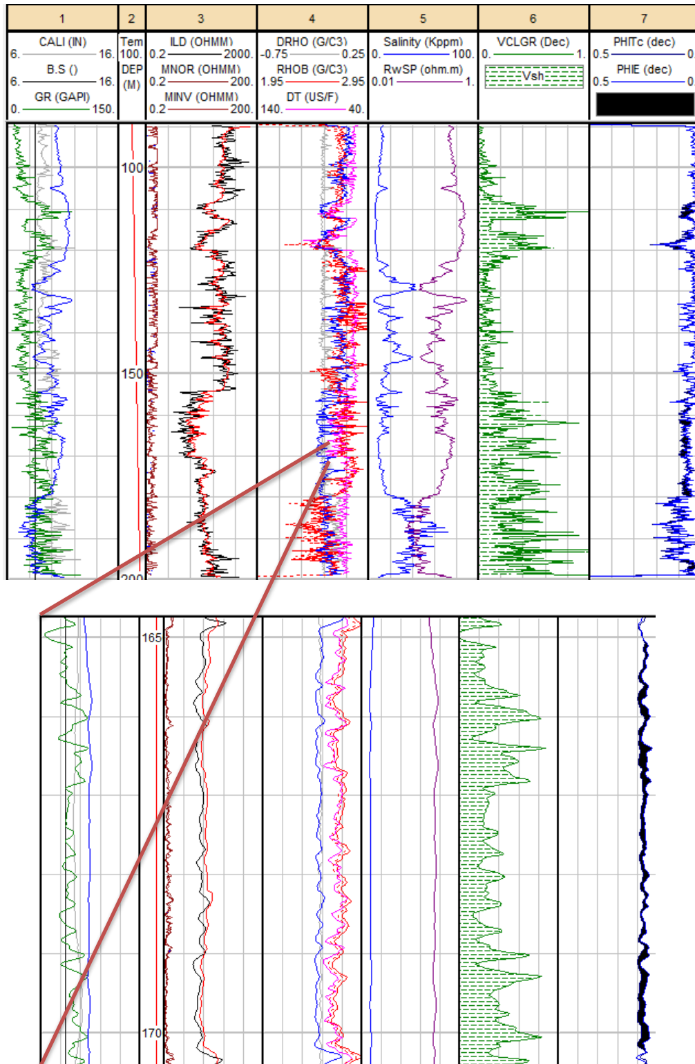
Figura 4.12.- Porosidad total y Porosidad efectiva (último track), se sombreó la diferencia de la curva de porosidad total y porosidad efectiva para visualizar la diferencia. Imagen de abajo está a una escala 1:500. Senergy, IP,2008.
