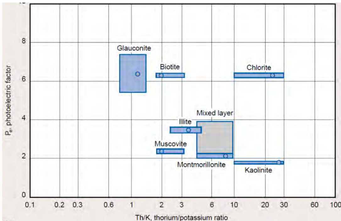
Gráfico de identificación de minerales arcillosos, minerales pesados. Th/K vs P_{ei} . (Schlumberger, 2000)
