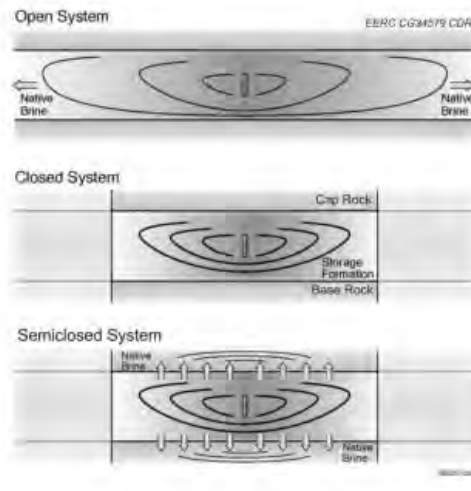
Figura 1.3.- Diagrama representativo de tres potenciales sistemas de entrapamiento en formaciones salinas (Zhou et al, 2008)
