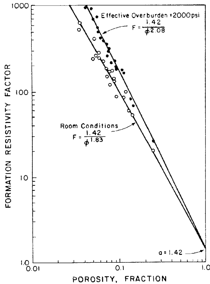
Fig. 2.6.- Relación entre \phi y F (Archie, 1952)
