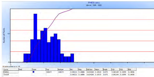
Figura 5.12.- a) Histograma de la porosidad efectiva, b) histograma de la permeabilidad con de la formación San Andrés. (Senergy, 2008)
