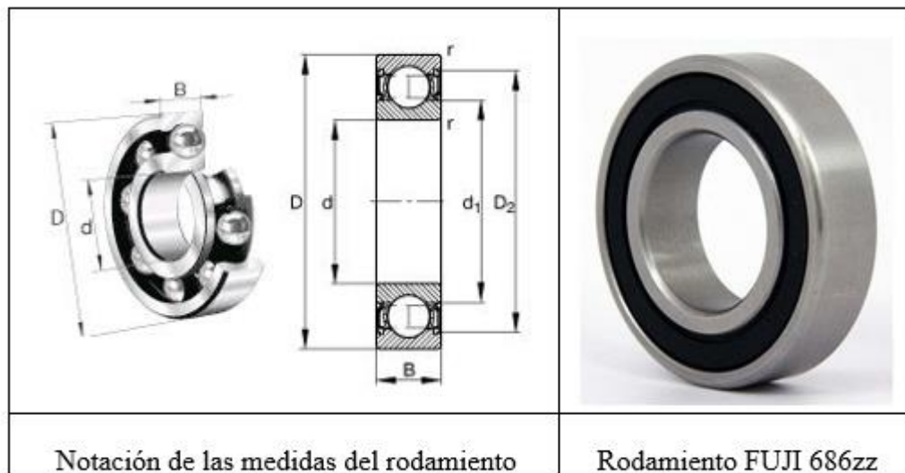
Imagen 3.5 Dimensiones del rodamiento FUJI 686z
