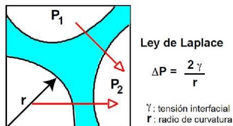
Fig. 26 Ecuación de Young- Laplace (FIRP #263)
