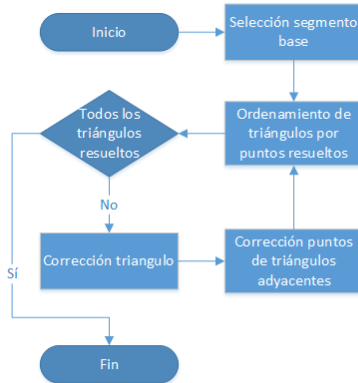
Ilustración 3.13. Diagrama de dimensionamiento
