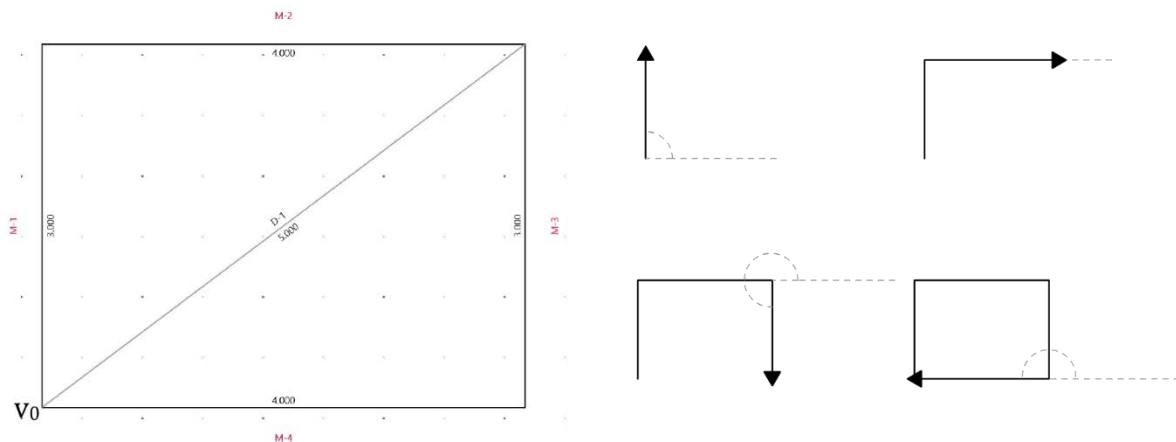
Ilustración 4.1. Dibujado de geometría de acabado. La geometría inicia en v_0 (x_0, y_0) y sigue la secuencia indicada por los vectores del lado derecho de la imagen
