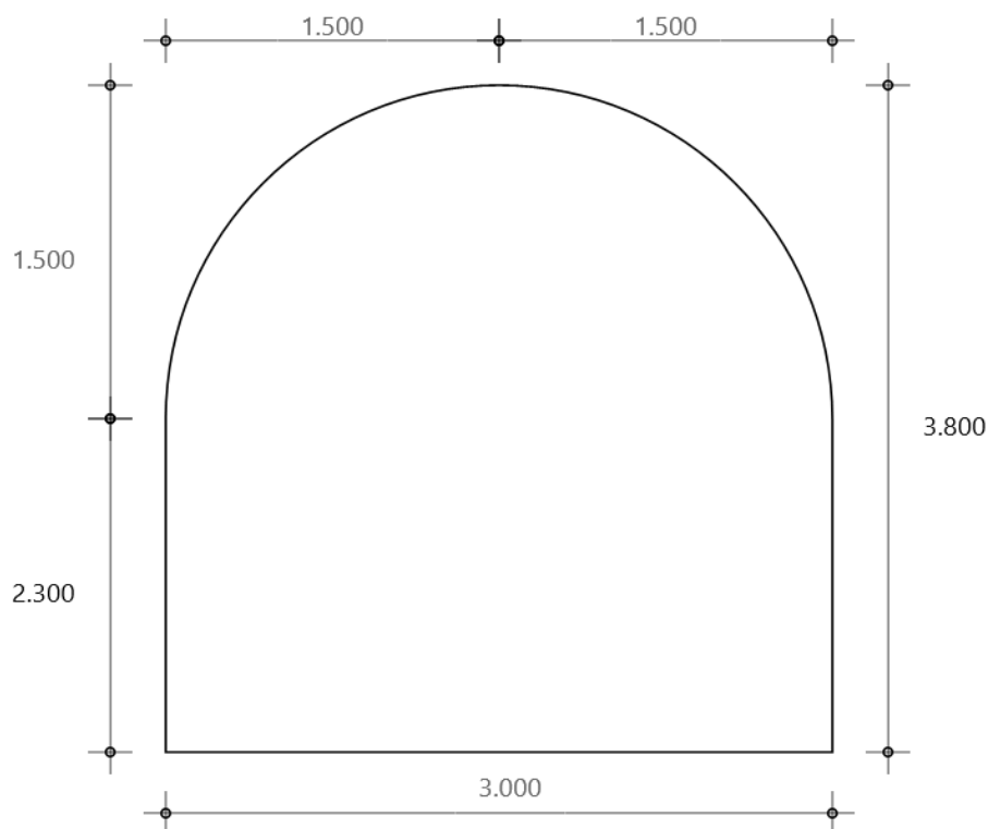
Ilustración 8.24. Dimensiones de muro con arco
