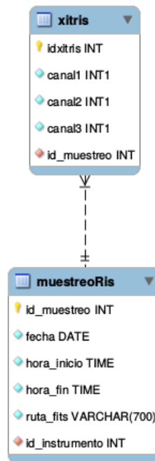
Figura 5.3: Tablas involucradas para el RIS
