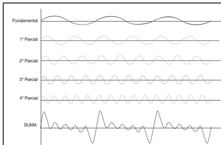
Figura (4.6) Onda senoidal distorsionada como suma de la fundamental y sus armónicas.
