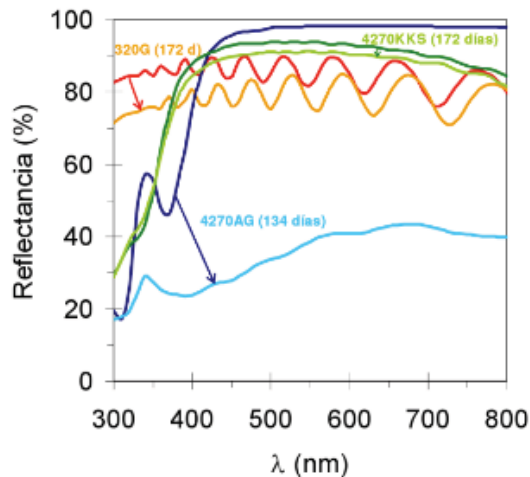
Fig. 33 Reflectancia del aluminio 320G, 4270AGy 4270KKS (Alanod Aluminium GmbH) y pérdida sufrida después de varios meses de envejecimiento en la cámara QUV 21
