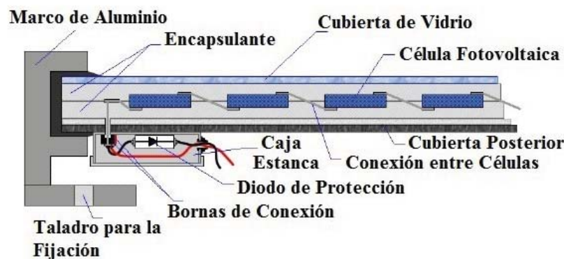
Fig. 22 Elementos de un panel fotovoltaico 9
