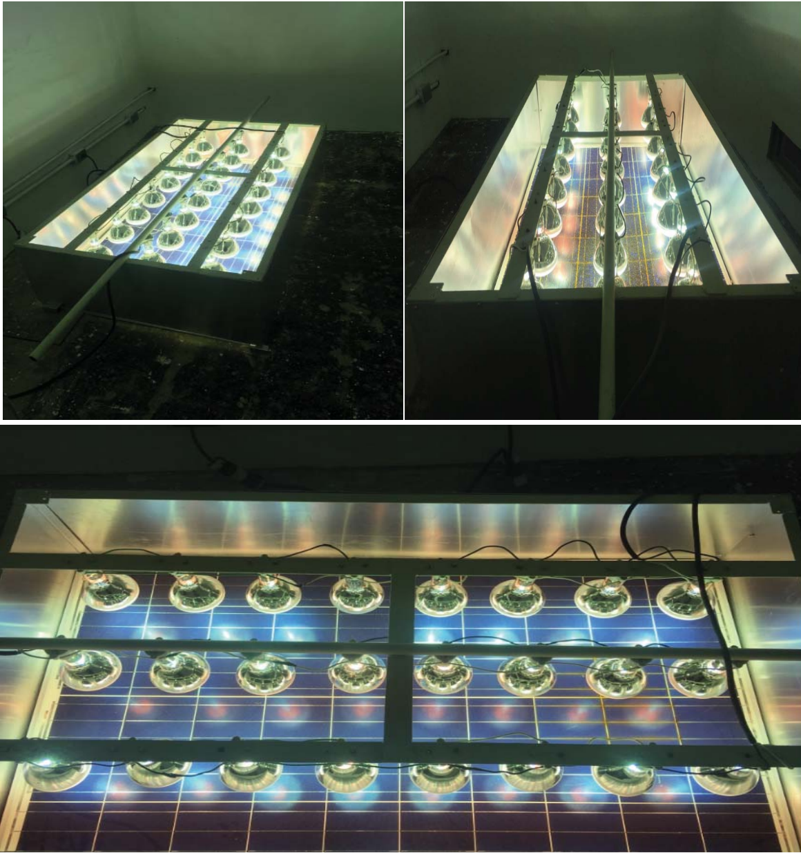
Fig. 41 Operación de la cámara de envejecimiento
