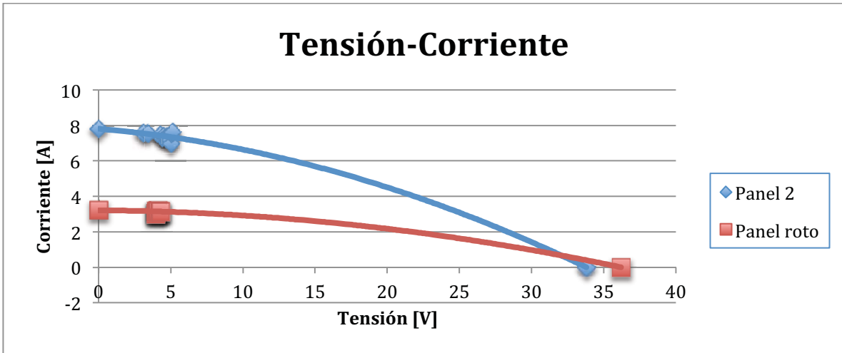
Gráfica 9 Curvas tensión-corriente
