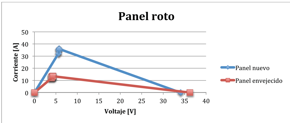
Gráfica 12 Diferencia en la potencia de salida del panel roto
