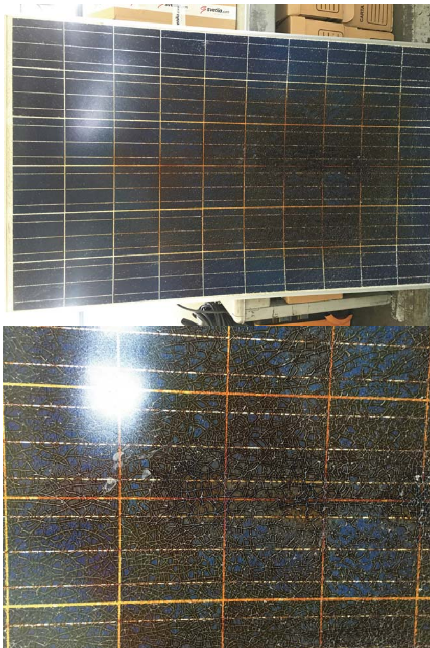
Fig. 46 Panel roto envejecido, parte frontal
