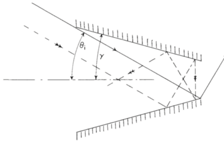
Fig. 29 Esquema de un concentrador cónico 17
