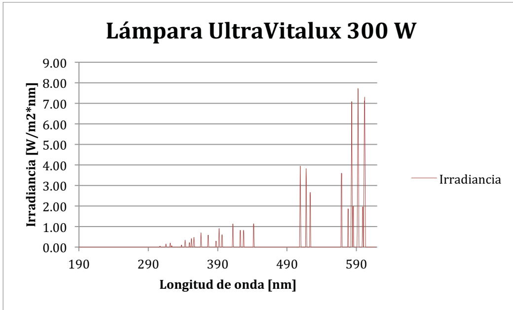
Gráfica 2 Espectro lámpara Ultravitalux
