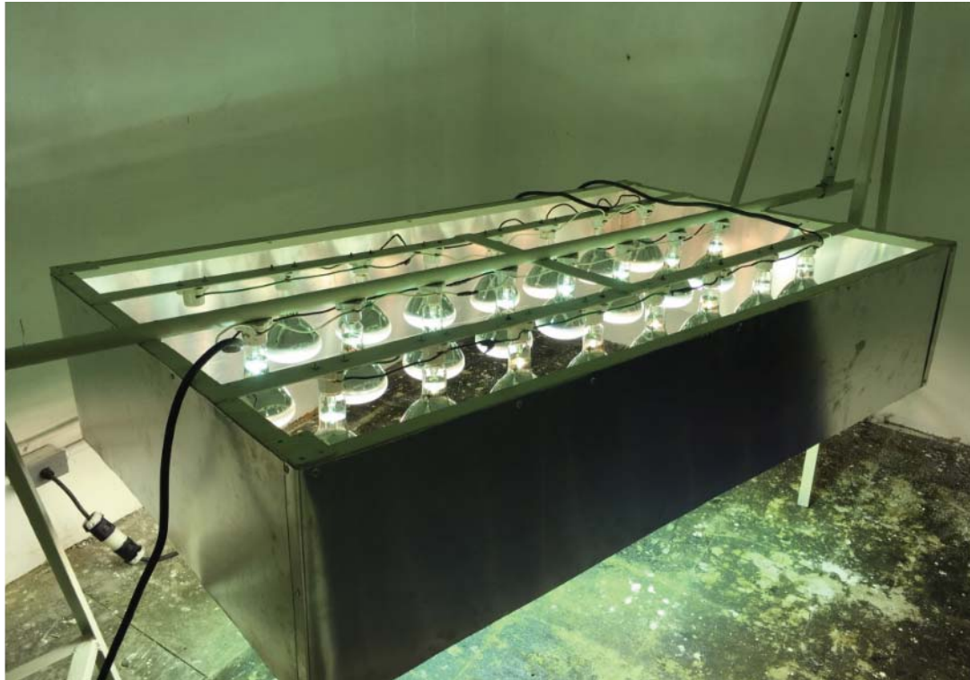
Fig. 35 Funcionamiento cámara de envejecimiento
