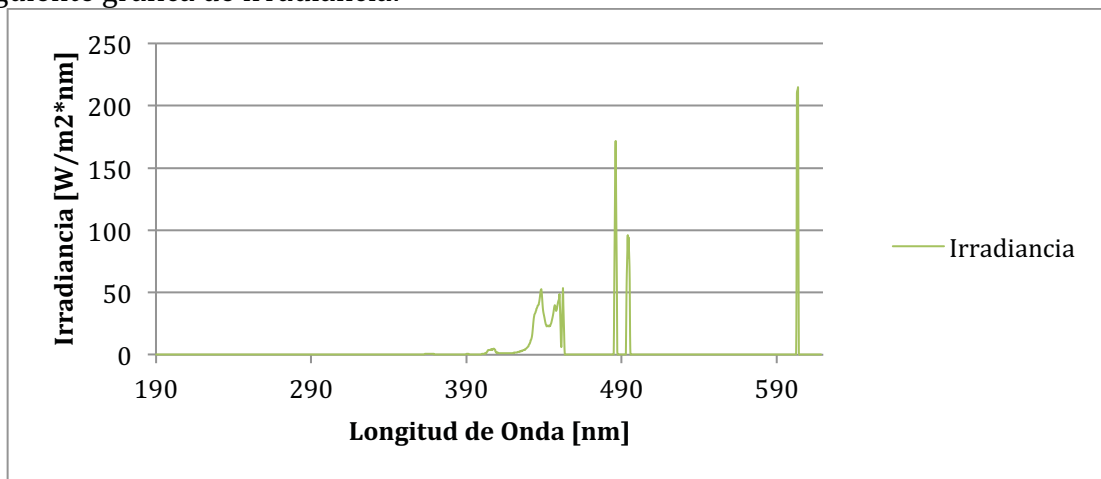
Gráfica 4 Espectro cámara de envejecimiento
