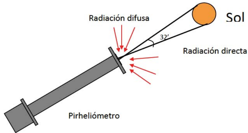
Fig. 15 Funcionamiento piranómetro 5
