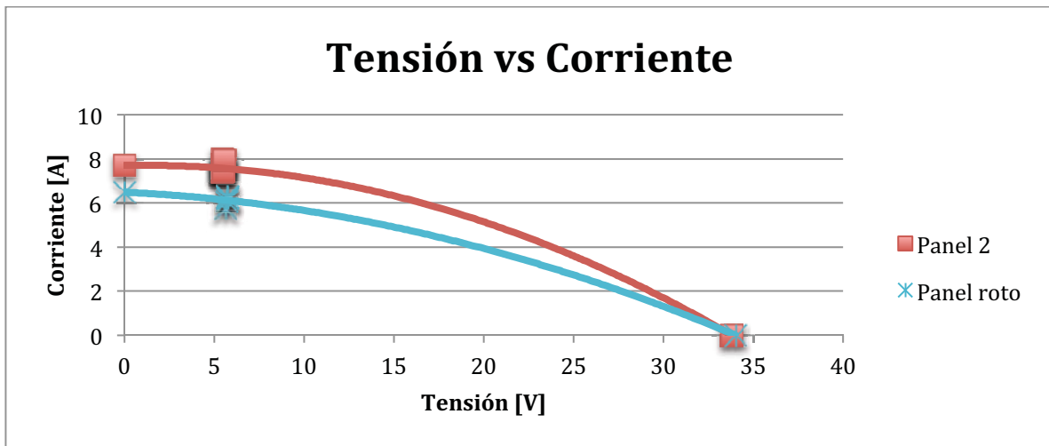
Gráfica 6 Curvas características paneles fotovoltaicos
