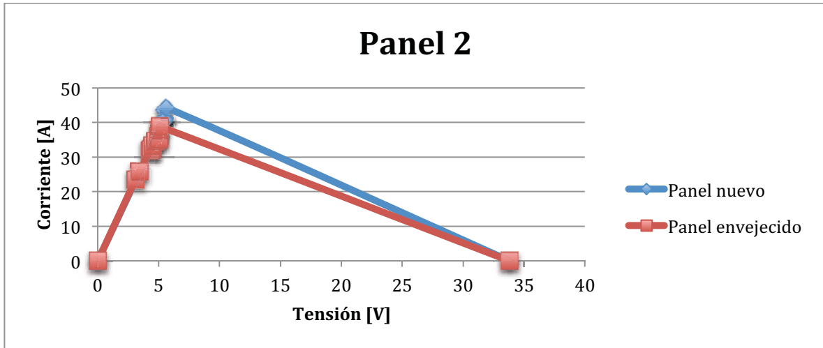
Gráfica 11 Diferencia en la potencia de salida del panel 2
