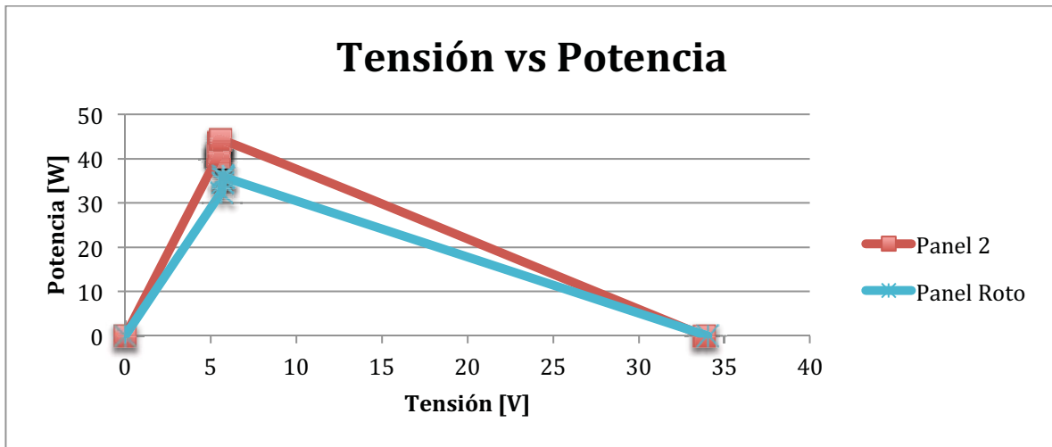
Gráfica 7 Curva de tensión vs potencia paneles fotovoltaicos
