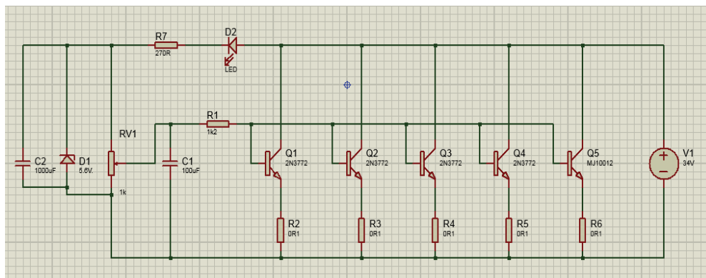
Fig. 38 Circuito carga variable
