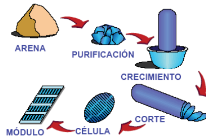
Fig. 12 Proceso de fabricación 9
