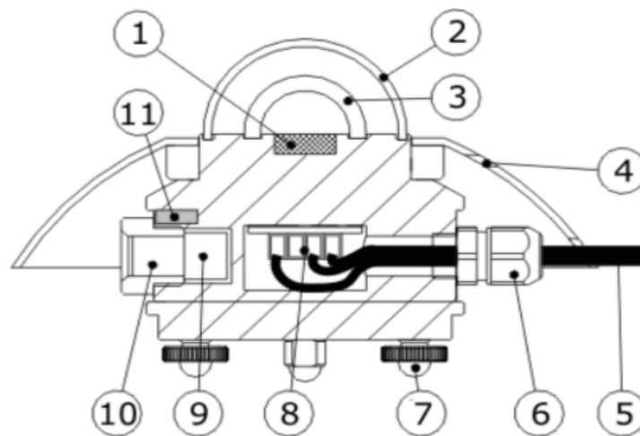
Fig. 16 Componentes de un piranómetro: 1 termopila, 2 cúpula exterior, 3 cúpula interior, 4 cuerpo, 5 cable, 6 conector, 7 tornillos de nivelación, 8 circuito, 9 desecante, 10 tapa del desecante, 11 nivel 11
