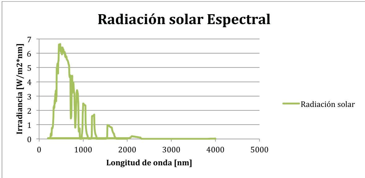
Gráfica 5 Radiación solar 04-02-2016
