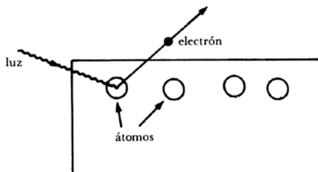
Fig. 6 Efecto Fotoeléctrico 2
