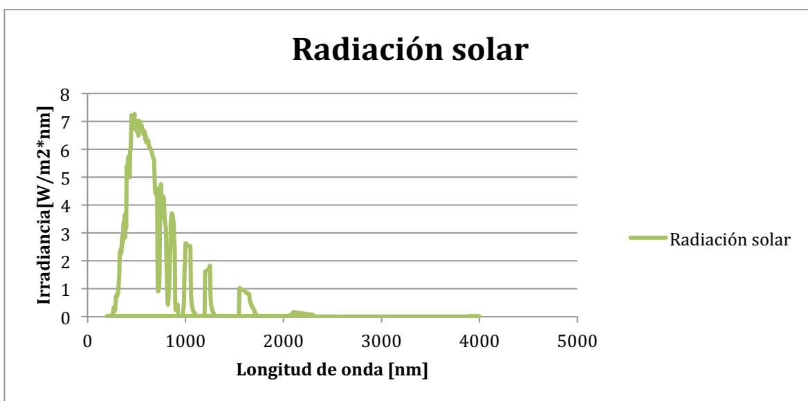
Gráfica 8 Radiación solar 04-08-2016
