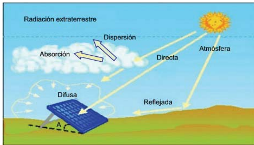
Fig. 5 Componentes de la radiación
