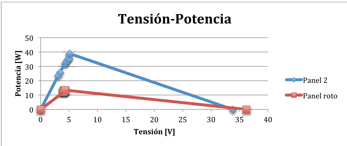
Gráfica 10 Curvas tensión-potencia
