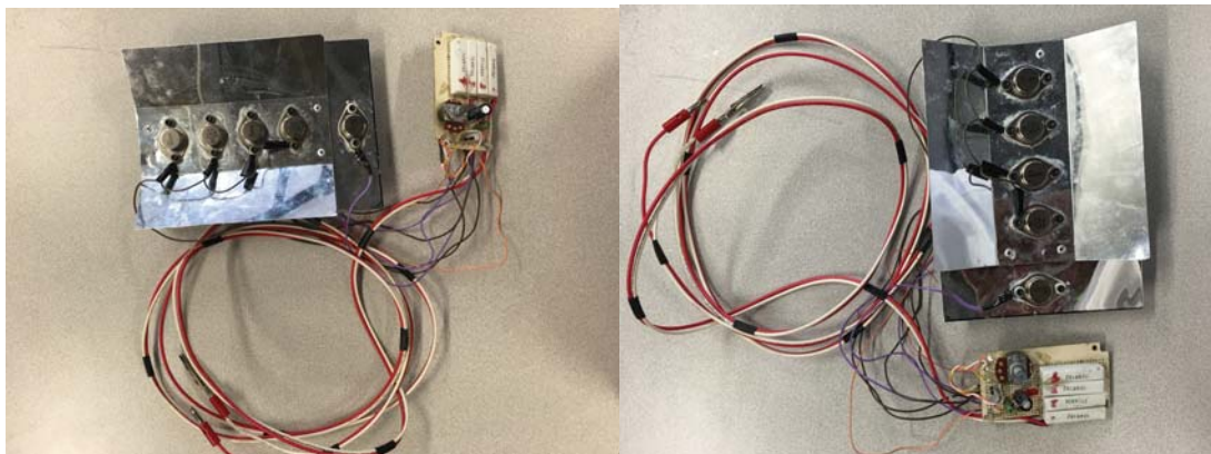
Fig. 39 Carga variable con disipador de calor
