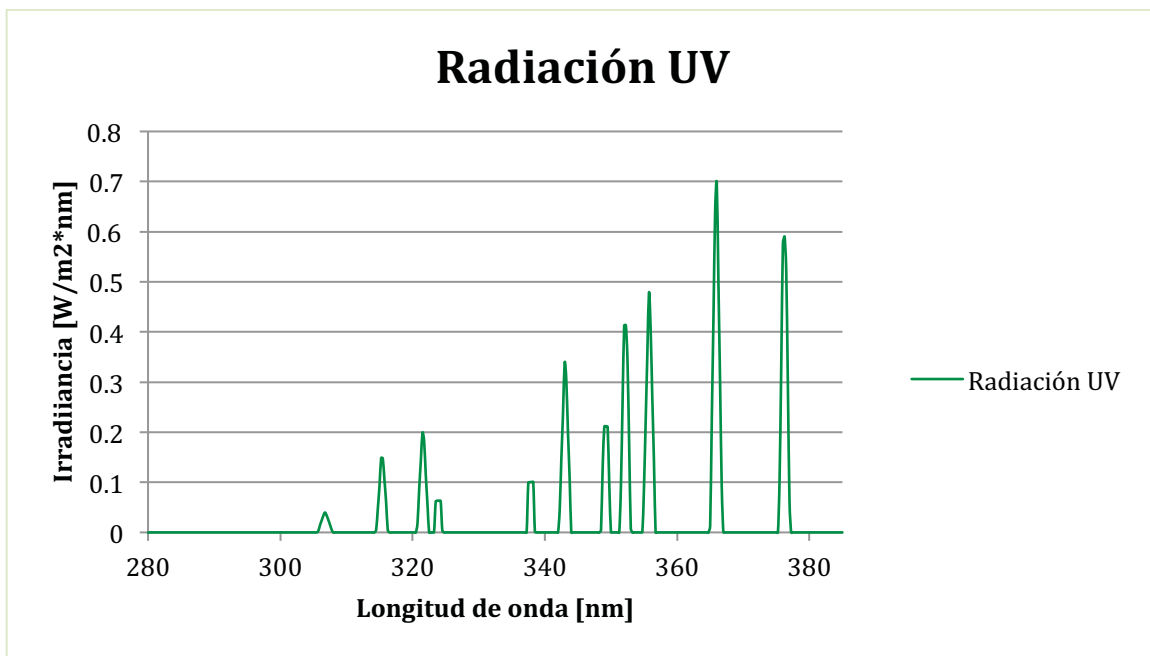
Gráfica 3 Espectro ultravioleta lámpara Ultravitalux
