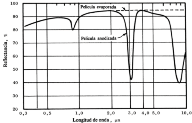
Fig. 30 Curva de reflectancia para aluminio comercial pulido con recubrimiento de aluminio anodizado ( Al_2O_3 ) 18
