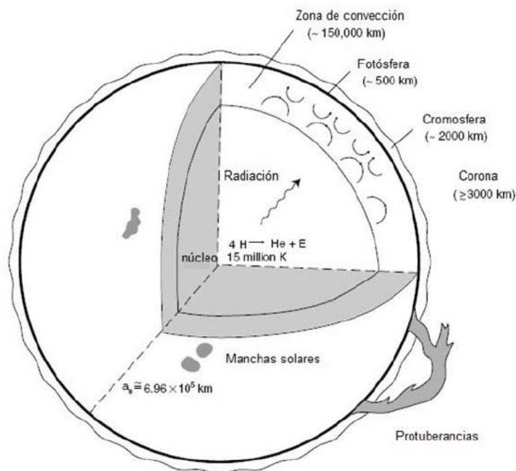
Fig. 3 Composición del Sol 5
