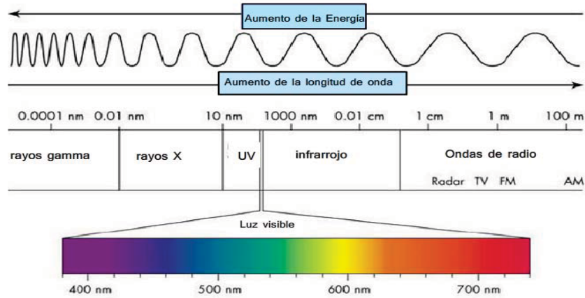
Fig. 4 Espectro electromagnético 6
