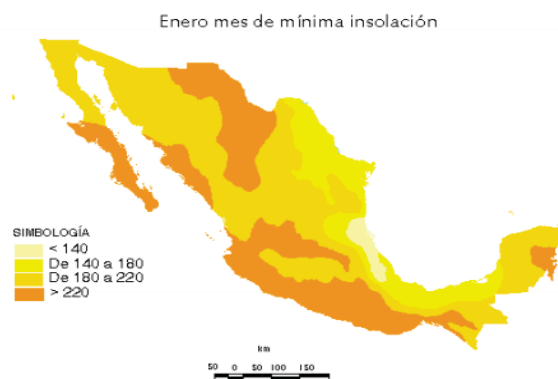
Fig. 13 Irradiancia solar mínima. En [ W/m^2 ] 3
