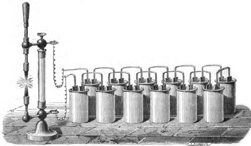
Fig. 23 Experimento de arco de carbono 16
