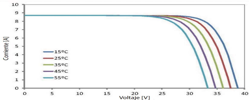
Fig. 36 Corriente-tensión para paneles fotovoltaicos policristalinos a diferentes temperaturas de operación
