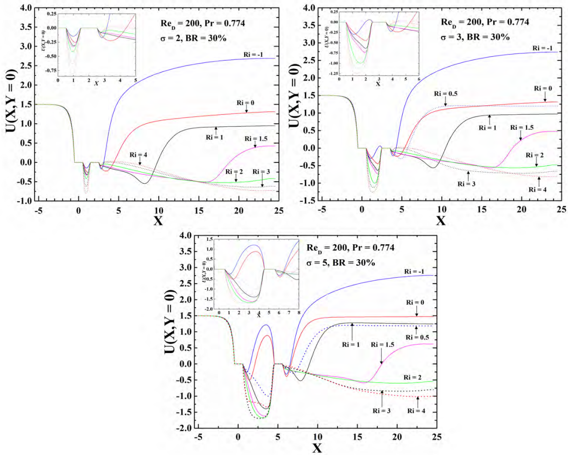
Figura 3.27: Perfiles adimensionales de velocidad axial a lo largo del plano de simetría como una función de la coordenada longitudinal para valores de \sigma = 2, 3 y 5 y para diferentes números de Richardson.
