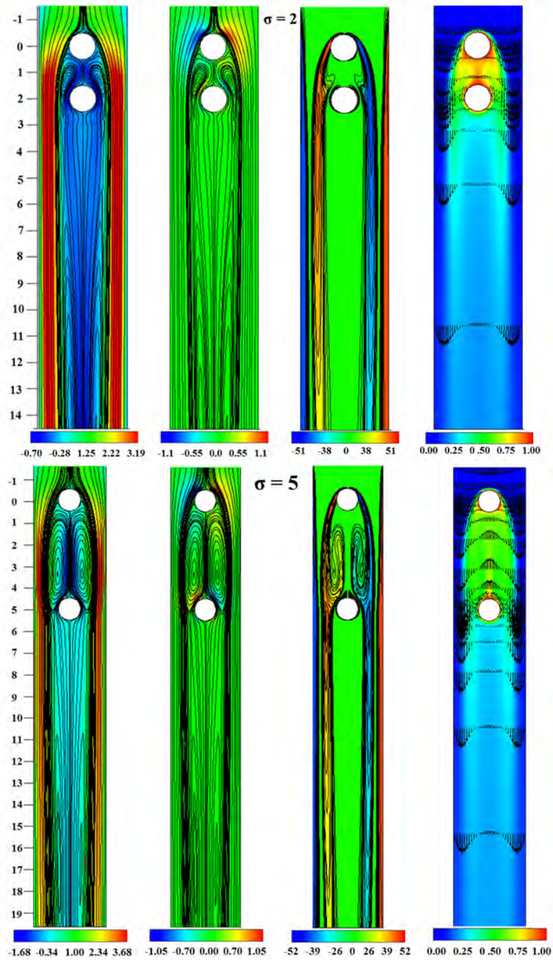
Figura 3.23: Valores del flujo promedio adimensional para Re_D = 200 , BR = 30\% y Ri = 2 ( Gr = 8 \times 10^4 ) para \sigma = 2 y 5 . De izquierda a derecha: componentes de velocidad U y V , vorticidad \Omega , y campos de temperatura \theta , respectivamente.
