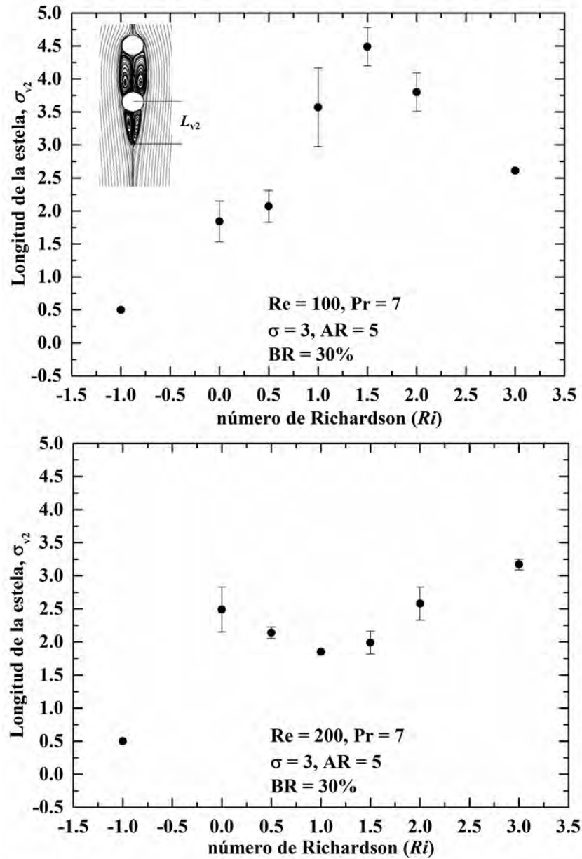
Figura 5.14: Valor promedio \pm DE de la longitud adimensional promedio de la estela del cilindro inferior \sigma_{v2}/D para Re = 100 y 200 como una función del número de Richardson. La longitud es medida desde el centro del cilindro inferior.
