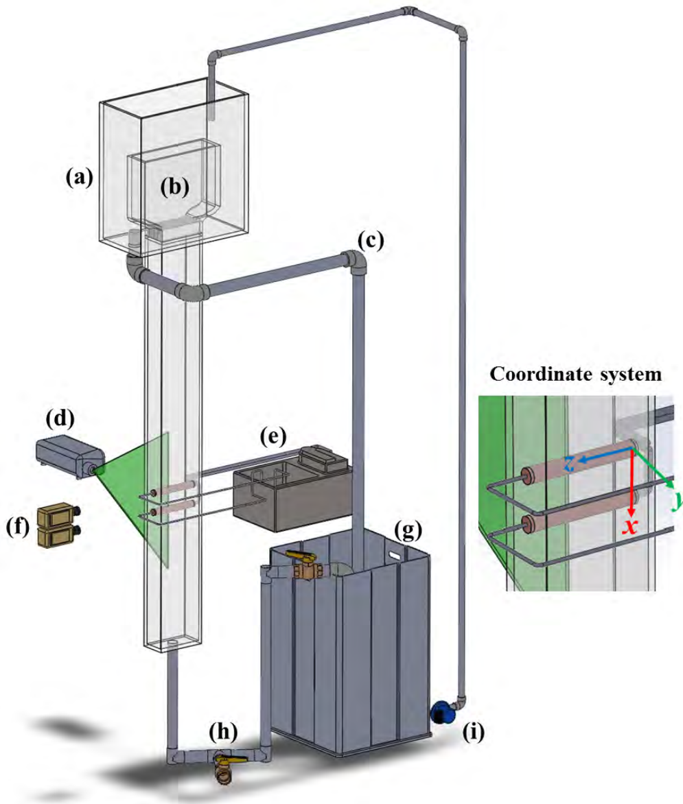
Figura 4.1: Diagrama esquemático del diseño experimental. (a) Depósito secundario. (b) Contracción a la entrada del canal con alineadores de flujo tipo panal de abeja. (c) Tubo de rebozadero. (d) Láser. (e) Baño térmico. (f) Cámaras digitales (CMOS). (g) Tanque de almacenamiento. (h) Válvula ajustable. (i) Bomba centrífuga.
