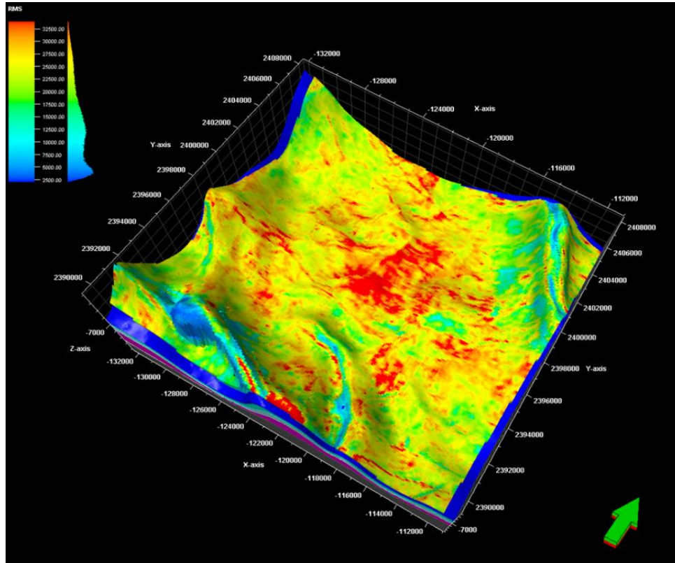
Figura IV.34 Distribución de las anomalías RMS para la zona estratigráfica del Cretácico (espesor bruto), en extracción volumétrica.
