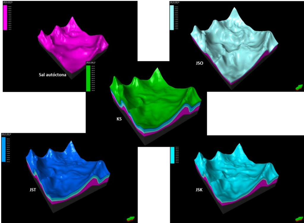
Figura IV.25 Zonas estratigráficas generadas entre dos horizontes estratigráficos o límites de secuencias
