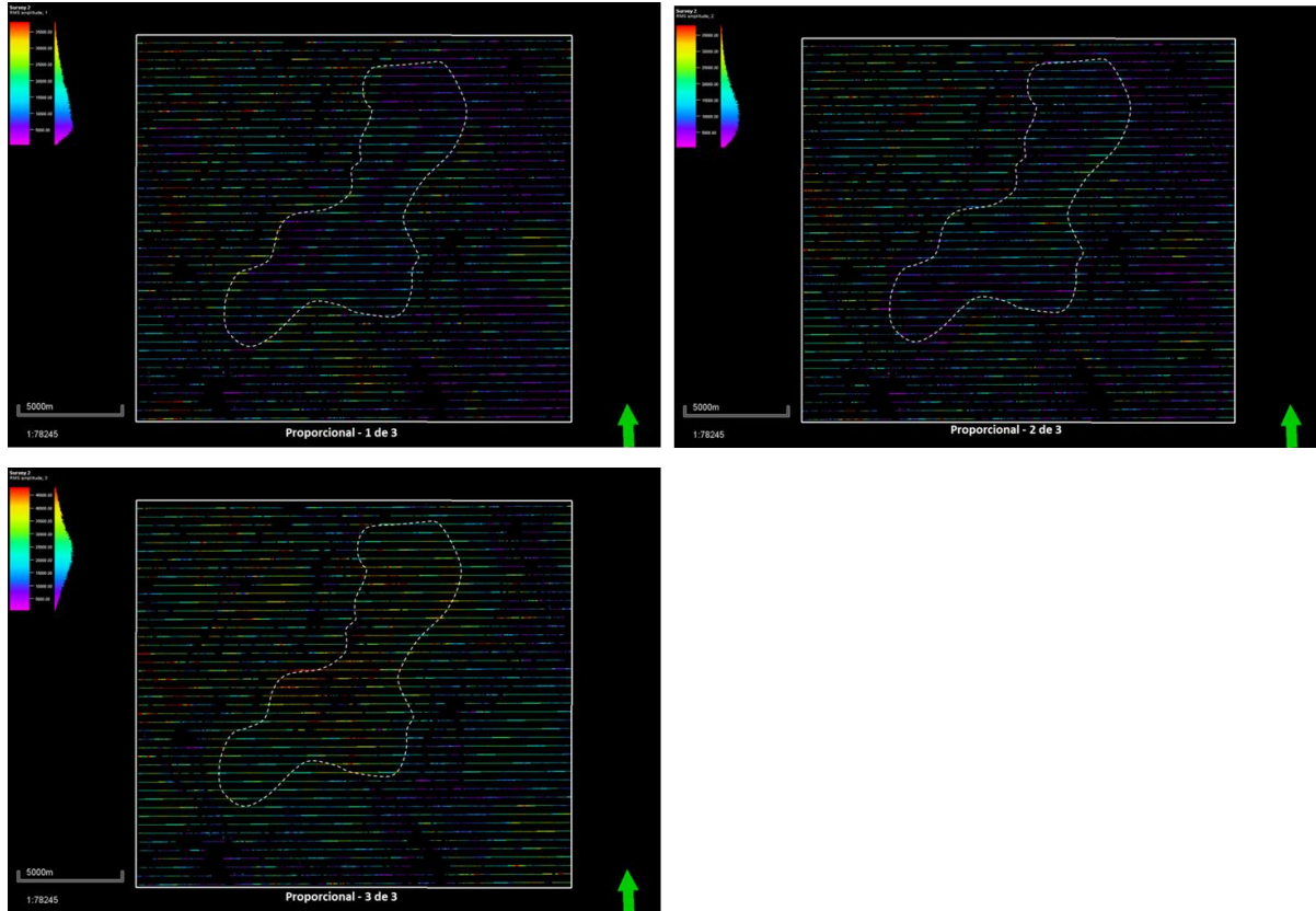
Figura IV.29 Distribución de las anomalías RMS para la zona estratigráfica del Cretácico, en una ventana de 150 ms y dividida en 3 proporcionales, la línea blanca discontinua delimita la mini cuenca principal.
