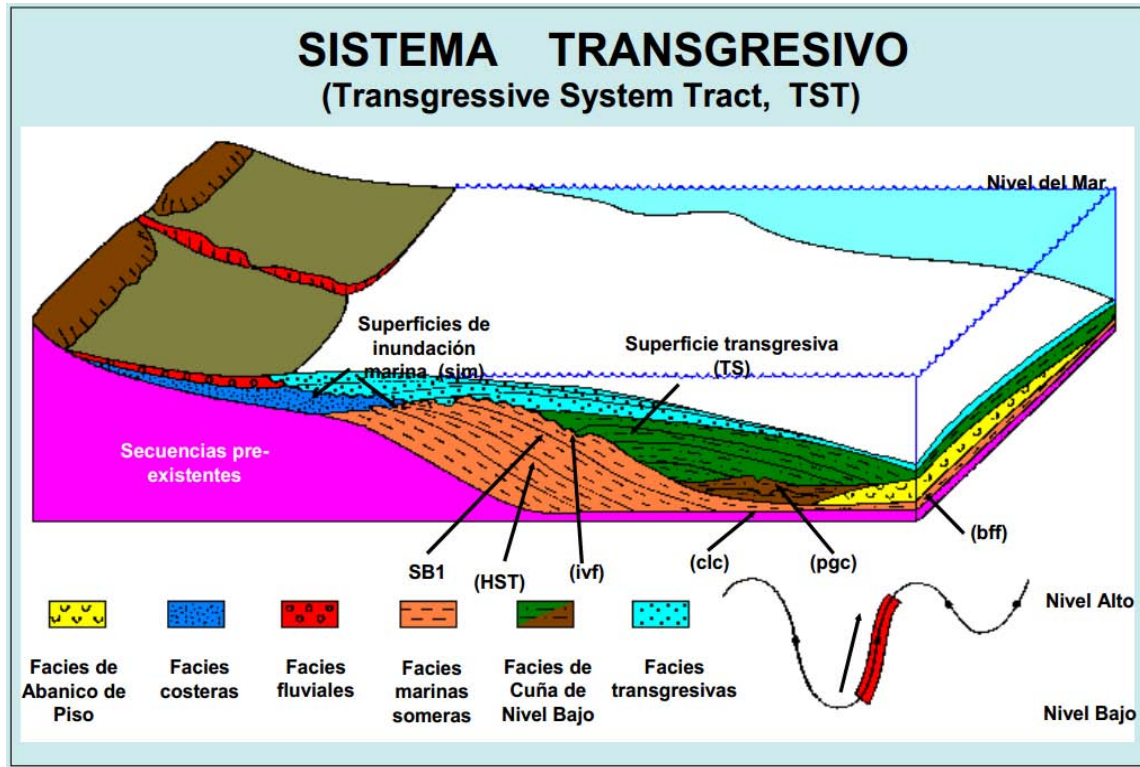
Figura III.5 Sistema Transgresivo ( Transgressive System Tract , TST), modificado de Posamentier y Vail, 1988.
