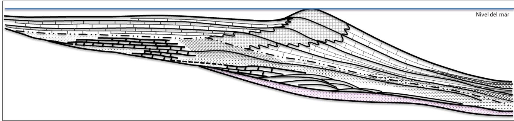
Figura V. 12 Modelo secuencial depositacional conceptual para las secuencias del: Oxfordiano (condiciones de lowstand, LST), Kimmeridgiano (lowstand, LST – transgresivo, TST), Tithoniano (transgresivo, TST) y Cretácico en general (secciones condensadas).
