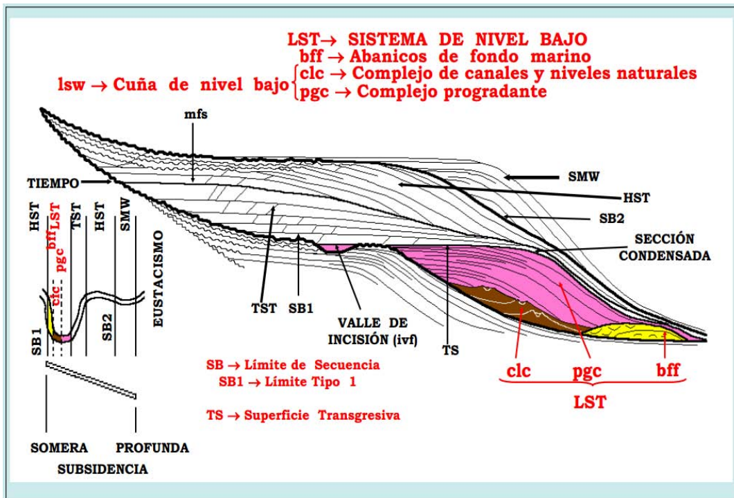
Figura III.3 Sistemas progradantes en cuña de nivel bajo de mar ( Lowstand System Tract, LST ), Modificado de Posamentier y Vail, 1988.
