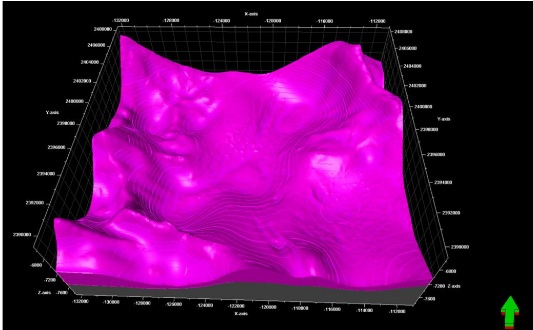
Configuración estructural para la cima de la sal autóctona
