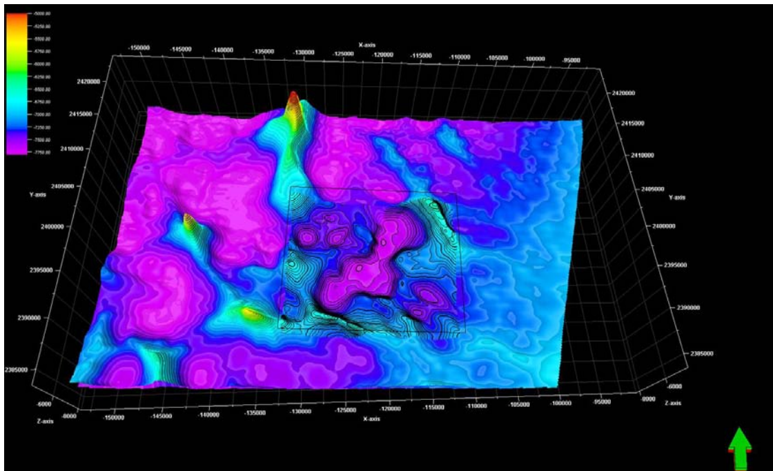
Figura IV.10 Configuración estructural para la posible cima del Oxfordiano mostrando un sector de minicuecas (recuadro negro), identificado hacia la porción central del área de estudio y es aquí donde la secuencia jurásica alcanza su mayor espesor.
