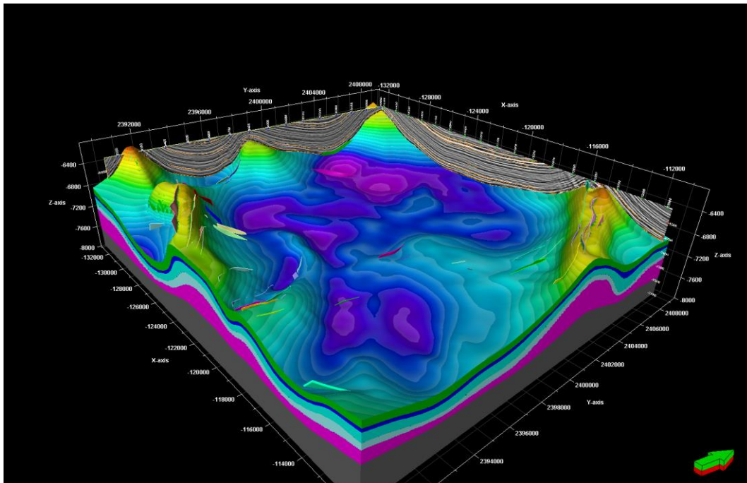
Figura IV.26 Integración de las zonas estratigráficas en el modelo estructural
