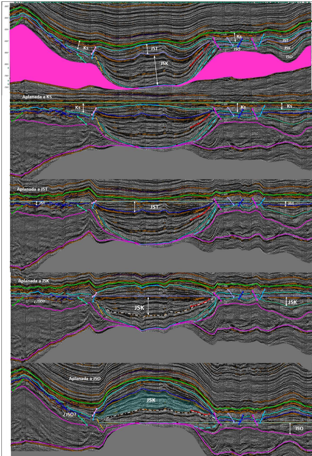
Figura IV.19 Minicuenca simétrica donde la sal se expulsó en su totalidad hasta generar una soldadura en el centro de la misma, la secuencia del Kimmeridgiano rellena la cuenca casi en su totalidad pero existe la posibilidad que esta contenga al miembro superior (carbonatado), del Oxfordiano (línea blanca discontinua), solo que no se aprecia contrastante de imagen entre ambas secuencias por ser de la misma constitución litológica.
