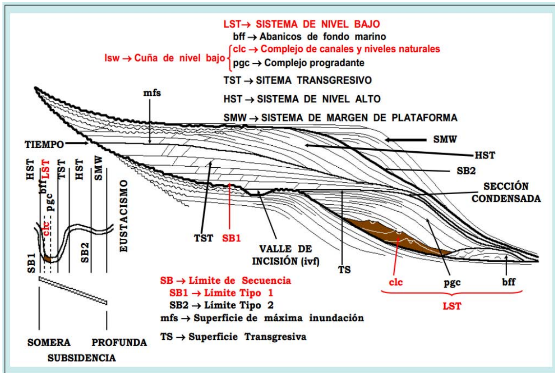
Figura III.4 Complejo de sistemas de borde o margen de plataforma de nivel bajo del mar (Lowstand System Tract, LST), Modificado de Posamentier y Vail, 1988.
