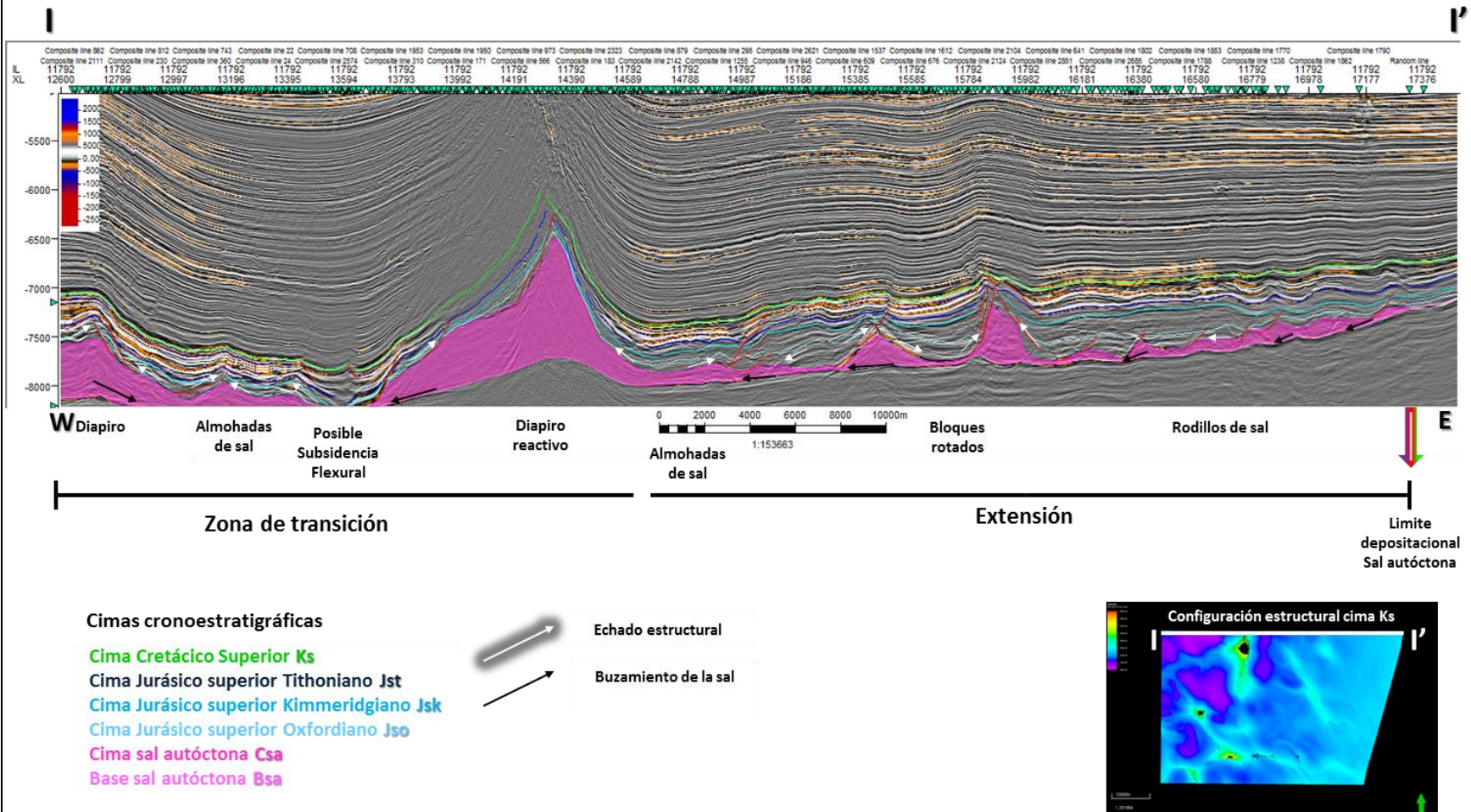
Figura V.1 Línea sísmica I-I' que muestra los estilos estructurales asociados a la tectónica salina, así como las componentes extensional y transicional de un sistema gravitacional en una cuenca salina.
