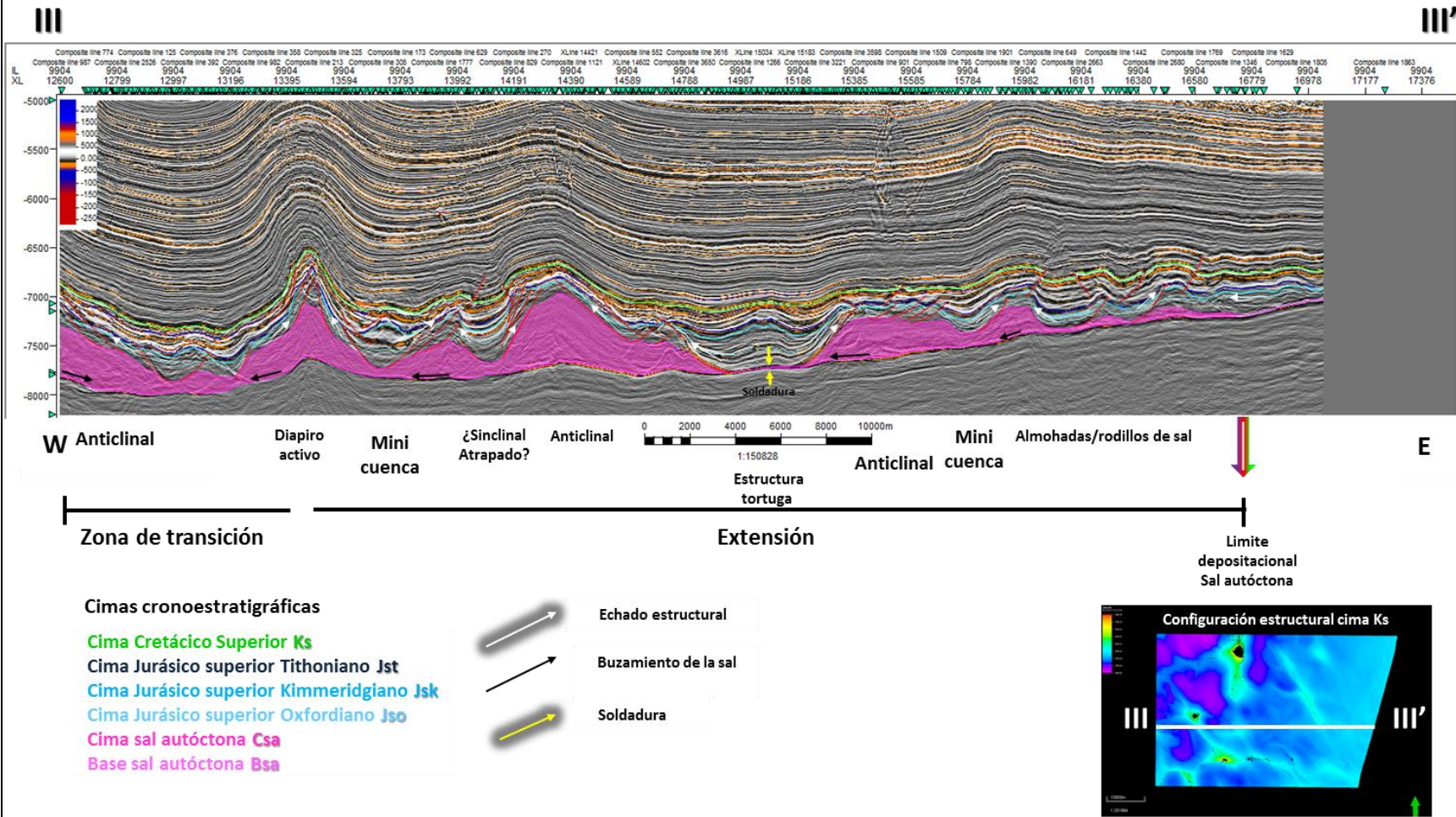
Figura V.3 Línea sísmica III-III' que muestra los estilos estructurales asociados a la tectónica salina así como las componentes extensional y transicional de un sistema gravitacional en una cuenca salina.
