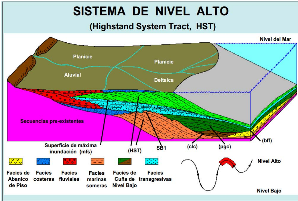
Figura III.6 Sistema de Nivel Alto del mar (“Highstand System Tract”), modificado de Posamentier y Vail, 1988.
