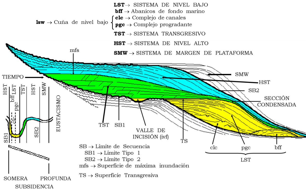
Figura III.1 Arquitectura de la estratigrafía de secuencias (Modificada de Peter Vail 1977).
