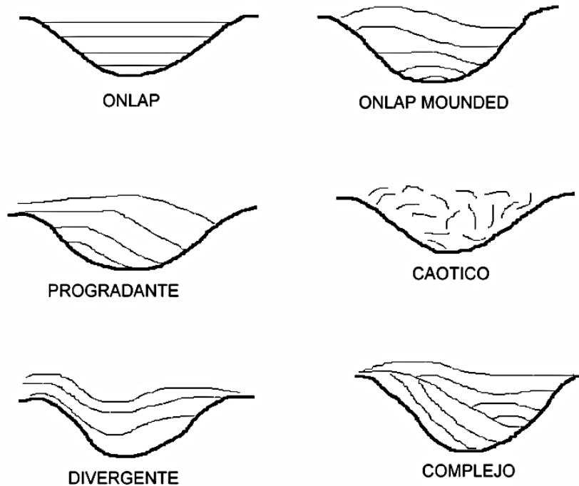
Figura III.8 Tipos de configuraciones internas
