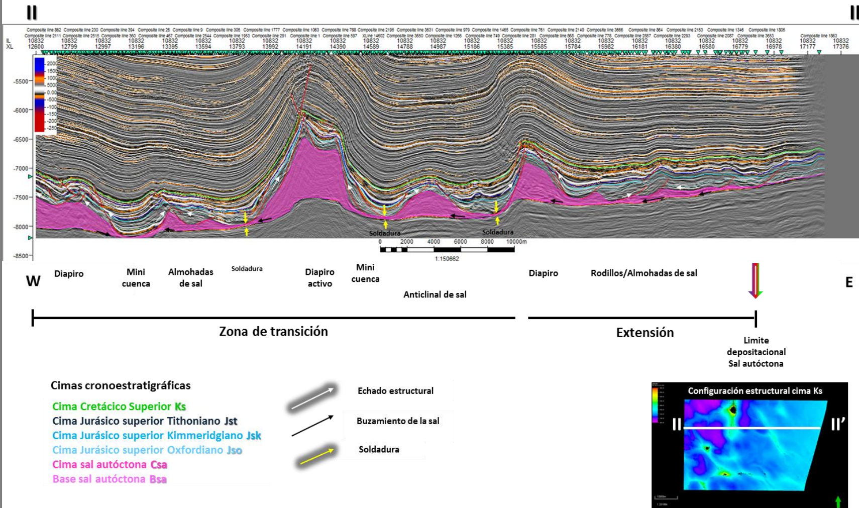
Figura V.2 Línea sísmica II-II' que muestra los estilos estructurales asociados a la tectónica salina así como las componentes extensional y transicional de un sistema gravitacional en una cuenca salina.
