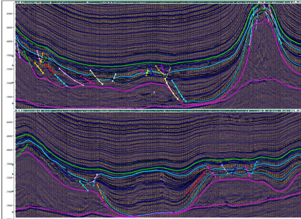
Figura IV.30 Control de calidad para la extracción de anomalías RMS para el horizonte correspondiente a la cima del JSK, en general muestra una buena correlación con la zona estratigráfica (línea negra continua sobrepuesta al horizonte Jsk).
