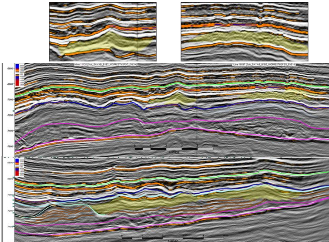
Figura IV.7 Línea compuesta que muestra rasgos sedimentarios interpretados a partir del análisis de facies sísmicas, en detalle (parte superior resaltadas en color amarillo), la imagen de en medio muestra la disposición de los rasgos al interior de la secuencia del Cretácico y la imagen inferior muestra los rasgos identificados para la secuencia Jurásica.
