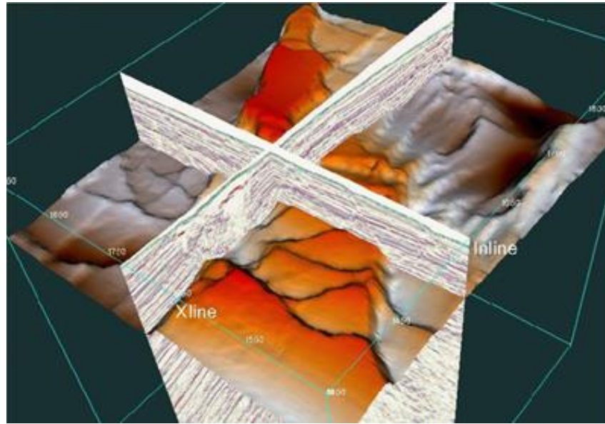
Figura III.12 Interpretación de terrazas estructurales a partir de sísmica 3D, apoyada en la geomorfología sísmica. Using 3D Seismic Data: Implications for Exploration and Development, Geological Society London, Memoirs, 29:11-24, doi:10.1144/GSL.MEM.2004.029.01.02
