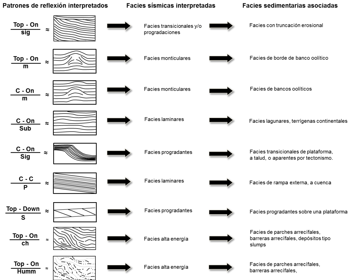
Figura III.11 Asociación de los patrones de reflexión con las facies sísmicas y estas a su vez con sus correspondientes facies sedimentarias.
