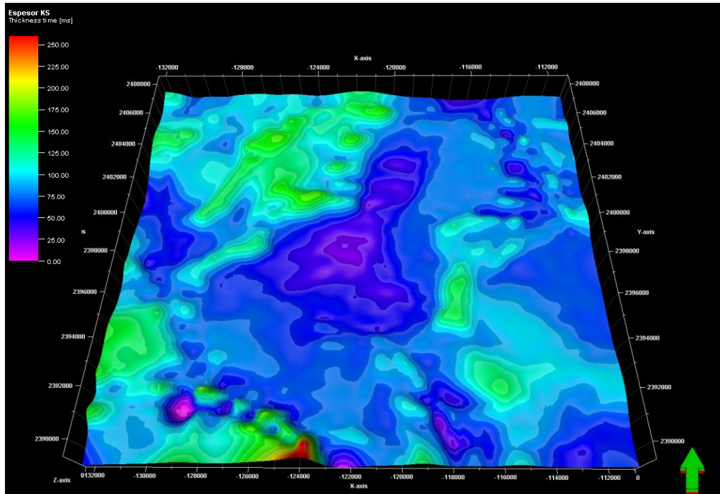
Figura IV.24 Distribución de isocoras para la secuencia Cretácica
