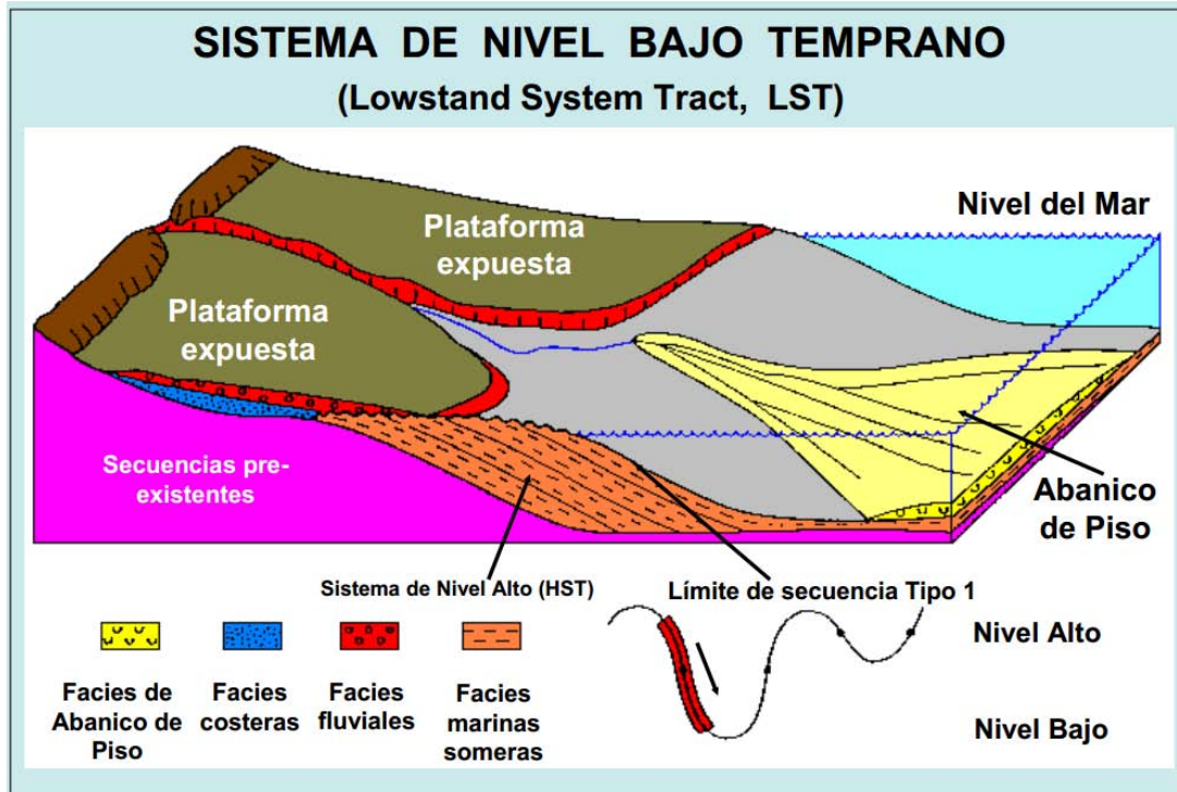
Figura III.2 Sistema de nivel bajo del mar temprano ( Lowstand System Tract, LST ), modificado de Posamentier y Vail, 1988.
