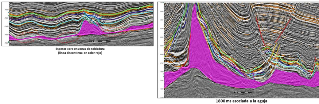
Figura IV.11 Configuración estructural para la cima de la sal autóctona y dos sectores que muestran los espesores máximos y mínimos identificados.
