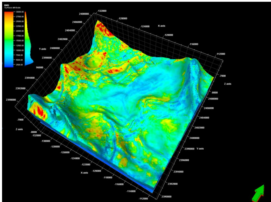
Figura IV.33 Distribución de las anomalías RMS para la zona estratigráfica del Kimmeridgiano (espesor bruto), en extracción volumétrica.
