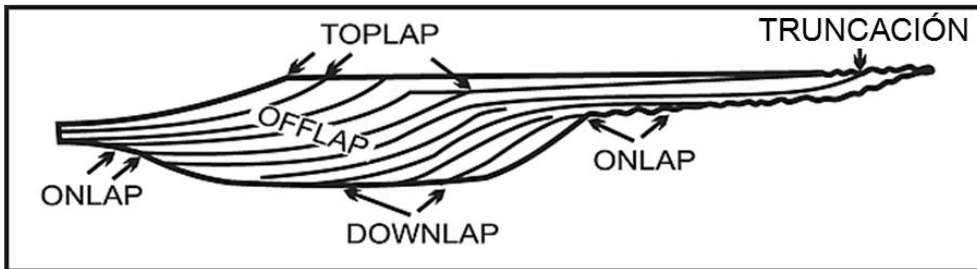
Figura III.7 Terminaciones para el reconocimiento de límites de secuencias.
