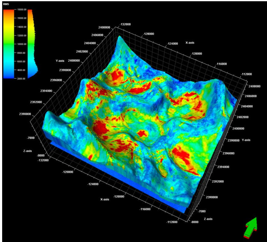
Figura IV.32 Distribución de las anomalías RMS para la zona estratigráfica del Oxfordiano (espesor bruto), en extracción volumétrica.
