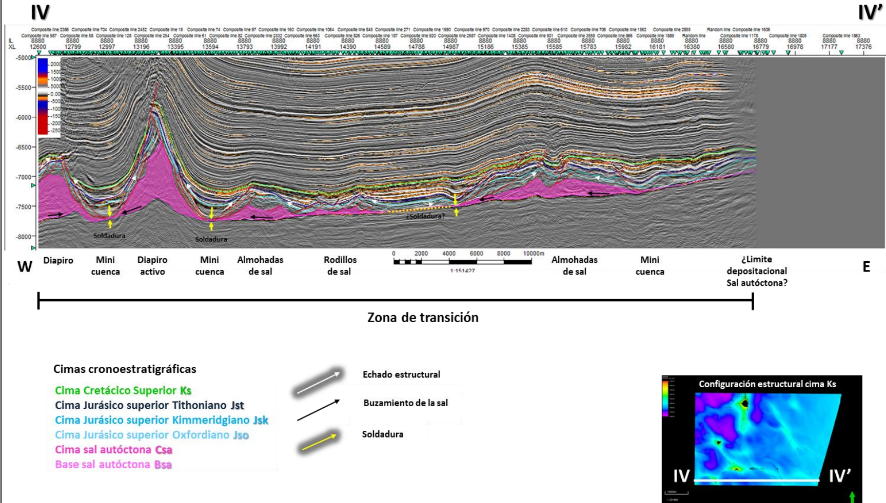
Figura V.4 Línea sísmica IV-IV' que muestra los estilos estructurales asociados a la componente transicional de un sistema gravitacional en una cuenca salina.
