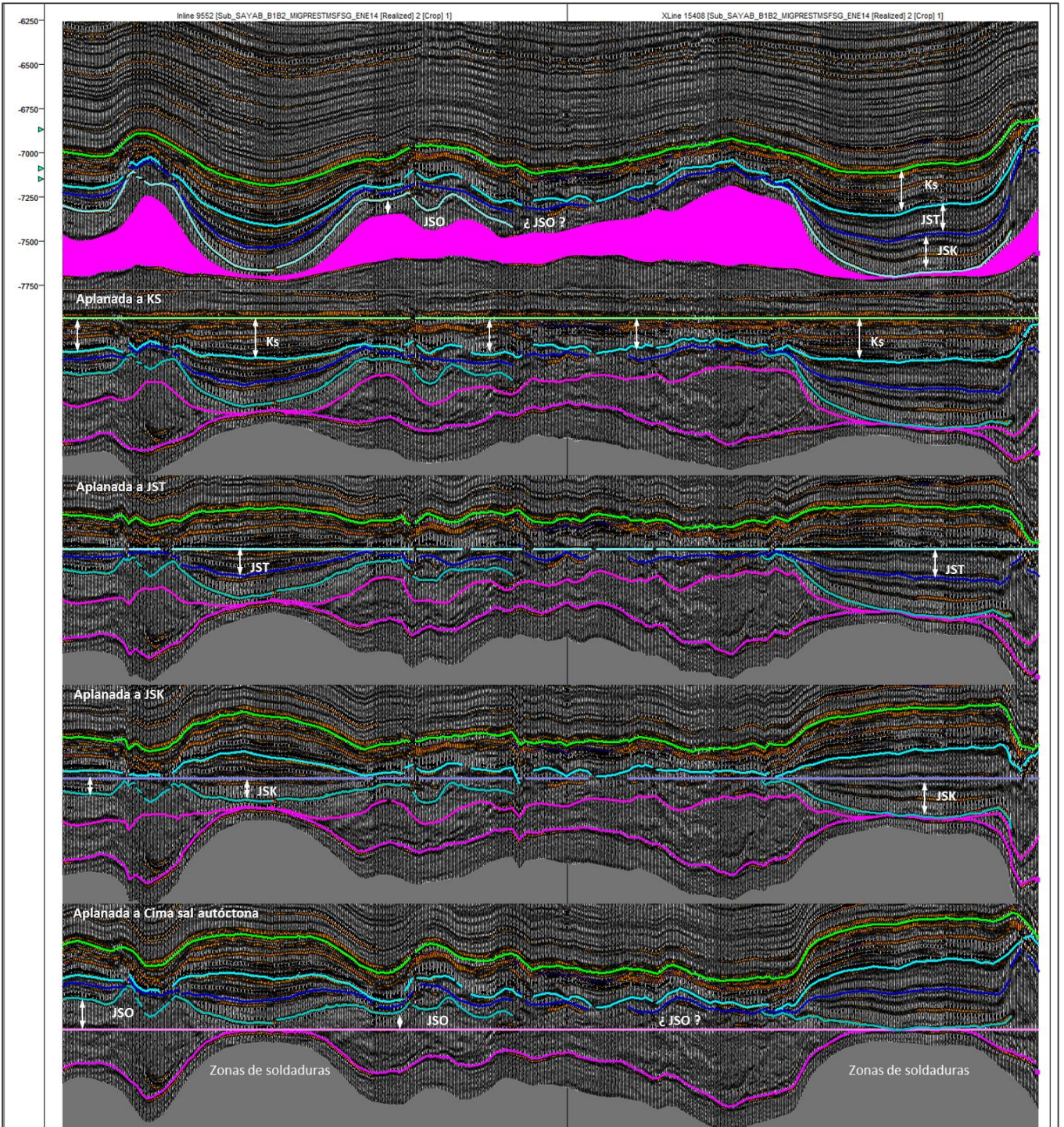
Figura IV.18 Línea sísmica (este - oeste) interpretada, en ella se aprecia la migración de las minicuevas en dirección este-oeste, debido al desarrollo limitado y simétrico de las mismas en el extremo occidental, mientras que en el sector oriental una minicueva asimétrica es aparentemente rellena por la secuencia del Kimmeridgiano, denotando que su desarrollo no fue sincrónico. El aplanado cronológico a cada uno de los límites de las secuencias permite observar su variación en espesor y/o desarrollo.
