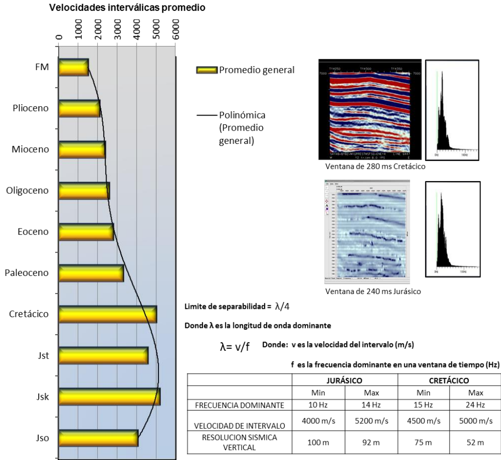
Figura IV.6 Grafica que muestra los rangos de la resolución sísmica estimada a partir de las velocidades de intervalo promedio y la longitud de onda (esta última en función de la frecuencia dominante) para el Cretácico y Jurásico no diferenciado.
