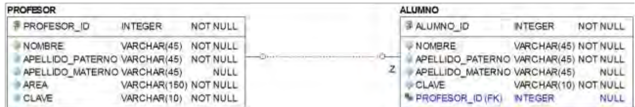
Img 13. Ejemplo relación uno a uno identificativa y no identificativa en el modelo relacional
