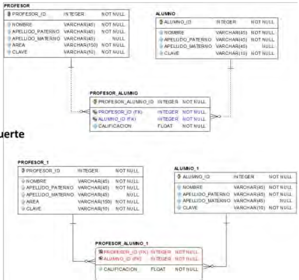
Img 15. Ejemplo relación muchos a muchos identificativa y no identificativa en el modelo relacional
