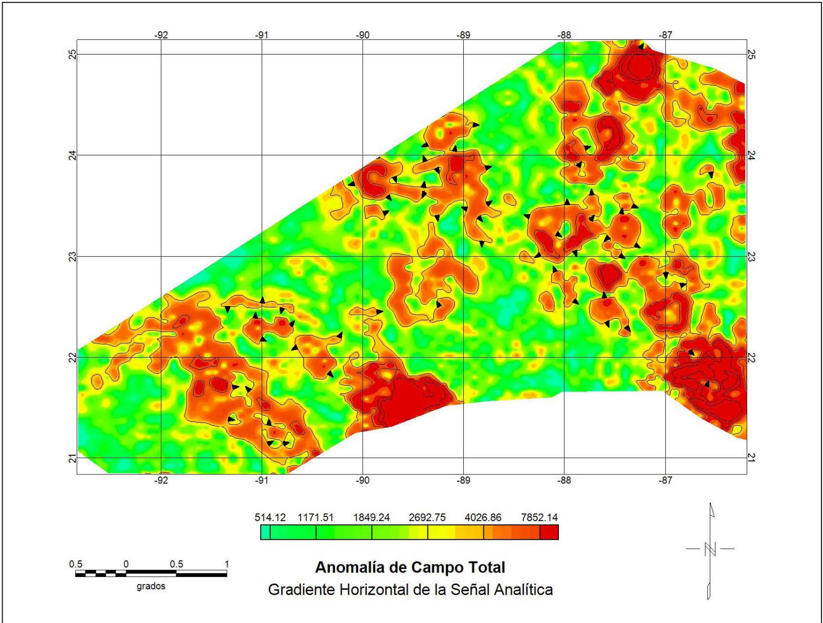
Figura 4. 19 Mapa de gradiente horizontal de la señal analítica.
