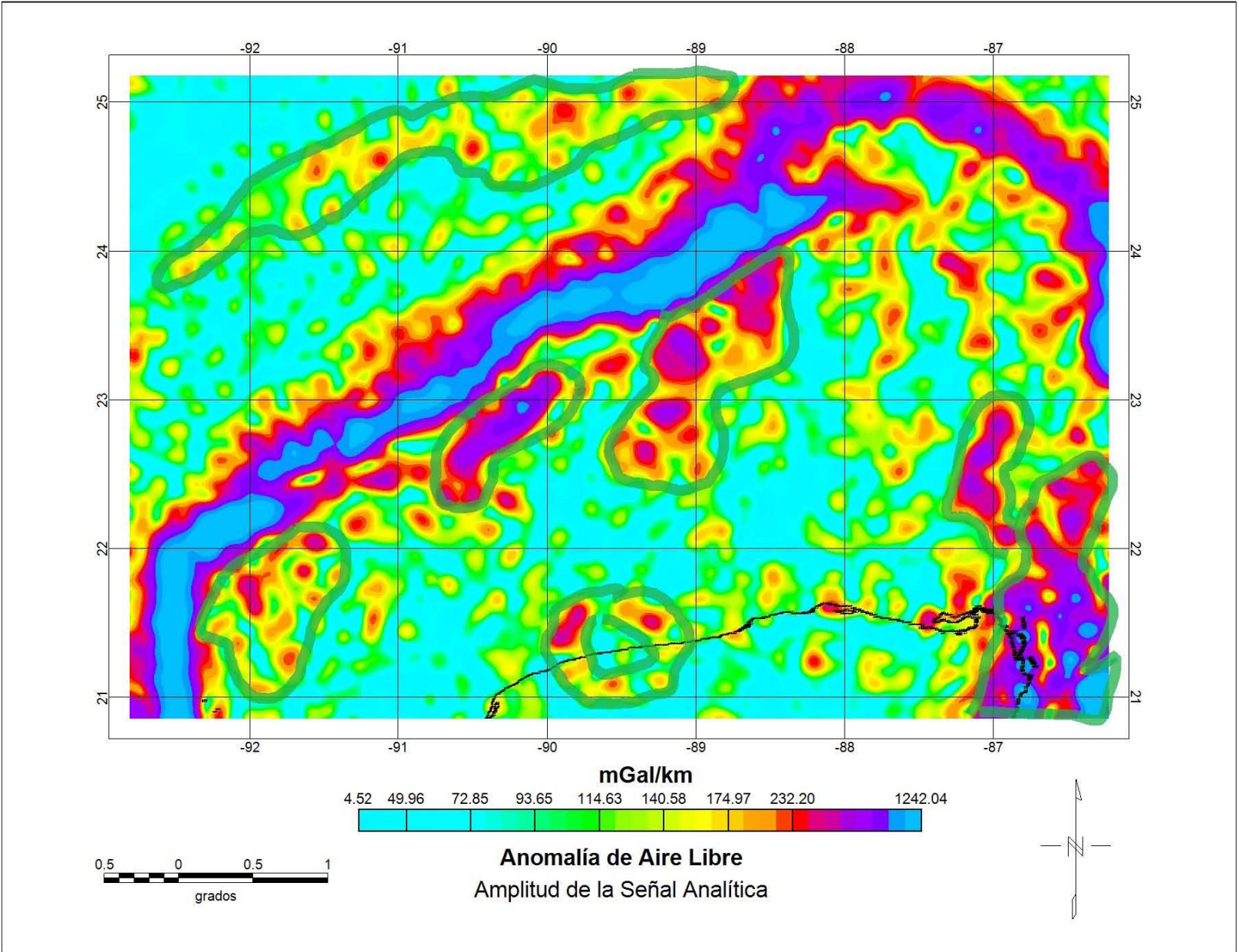
Figura 4. 8 Mapa de amplitud de la señal analítica. Con color verde se encuentran delimitados, los patrones mejor definidos.
