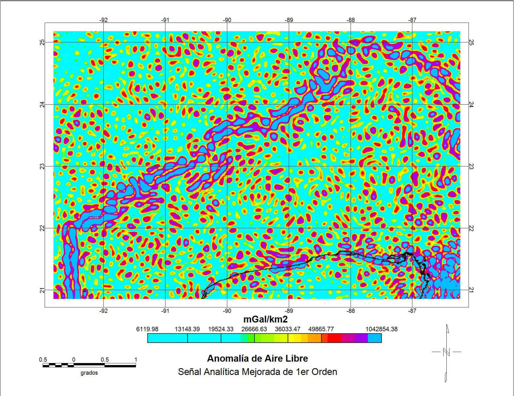
Figura 4. 11 Mapa de la señal analítica mejorada de 1er orden.
