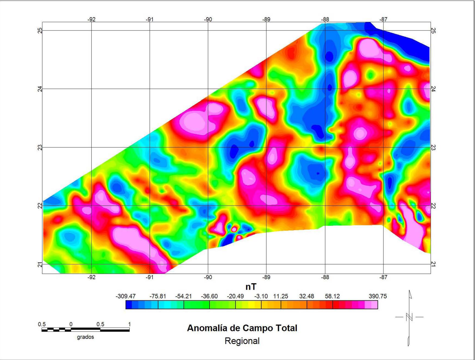
Figura 4. 13 Mapa de la anomalia de campo total.
