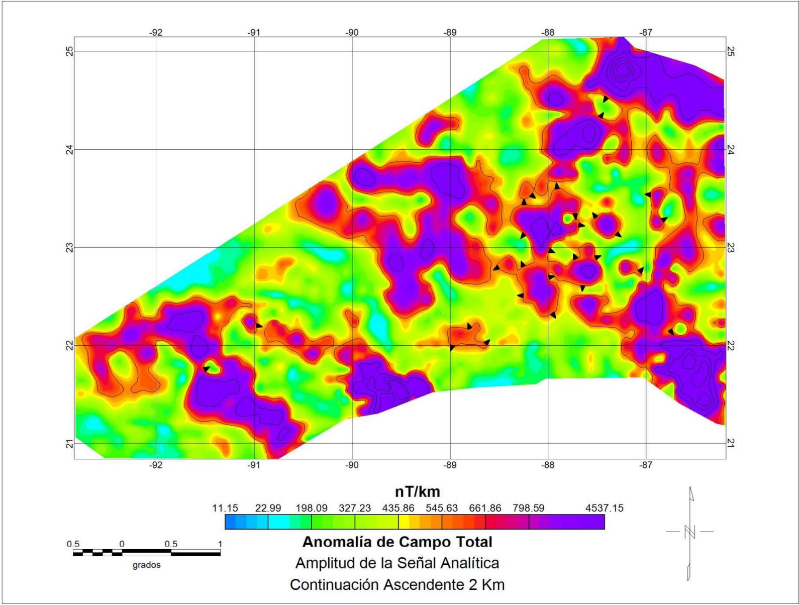
Figura 4. 16 Mapa de amplitud de la señal analítica con continuación ascendente a 2 km.
