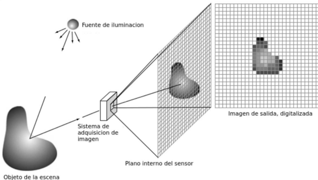
Figura 2.19: Diagrama de una matriz de sensores CCD y su recepción de datos
