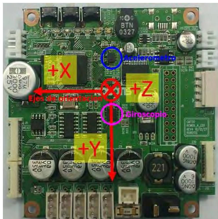
Figura 3.6: Sensores acelerómetro y giroscopio
