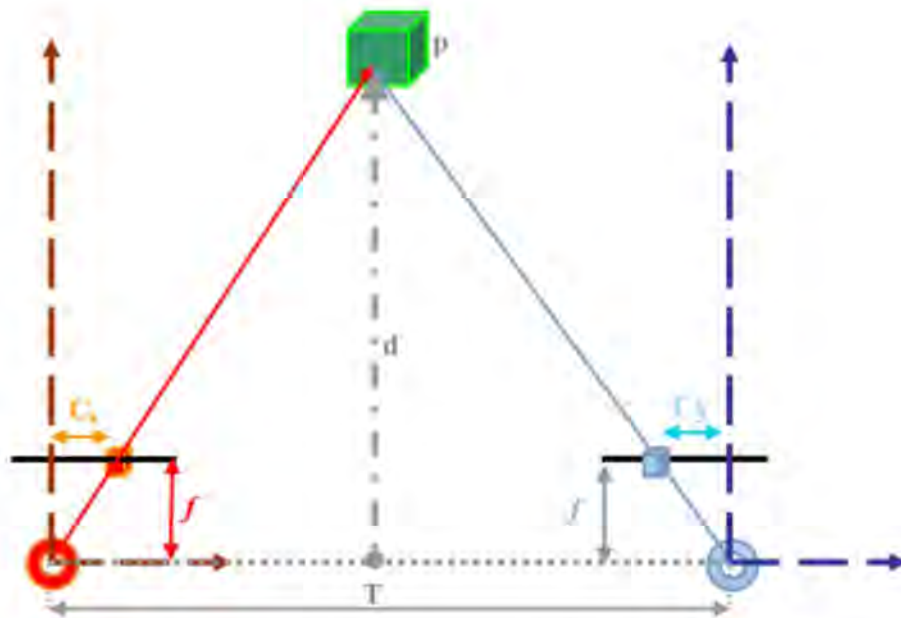
Figura 4.4: Diagrama de distancias en el sistema estereoscópico
