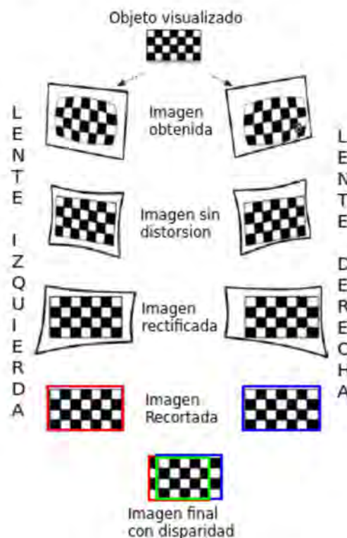
Figura 4.3: Rectificación de las 2 imágenes entregadas por la cámara estereoscópica
