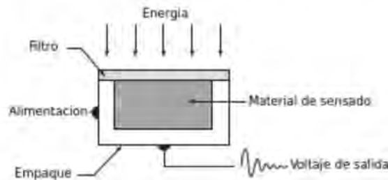
Figura 2.18: Modelo básico ejemplificando un sensor CCD
