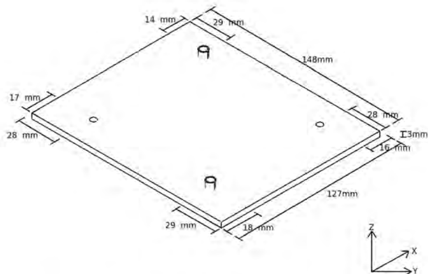
Figura H.1: CAD de la base para la mini-PC, vista axonométrica
