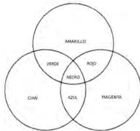
Figura 2.12: Espacio de color sustractivo (YCM).
