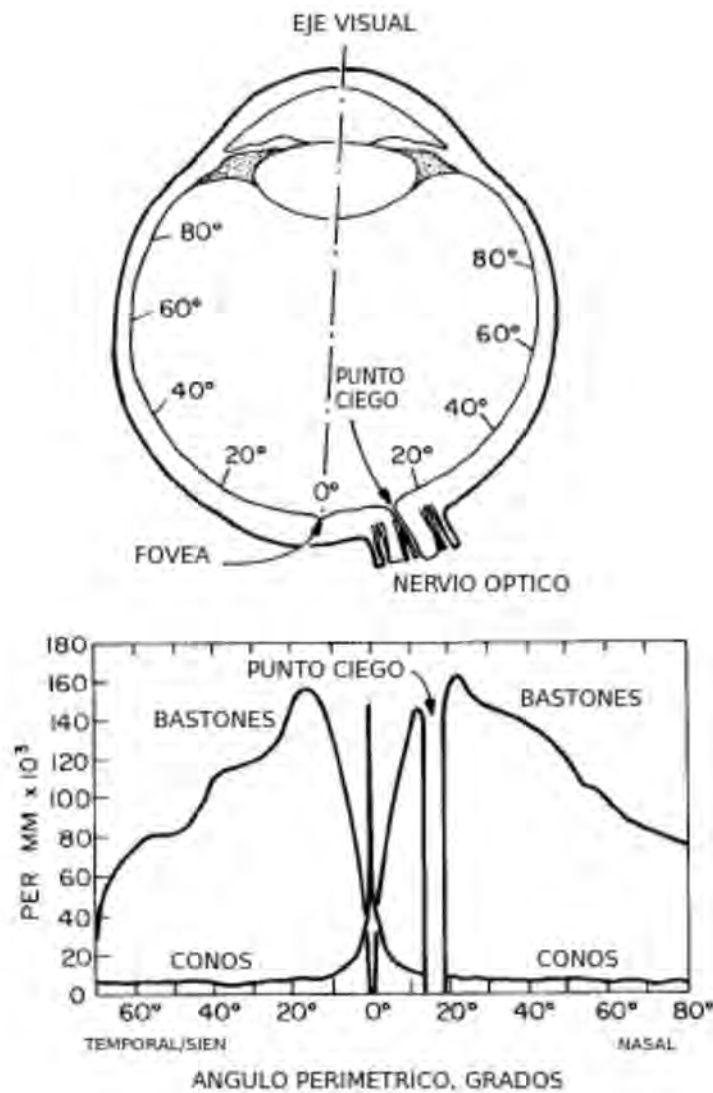
Figura 2.15: Distribución del ángulo de visión humana
