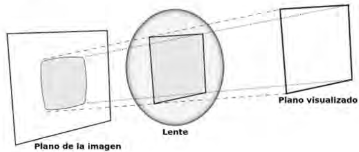
Figura 4.1: Distorsión radial
