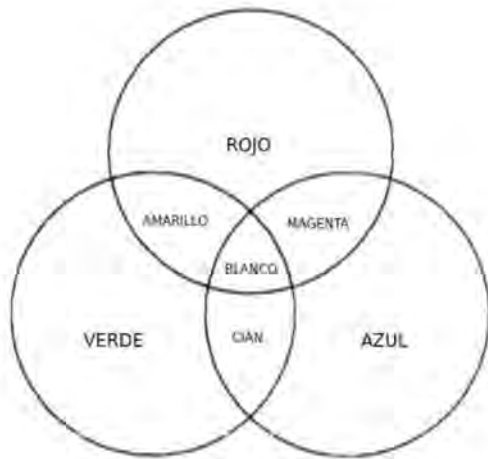
Figura 2.11: Espacio de color aditivo (RGB).
