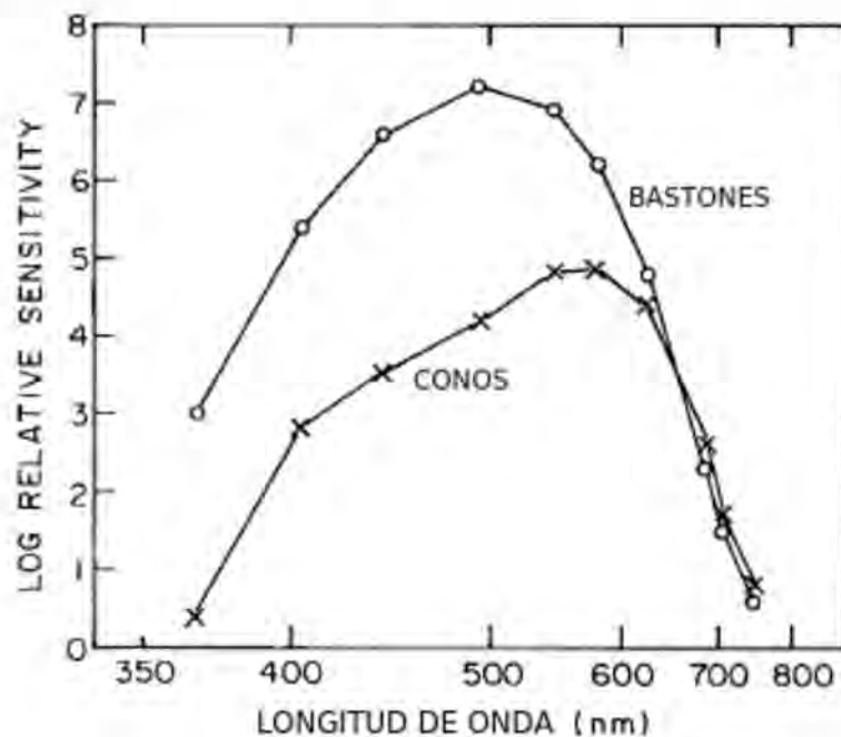
Figura 2.14: Rango de luz absorbida por los conos y bastones
