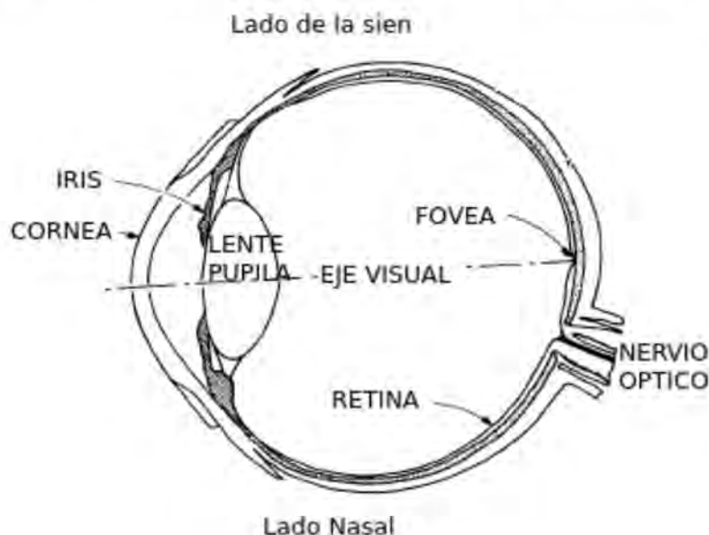
Figura 2.13: Diagrama transversal del ojo
