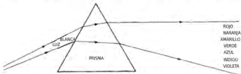
Figura 2.9: Descomposición de la luz en colores
