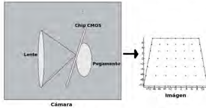
Figura 4.2: Distorsión tangencial
