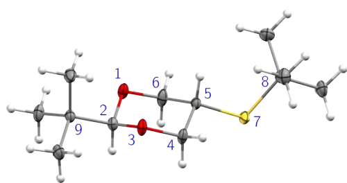
FIGURA 6.1.1: Análisis de rayos X del trans -2- tert -butil-5-( tert -butilsulfenil)-1,3-dioxano ( Trans-3 ). Figura: Diagrama ORTEP de Trans-3 (Elipsoides térmicos a un nivel de probabilidad del 50%, T = 103 \text{ K} ). Tabla: Datos correspondientes a los parámetros internos de la estructura.
