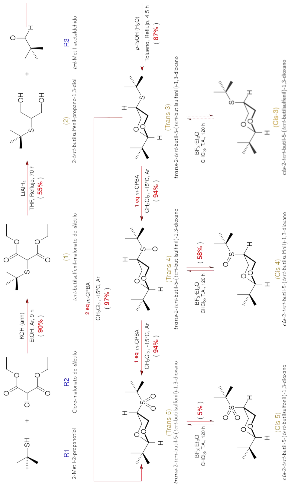
ESQUEMA 4.1.1: Ruta de síntesis de los compuestos de interés.
