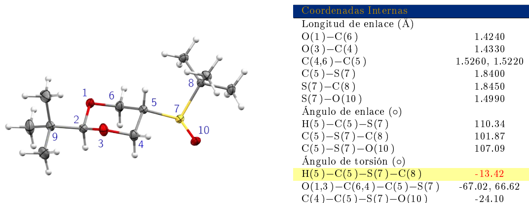
FIGURA 6.1.6: Análisis de rayos X del trans -2- tert -butil-5-( tert -butilsulfinil)-1,3-dioxano ( Trans -4). Figura: Diagrama ORTEP de Trans -4 (Elipsoides térmicos a un nivel de probabilidad del 50 %, T = 150 K). Tabla: Datos correspondientes a los parámetros internos de la estructura.
