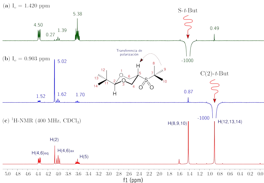
FIGURA 6.1.13: Espectros NOESY-1D del compuesto trans -2- tert -butil-5-( tert -butilsulfonyl)-1,3-dioxano. En el espectrómetro de 400 MHz en \text{CDCl}_3 a temperatura ambiente.
