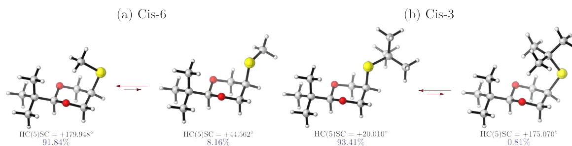
FIGURA 6.1.4: Equilibrio conformacional del diastereoisómero axial del sulfuro del 1,3-dioxano. Estructuras derivadas del estudio conformacional al nivel de teoría M06-2X/6-311++G(2d,2p).
