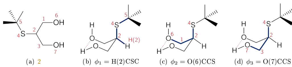
FIGURA 5.0.2: Ángulos de torsión en el 2-tert-butilsulfenil-propano-1,3-diol (2). (a) Numeración empleada en 2; (b–d) Segmentos de la molécula que definen los ángulos de torsión.
