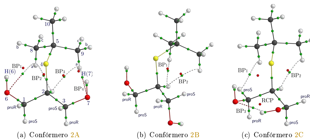
FIGURA 5.3.9: Gráficos moleculares de los conformeros del 2-tert-butilsulfenil-propano-1,3-diol.
