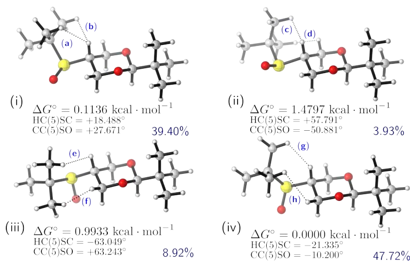
FIGURA 6.1.7: Conforméros del trans -2- tert -butil-5-( tert -butilsulfinil)-1,3-dioxano. Estructuras optimizadas al nivel de teoría empleado: M06-2X/6-311++G(2d,2p). Distancia entre hidrógenos: (a) 2.09490 Å; (b) 2.27495 Å; (c) 2.28482 Å; (d) 2.03027 Å; (e) 2.33425 Å; (f) 2.01705 Å; (g) 2.10934 Å y (h) 2.23976 Å.
