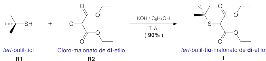
ESQUEMA B.3.1: Reacción de sustitución nucleofílica.
