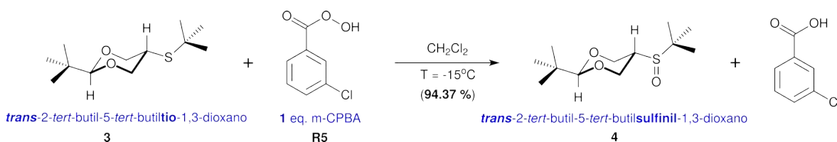
ESQUEMA B.3.6: Oxidación parcial del sulfuro de alquilo.
