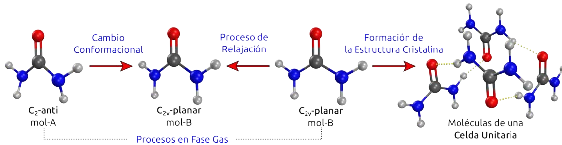
FIGURA 3.5.1: Formación de la estructura cristalina para la urea.
