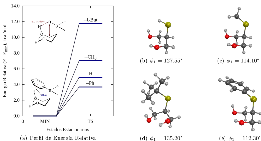
FIGURA 5.1.4: Estructuras de transición del 1,3-propanodiol-2-sustituido. (a) Perfil de energía relativa asociado a la rotación del ángulo de torsión \phi_1 ; (b–e) Estructura de transición del estado denotado como EC 1 en la proyección de Newman de la Figura 5.1.2 .
