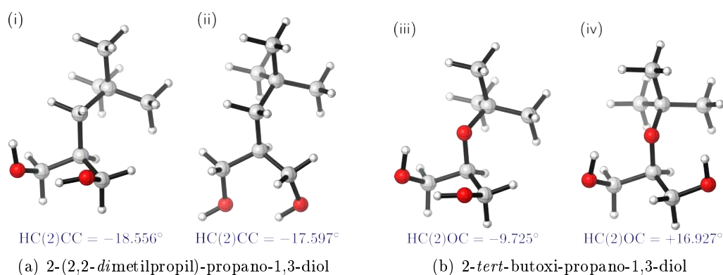
FIGURA 5.1.5: Conformeros eclipsados del 1,3-propanodiol-2-sustituido. Estructuras optimizadas al nivel de teoría M06-2X/6-311++G(2d,2p).
