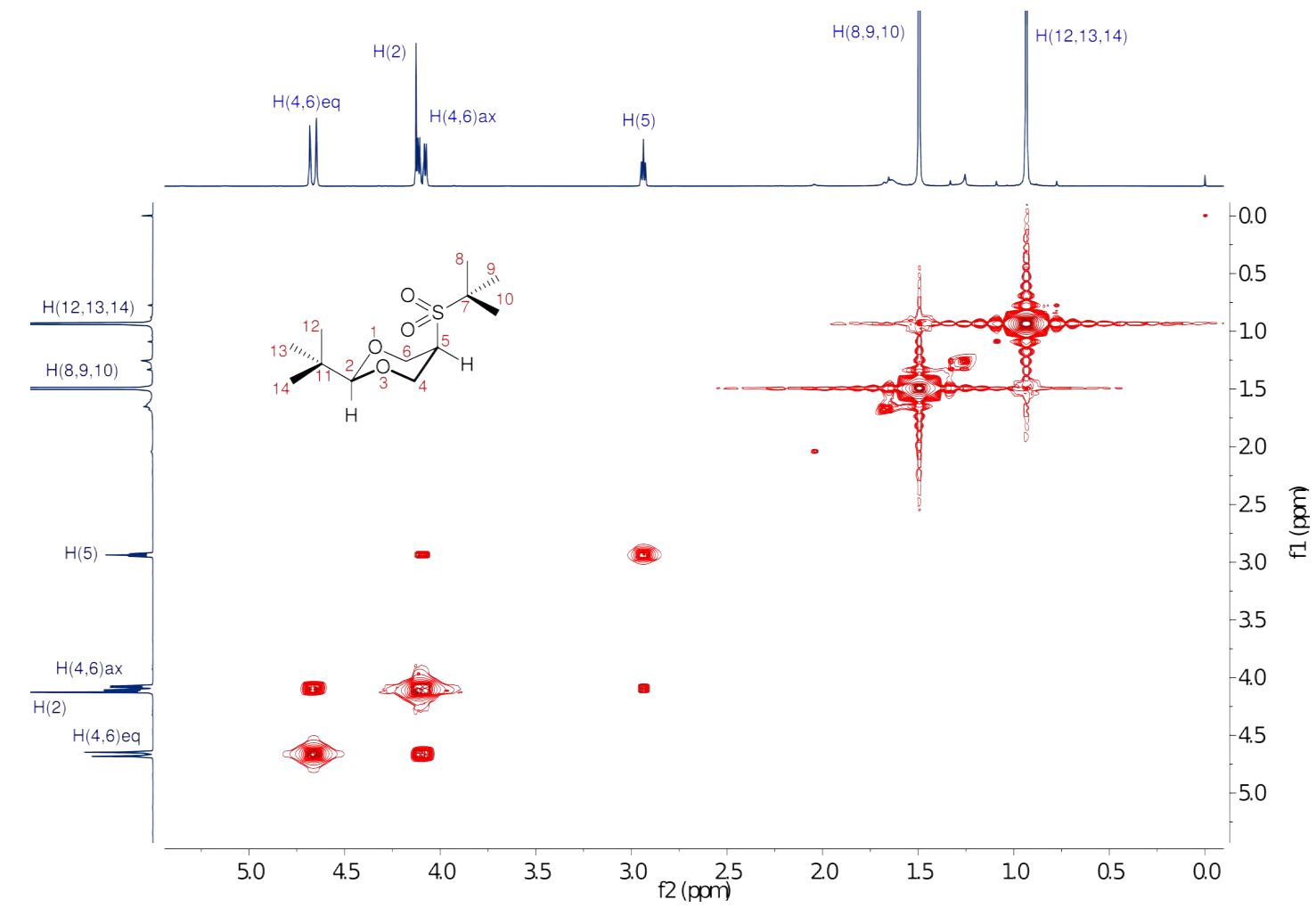
FIGURA B.3.16: Espectro COSY-400MHz del cis -2- tert -butil-5-( tert -butilsulfoni)-1,3-dioxano.
