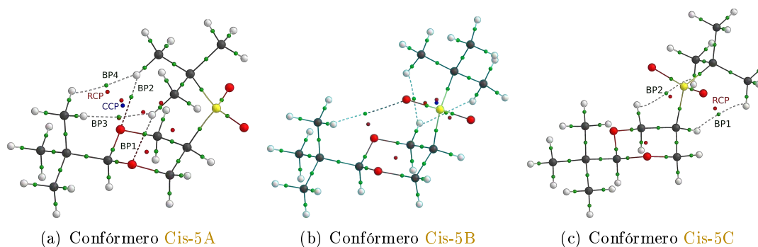
FIGURA 6.2.1: Gráficos moleculares para los conforméros del cis-2-tert-butil-5-(tert-butilsulfonyl)-1,3-dioxano.
