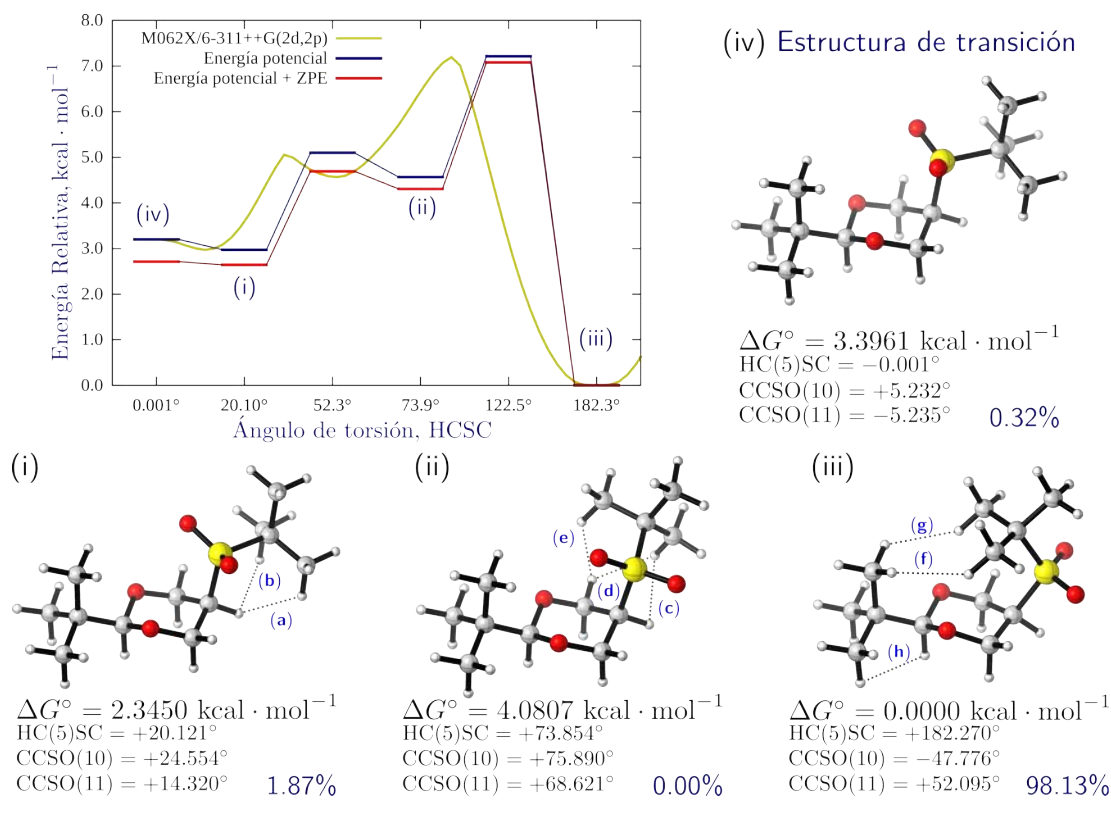
FIGURA 6.1.15: Conformémeros del cis-2- tert -butil-5-( tert -butilsulfonyl)-1,3-dioxano. Estructuras optimizadas al nivel de teoría: M06-2X/6-311++G(2d,2p). Distancia entre hidrógenos: (a) 2.1366 Å; (b) 2.3279 Å; (c) 2.5877 Å; (d) 2.1267 Å; (e) 2.0108 Å; (f) 2.3312 Å; (g) 2.3911 Å y (h) 2.4811 Å.
