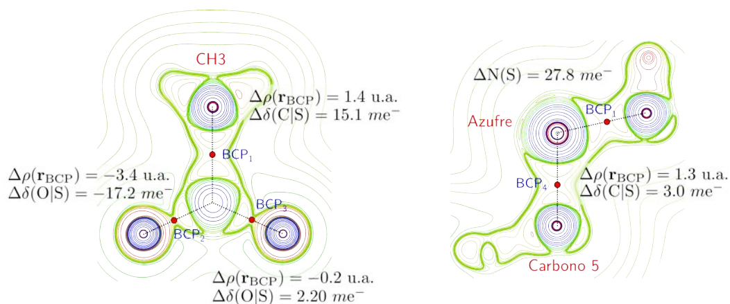
FIGURA 6.1.19: Curvas de contorno del \nabla^2\rho(\mathbf{r}) sobre el fragmento \text{SO}_2 . Los valores del \Delta\Phi resultan de restar a los valores en el conformero Cis-8B los del conformero Cis-8A.
