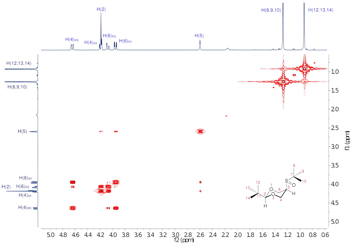
FIGURA B.3.11: Espectro COSY-400MHz del cis -2- tert -butil-5-( tert -butilsulfoni)-1,3-dioxano.
