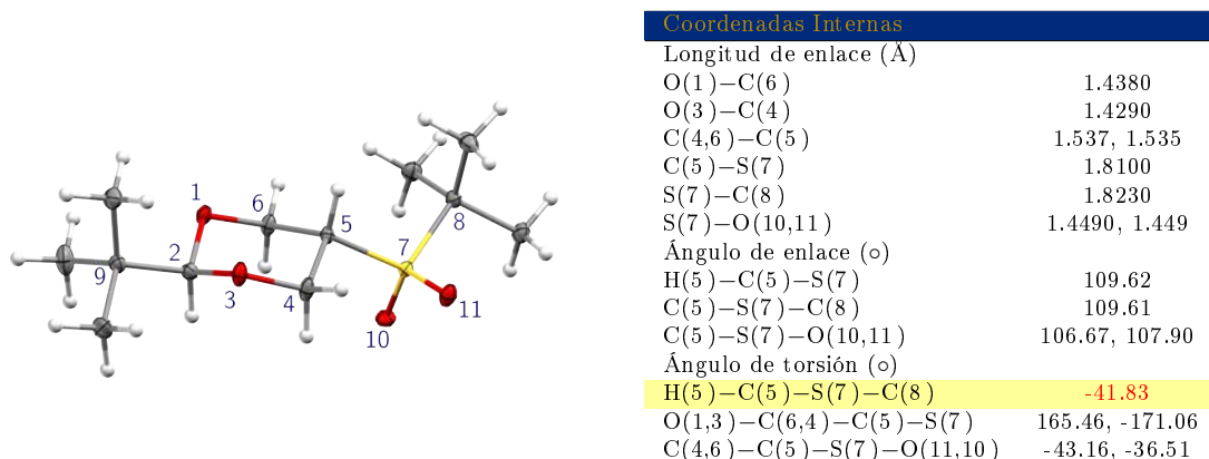
FIGURA 6.1.11: Análisis de rayos X del trans -2- tert -butil-5-( tert -butilsulfinil)-1,3-dioxano ( Trans -5). Figura: Diagrama ORTEP de Trans -5 (Elipsoides térmicos a un nivel de probabilidad del 50 %, T = 100 K). Tabla: Datos correspondientes a los parámetros internos de la estructura molecular.
