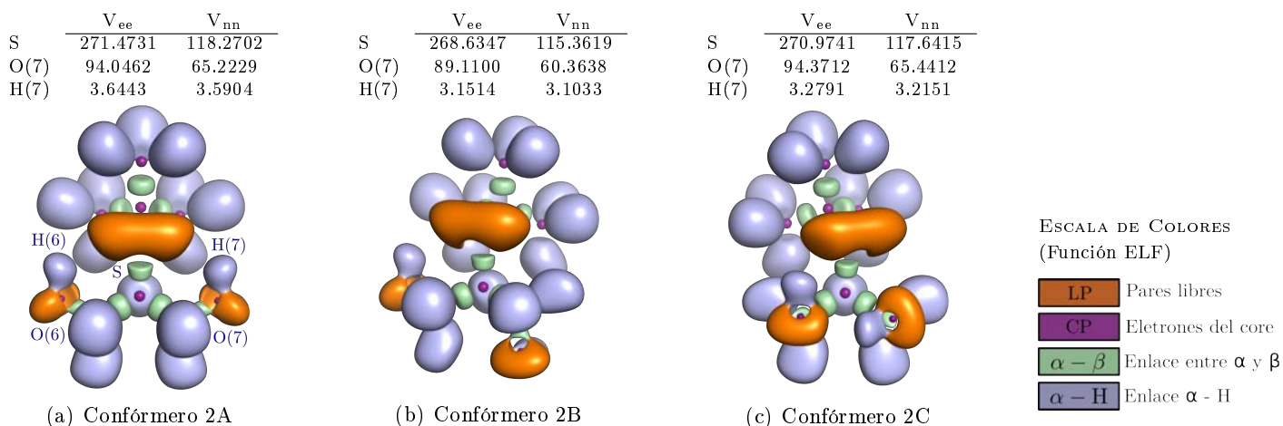
FIGURA 5.3.10: Isosuperficies ELF ( \eta = 0.8 ) de los confórmeros del 2- tert -butilsulfenilpropano-1,3-diol. Valores de energía potencial de repulsión en u.a., derivadas del análisis de densidad electrónica bajo el esquema QTAIM.
