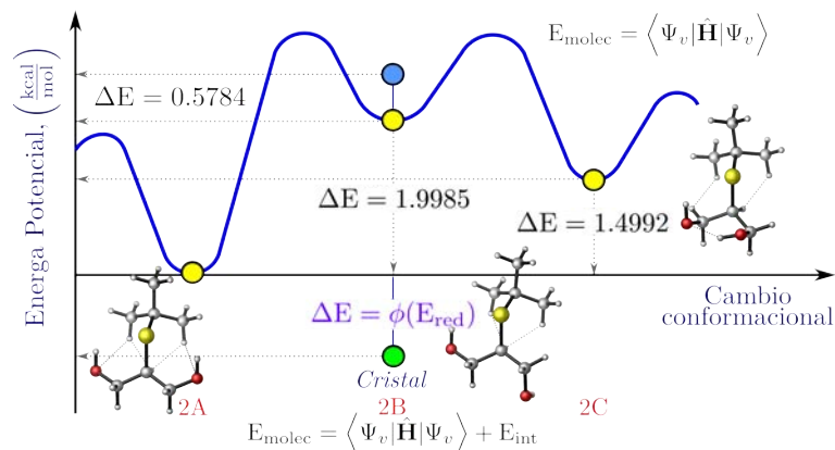
FIGURA 5.3.7: Cambio conformacional en el 2- tert -butilsulfenil-propano-1,3-diol. Datos derivados del análisis de la PES, empleando el nivel de teoría M06-2X/6-311++G(2d,2p).
