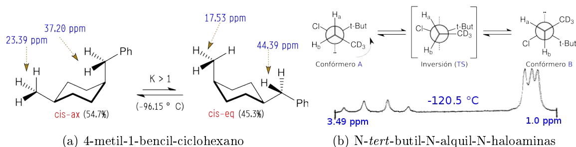
FIGURA 3.3.5: Análisis conformacional en sistemas dinámicos. (a) Equilibrio de inversión del 4-metil-1-bencil-ciclohexano; (b) A T = -120.5\text{ }^{\circ}\text{C} , se logra diferenciar los protones del metileno ( -\text{CH}_2- ), correspondiente a dos ambientes químicos diferentes, el del confórmero A y el confórmero B , además de la diferenciación de los metilenos del grupo -tert -butilo [41].
