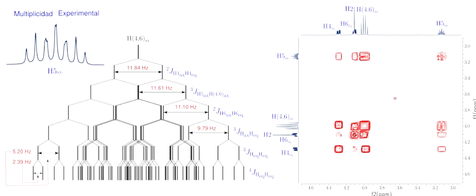
FIGURA B.2.5: Multiplicidad del protón H 5,ax para el trans -2-tert-butil-5-(tert-butilsulfinil)-1,3-dioxano (Trans-4). Segmento del espectro COSY (500 MHz, CDCl 3 , 25 °C TMS) .
