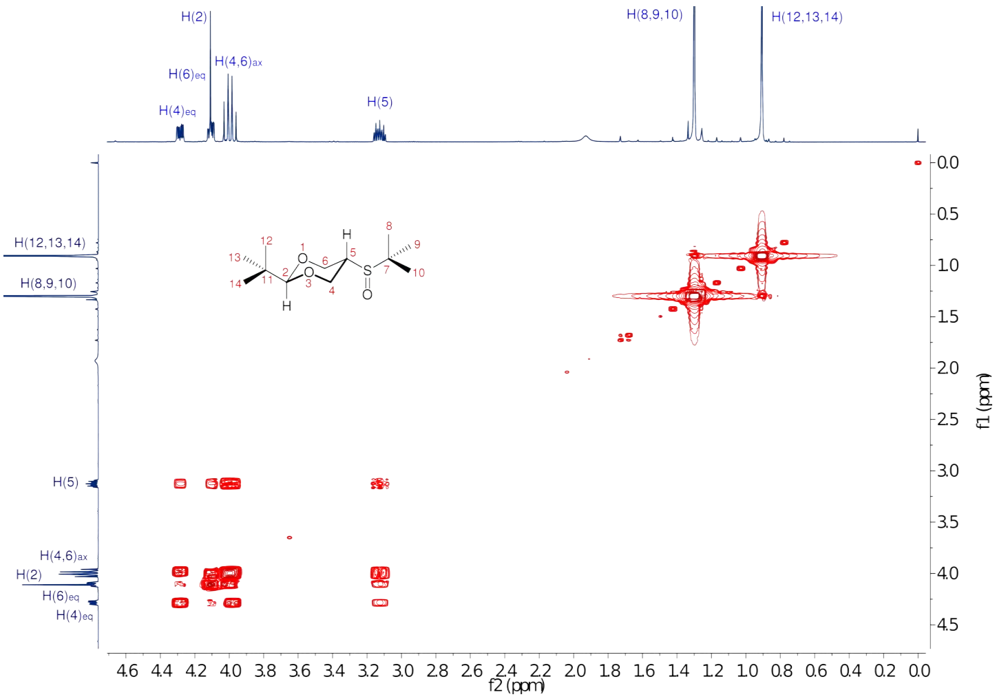
FIGURA B.3.9: Espectro Cosy-500MHz del trans -2- tert -butil-5-( tert -butilsulfínil)-1,3-dioxano.
