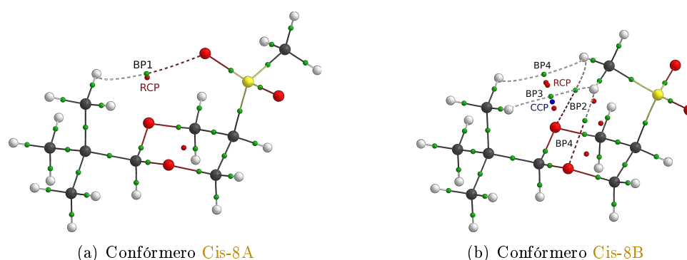
FIGURA 6.1.18: Diagramas Moleculares Resultantes de la Integración Sobre la Densidad para cis -2- tert -butil-5-(metilsulfonil)-1,3-dioxano.
