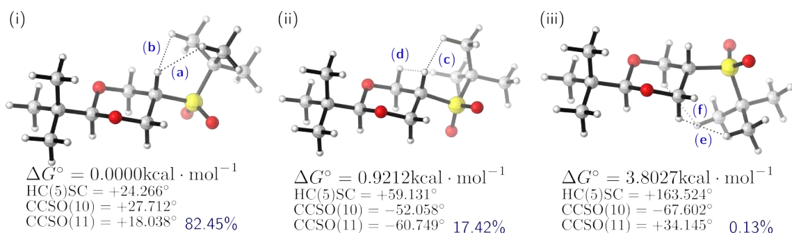
FIGURA 6.1.11: Análisis de rayos X del trans -2- tert -butil-5-( tert -butilsulfinil)-1,3-dioxano ( Trans -5). Figura: Diagrama ORTEP de Trans -5 (Elipsoides térmicos a un nivel de probabilidad del 50 %, T = 100 K). Tabla: Datos correspondientes a los parámetros internos de la estructura molecular.
