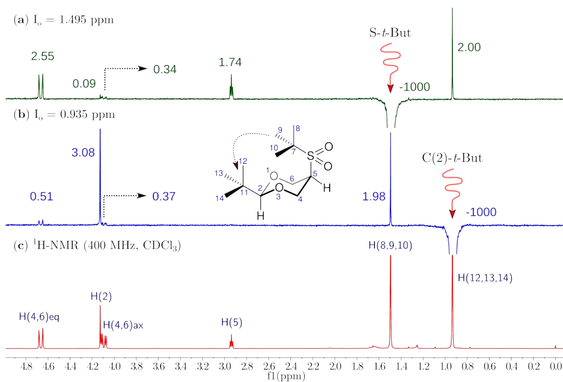
FIGURA 6.1.16: Espectros NOESY-1D del compuesto cis -2- tert -butil-5-( tert -butilsulfonyl)-1,3-dioxano. En el espectrómetro de 400 MHz en \text{CDCl}_3 a temperatura ambiente.
