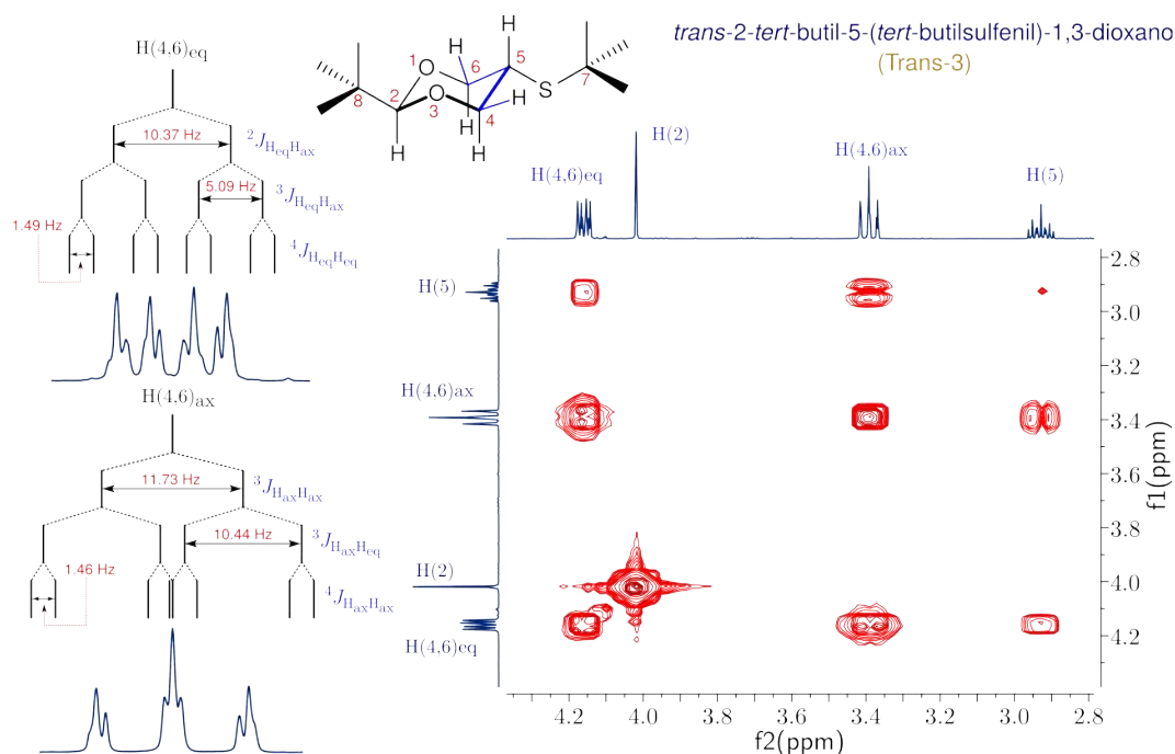
FIGURA B.2.2: Multiplicidad de Hidrógenos H ax y H eq en el 2- tert -butil-5-( tert -butilsulfenil)-1,3-dioxano ( Trans-3 ). Segmento del espectro bidimensional COSY (500 MHz, CDCl 3 , 25 °C TMS) donde se comprueban los acoplamientos a tres enlaces de distancia.
