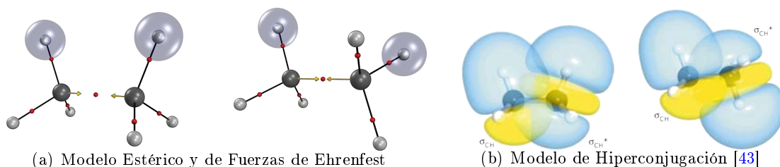
FIGURA 3.4.1: Modelos empleados en el estudio conformacional. Sistema Etano.
