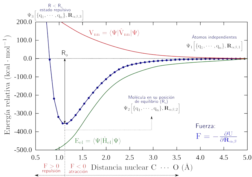
FIGURA 3.1.1: Curva de energía potencial de la molécula de monóxido de carbono.
