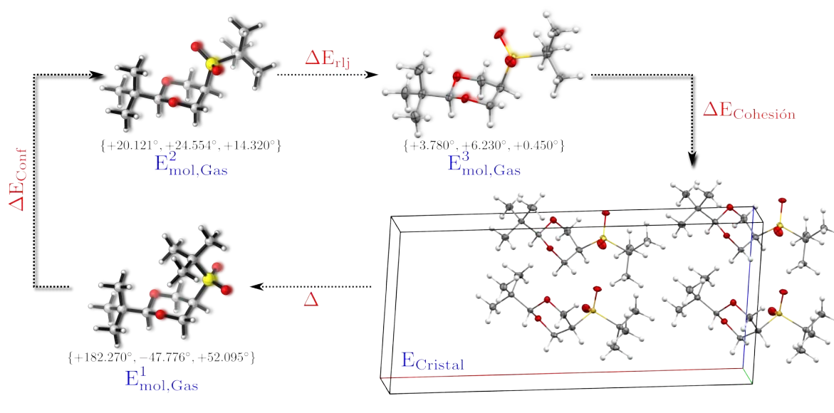
FIGURA 6.2.2: Cambio conformacional en el proceso de cristalización del cis -2- tert -butil-5-( tert -butilsulfonyl)-1,3-dioxano. Los valores entre llaves corresponde a los ángulos de torsión \{\phi_1, \phi_2, \phi_3\} \equiv \{\text{HCSC}, \text{CCSO}(10), \text{CCSO}(11)\} .
