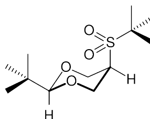
cis -2- tert -Butil-5-( tert -butilsulfonil)-1,3-dioxano
