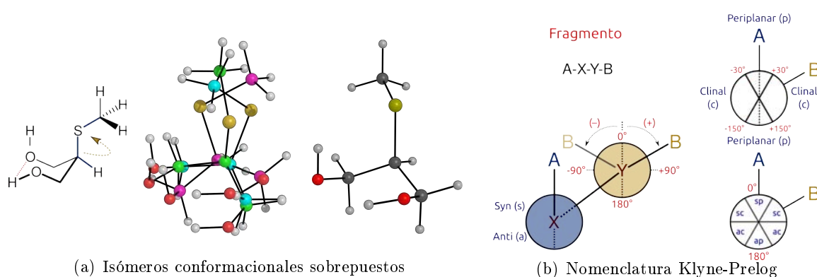
FIGURA 3.3.1: Análisis conformacional. (a) Población de isómeros conformacionales, y conforméromo más estable, generados al rotar el enlace C–S del 2-metilsulfenil-propano-1,3-diol; (b) Nomenclatura propuesta por Klyne y Prelog.
