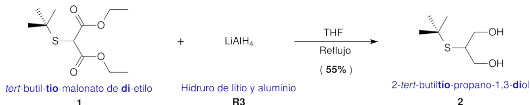
ESQUEMA B.3.4: Reducción del grupo ester a alcohol.
