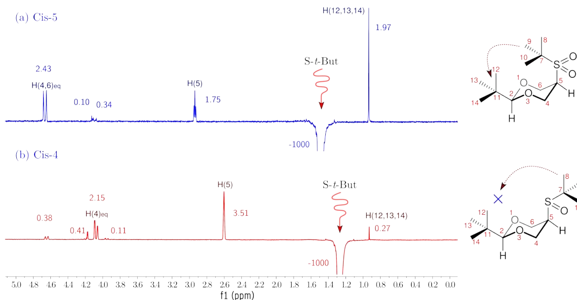
FIGURA 6.1.17: Comparación de espectros NOESY-1D del compuesto cis -2- tert -butil-5-( tert -butilsulfinil)-1,3-dioxano y del cis -2- tert -butil-5-( tert -butilsulfonyl)-1,3-dioxano. En el espectrómetro de 400 MHz en \text{CDCl}_3 a temperatura ambiente.
