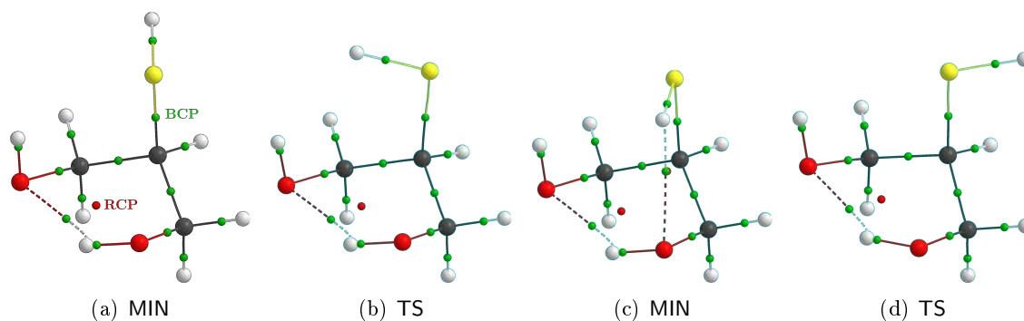
FIGURA 5.3.3: Gráficos moleculares del 2-mercapto-propano-1,3-diol. (a) E_{\text{molec}} = -667.73624526 u.a.; (b) E_{\text{molec}} = -667.72842562 u.a.; (c) E_{\text{molec}} = -667.73822994 u.a.; (d) E_{\text{molec}} = -667.73090455 u.a. Resultados obtenidos con M06-2X/6-311++G(2d,2p).
