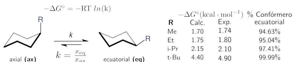
FIGURA 1.0.1: Equilibrio conformacional del ciclohexano monosustituido con algunos grupos alquilo. Los valores de \Delta G^\circ se encuentran a T = 298.15 \text{ K} . [1, 2]
