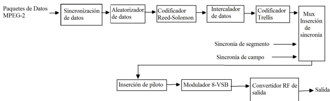
Figura 1.1 Diagrama de bloques ATSC
