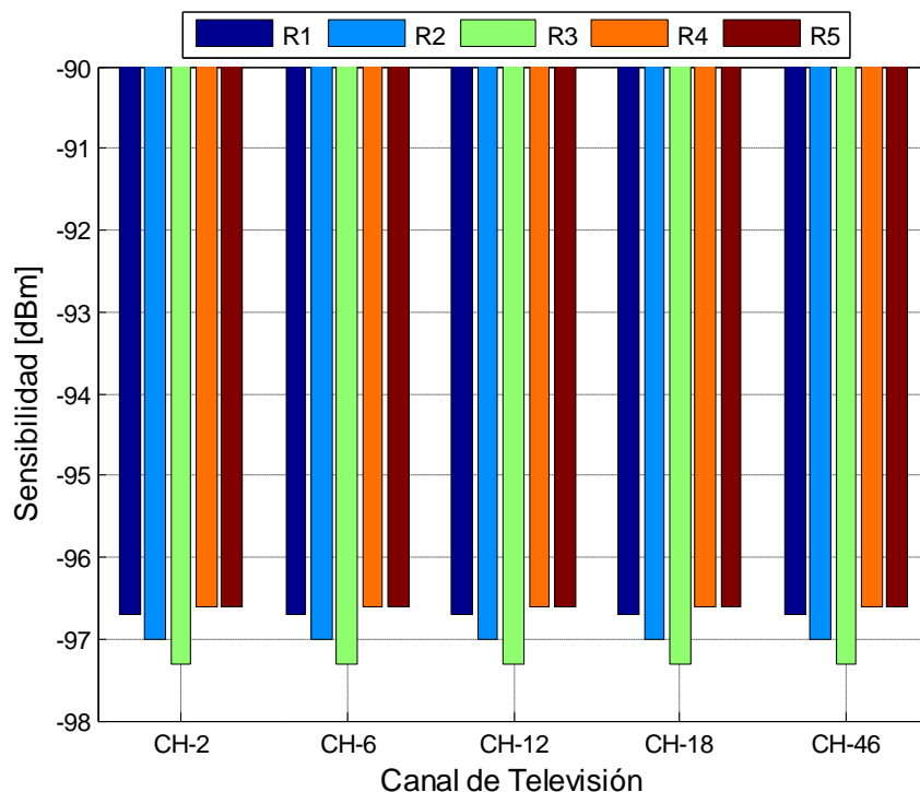
Figura 4.1 Sensibilidad medida de cada receptor ATSC-M/H en cinco diferentes canales de televisión al utilizar la configuración C1 (QQQQ RS 48)
