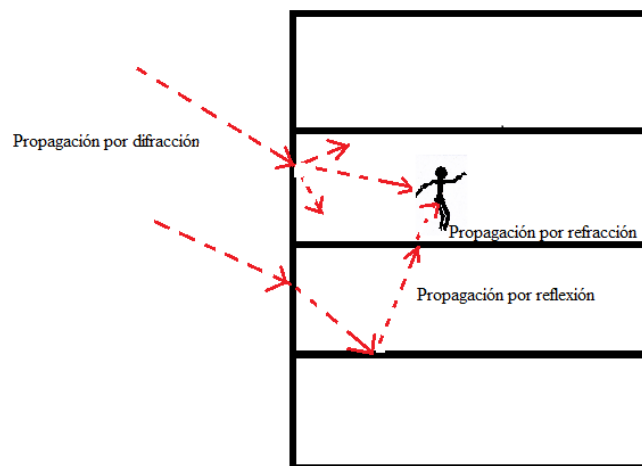
Figura 2.2 Entorno de propagación dentro de un edificio
