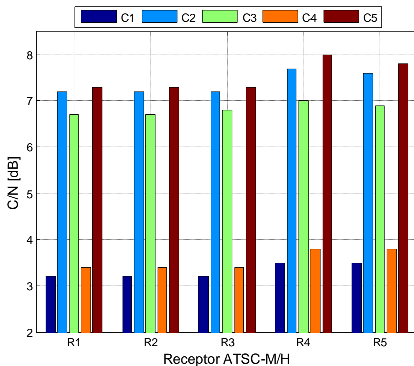
Figura 4.4 Umbral de C/N medido de cada receptor ATSC-M/H en el canal 18 al utilizar las cinco diferentes configuraciones de FEC
