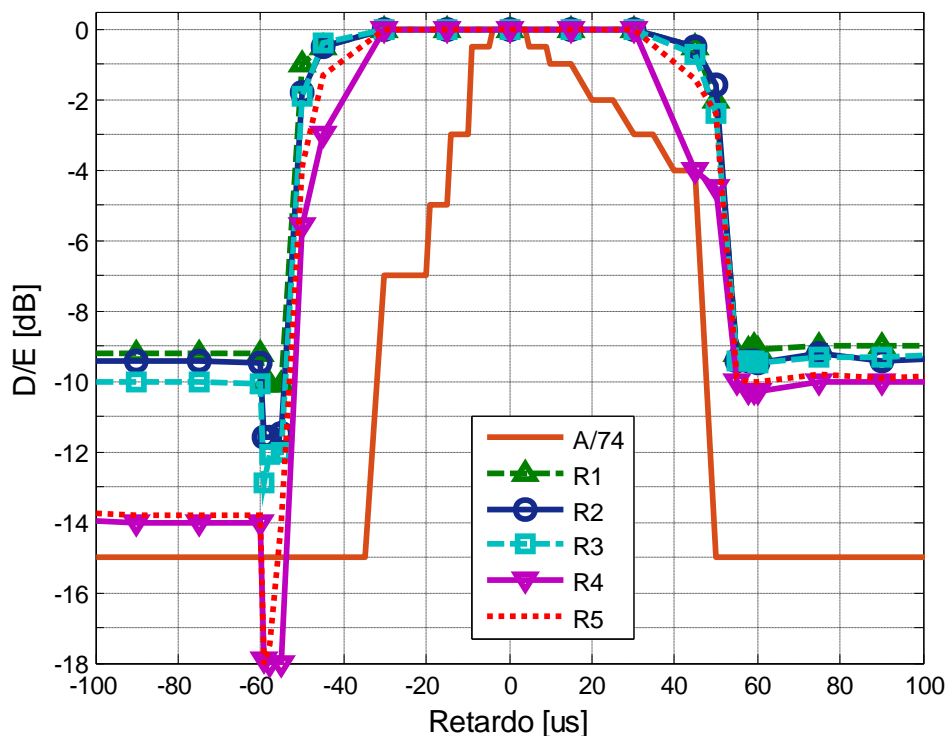
Figura 4.16 Respuesta de los receptores ante una red SFN de dos transmisores al utilizar la configuración C3 (HQQ RS 48) dentro de un modelo de recepción fija en interiores
