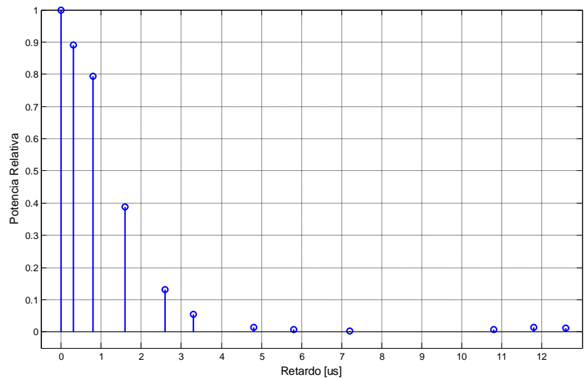
Figura 2.10 Canal de propagación Vehicular Urbano en una red SFN (30 km/h)
