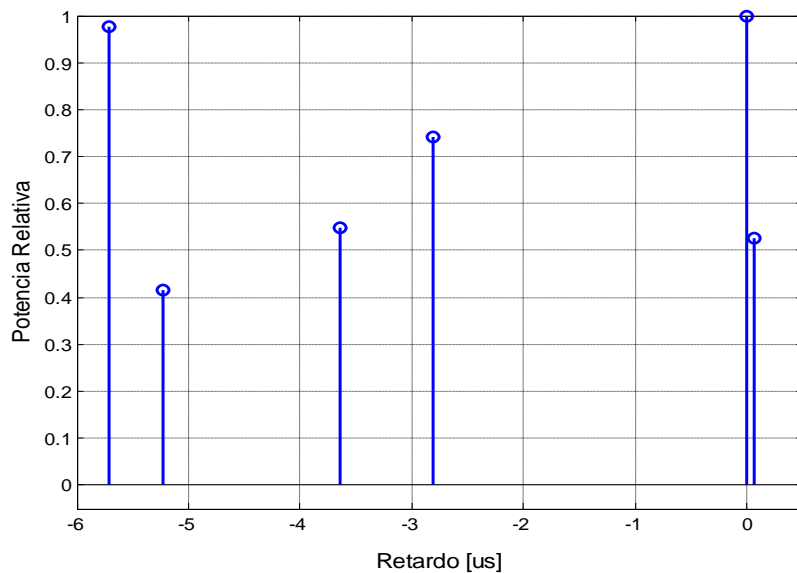
Figura 2.5 Canal de propagación Brasil D
