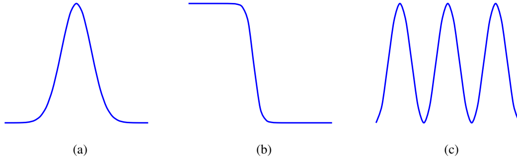
Figura 3.2: Ondas viajeras con distintas formas: Pulso en a), Frente en b), Trenes de onda en c)
