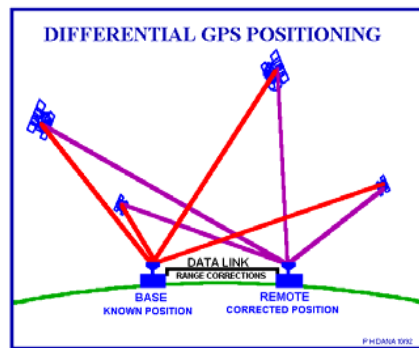
Figura 22. Esquema de funcionamiento de GPS diferencial.
