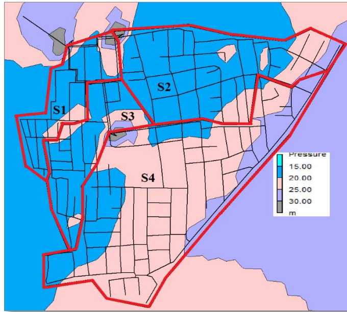
Fig. IV-28 Regulación de presiones con 4 sectores – Caso 2
