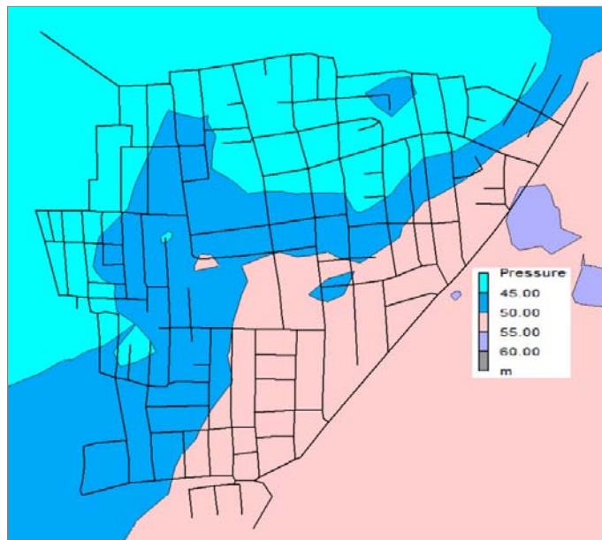
Fig. II-21 Presiones con 75% de roturas en la red
