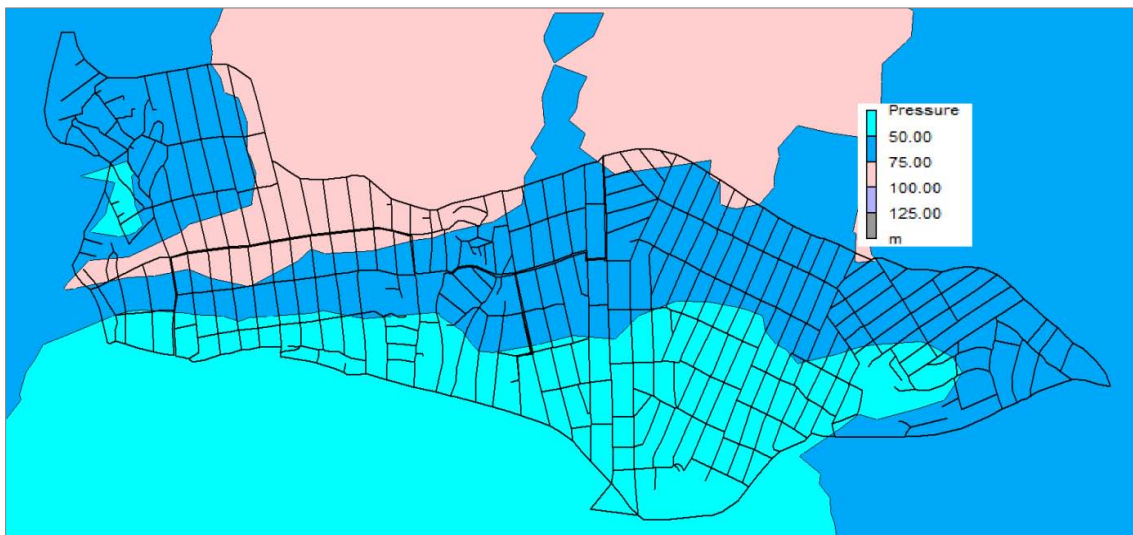
Fig. II-12 Presiones con el 75% de roturas en la red
