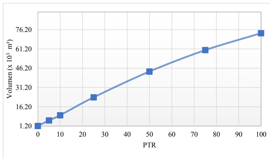
Fig. II-23 Volumen total sin sectorizar y sin control de presiones
