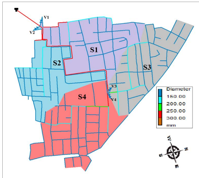
Fig. IV-13 Red con 4 sectores, diámetros y VRP – Caso 1
