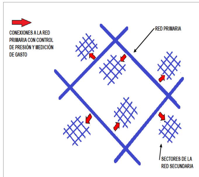
Fig. III-1 Sectorización de una red de agua potable
