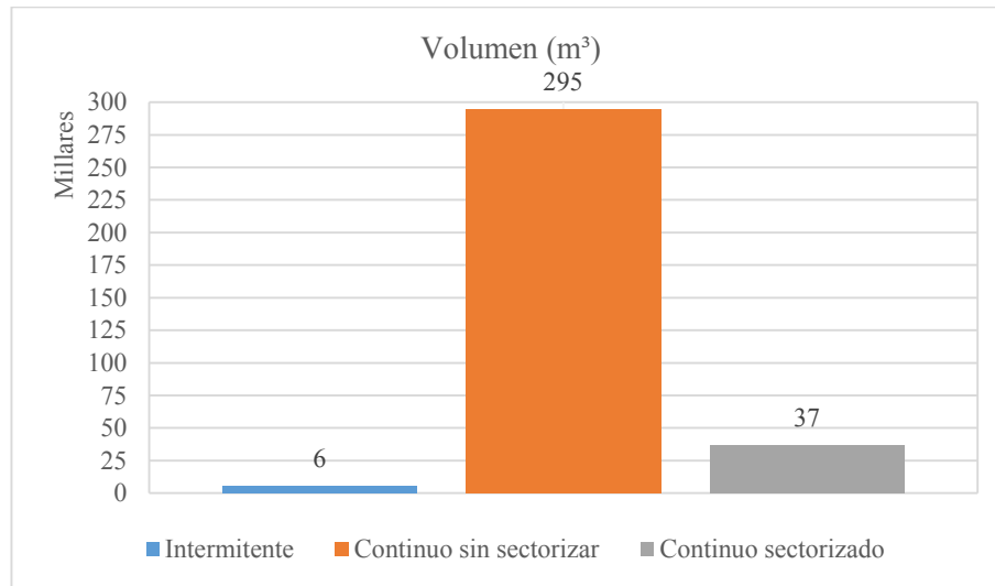
Fig. V-11 Volumen suministrado en un día con 15% de roturas en la red
