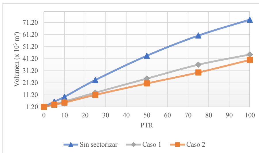
Fig. V-10 Volumen total con y sin regular presiones para 4 sectores
