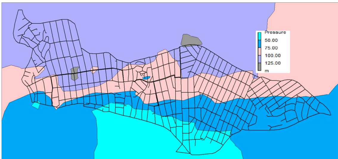
Fig. II-10 Presiones con el 25% de roturas en la red
