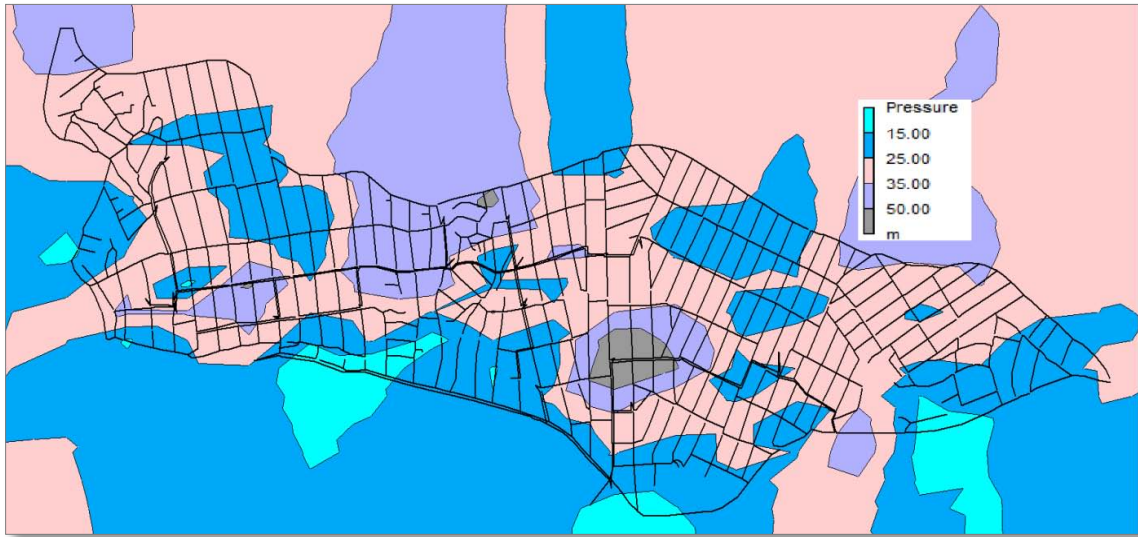
Fig. IV-8 Control de presiones con 75% de roturas en la red
