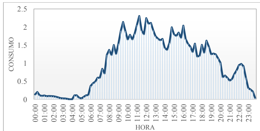
Fig. II-4 Patrón de demanda sin fugas
