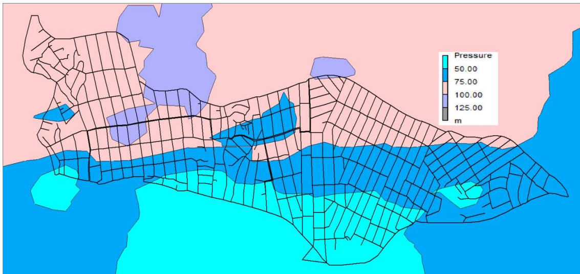
Fig. II-11 Presiones con el 50% de roturas en la red
