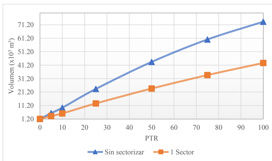
Fig. V-7 Volumen total con y sin regular presiones
