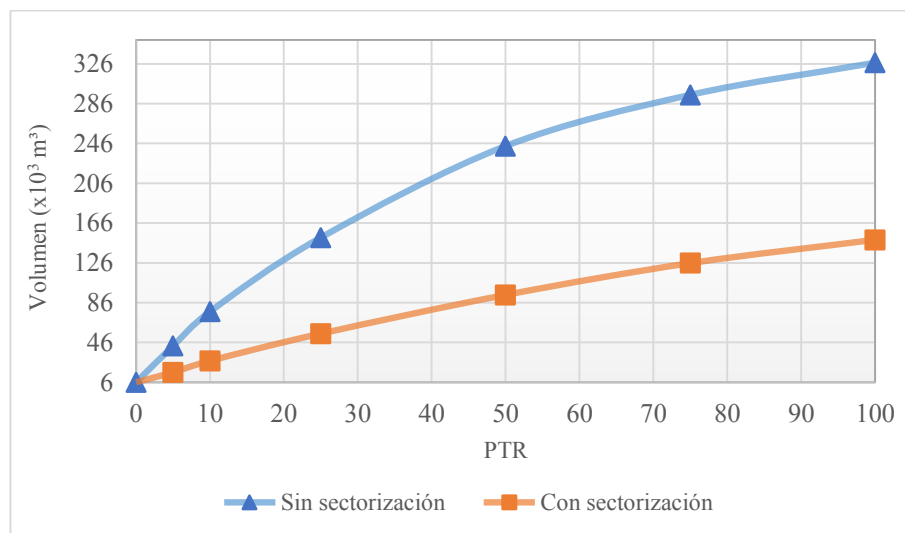
Fig. V-6 Volumen total con y sin sectorización
