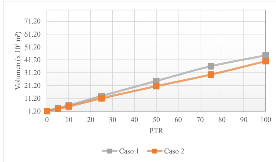
Fig. IV-17 Volumen total con sectorización y control de presiones
