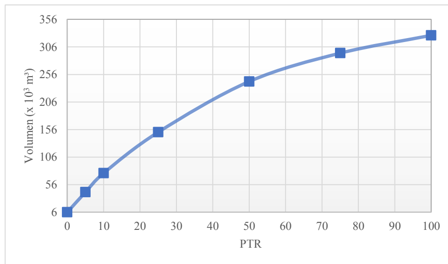
Fig. II-14 Volumen total sin sectorizar y sin control de presiones
