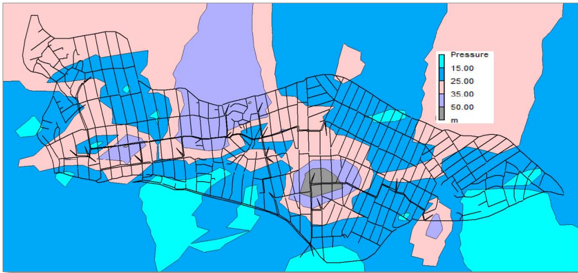
Fig. IV-9 Control de presiones con 100% de roturas en la red
