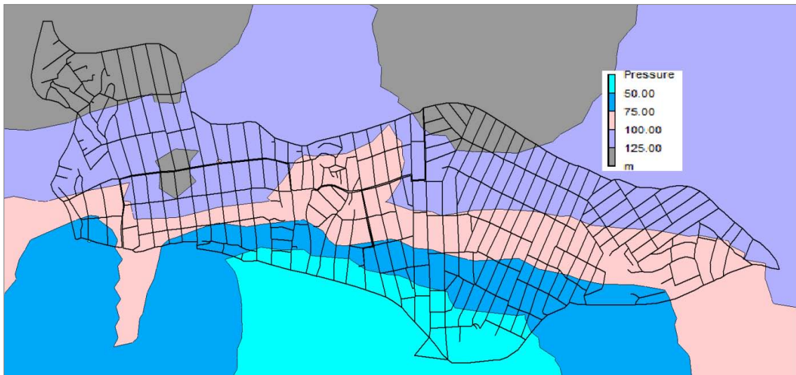
Fig. II-9 Presiones con 0, 5 y 10 % de roturas en la red
