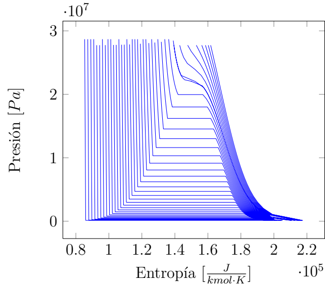
Figura 5.8: Diagrama de presión-entropía para el agua. Las líneas azules representan isothermas.
