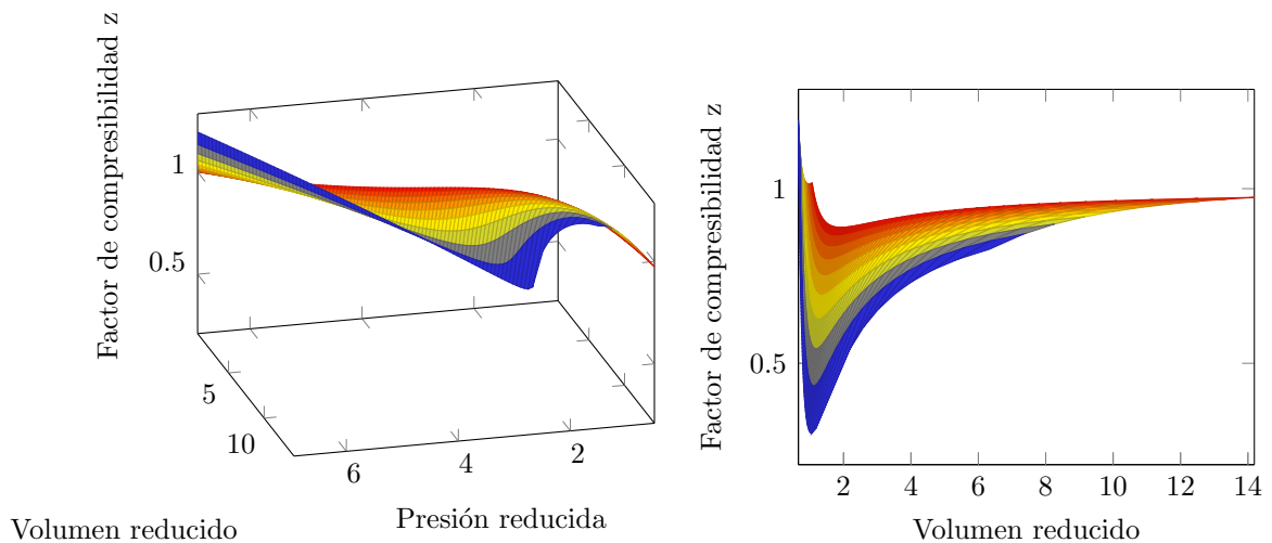
Figura 5.4: Izquierda: Diagrama tridimensional 'Factor de compresibilidad'-'volumen reducido'-'presión reducida'. Derecha: 'Factor de compresibilidad'-'volumen reducido'. Ambas figuras calculadas con la ecuación de Van Der Waals para el heptano
