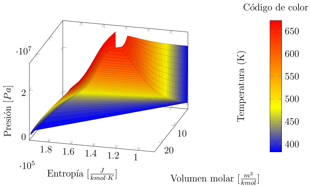
Figura 5.9: Diagramas tridimensional presión-entropía-‘volumen molar’ para el agua.
