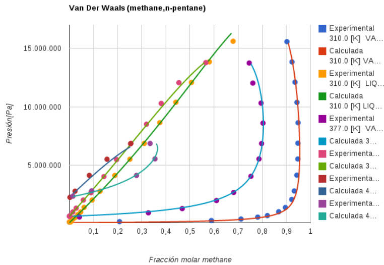
Figura 8.1: Comparación para el sistema (1)Metano,(2)Pentano con la regla de mezclado de Van Der Waals y la ecuación de estado PRSK. Izquierda figura obtenida con la librería Materia , Derecha Figura del libro [8] página 27.
