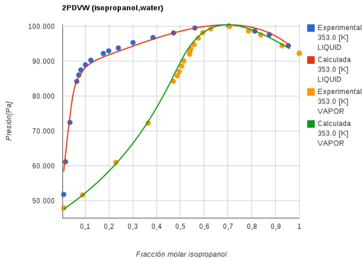
Figura 8.2: Comparación para el sistema (1)2-Propanol,(2)Agua con la regla de mezclado de Van Der Waals de 2 parámetros '2PVDW' y la ecuación de estado PRSK. Izquierda figura obtenida con la librería Materia , Derecha Figura del libro [8] página 37.
