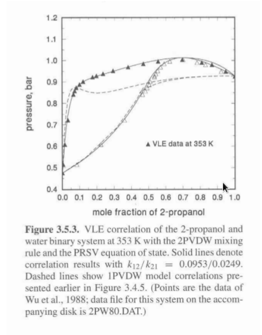
Figura 8.2: Comparación para el sistema (1)2-Propanol,(2)Agua con la regla de mezclado de Van Der Waals de 2 parámetros '2PVDW' y la ecuación de estado PRSK. Izquierda figura obtenida con la librería Materia , Derecha Figura del libro [8] página 37.
