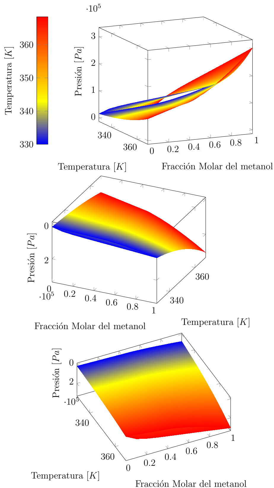
Figura 5.15: Diagramas tridimensionales de presión-composición-temperatura para el sistema metanol-agua. En la figura podemos observar los planos formados por el líquido y el vapor saturado obtenidos con el cálculo de presión de burbuja. Los diagramas son la misma figura vista desde diferentes ángulos.
