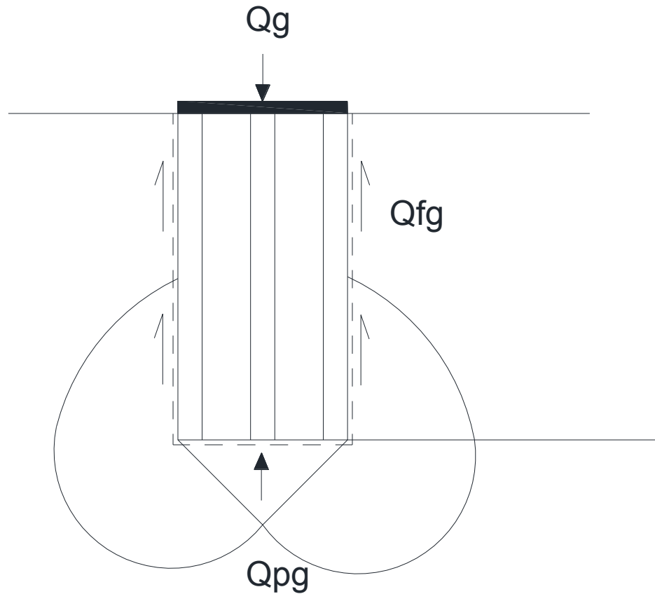
Figura 2.18: Falla de un grupo de pilotes, Tamez (2001).
