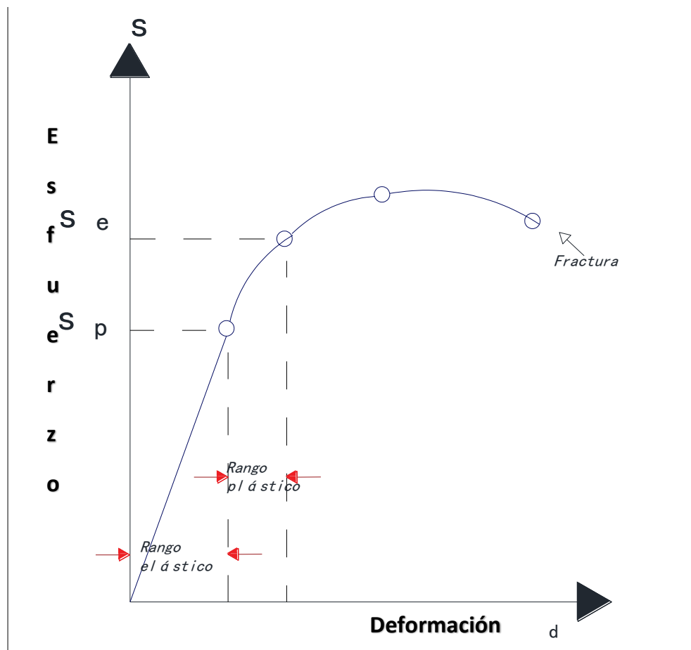
Figura 3.6: curva esfuerzo-deformación
