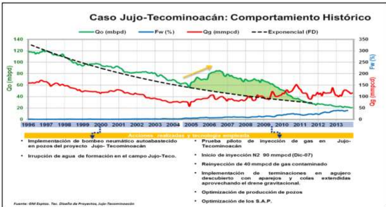
Comportamiento Histórico Jujo-Ticomán. GM.Tec, diseño de proyectos Jujo-Ticomán. Gráfica 4.
