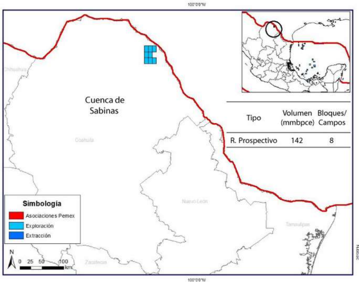
Mapa de yacimientos no convencionales de gas a nivel nacional. Fuente: Sistema de Información Energética, Secretaría de Energía, 2015. Figura 6.
