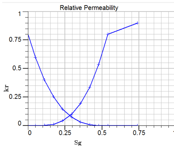
Ilustración 64 - Curvas de permeabilidad aceite-agua para matriz .
