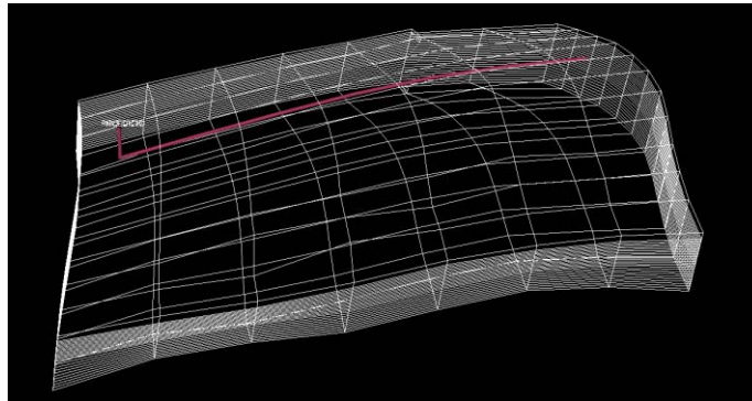
Ilustración 147- Malla del elemento de simetría y localización de pozos.
