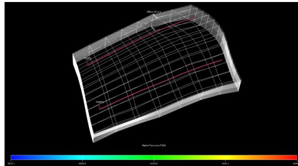
Ilustración 173- Malla del elemento de simetría y localización de los pozos.
