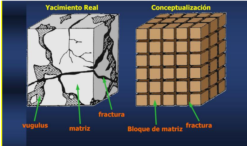
Ilustración 27-Diagrama del modelo de Warren y Root (Tomado de apuntes del seminario “Simulación de Yacimientos Naturalmente Fracturados”, Instituto de Geofísica UNAM, 2006))
