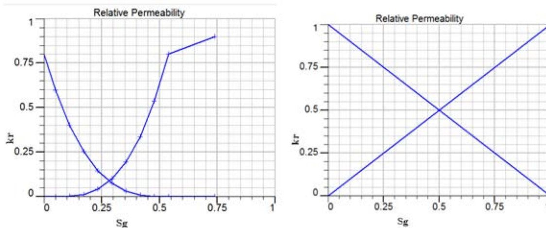
Ilustración 92 Curvas de permeabilidad de aceite-gas para matriz y fractura.
