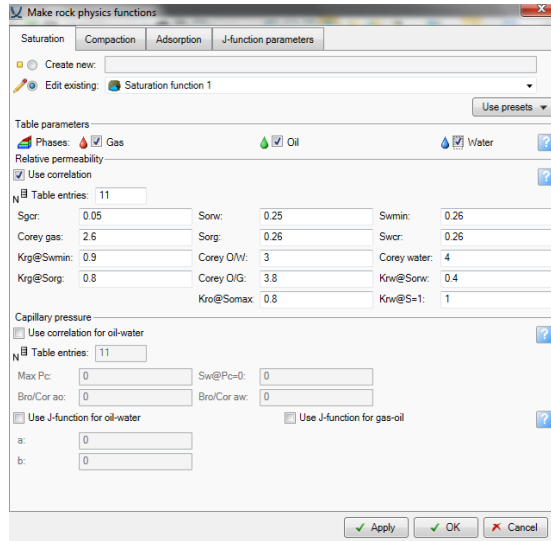
Ilustración 60- Muestra de la aplicación de Petrel para creación de curvas de permeabilidad aceite-agua.
