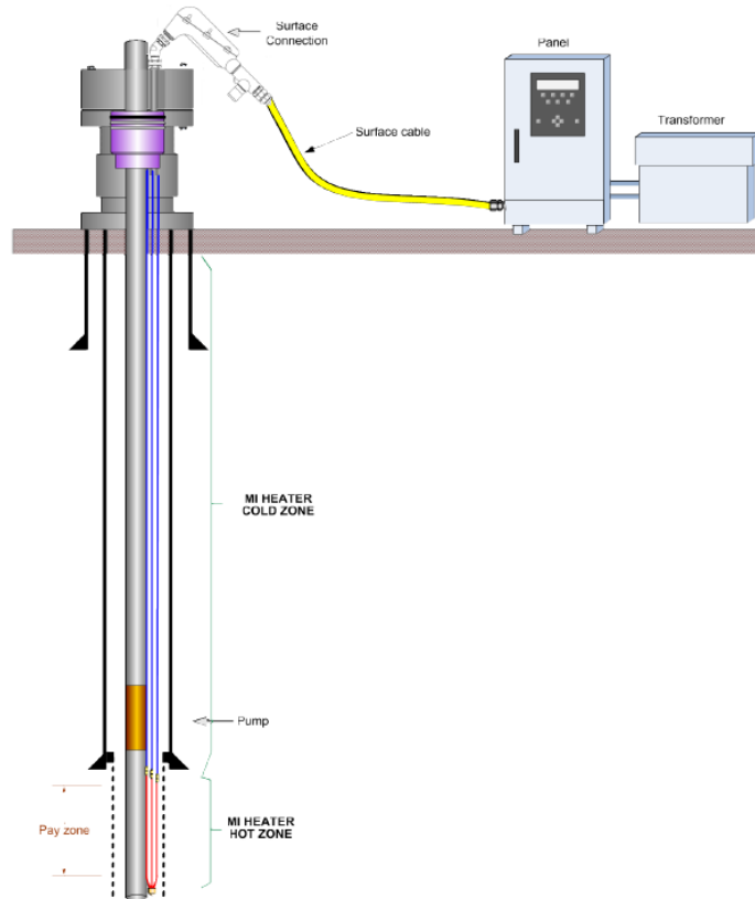
Ilustración 26 Diagrama típico de pozos en California (Samuel s. Ojeda y David G. Parman, SPE 167347 2013)
