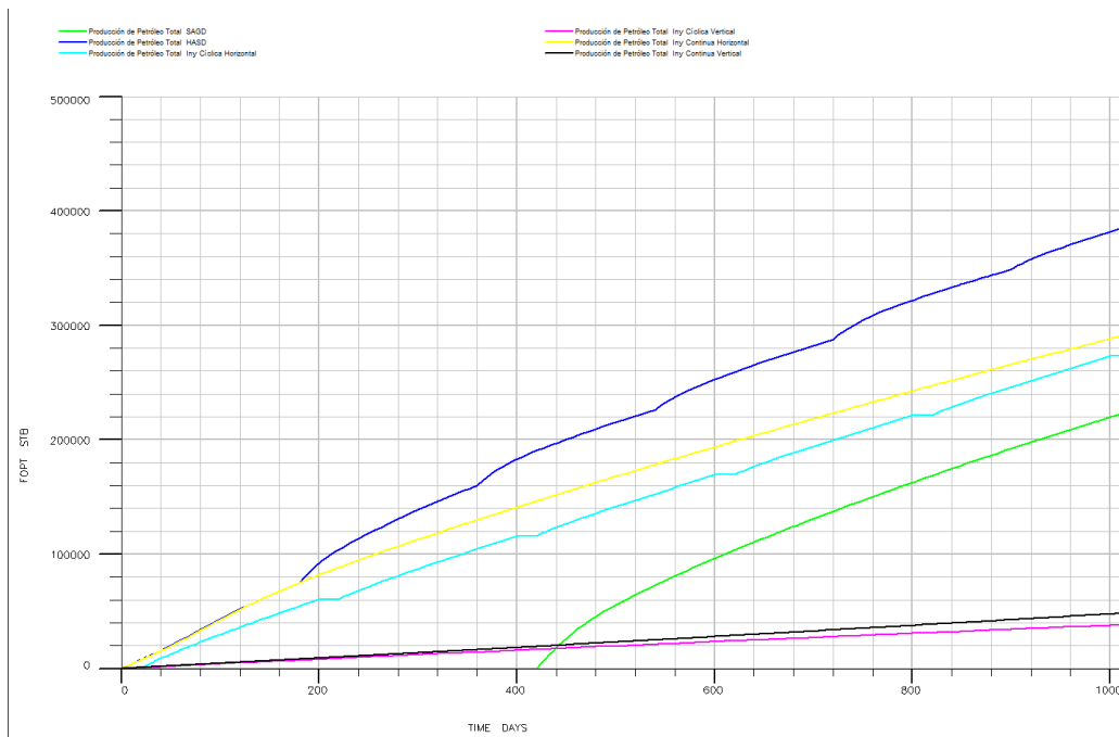
Ilustración 142 - Curvas de producción acumulada de los métodos normalizados.
