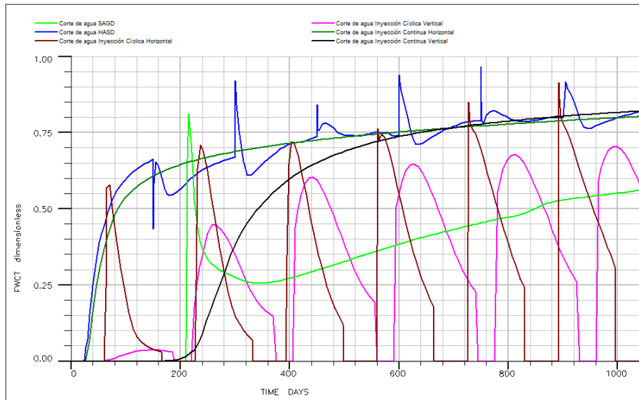
Ilustración 187 Curvas de corte de agua para los casos normalizados.
