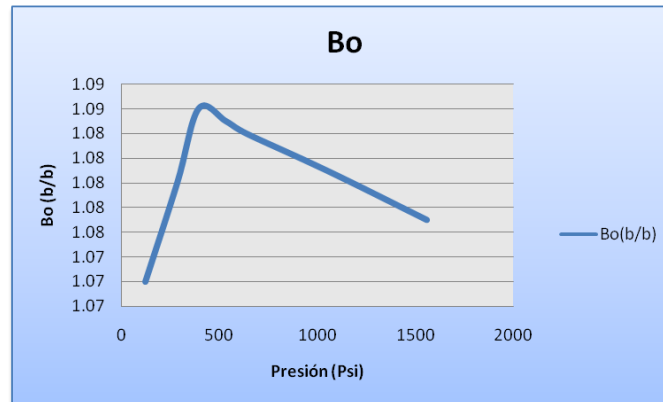
Ilustración 56 - Comportamiento del B_o del fluido PVT
