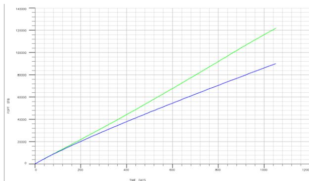
Ilustración 122- Gráfica de producción acumulada por producción natural (línea azul) y método aplicado (línea verde).
