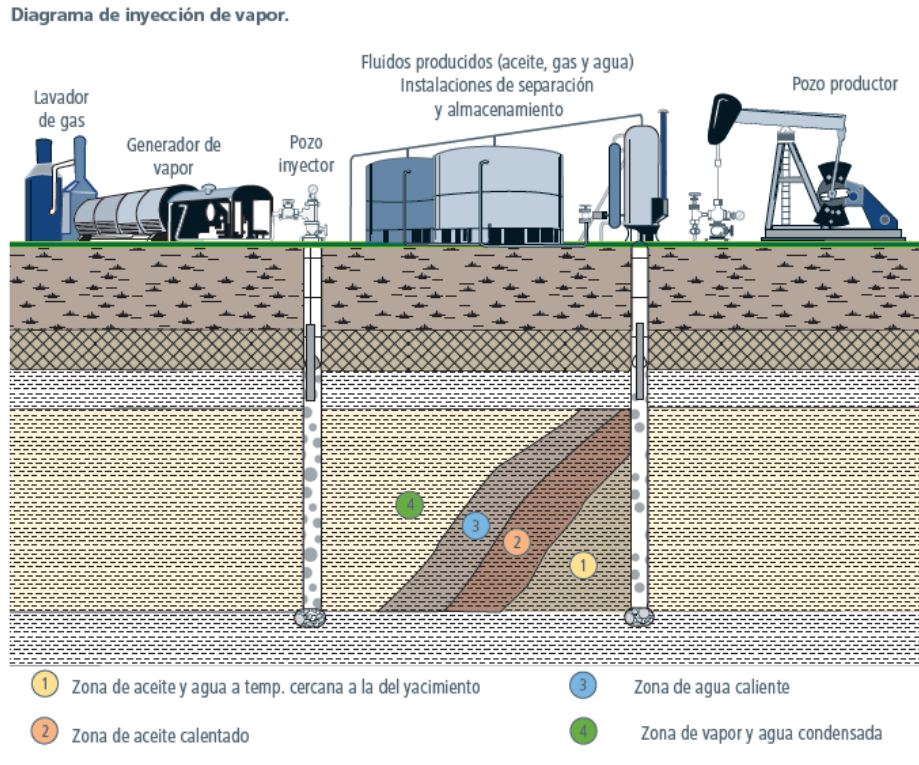
Ilustración 6-Diagrama del Proceso de Inyección Continua de Vapor (Tomada de “El Futuro de la Producción de Aceite en México: Recuperación Avanzada y Mejorada IOR EOR”, Dr. Edgar Rangel German)
