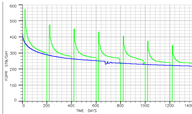
Ilustración 99 - Gráfica de producción diaria por producción natural (línea azul) y método aplicado (línea verde).
