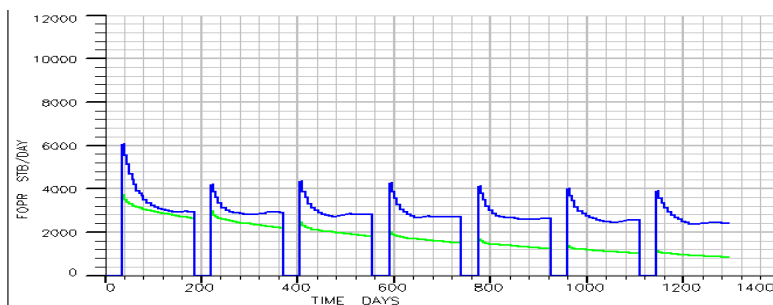
Ilustración 158- Gráfica de producción diaria por producción natural (línea verde) y método aplicado (línea azul).
