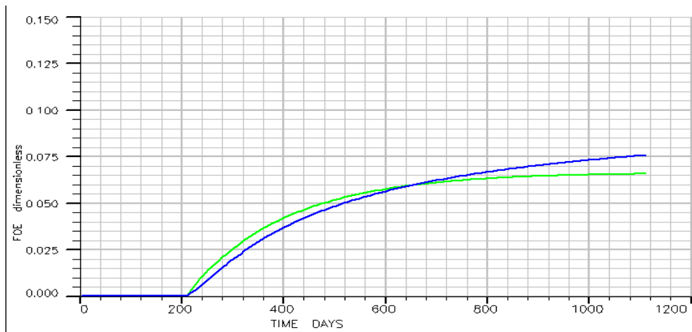
Ilustración 182- Gráfica de factor de recuperación por producción natural (línea verde) y método aplicado (línea azul).
