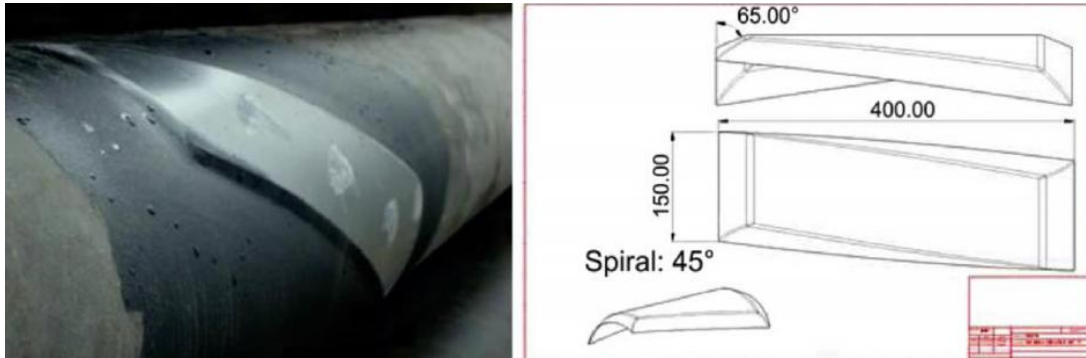
Ilustración 23-Imagen de las cuchillas de un centrador y configuración usada durante la cementación de un pozo para inyección de vapor (Tomado de SPE 171045, F. Ramírez Vázquez y R. Hernández Henrique, H. Briseño, S.E. Moreno Colín, 2014)
