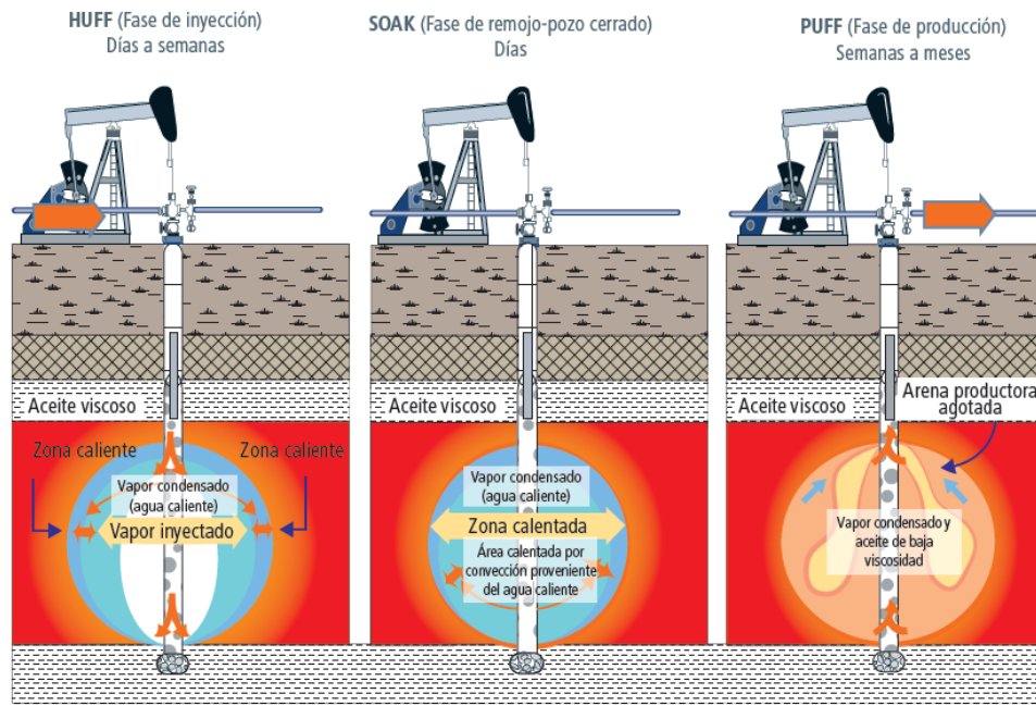
Ilustración 4-Diagrama del Proceso de Inyección Cíclica de Vapor (Tomada de “El Futuro de la Producción de Aceite en México: Recuperación Avanzada y Mejorada IOR EOR”, Dr. Edgar Rangel Germán)
