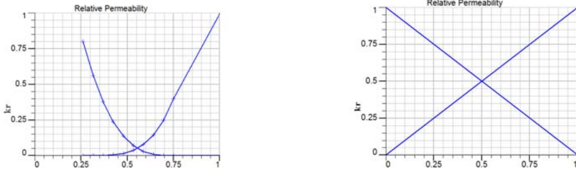
Ilustración 61 - Curvas de permeabilidad aceite-agua para matriz y fractura del elemento de simetría A.
