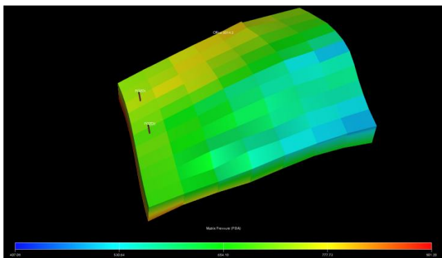
Ilustración 126- Elemento de simetría y localización de pozos.
