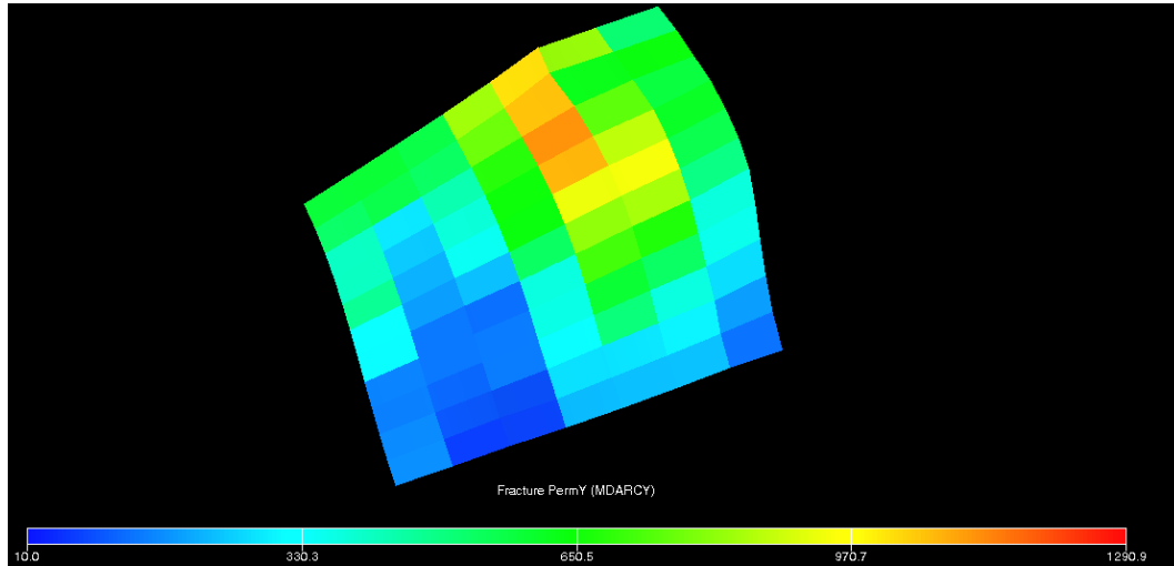
Ilustración 46 - rango y distribución de la permeabilidad en Y de la matriz en el elemento de simetría A.
