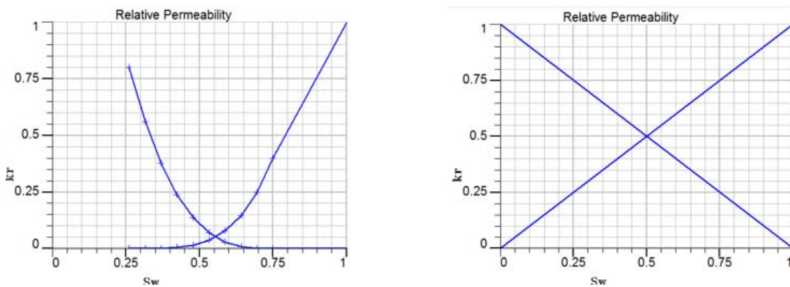
Ilustración 89 - Curvas de permeabilidad de aceite-agua para matriz y fractura.
