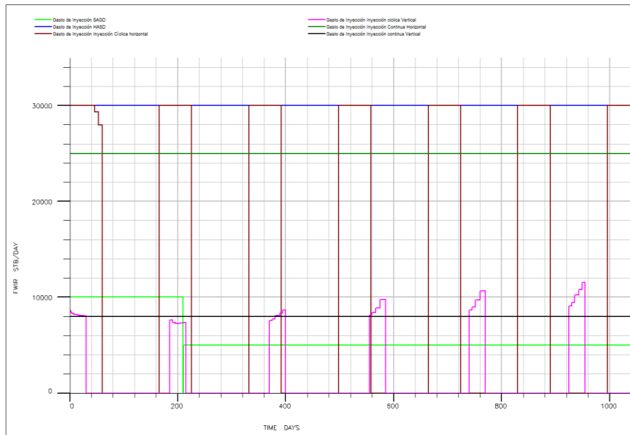
Ilustración 188- Gráfica de gasto de inyección para los casos normalizados.
