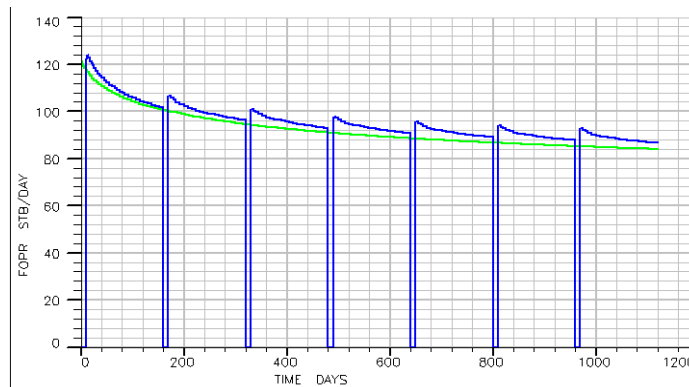
Ilustración 107- Gráfica de producción diaria por producción natural (línea verde) y método aplicado (línea azul).
