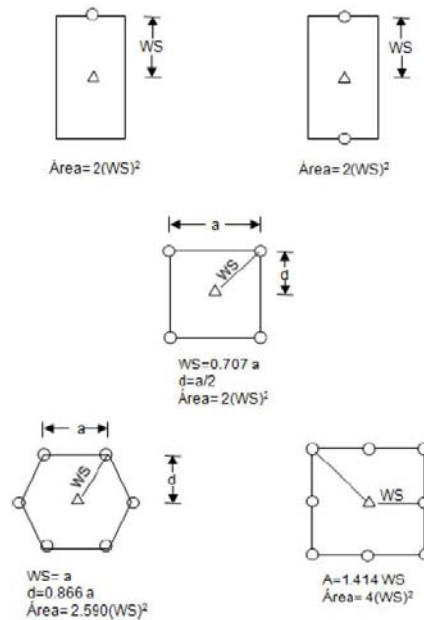
Ilustración 22-Esquema de Tipos de Arreglo ( Jones. J.)
