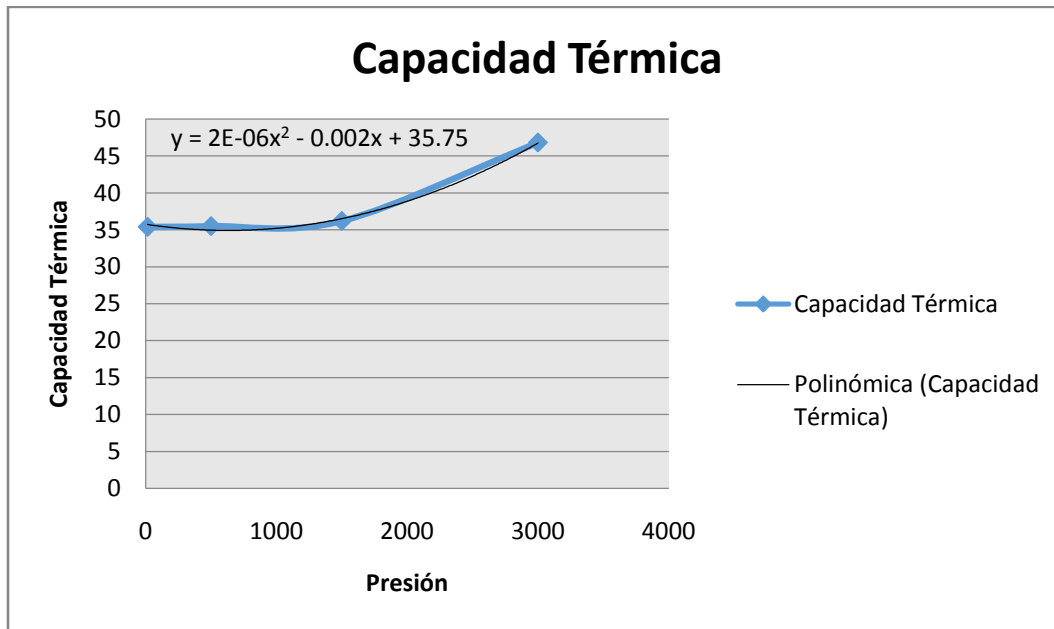
Ilustración 50 - Representación de la capacidad térmica con respecto a la presión.
