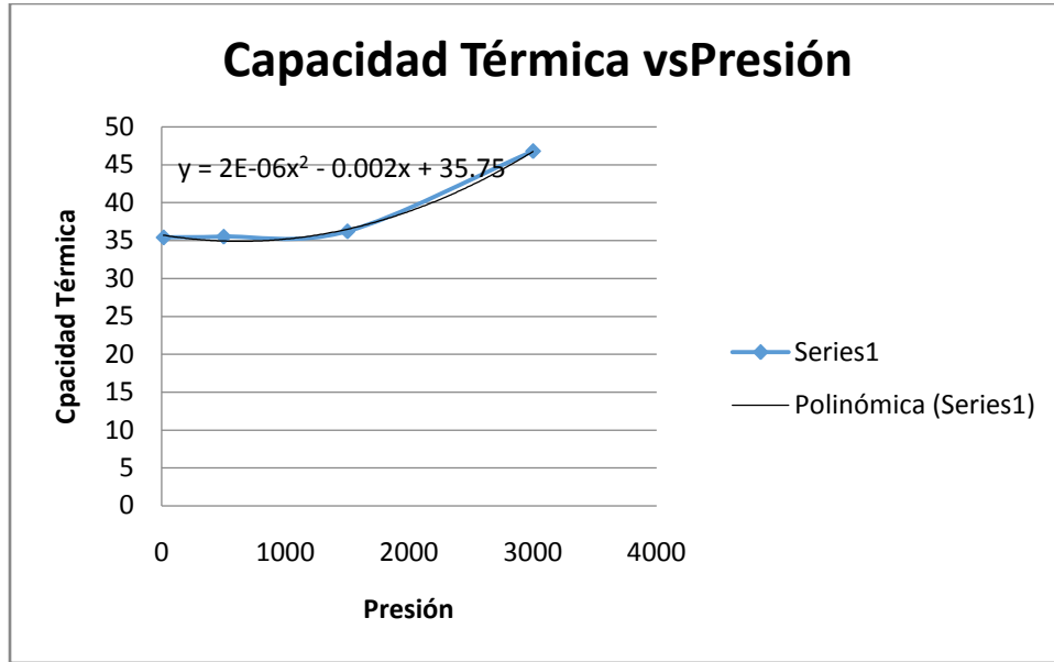
Ilustración 79 Representación de la capacidad térmica con respecto a la presión
