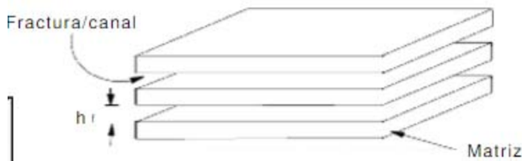
Ilustración 28 Diagrama del modelo de Warren y Root(Tomado de tesis de Miguel Danilo Molina Bohorquez, 2004)
