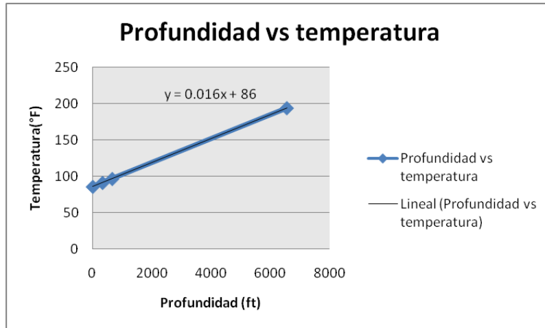
Ilustración 51 - Representación y tendencia de las variables profundidad vs temperatura.
