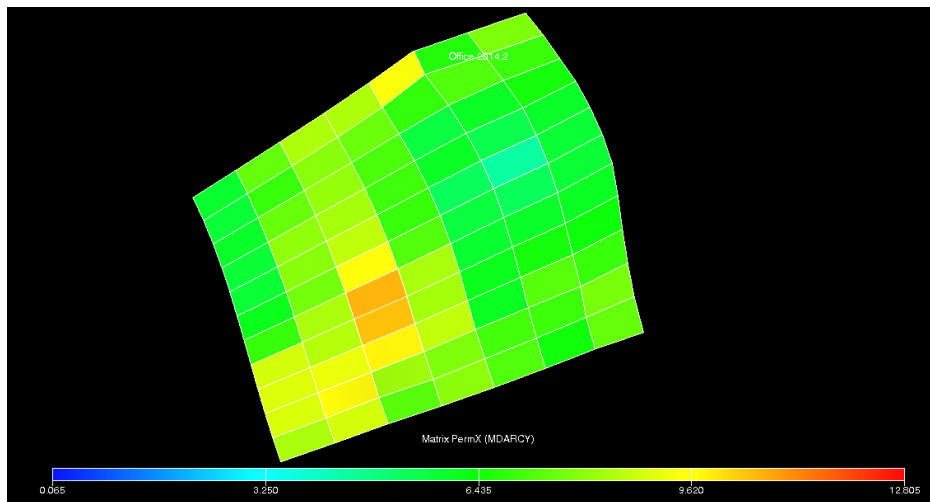
Ilustración 40 - Rango y distribución de permeabilidades en X en la matriz del elemento de simetría A.
