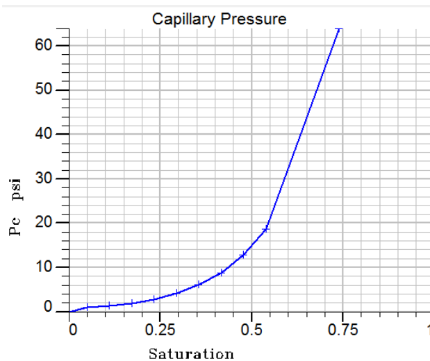
Ilustración 93- Curva de presión capilar en la fase aceite-gas
