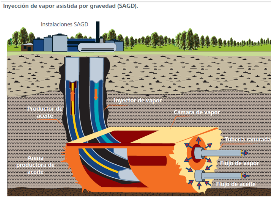
Ilustración 10-Diagrama Del Proceso Segregación Gravitacional Asistida Por Vapor (Tomada de “El Futuro de la Producción de Aceite en México: Recuperación Avanzada y Mejorada IOR EOR”, Dr. Edgar Rangel German)
