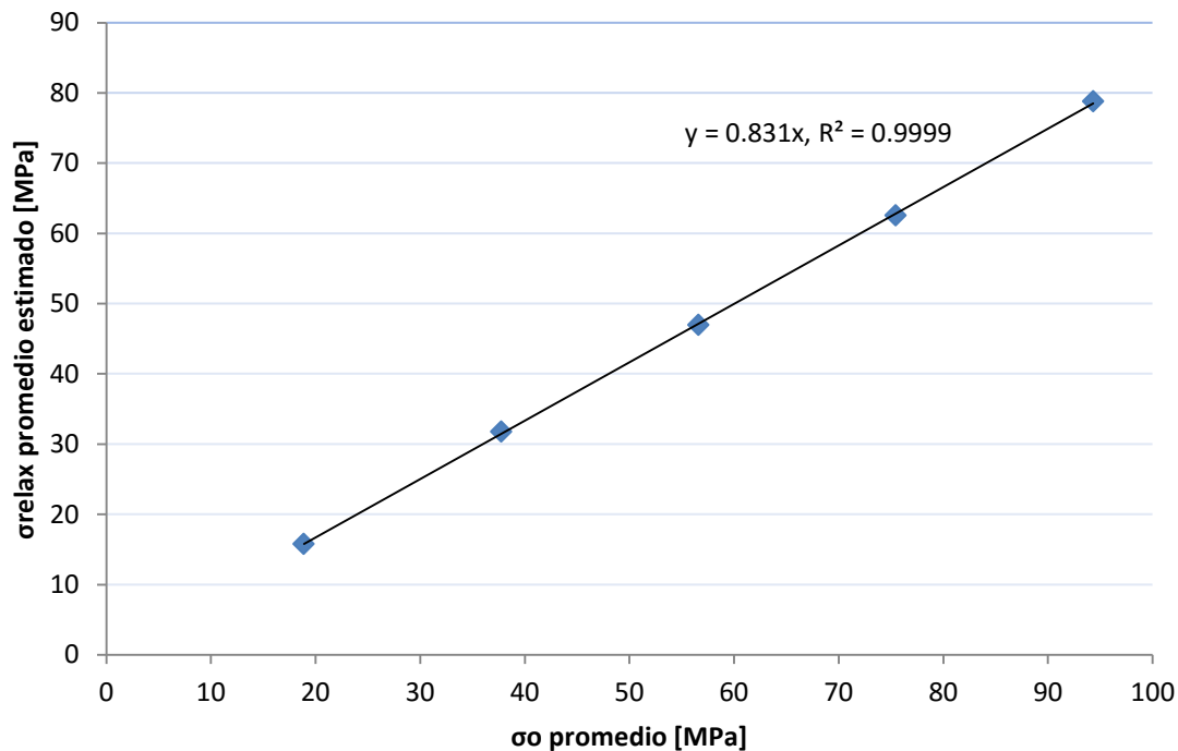
Figura 4.19 Gráfica de los valores promedio del esfuerzo de relajación estimado respecto a la respuesta a la precarga, se observa un comportamiento lineal con una r^2 = 0.9999 y un coeficiente de proporcionalidad de 0.831.
