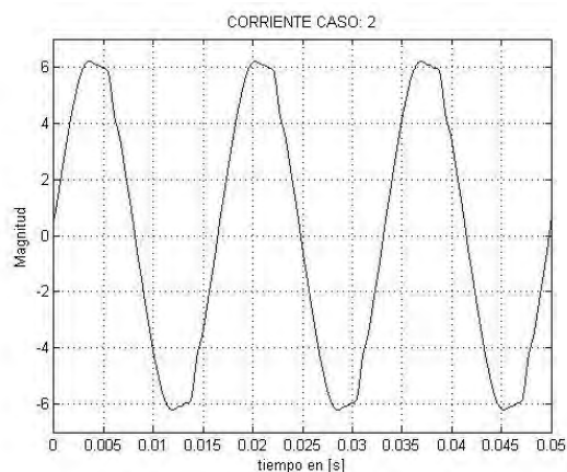
Figura 4.11 “Gráfica de corriente simulada caso 2”
