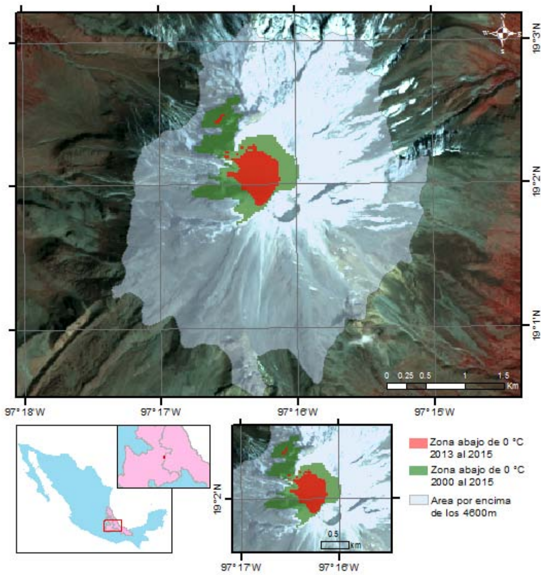
Figura V.5: Resultado del análisis de LST
