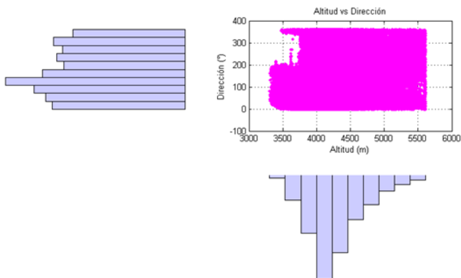
Figura IV.7: Distribución de pixeles del MDE representando la Altitud (m) vs Dirección de pendiente (°) mostrando sus histogramas de lado izquierdo y debajo de la gráfica
