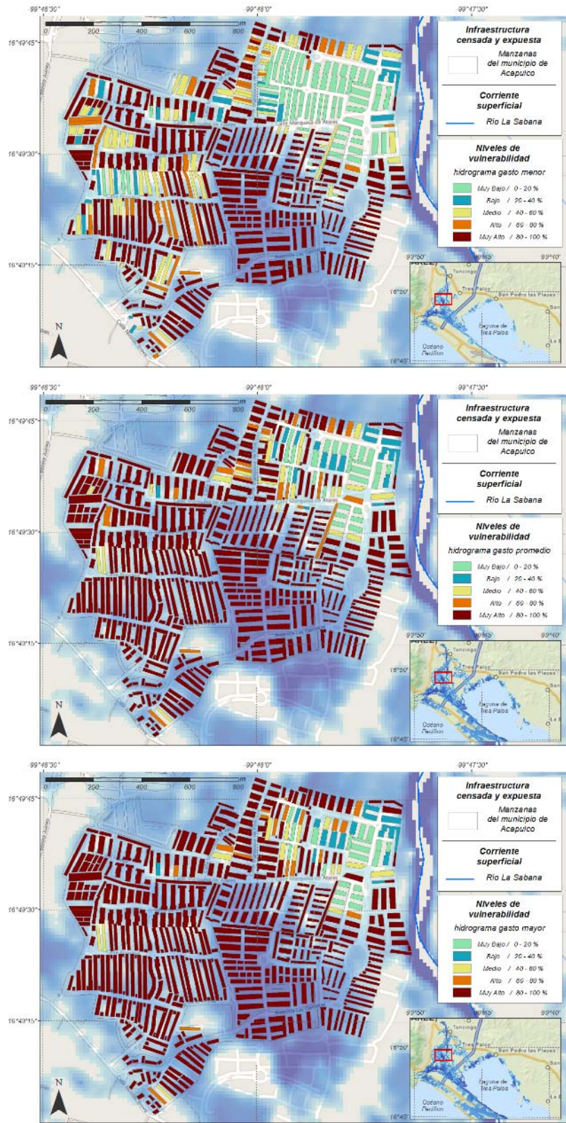
Figura 4.4 Niveles de vulnerabilidad en las delimitaciones de manzanas, producto de las simulaciones de los hidrogramas; a) mínimo, b) medio, c) máximo
