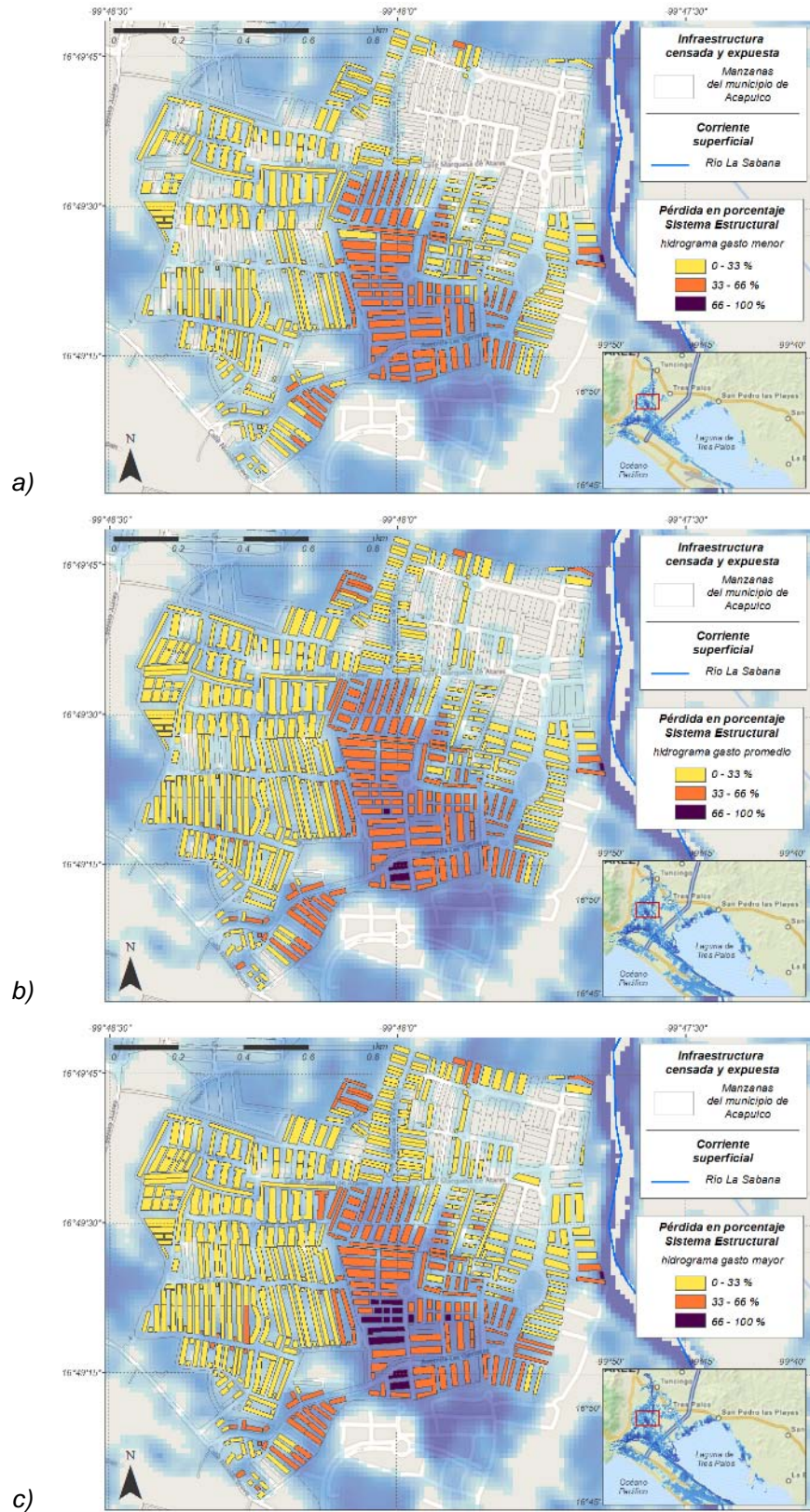
Figura 5.7 Porcentaje de pérdida en sistemas estructurales bajo las condiciones de caudales; a) menor, b) promedio, c) mayor
