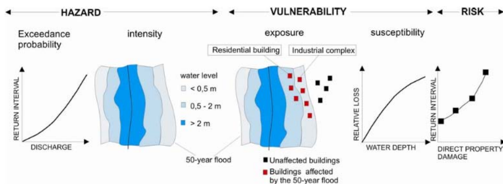
Figura 1.1 Riesgo por inundación; interacción de amenaza y vulnerabilidad, Fuente: Merz y Thielen (2004)
