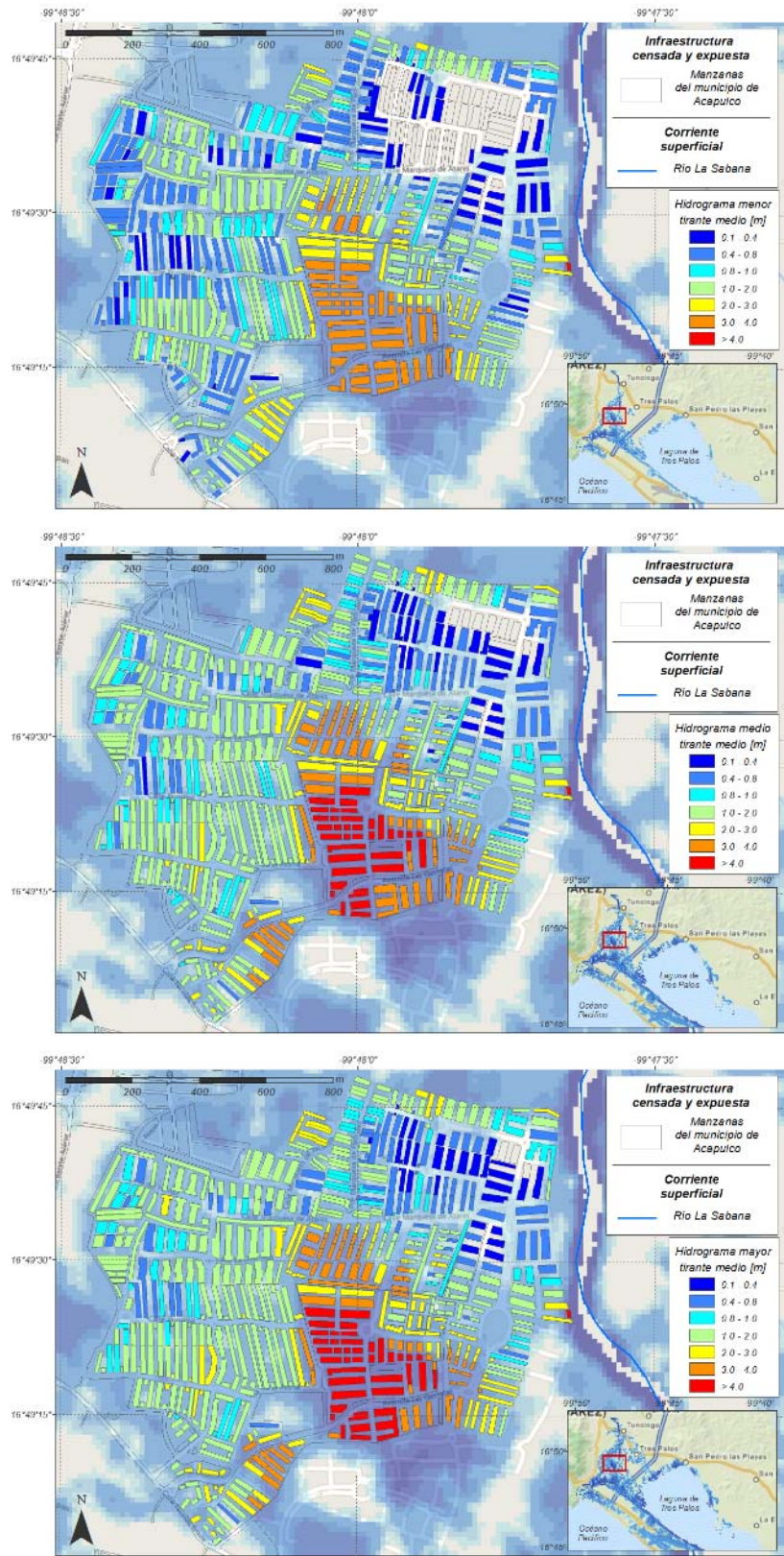
Figura 4.3 Tirantes medios inundables en las delimitaciones de manzanas, producto de las simulaciones de los hidrogramas; a) mínimo, b) medio, c) máximo
