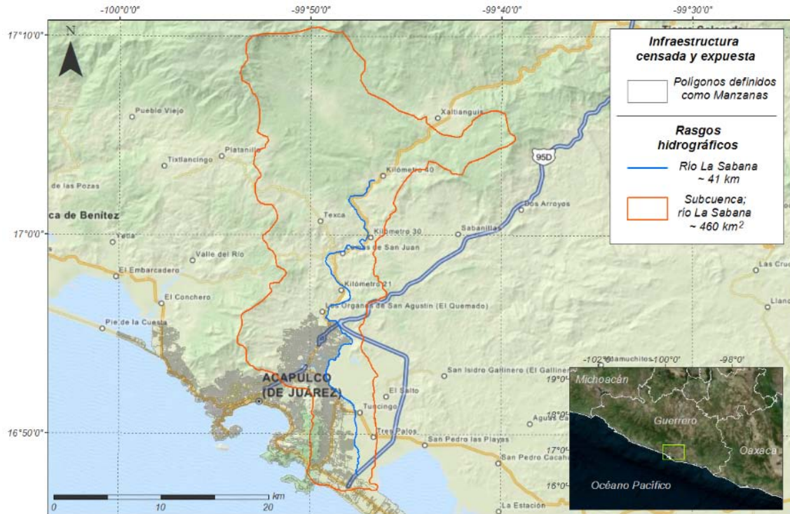
Figura 2.1 Configuración espacial de la zona de estudio, el cauce río La Sabana y la subcuenca de aportación hacia la infraestructura expuesta
