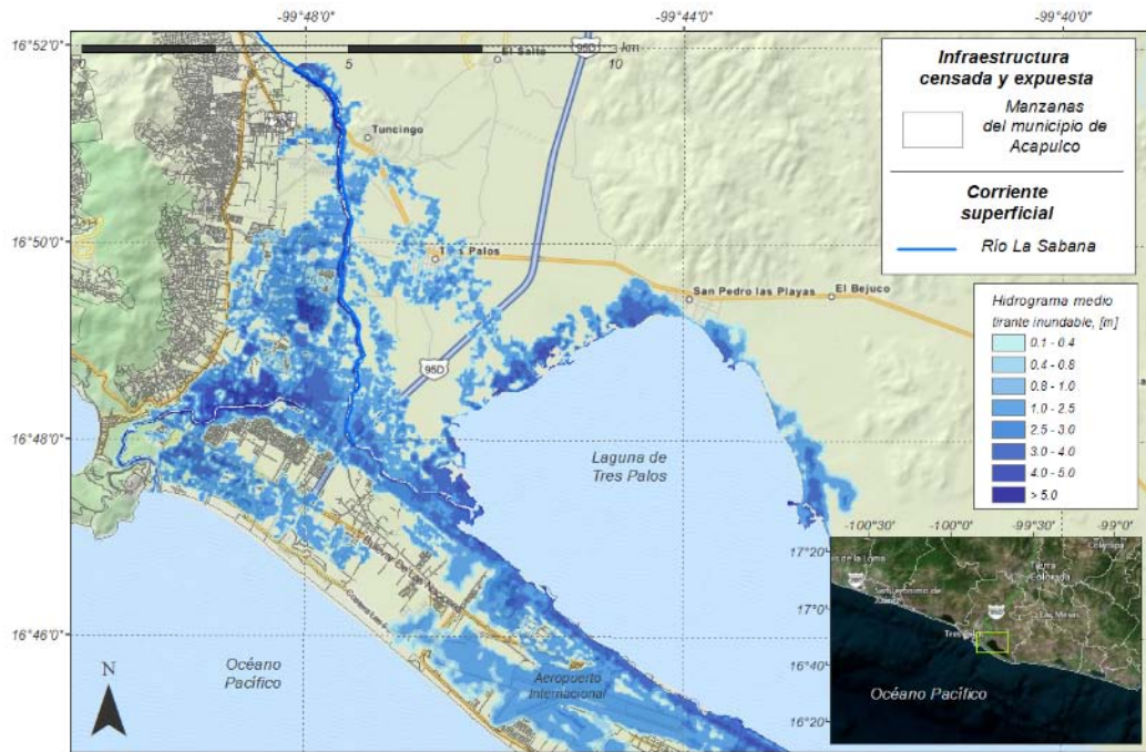
Figura 3.4 Inundación generada por la simulación hidrodinámica del hidrograma de condición de gasto promedio
