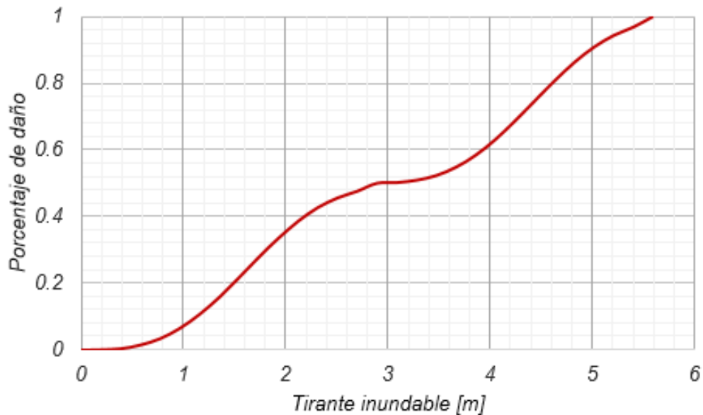
Figura 5.6 Función de vulnerabilidad para sistemas estructurales característicos de viviendas del conjunto habitacional
