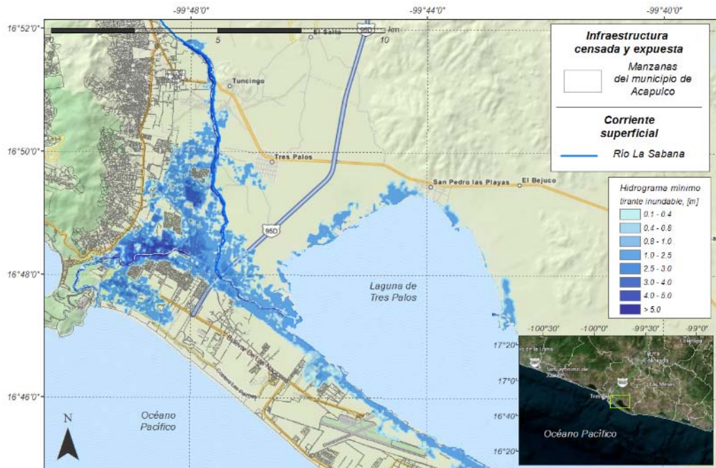
Figura 3.3 Inundación generada por la simulación hidrodinámica del hidrograma con menor condición de gasto
