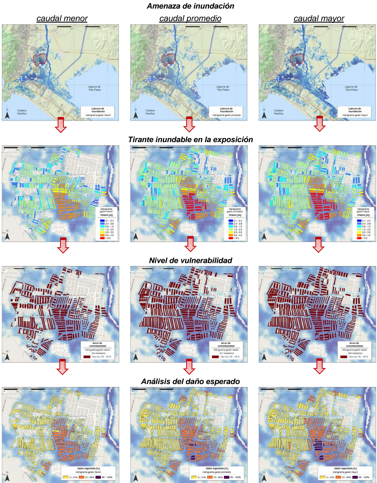
Figura 5.1 Esquema de trabajo desarrollado en el análisis y evaluación de daño
