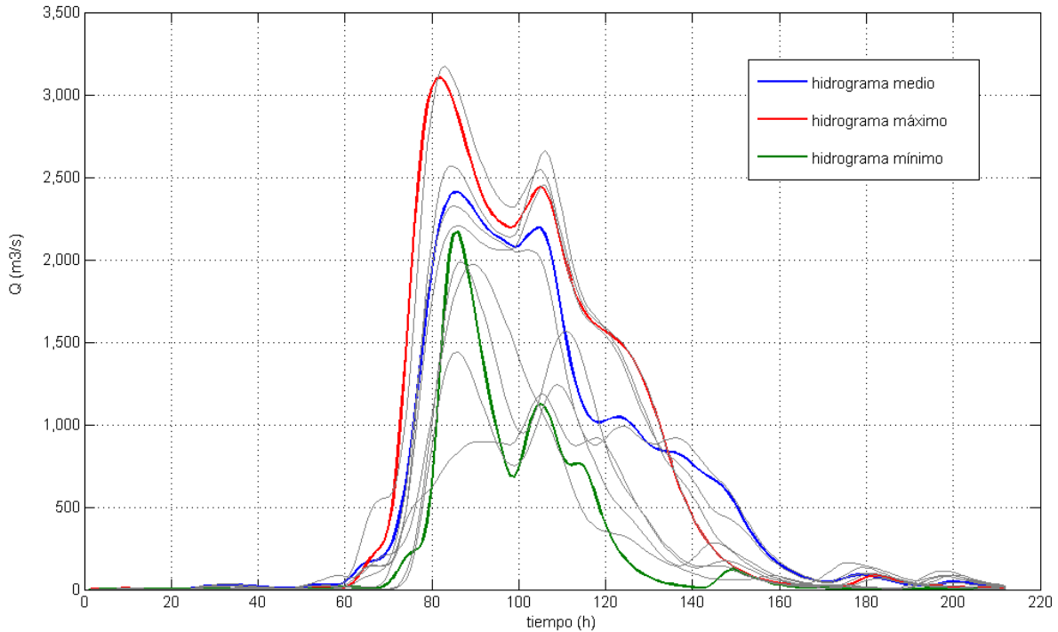
Figura 3.2 Hidrograma de descarga; río La Sabana
