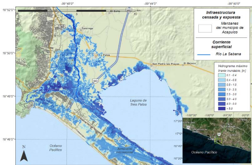
Figura 3.5 Inundación generada por la simulación hidrodinámica del hidrograma con mayor condición de gasto
