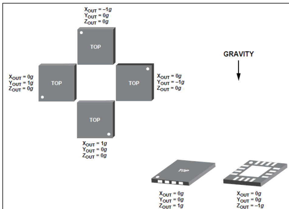
Figura 2.5. Comportamiento de los tres ejes en diferentes direcciones [6]
