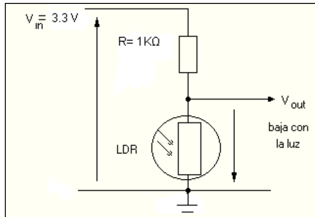
Figura 3.3.1 Circuito Divisor de Voltaje para la obtención de luminosidad
