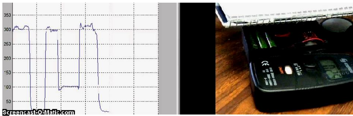
Figura 3.15.1. Comparación del valor dado por el luxómetro y el dispositivo respectivamente
