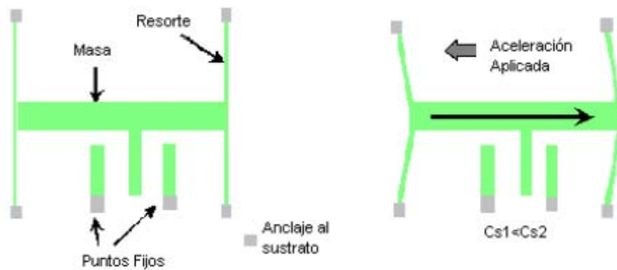
Figura 2.2. Funcionamiento de un acelerómetro capacitivo[5]
