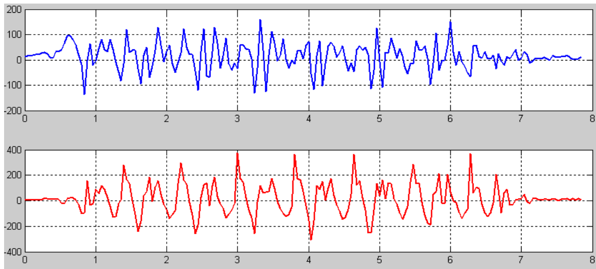
Figura 3.10. Prueba corriendo sujeto 2 [Volts VS segundos]
