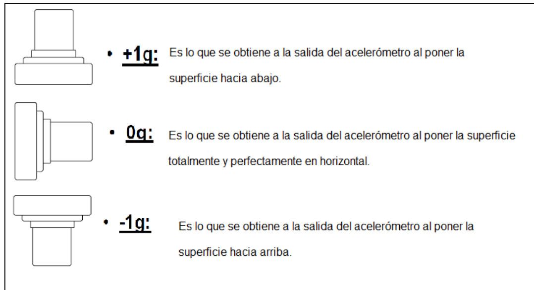
Figura 2.3. Demostración del comportamiento de las “g” según la posición del acelerómetro
