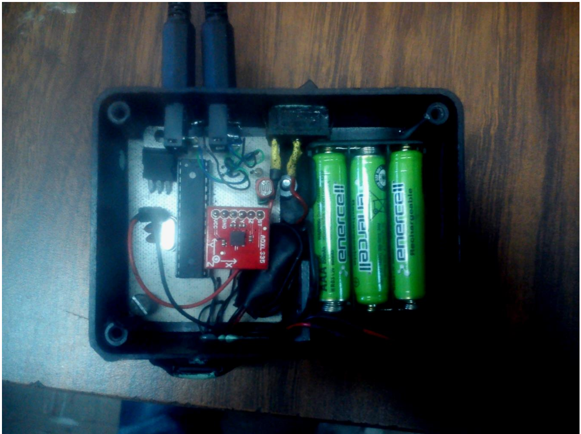
Figura 3.16. Dispositivo diseñado para medir actividad física y luminosidad
