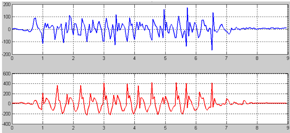
Figura 3.9. Prueba corriendo sujeto 3 [Volts VS segundos]
