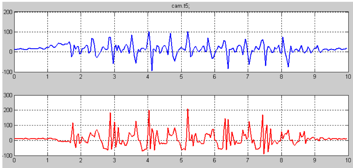
Figura 3.8. Grafica azul (eje x) y roja (eje y) de la prueba caminando de sujeto 2 [Volts VS segundos]
