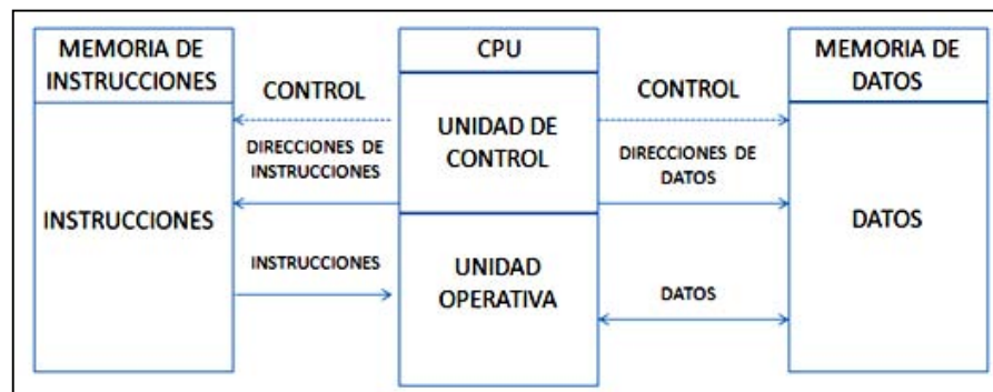
Figura 2.9. Arquitectura Harvard
