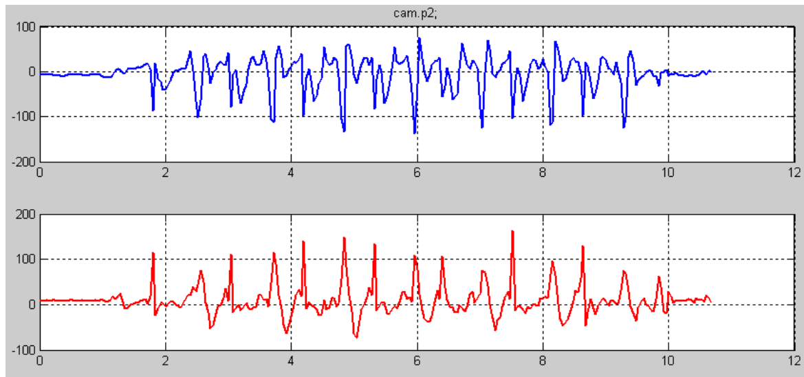
Figura 3.7. Grafica azul(eje x) y roja(eje y) prueba caminando de sujeto 3 [Volts VS segundos]
