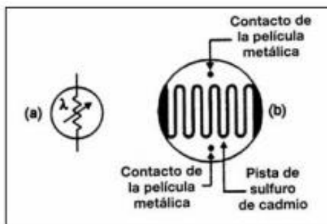
Figura 2.7. Composición de fotorresistencia
