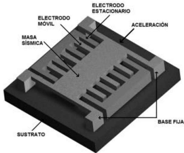
Figura 2.1. Estructura de un acelerómetro para un eje.[4]
