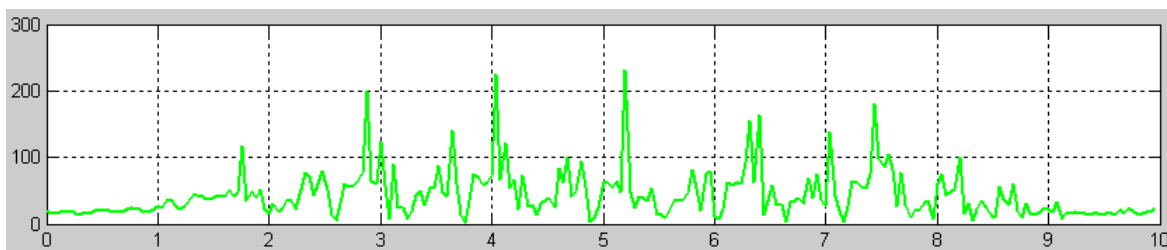
Figura 3.14. Suma vectorial de las componentes “x” y “y” en la prueba caminando sujeto 2
