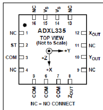
Figura 2.4. Pines Acelerómetro ADXL335[6]
