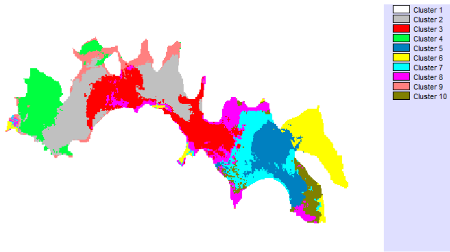
Figura 5.22 Clasificación fina (15 de junio de 2014)
