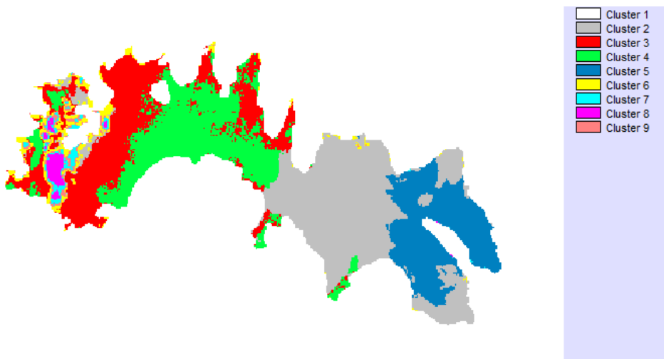
Figura 5.29 Clasificación gruesa (08 de diciembre de 2014)
