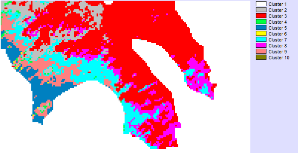
Figura 6.6 Zona C (11 de marzo de 2014)
