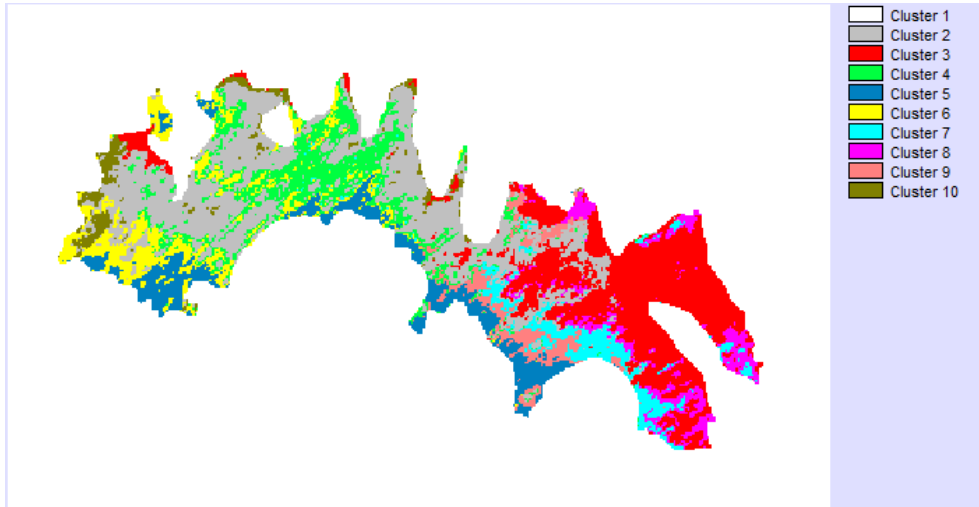
Figura 5.18 Clasificación fina (11 de marzo de 2014)
