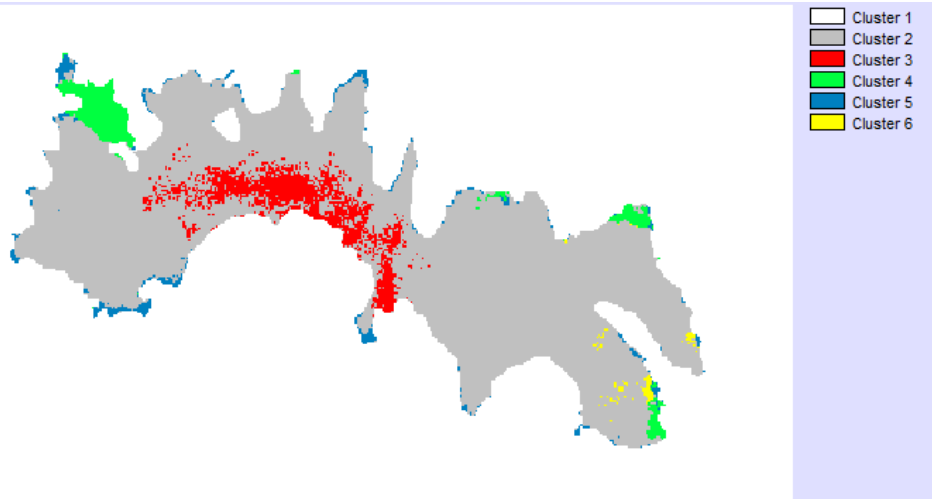
Figura 5.28 Clasificación fina (06 de noviembre de 2014)
