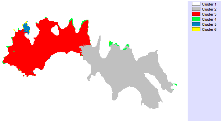
Figura 5.15 Clasificación gruesa (22 de enero de 2014)
