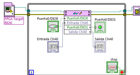
(b) Diagrama de bloques básico
