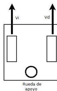
Figura 1.11 Configuración diferencial
