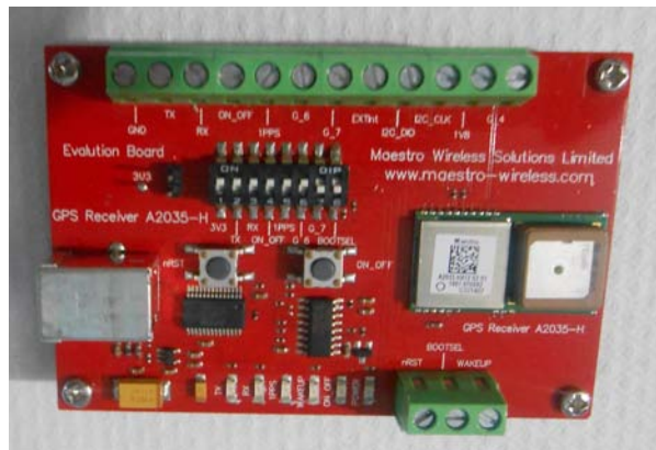
Figura 2.23 Módulo GPS EVA2035-H.
