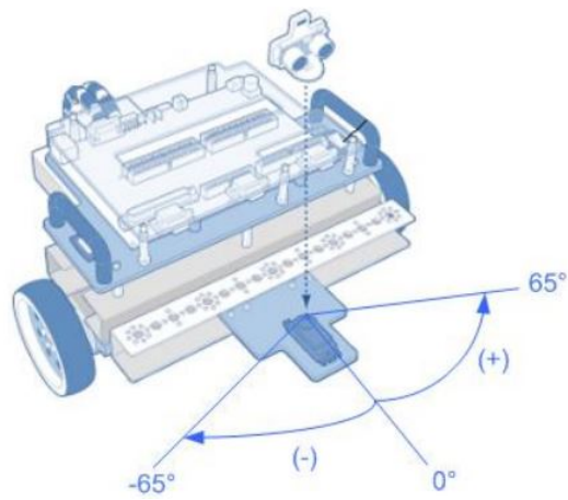
Figura 2.16 [Rango de barrido del sensor ultrasónico] Recuperado de: [18]
