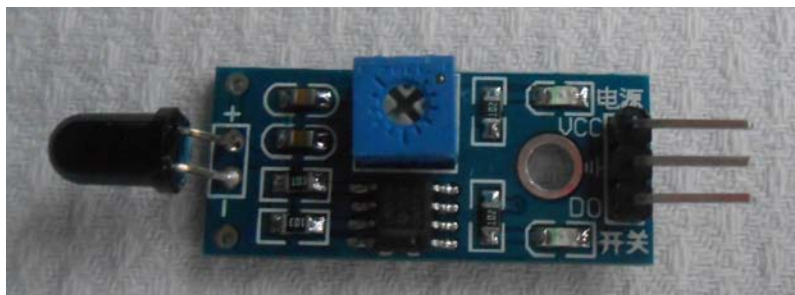
Figura 2.22 Módulo detector de flama.
