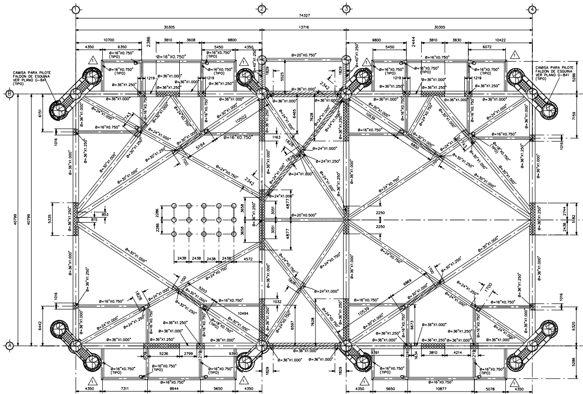
PLANTA ESTRUCTURAL EN ELEV. (-115.950 M.)
