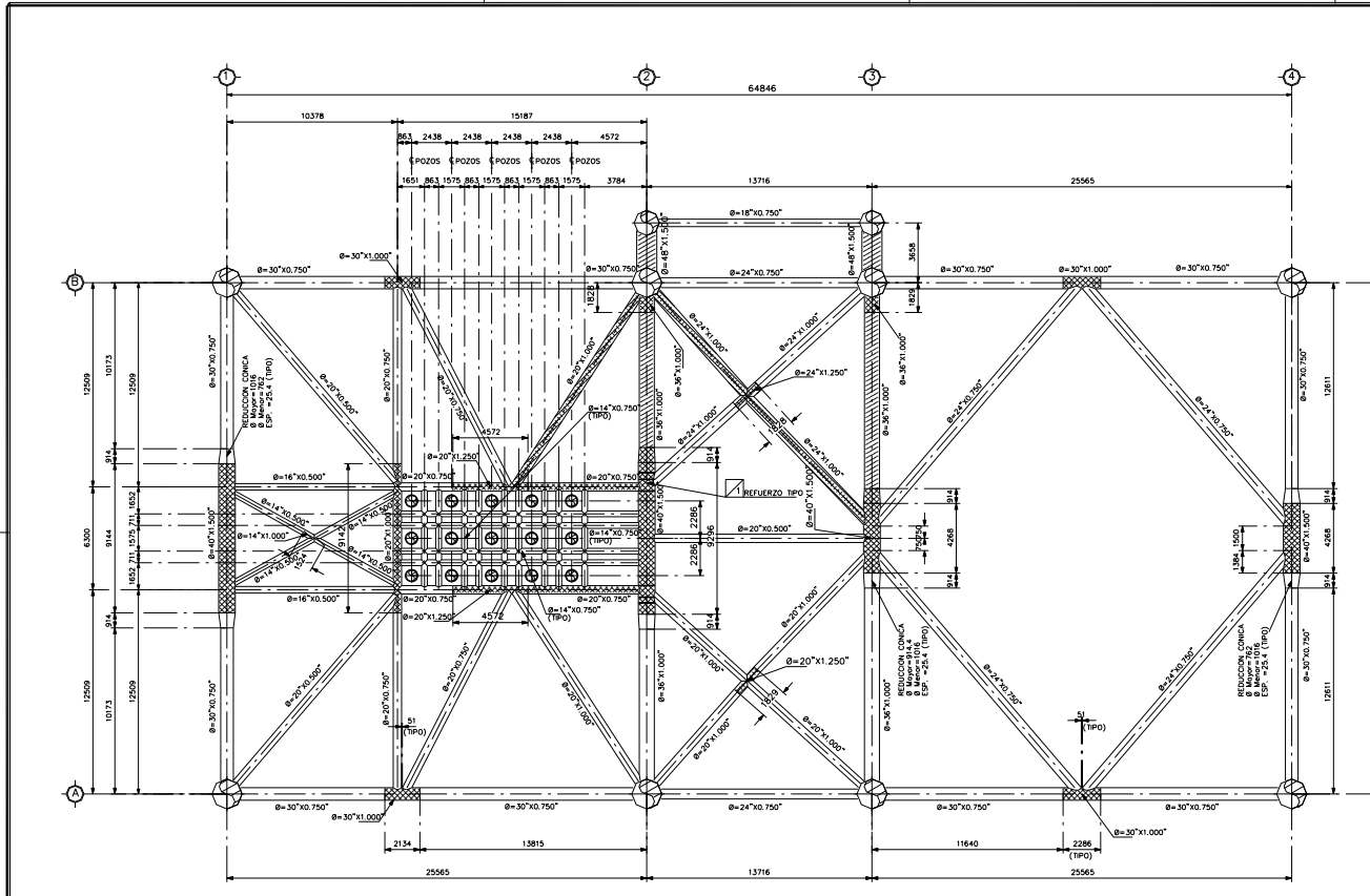
PLANTA ESTRUCTURAL EN ELEV. (-)63.093 M. ESC. 1: 120
