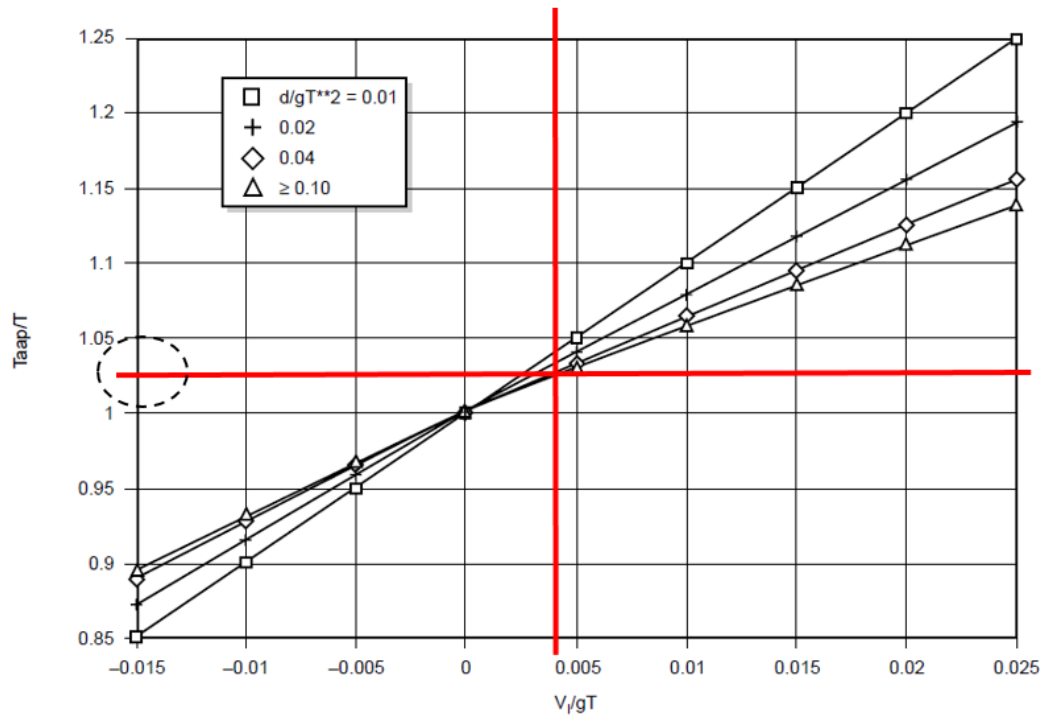
Figura 5.25. Cálculo del periodo aparente para condiciones de Operación
