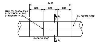
(D-1) ELEVACION
