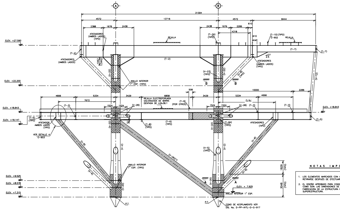
ELEVACION MARCO EJE 4
