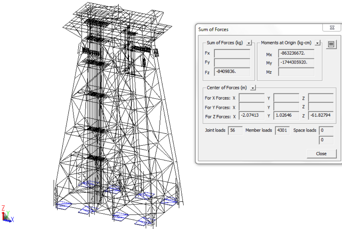
Figura 5.1. Peso propio
