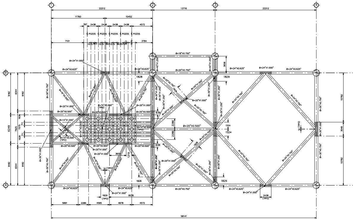
PLANTA ESTRUCTURAL EN ELEV. (-)36.271 M.
