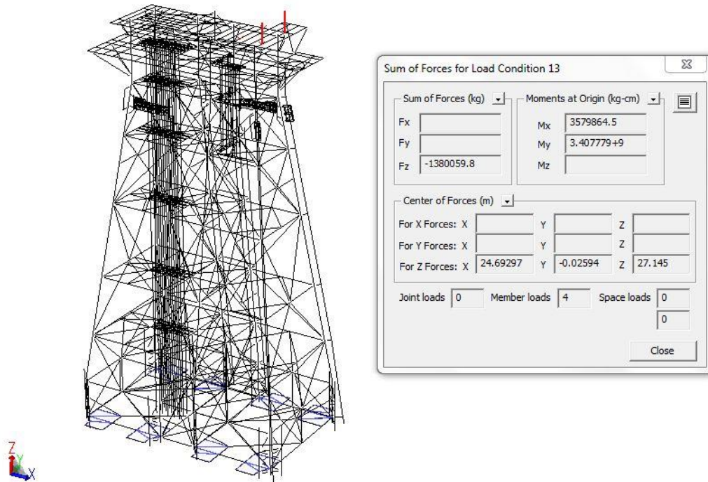
Figura 5.13. Carga de modulo habitacional (Operación)
