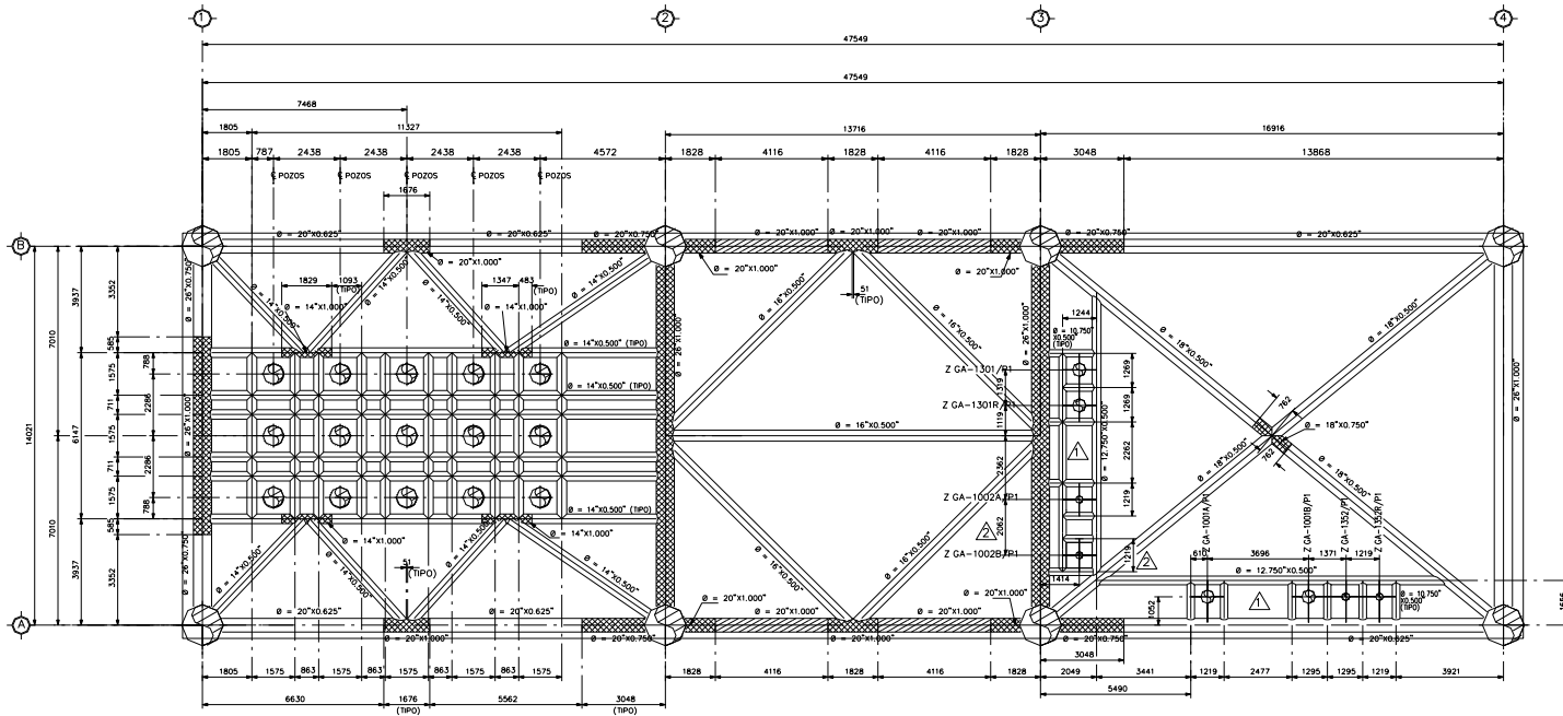
PLANTA ESTRUCTURAL EN ELEV. (+)6.096 M. ESC. 1: 75
