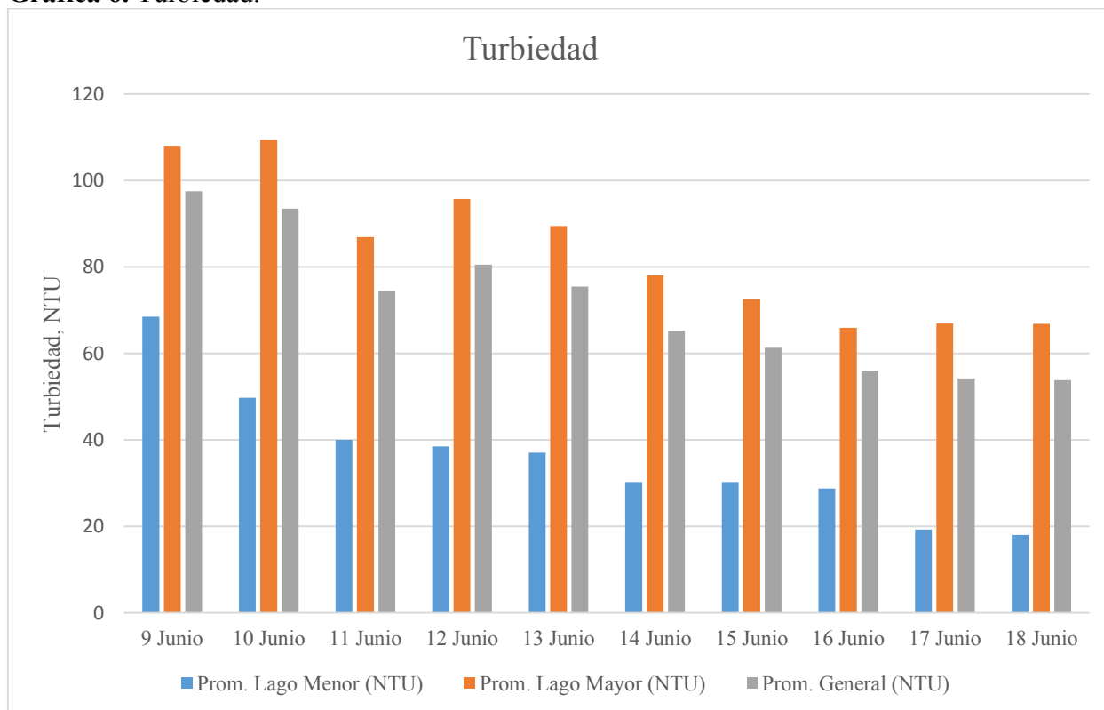
Gráfica 6. Turbiedad.
