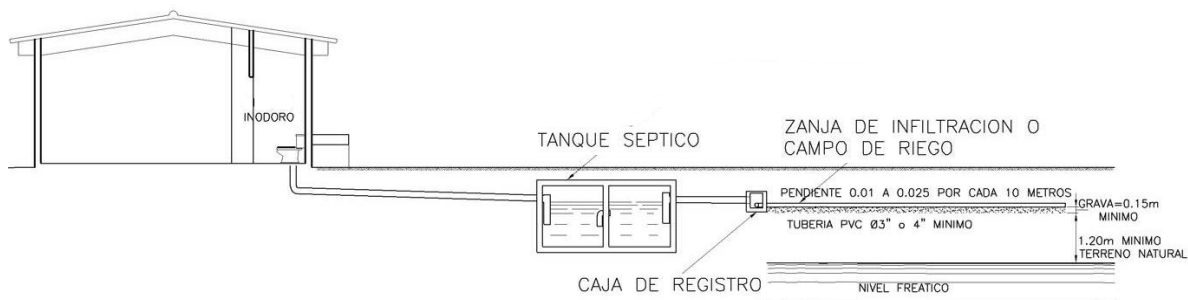
Figura 3.22 Tanque séptico con zanja de infiltración.
