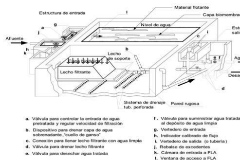
Figura 2.12 Esquema del filtro lento de arena.
