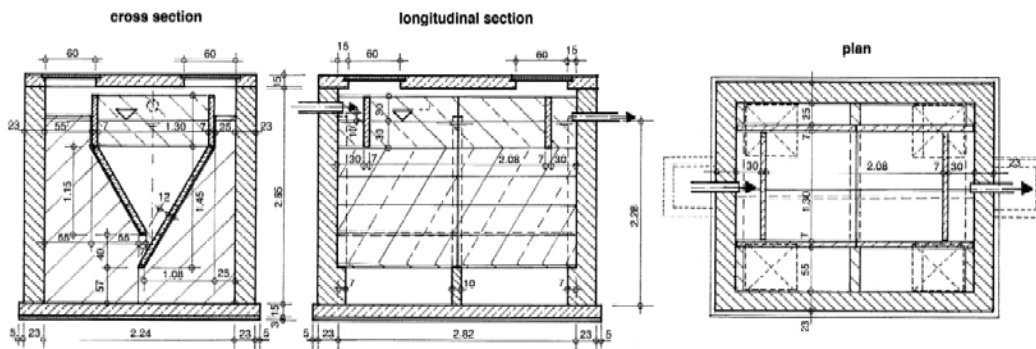
Figura 4.28 Tanque Imhoff para 25 m³ de agua residual doméstica por día.
