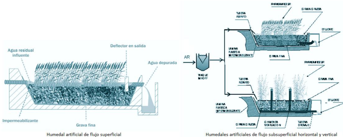
Figura 3.9 Tipos básicos de humedales artificiales.
