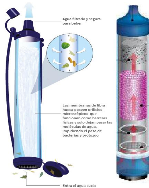
Figura 2.13 Esquema del LifeStraw®.
