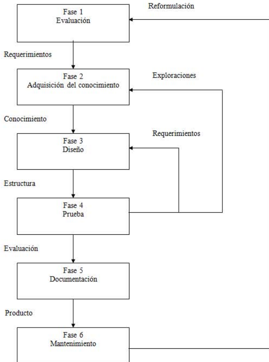
Figura 3.2. Metodología de Ingeniería del Conocimiento de John Durkin [24].
